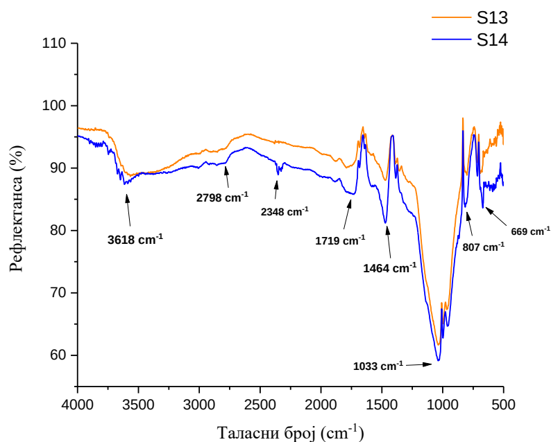
Слика 30. DRIFT анализа узорака S13 и S14
