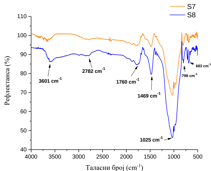
Слика 27. DRIFT анализа узорка S7 и S8
