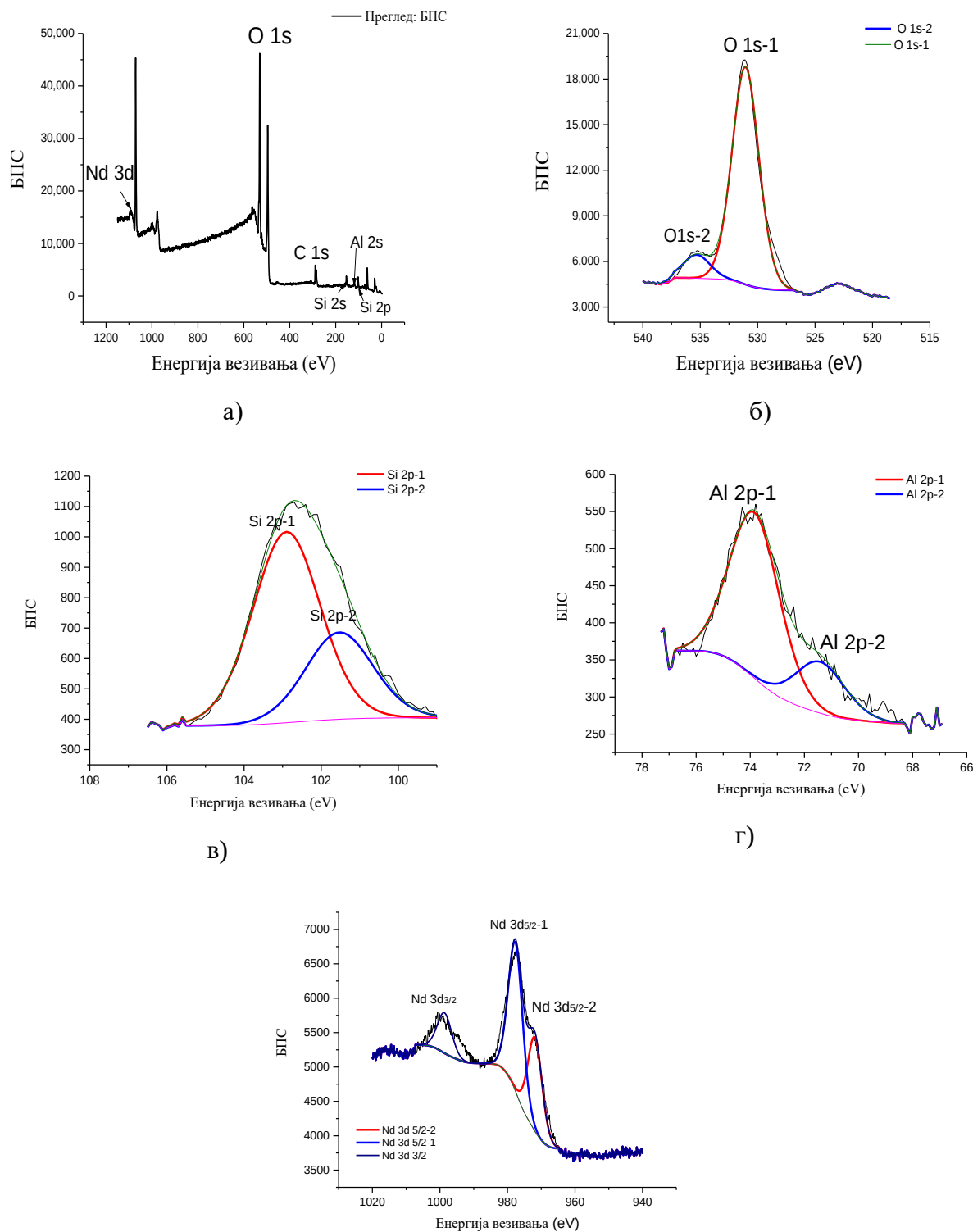
Слика 14. XPS анализа узорка S1 а) прегледни спектар, б) O1s, в) Si2p, г) Al2p, д) Nd3d
