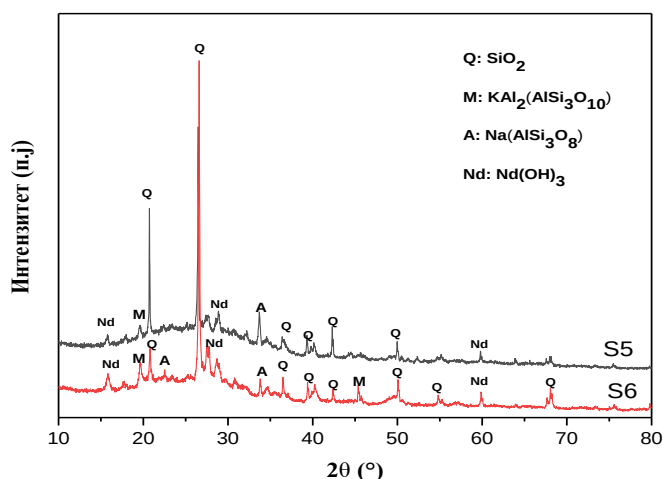
Слика 20. Рендгенски дифрактограми праха узорака S5 и S6
