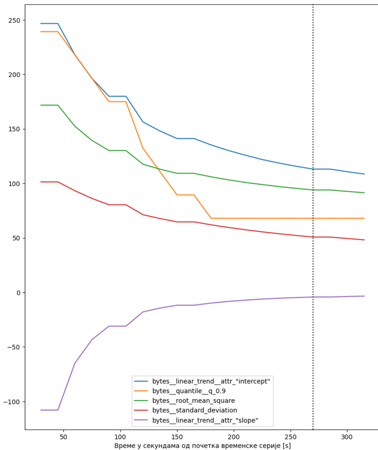
Слика 18: График зависности најбитнијих одлика у времену за бојнећ саобраћај - 2
