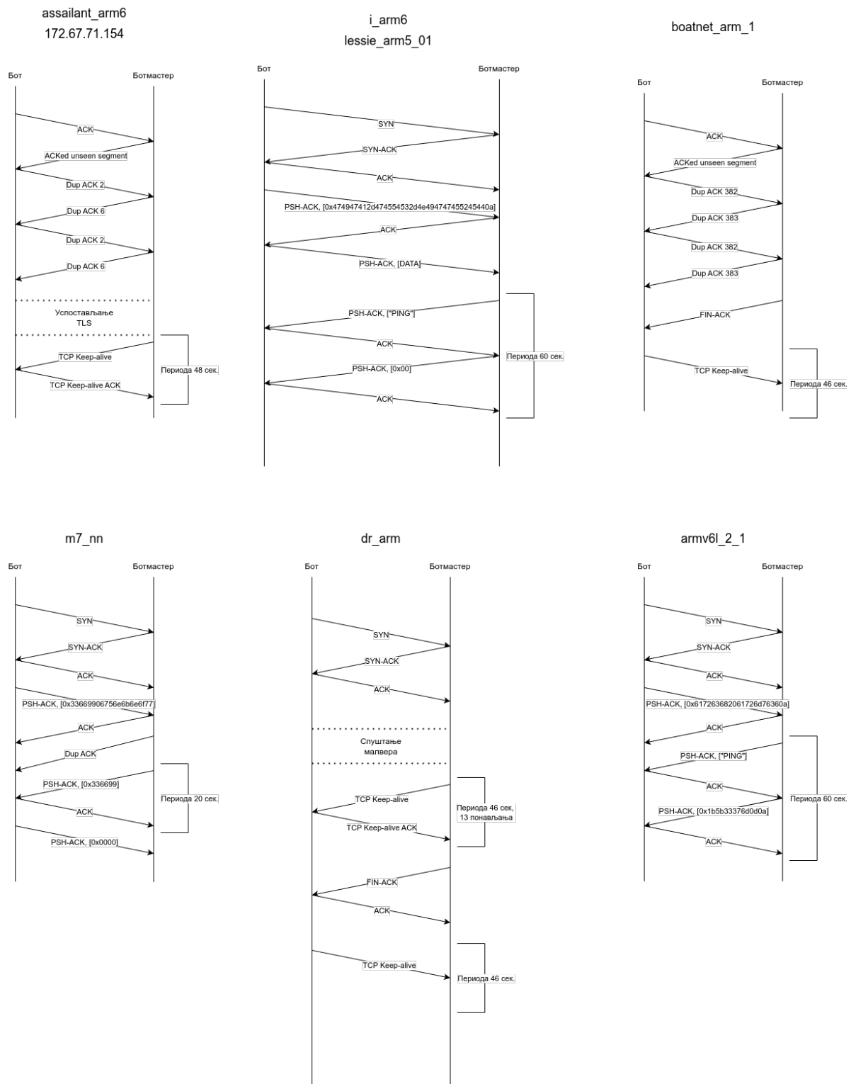
Слика 13: Бојнети саобраћај малвер узорака прикућених у периоду 2022-2023 - 2
