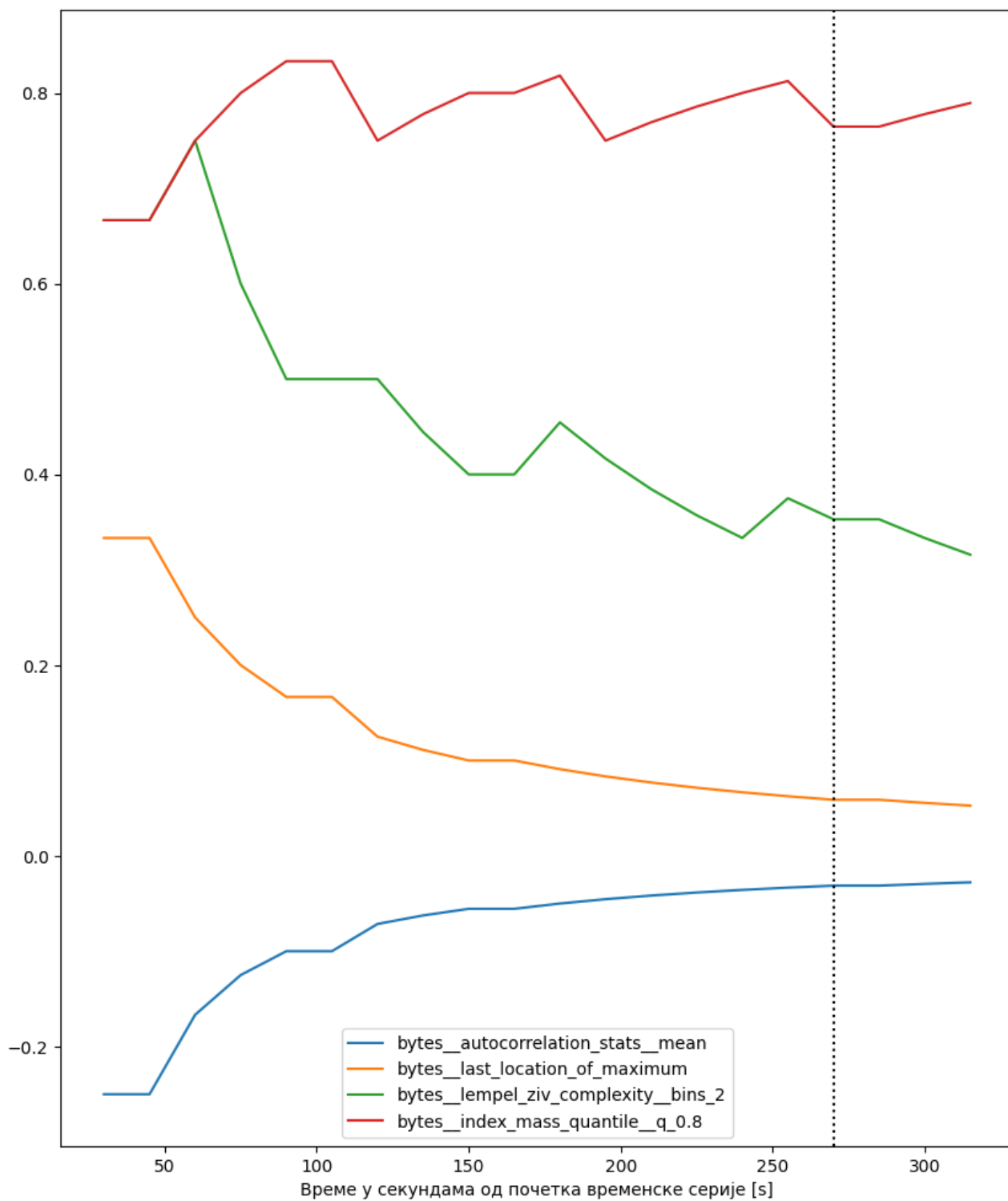
Слика 17: График зависности најбитнијих одлика у времену за бојнећ саобраћај - 1
