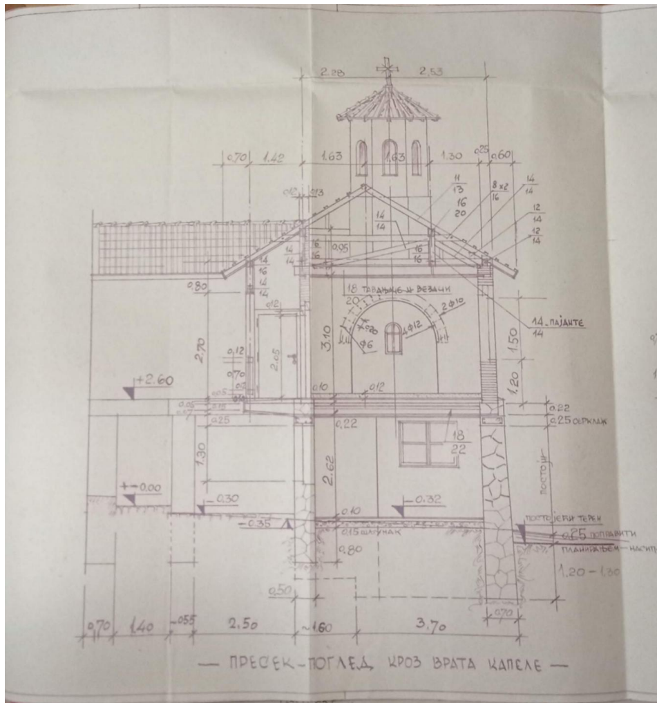
Прилог 27. Конак бр. 2, Пресек – поглед кроз врата капеле, (архива Епархије рашко-призренске).
