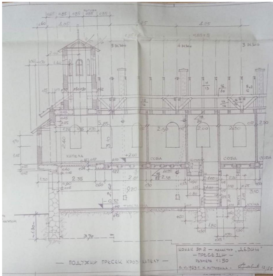
Прилог 26. Конак бр. 2, Подужни пресек кроз капелу, (архива Епархије рашко-призренске).
