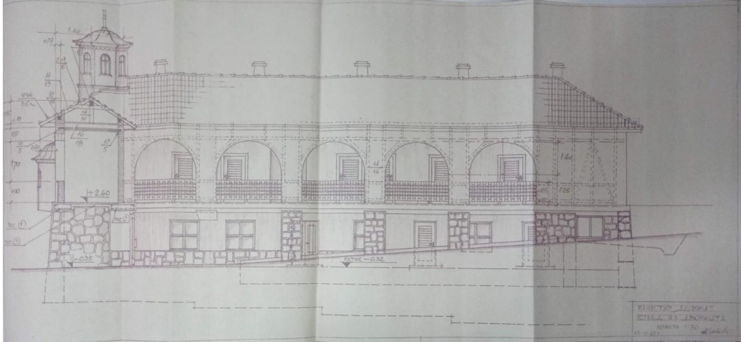
Прилог 28. Конак бр. 2, Поглед из дворишта , (архива Епархије рашко-призренске).
