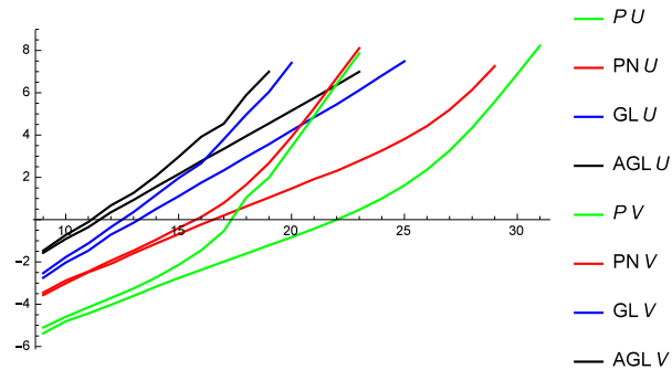
Слика 3.5: Логаритам времена извршавања израженог у милсекундама за U_n и V_n за све четири групе.
