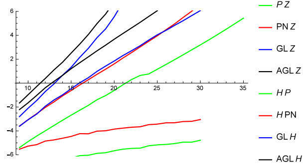
Слика 3.7: Логаритам времена извршавања у милисекундама при одређивању циклусног индекса и табеле H за све четири групе.
