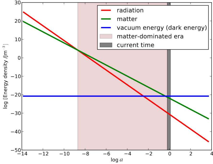
Slika 1.2: Različite epohe evolucije Univerzuma. Linijama su predstavljene promene gustine energije sa faktorom skaliranja, a . Crvenom linjom je predstavljena gustina energije zračenja, zelenom materije, a plavom tamne energije. Osenčeni region predstavlja epohu u kojoj dominira materija. Slika je preuzeta iz rada Dirisa (2012).
