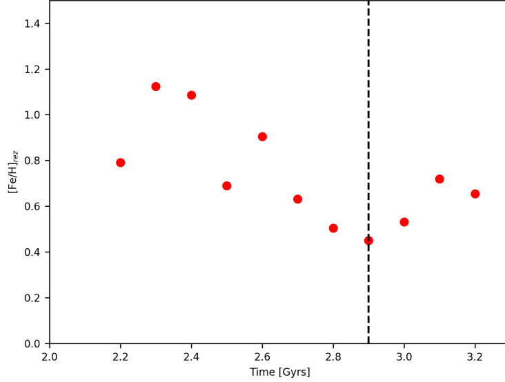
Slika 4.13: Rezidualne metaličnosti za različite vremenske trenutke. Naš model sugerše da je najbolje poklapanje simulirane i posmatrane raspodele metaličnosti posle 2,9 milijardi godina od početka simulacije.
