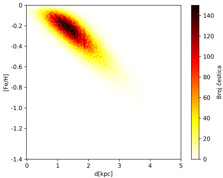
Slika 4.9: Raspodela čestica po metaličnosti za različite radijalne udaljenosti u patuljastoj galaksiji (od koje je nastao GSS) na početku simulacija u d - [\text{Fe}/\text{H}] ravni, gde je d radijalna udaljenost od centra galaksije.
