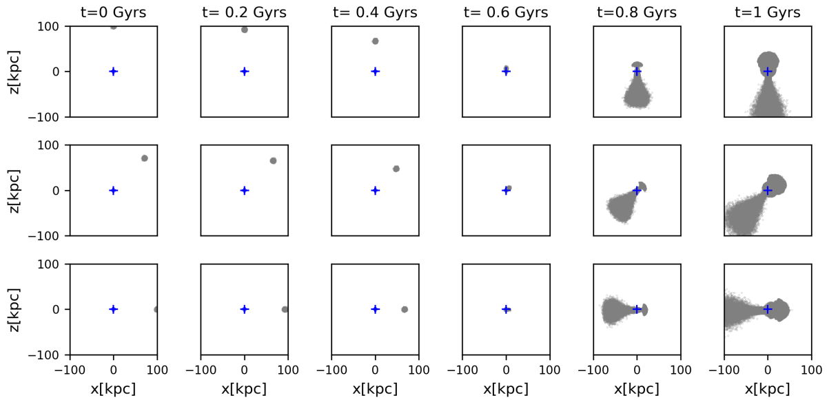
Slika 3.1: Istorija sudara spiralne i dSph patuljaste galaksije, od početka simulacije do 1 milijarde godina. Sive tačke predstavljaju čestice patuljaste galaksije, a plavi krstić je centar diska spiralne galaksije. Čestice spiralne galaksije su izuzete sa grafika, radi bolje vidljivosti promene strukture patuljaste. Gornji red reprezentuje sudar u slučaju S0 scenarija sudara, srednji red S1 i donji red S3 scenario.
