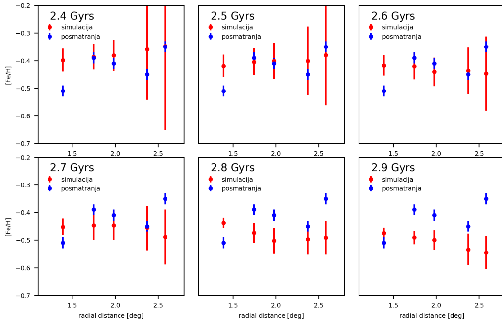
Slika 5.9: Raspodela metaličnosti za posmatračka polja iz NE ljuske za interval između 2,4 i 2,9 milijardi godina. Plave tačke su posmatračke vrednsoti iz Escala et al. (2022), a crvene su simulirane vrednosti metaličnosti.
