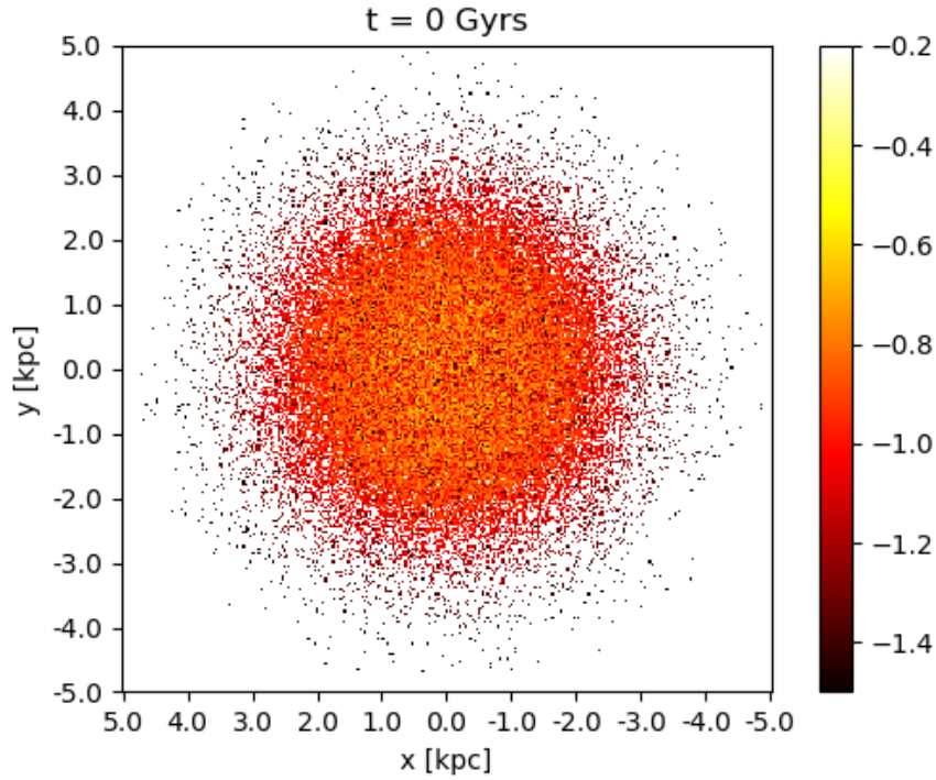
Slika 4.8: Mapa početne raspodele metaličnosti u patuljastoj galaksiji.
