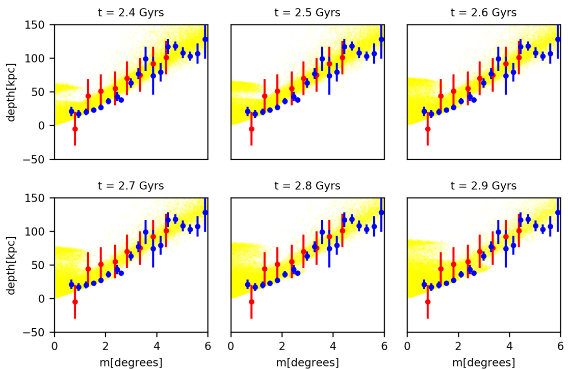
Slika 4.2: Udaljenosti od centra M31 u funkciji koordinate duž toka, m , dobijene iz naše simulacije N-tela (žute tačke). Crvene tačke sa intervalima pouzdanosti su posmatranja iz McConnachie et al. (2003), dok su plave tačke posmatrački podaci iz Conn et al. (2016). Paneli predstavljaju različite trenutke sudara između 2,4 i 2,9 milijardi godina.
