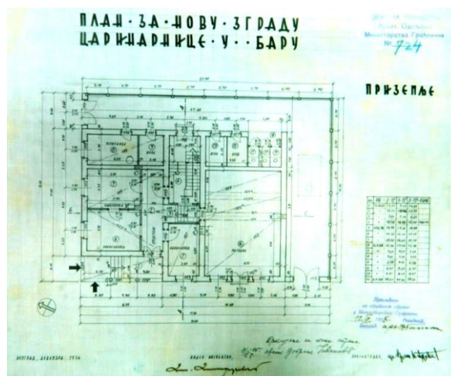
Прилог 132, 1-3 Зграда Царинарнице у Бару, План, арх. Драган Гудовић, 1934, изгледи, пресјеци и основа приземља (Архив Југославије-Београд, Збирка планова Архитектонског одељења Мин. грађевина КЈ бр. 724)
