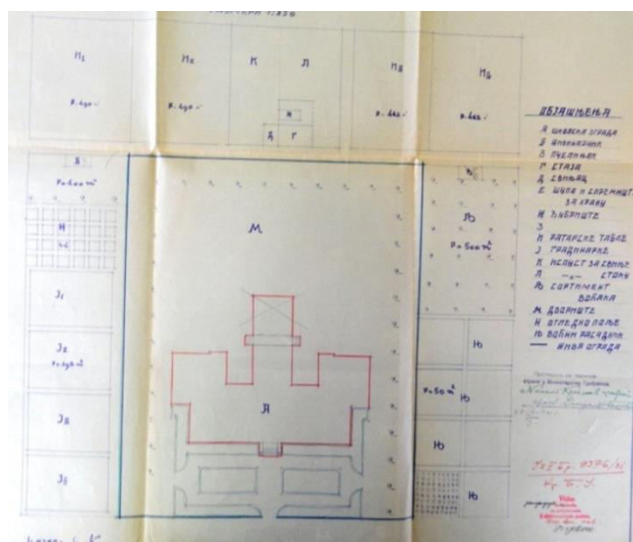
Прилог 107 Пројекат за четвороразредну основну школу, арх. Петар Вукотић и Иван Латишев, 1931, основа првог спрата; Прилог 108 Ситуациони и културни план за основне школе, 1931. (ДАЦГ, Фонд Краљевске Банске управе Зетске бановине-Техничко одјељење, Ф50-Планови-основне школе-разни типови)
