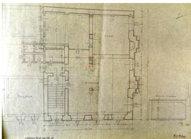
Прилог 35, 1-4 Кућа Марка Милошевића-хотел „Њујорк“ на Цетињу, План, перспективни изглед, пресјек А-В, основа приземља, основа првог спрата (ДАЦГ, Фонд Краљевске Банске управе Зетске бановине-Техничко одјељење, Ф 28 - Срез Цетињски)
