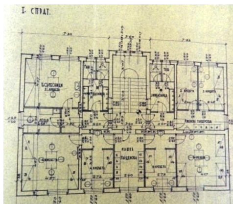
Прилог 137, 1-3 Зграда Берзе рада и радничког склоништа у Шкаљарима у Котору, Пројекат, инж. Вилим Хофман, 1936, изгледи, основа приземља и првог спрата (ДАЦГ, Фонд Краљевске Банске управе Зетске бановине-Техничко одјељење, Ф 16-Срез Котор)
