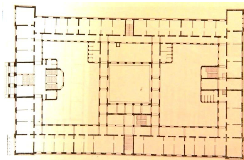
Прилог 83-2 Основа приземља Банске палате (D.Martinović-U.Martinović, Cetinje. Spomenici arhitekture, Cetinje 1980)
