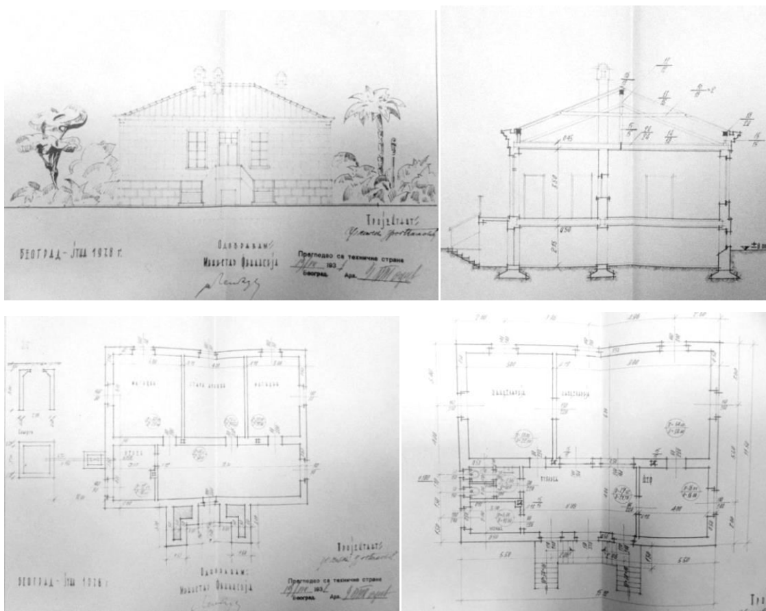
Прилог 125, 1-4 Зграда Пореске управе у Бару, Пројекат, арх. Драг. Плаовић, 1938, главни изглед, пресјек, основе сутерена и приземља (Архив Југославије-Београд, Фонд Министарства грађевина бр. 62, општа архива - фасцикла бр. 1554)
