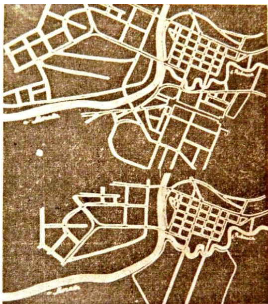
Прилог 218 План Подгорице, инж. Владимир Ворман, 1886. (Zdravko Ivanović, Vormanov plan Podgorice 1886. године, Архитектура-Урбанизам, 68-69, Београд 1971)
