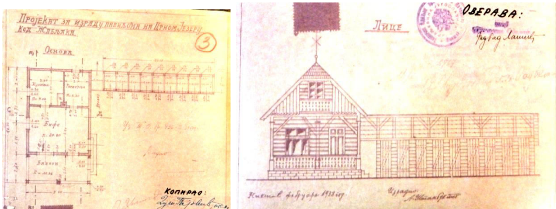
Прилог 168, 1-2 Павиљон на Црном језеру код Жабљака, Пројекат, техн. Андрија Штамбук, 1938, основа и изглед (ДАЦГ, Фонд Краљевске Банске управе Зетске бановине-Техничко одјељење, Ф 44 - Срез Шавник)
