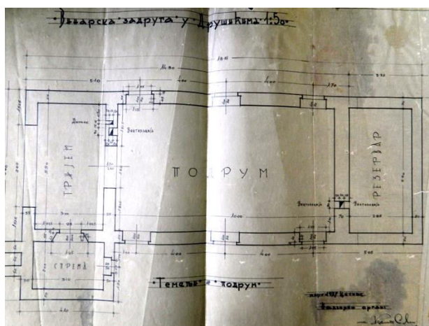
Прилог 146 Нацрт темеља и подрума Винарске задруге у Друшићима (ДАЦГ, Фонд Краљевске Банске управе Зетске бановине-Техничко одјељење, Ф 28 - Срез цетињски)
