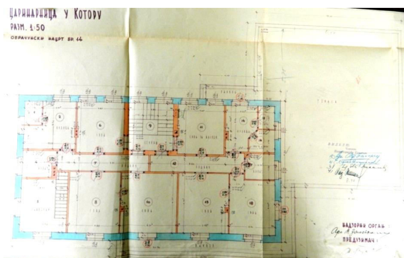
Прилог 131-1 Царинарница у Котору, Пројекат арх. Милана Злоковића, 1935, преглед столарије Прилог 131-2 Царинарница у Котору, Пројекат-обрачунски нацрт бр. 14, цртеж основе (ДАЦГ, Фонд Краљевске Банске управе Зетске бановине-Техничко одјељење, Ф 16-Срез Котор)
