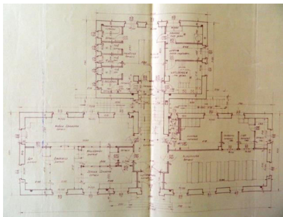
Прилог 136, 1-3 Јавна берза рада у Подгорици, План, 1936, изглед прочеља, основа приземља, пресјек (ДАЦГ, Фонд Краљевске Банске управе Зетске бановине -Техничко одјељење, Ф 24-Срез подгорички)
