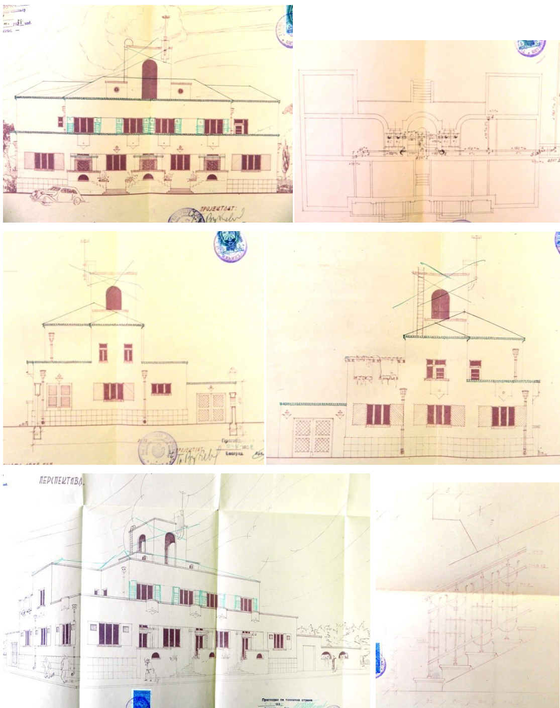
Прилог 134, 1-6 Царинарница у Риједи Црнојевића, Пројекат, инж. Глигорије Вукчевић, 1938, главни изглед, основа приземља, попречни изглед из дворишта, попречни изглед из улице, перспективни изглед, детаљ степенишне ограде (ДАЦГ, Фонд Кр. Банске управе Зетске бановине-Техничко одјељење, Ф34-Срез Цетиње)
