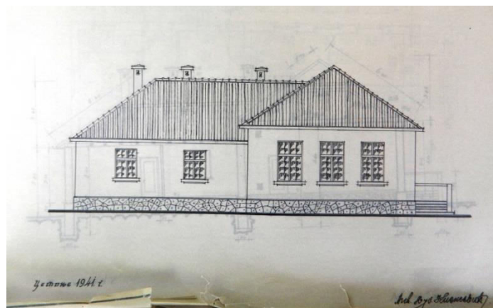
Прилог 110- 1 План за основну школу у_ , арх. Љубомир Кнежевић, 1941. (ДАЦГ,Фонд Краљевске Банске управе Зетске бановине-Техничко одјељење,Ф50-Планови-основне школе-разни типови)
