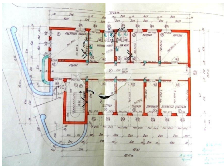
Прилог 176, 1-2 Зграда поште у Херцег Новом, План, арх. Драган Гудовић, 1935-36, основа приземља и ситуација; основа међуспрата
