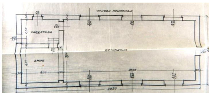
Прилог 182, 1-3 Соколска вјежбаоница у Каменом, Нацрт, 1936, изглед са стране и основа приземља (ДАЦГ, Фонд Краљевске Банске управе Зетске бановине-Техничко одјељење, Ф 17-Срез Котор)
