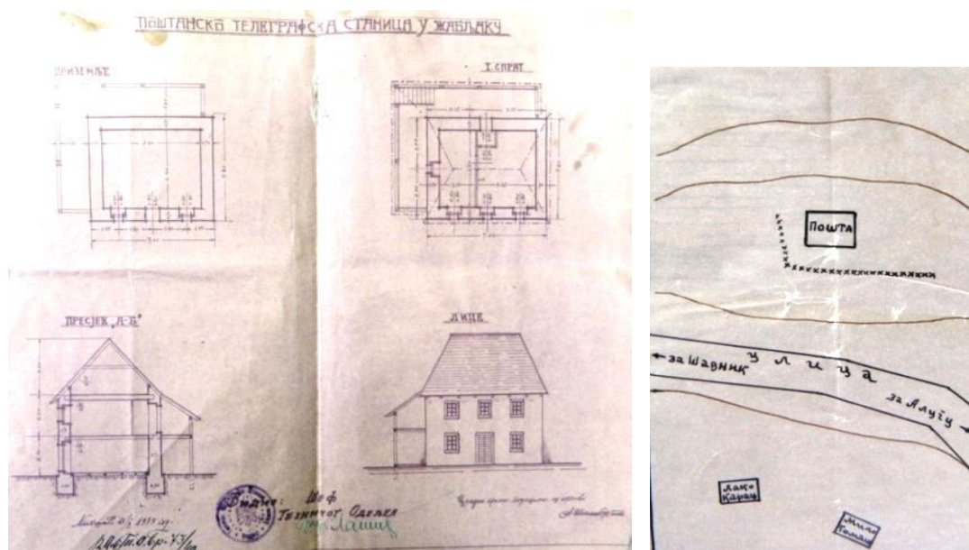
Прилог 178, 1-2 Поштанско-телеграфска станица на Жабљаку, План зграде и цртеж ситуације, техн. Андрија Штамбук, 1939. (ДАЦГ, Фонд Краљевске Банске управе Зетске бановине-Техничко одјељење, Ф 15-Срез колашински)
