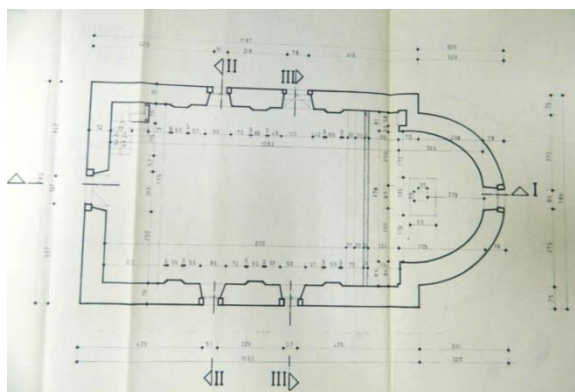
Прилог 56, 1-2 Црква св. Ђорђа у Гусињу, изглед и цртеж основе ( www.velika.me/index.php?page_id=537&lang=srpski ) (Пројекат санације из 1988. године, УЗКД Црне Горе)
