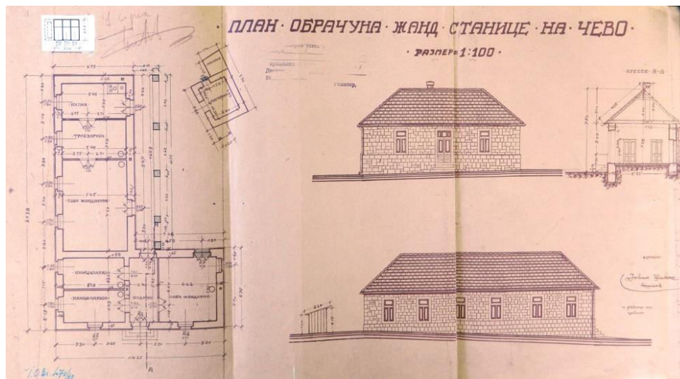
Прилог 5 Жандармеријска станица на Чеву, План обрачуна из 1928. (ДАЦГ, Фонд Краљ. Банске управе Зетске бановине -Техничко одјељење, Ф 29-Срез цетињски)
