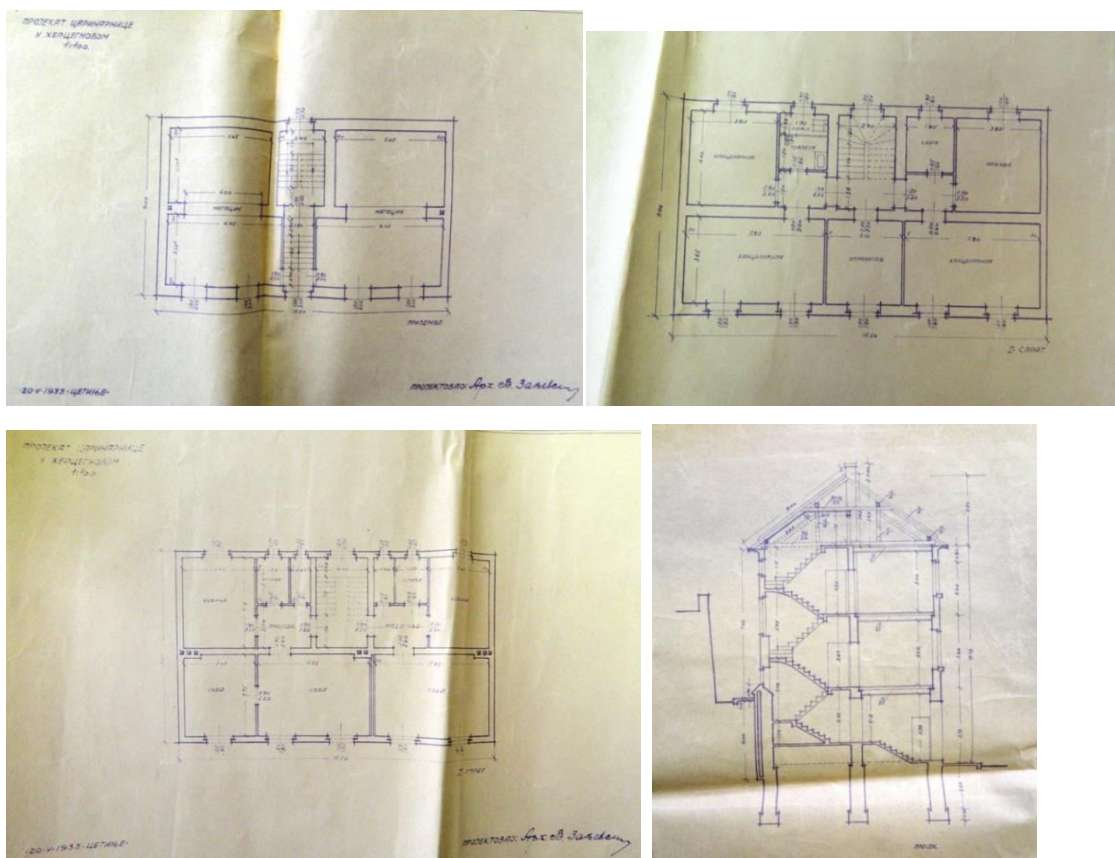
Прилог 128, 1-4 Царинарница у Херцег Новом, Пројекат, арх.Виктор Заљевскиј, 1933, основе приземља, првог и другог спрата и пресјек (ДАЦГ, Фонд Краљевске Банске управе Зетске бановине-Техничко одјељење, Ф 16-Срез Котор)
