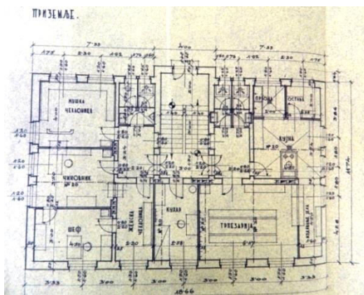
Прилог 137, 1-3 Зграда Берзе рада и радничког склоништа у Шкаљарима у Котору, Пројекат, инж. Вилим Хофман, 1936, изгледи, основа приземља и првог спрата (ДАЦГ, Фонд Краљевске Банске управе Зетске бановине-Техничко одјељење, Ф 16-Срез Котор)
