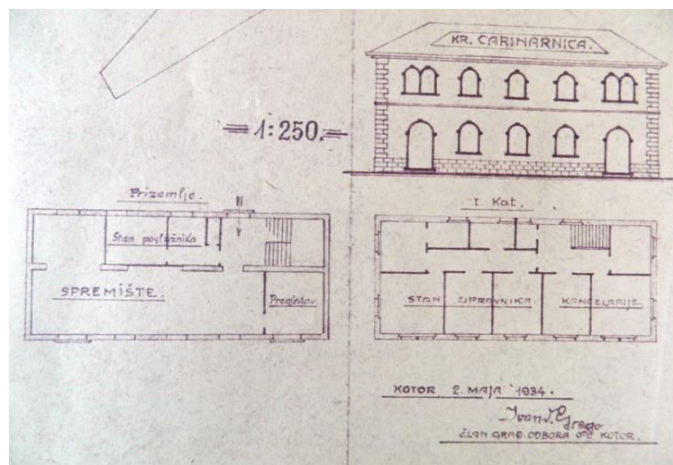
Прилог 129 План Царинарнице у Котору, Иван Грегo, 1934. (ДАЦГ, Фонд Краљевске Банске управе Зетске бановине-Техничко одјељење, Ф 16 Срез Котор)
