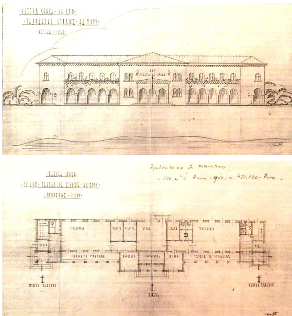
Прилог 185, 1-2 Идејна скица за Дом Јадранске страже на мору, арх. Ђ. Б., главна фасада, основа приземља (ДАЦГ, Фонд Краљевске Банске управе Зетске бановине-Техничко одјељење, Ф 4-Срез барски)
