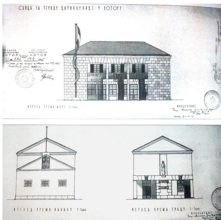
Прилог 130, 1-2 Царинарница у Котору, Пројекат Милана Злоковића из 1935. и недатирана скица пројекта (Ljiljana Blagojević, Itinerari. Moderna i Mediteran..., Beograd 2015)
