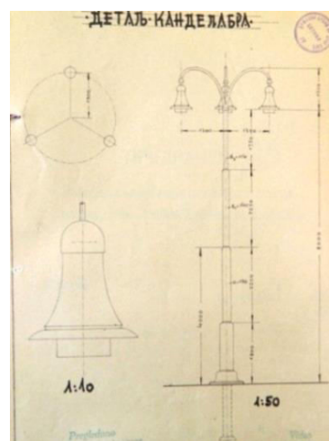
Прилог 83, 4-5 Пројекат за паркирање терена пред Банском палатом и детаљ канделабра, техн. Косто Лигутић, 1935. (ДАЦГ, Фонд Краљевске Банске управе Зетске бановине-Техничко одјељење, Ф 35 - Срез Цг.)
