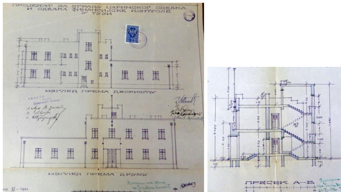
Прилог 126, 1-5 Зграда Царинског одјелка и одјелка Финансијске контроле у Тузима, Пројекат, арх. Димитрије М. Леко, 1931, основе призеља и спрата, изгледи са стране, изгледи према дворишту и друму и пресјек (ДАЦГ, Фонд Краљевске Банске управе Зетске бановине -Техничко одјељење, Ф 24-Срез подгорички)
