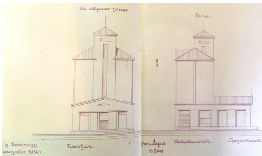
Прилог 145 Силос у Беранама, Пројекат, 1939, изгледи
