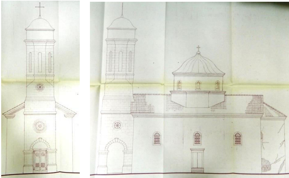
Прилог 253, 1-2 Црква св. Недеље у Јошици, изгледи западне и јужне фасаде (Главни пројекат санације цркве св. Недеље-Јошице, мај 1987, Управа за заштиту културних добара)
