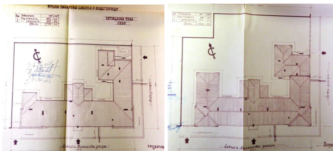
Прилог 105- 5 Мушка занатска школа у Подгорици, ситуациони план, 1938.
