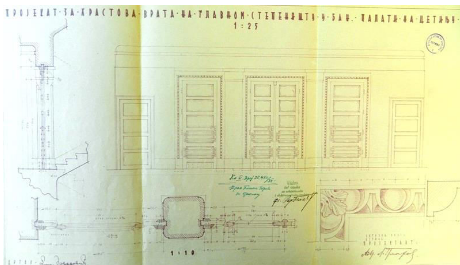
Прилог 83, 6-7 Пројекат за храстова врата на главном степеништу, арх. Лав Плахов, 1935, два изгледа (ДАЦГ, Фонд Краљ. Банске управе Зетске бановине-Техничко одјељење, Ф 35 - Срез Цт.)
