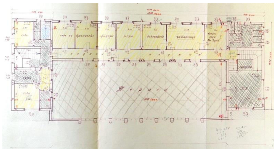
Прилог 89, 1-3 Официрски дом на Цетињу, Пројекат, арх. Мил. Вражалић, главни изглед, основа приземља и основа првог спрата (ДАЦГ, Фонд Кр. Банске управе Зетске бановине-Техничко одјељење, Ф32- Срез Цетиње)
