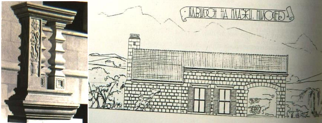
Прилог 194, 5-7 Вила „Топлиш“ на Милочеру, Пројекат, арх. Рајко Татић, 1938, изгледи фасада; балкон-детал; павиљон на плажи (Саша Михајлов, Рајко М. Татић (1900-1979), Београд 2013)
