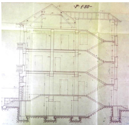
Прилог 95, 5-10 Мања зграда чиновничких станова на Цетињу, Пројекат, арх. Гојко Тодић, 1930, главни изглед, основе сутерена, приземља и првог спрата, пресјек 1:50, пресјек 1:100 (ДАЦГ, Фонд Кр. банске управе Зетске бановине-Техничко одјељење, Ф 63-Чиновнички станови-Цетиње)
