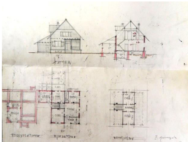
Прилог 165 Кућица за чувара шуме на путу Колашин-Биоградско језеро, скица, техн. Косто Лигутић, 1932. (ДАЦГ, Фонд Краљевске Банске управе Зетске бановине-Техничко одјељење, Ф 15-Срез колашински)
