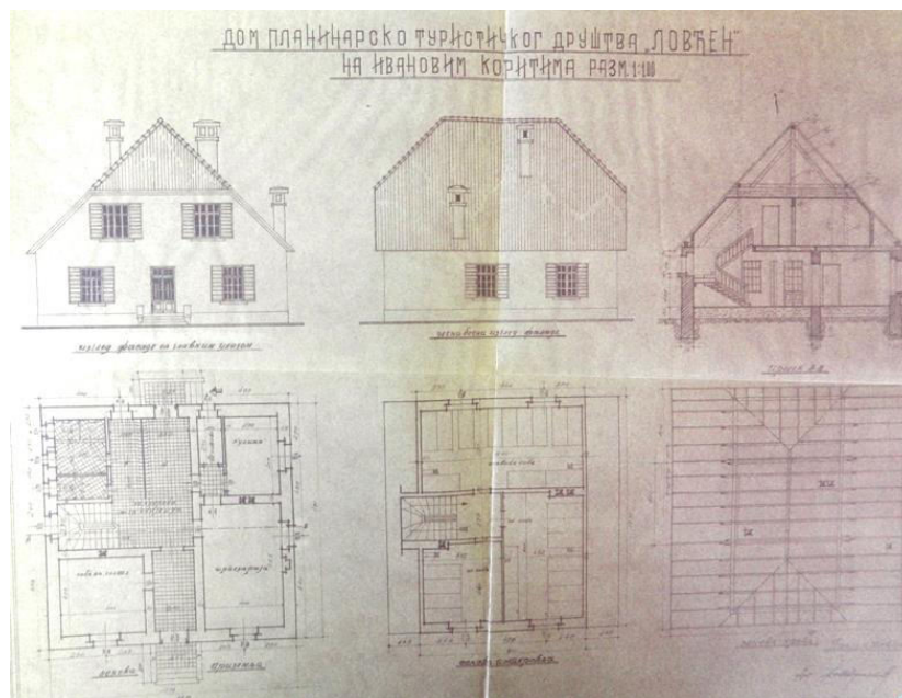
Прилог 166 Дом планинарско-туристичког друштва „Ловћен“ на Ивановим Коритима, План, арх. Новица Вушовић, изгледи, основе и пресјек
