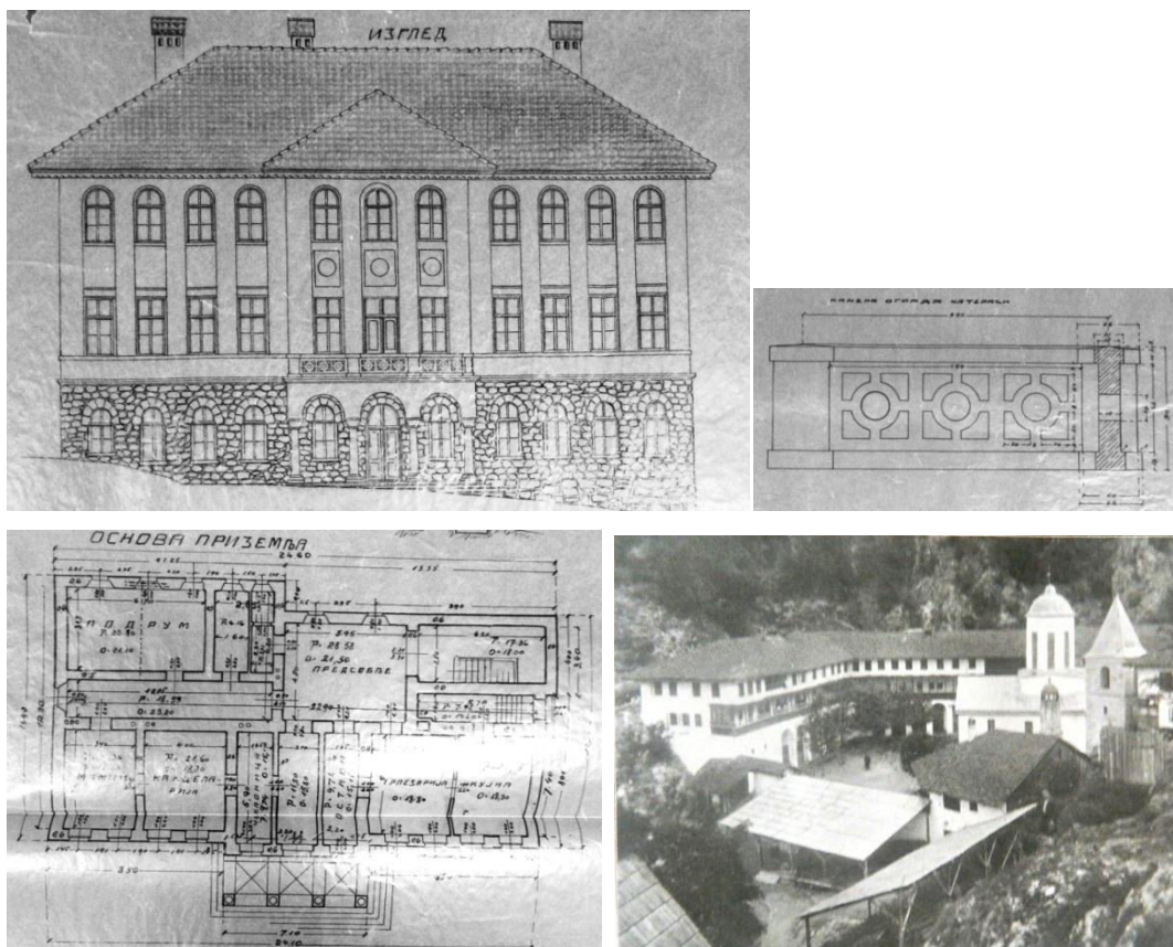
Прилог 74, 2-5 План зграде конака манастира св. Тројице Пљеваљске, арх. Рада Миливојевић, 1925, изглед, детаљ оградe на тераси, основа приземља (Архив Југославије-Београд,Збирка планова Архитект. одељења Министарства грађевина КЈ без броја-227); Манастир Св. Тројица Пљеваљска, изглед ( Илустровани званични алманах-шематизам Зетске бановине , Сарајево 1931)
