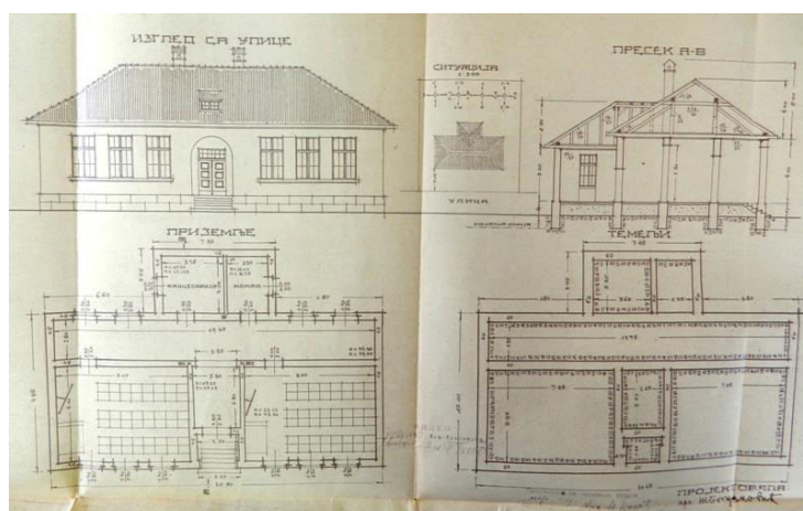
Прилог 106, 1-3 Тип за основну школу у селу са једном учионицом и учитељским станом, арх. Станислава Јовановић, 1929; Тип за основну школу у селу са двије учионице и два учитељска стана, арх. Живана Богдановић, 1929; Тип за основну школу у селу са двије учионице, арх. Живана Богдановић (ДАЦГ, Фонд Краљевске банске управе Зетске бановине-Техничко одјељење, Ф50-Планови-основне школе-разни типови)
