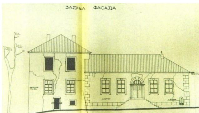
Прилог 14, 1-3 Основна школа у Глухом Долу, Пројекат санације, 1985, основа приземља, прочељна и задња фасада (УЗКД); Прилог 14 -4 Изглед прочеља 2016. (Слађана Жуњић)
