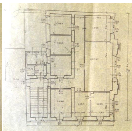
Прилог 35, 1-4 Кућа Марка Милошевића-хотел „Њујорк“ на Цетињу, План, перспективни изглед, пресјек А-В, основа приземља, основа првог спрата (ДАЦГ, Фонд Краљевске Банске управе Зетске бановине-Техничко одјељење, Ф 28 - Срез Цетињски)
