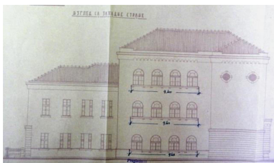
Прилог 105, 7-9 Трговачка академија и Занатска школа у Подгорици, Пројекат, арх. Петар Вукотић, 1940, главни изглед и бочни изгледи, са западне и источне стране (ДАЦГ, Фонд Краљевске Банске управе Зетске бановине-Техничко одјељење, Ф 23 - Срез подгорички)
