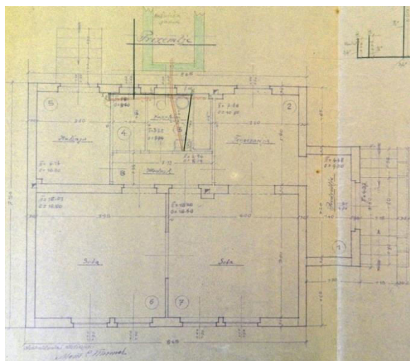
Прилог 91-2 План зграде бр. 11 официјерског стана на Обилића пољани у Цетињу
