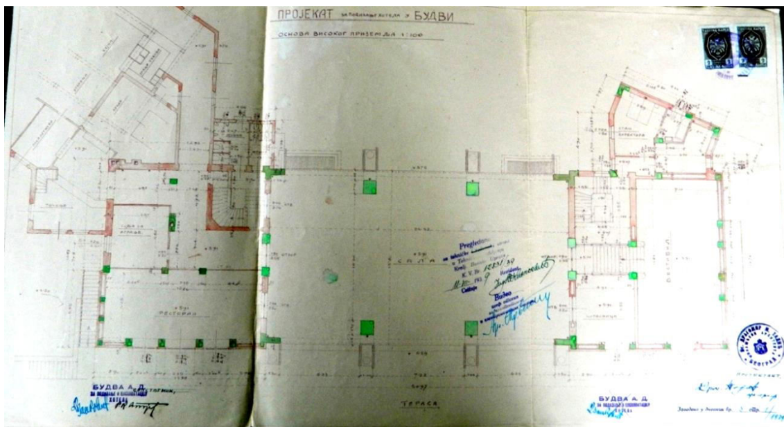
Прилог 156, 5-7 Пројекат за подизање хотела у Будви, арх. Драгомир Тадић, ситуациони план, пресејци, основа високог приземља (ДАЦГ, Фонд Краљевске Банске управе Зетске бановине-Техничко одјељење, Ф 16-Срез Котор)
