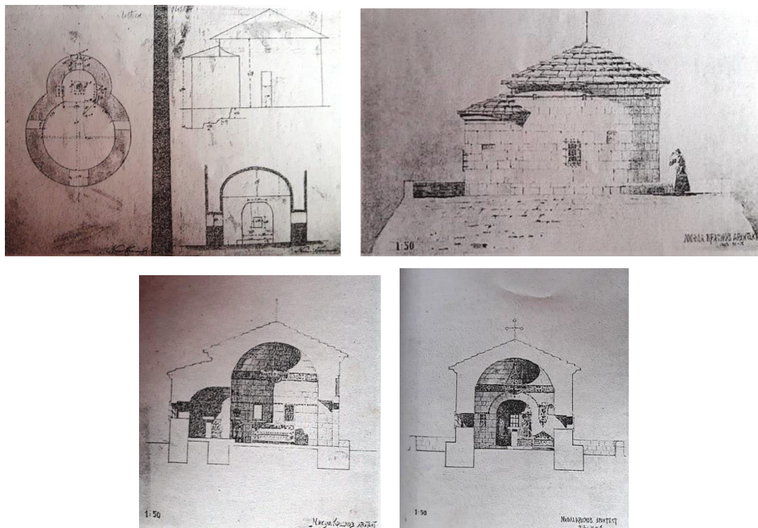
Прилог 68- 6 Скице основе и величине Цркве на Ловћену и њеног олтара, арх. Николај Краснов Прилог 68, 7-9 План за обнову Цркве на Ловћену, арх. Николај Краснов, 21.10.1923, акварели, сјеверна страна, подужни и попречни пресјек (Љ. Дурковић-Јакшић, Његош и Ловћен, Београд 1971)
