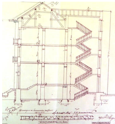
Прилог 95, 5-10 Мања зграда чиновничких станова на Цетињу, Пројекат, арх. Гојко Тодић, 1930, главни изглед, основе сутерена, приземља и првог спрата, пресјек 1:50, пресјек 1:100 (ДАЦГ, Фонд Кр. банске управе Зетске бановине-Техничко одјељење, Ф 63-Чиновнички станови-Цетиње)
