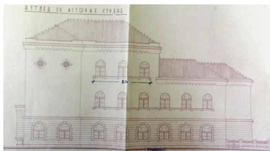
Прилог 105, 7-9 Трговачка академија и Занатска школа у Подгорици, Пројекат, арх. Петар Вукотић, 1940, главни изглед и бочни изгледи, са западне и источне стране (ДАЦГ, Фонд Краљевске Банске управе Зетске бановине-Техничко одјељење, Ф 23 - Срез подгорички)
