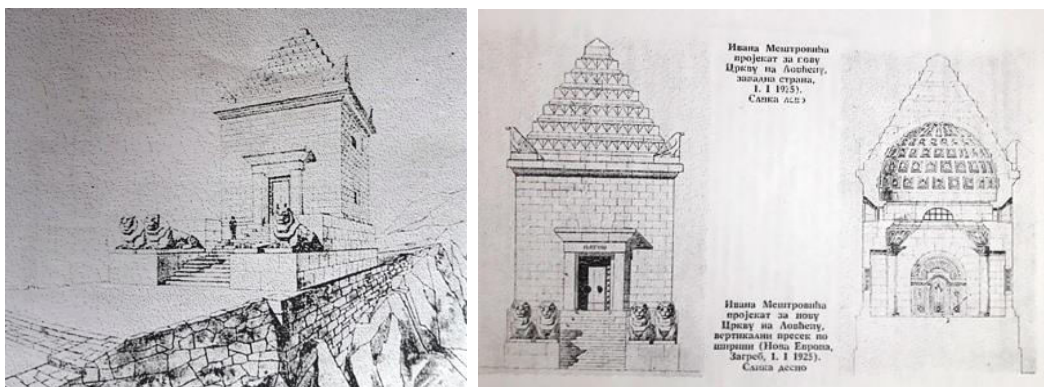
Прилог 68, 10-11 Пројекат за нову Цркву на Ловћену, Иван Мештровић, објављен у листу „Нова Европа“ 1.1.1925, изглед, улазна фасада, попречни пресјек (Љубомир Д.-Јакшић, Његош и Ловћен, Београд 1971)
