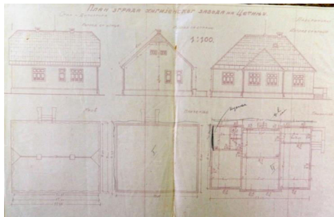
Прилог 19, 2-3 План за одводњавање земљишта Хигијенског завода на Цетињу из 1931; План зграда Хигијенског завода на Цетињу, стан директора и лабораторија (ДАЦГ, Фонд Краљ. Банске управе Зетске бановине-Техничко одјељење, Ф 33 - Срез цетињски)
