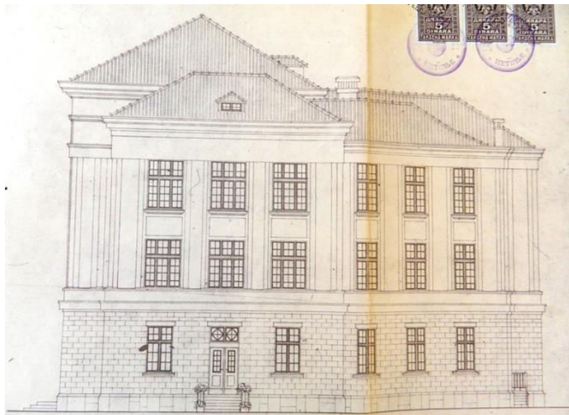
Прилог 12, 1-6 Зграда гимназије у Подгорици, Извођачки пројекат, арх. Фридрих Валента, 1926, основе приземља и првог спрата, пресјек А-Б, пресјек Ц-А, изглед из дворишта, изглед са стране (ДАЦГ, Фонд Краљ. Банске управе Зетске бановине -Техничко одјељење, Ф 23-Срез подгорички)
