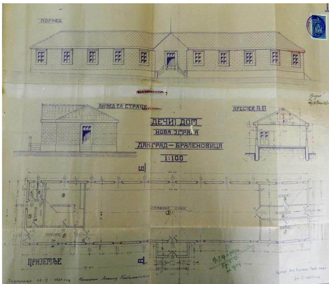
Прилог 29-5 Нова зграда Дјечијег дома на Бранеловици, цртеж из 1924.
