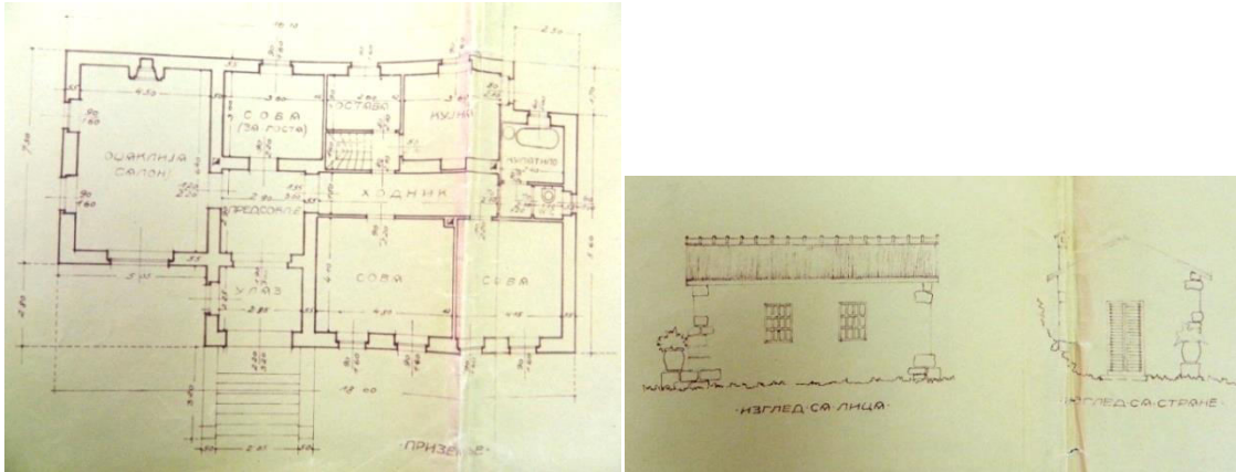
Прилог 41, 2-4 Вила Милована Џаковића и његове сестре С. Брковић на Цетињу, План, арх. Миладин Прљевић, pročеље, основа приземља и помоћни објекат (ДАЦГ, Фонд Краљевске Банске управе Зетске бановине - Окружни суд Цетиње, 1930. година, тапије 101-171, Ф 407)
