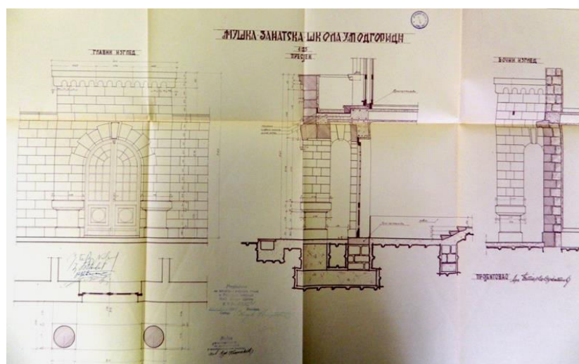
Прилог 105, 1-4 Мушка занатска школа у Подгорици, Пројекат, арх. Петар Вукотић, 1938, основа приземља и оградe, главни изглед, бочни изглед, улазни трем (ДАЦГ, Фонд Краљевске Банске управе Зетске бановине-Техничко одјељење, Ф 23 - Срез подгорички)
