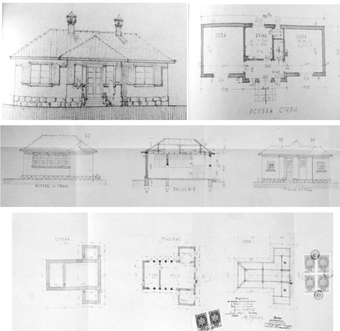
Прилог 140, 1-2 Кућа за главног машинисту Електричне централе у Беранама, Пројекат, арх. Др. Петковић, 1938, изглед главне фасаде и основа стана; Прилог 140, 3-4 Машинска кућа Електричне централе у Беранама, Пројекат, арх. Др. Петковић, 1938, изгледи фасада, пресјек и основе (ДАЦГ, Фонд Краљ. Банске управе Зетске бановине-Техничко одјељење, Ф 10-Срез берански и Бијело Поље)
