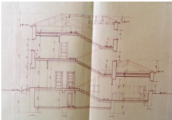
Прилог 136, 1-3 Јавна берза рада у Подгорици, План, 1936, изглед прочеља, основа приземља, пресјек (ДАЦГ, Фонд Краљевске Банске управе Зетске бановине -Техничко одјељење, Ф 24-Срез подгорички)
