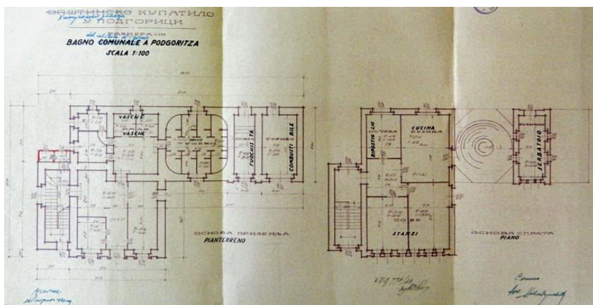
Прилог 20, 1-2 Дом народног здравља у Подгорици, главна фасада и пресјек, основе, снимко арх. Новица Вушовић, 1943; Прилог 20, 3-4 Купатило у Подгорици, изглед прочеља, основе приземља и спрата, снимко арх. Новица Вушовић, 1943.
