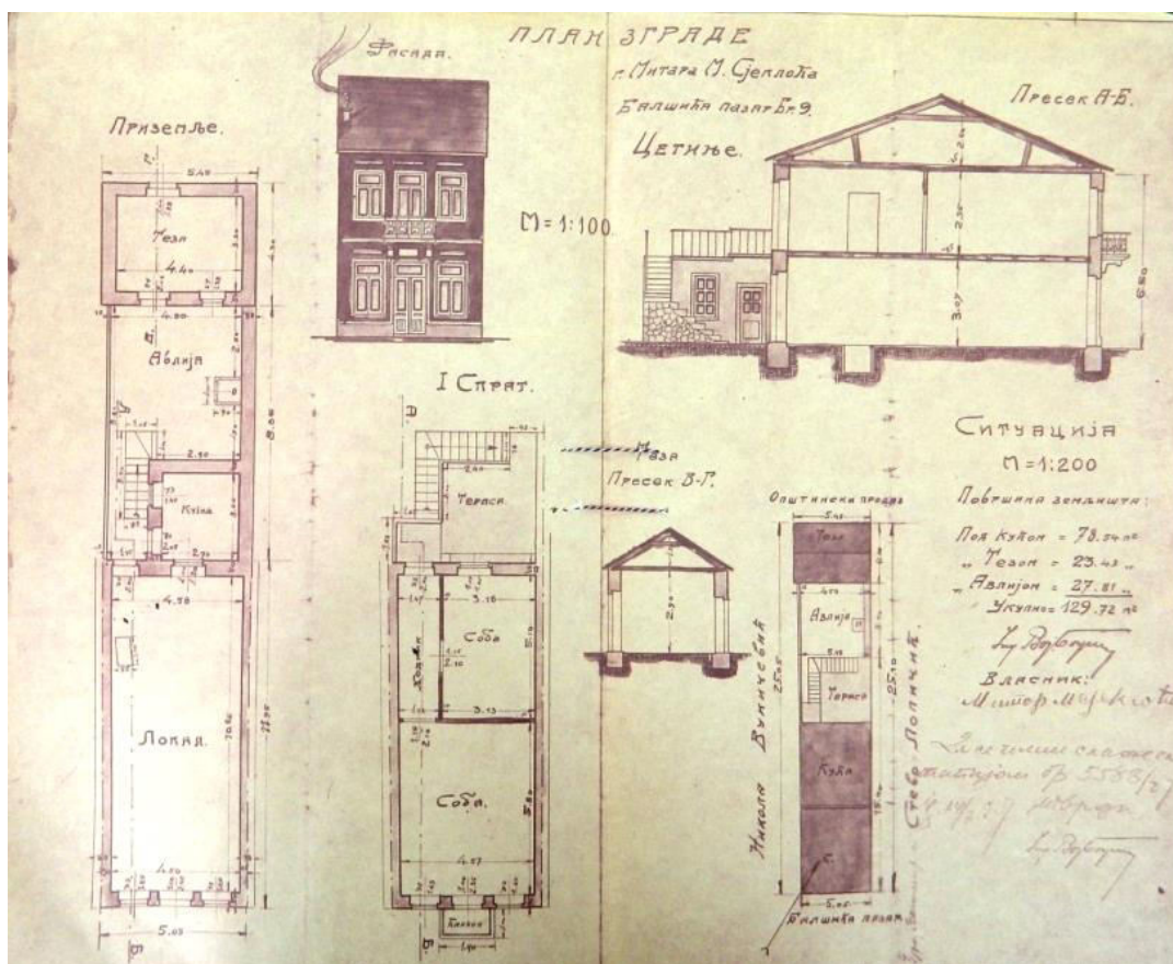
Прилог 40 План куће Митра Сјеклоће на Цетињу, Балшића пазар бр. 9
