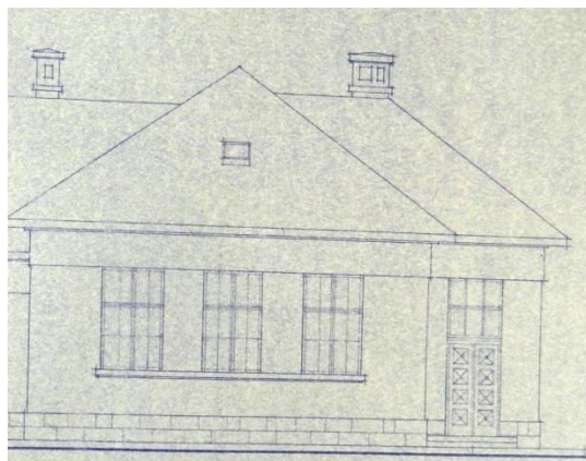
Прилог 115, 1-3 Основна школа у Созини, Пројекат, арх. Виктор Заљевски, 1936, изглед, основа приземља, изглед школских просторија (ДАЦГ,Фонд Краљ. Банске управе Зетске банов.-Техничко одјељење,Ф50-Планови-основне школе-разни типови)
