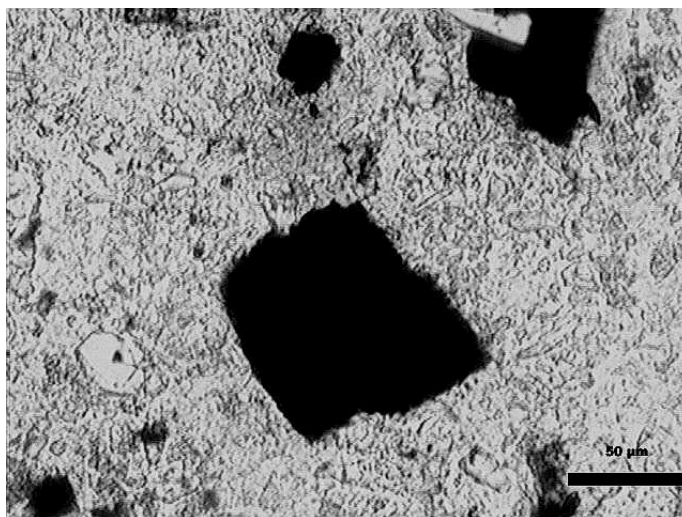
Слика 3.1. Кристал пирита у основној маси узорка зеолитског туфа лежишта Златокоп
