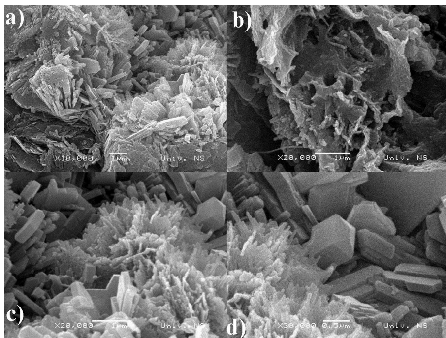
Слика 3.14. Микрофотографије минерала зеолита из лежишта Сланци, скенирајућа електронска микроскопија.
