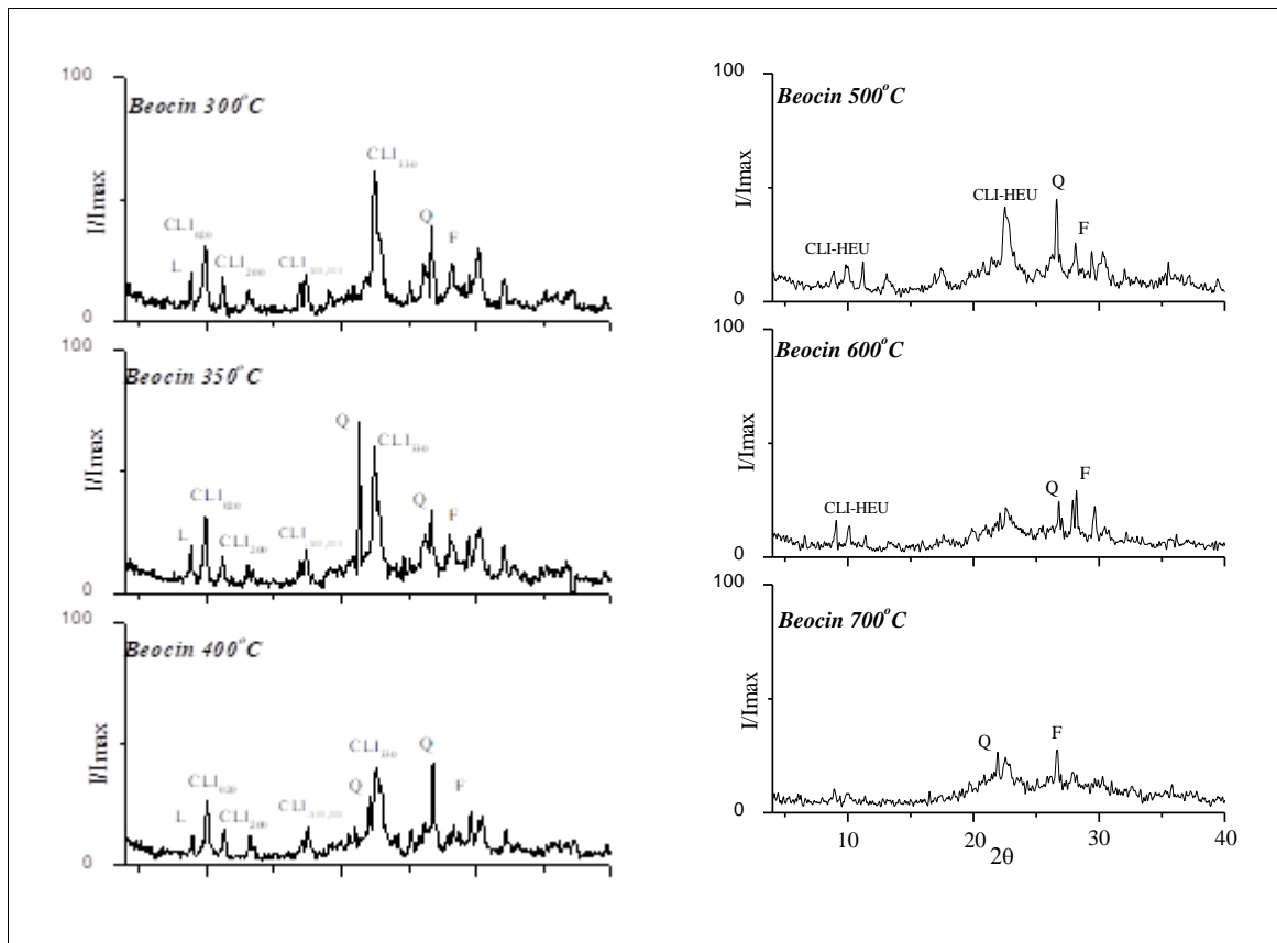
Слика 3.18. Упоредни рендгенски дијаграми праха термички третираног клиноптилолитског туфа лежишта Опћине-Беоцин (зеолити HEU-типа, CLI-клиноптилолит, Q-кварц, F-фелдспати).
