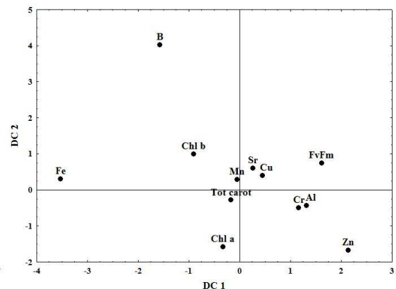
Slika 15. Razlike između ispitivanih lokaliteta na osnovu sadržaja potencijalno toksičnih elemenata, Fv/Fm, Chl a, Chl b i Tot Carot u listovima mleča (1a, 1b); javora (2a, 2b) i breze (3a, 3b); DC - diskriminantna funkcija.
