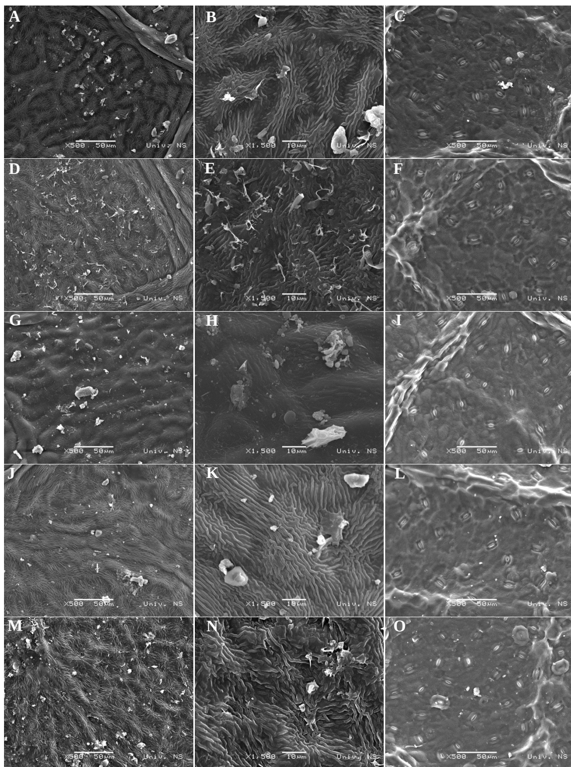
Slika 19. SEM mikrofija lica (LL) i naličja (NL) lista mleča u junu: Pančevo A (LLx500), B (LLx1500), C (NLx500), Smederevo D (LLx500), E (LLx1500), F (NLx500), Obrenovac G (LLx500), H (LLx1500), I (NLx500), Beograd J (LLx500), K (LLx1500), L (NLx500), kontrolni lokalitet M (LLx500), N (LLx1500), O (NLx500).
