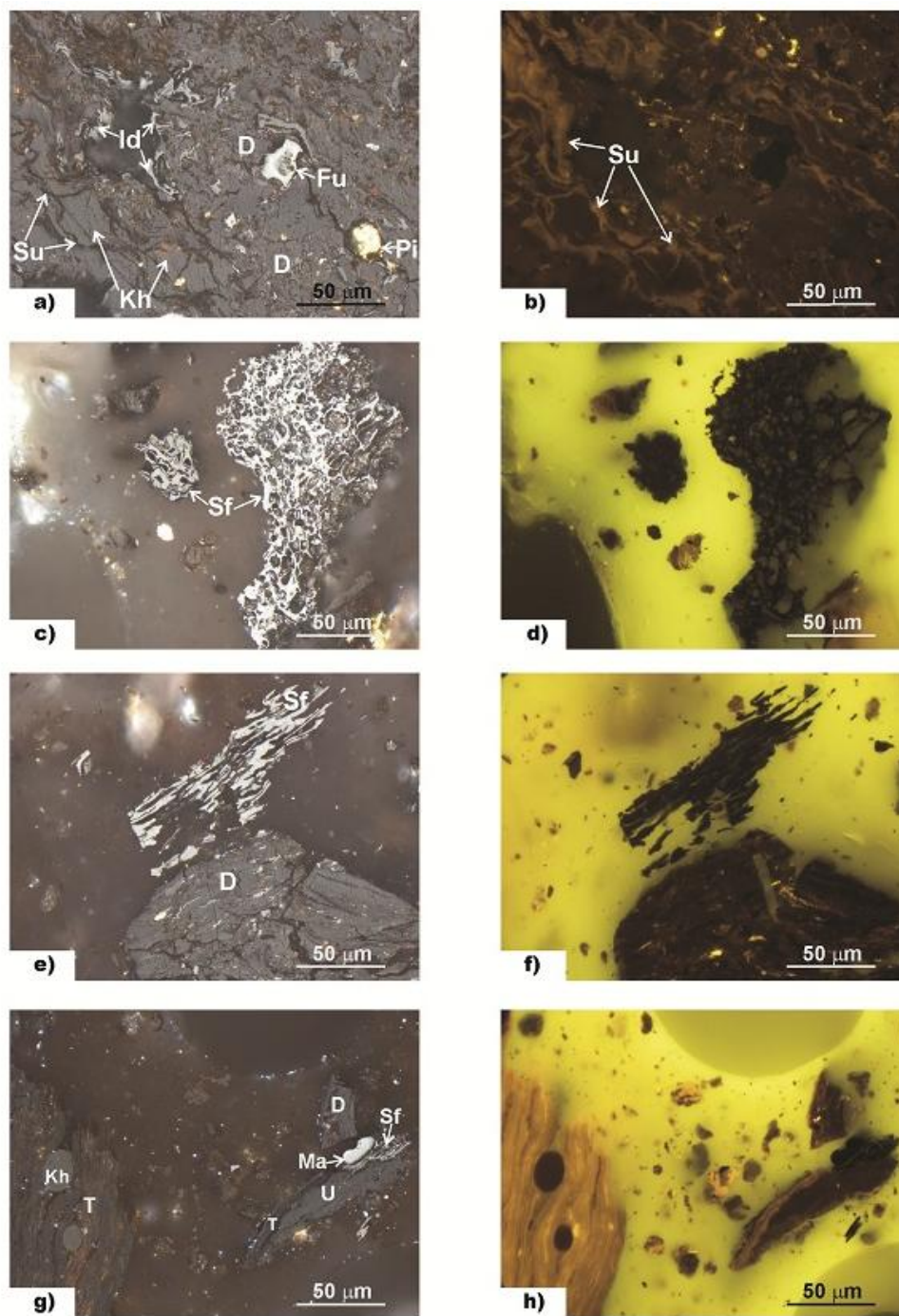
Slika 4. Karakterističan izgled macerala iz ležišta uglja „Kovin“ u normalnoj svetlosti (a, c, e, g) i ultraljubičastoj svetlosti (b, d, f, h).
