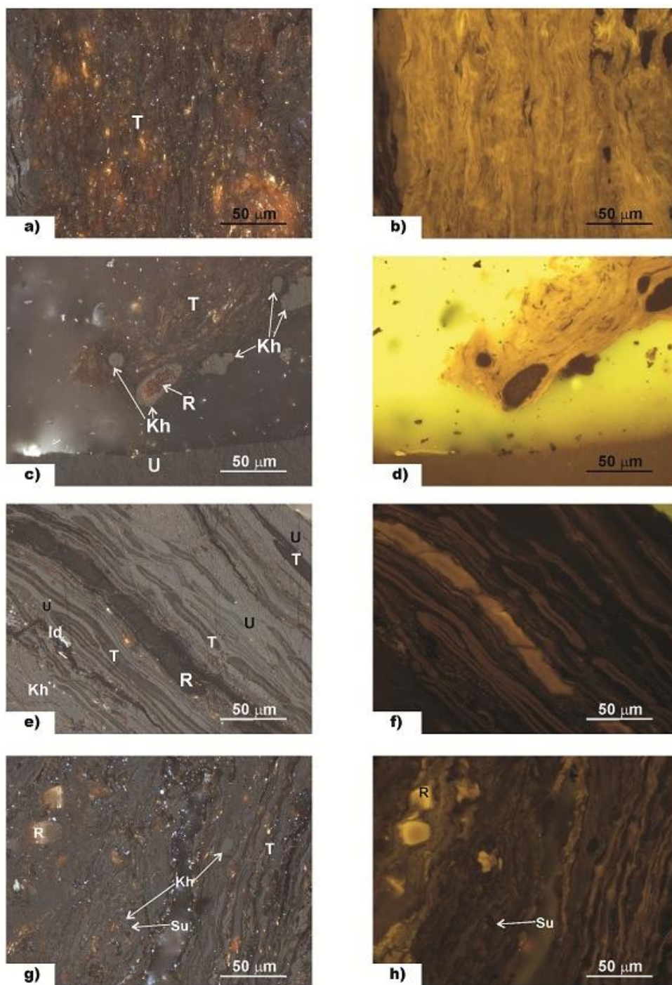
Slika 2. Karakterističan izgled macerala iz ležišta uglja „Kovin“ u normalnoj svetlosti (a, c, e, g) i ultraljubičastoj svetlosti (b, d, f, h).
