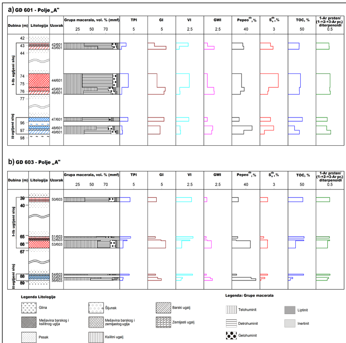
Slika 66. Makropetrografski profili bušotina GD-601 (a) i GD-603 (b) i vertikalna distribucija maceralnih grupa, TPI, GI, VI, GWI, pepela, ukupnog sumpora (S u ), ukupnog organskog ugljenika (TOC) i parametra 1-Ar prsten/(1+2+3-Ar pr.)diterpenoidi.
