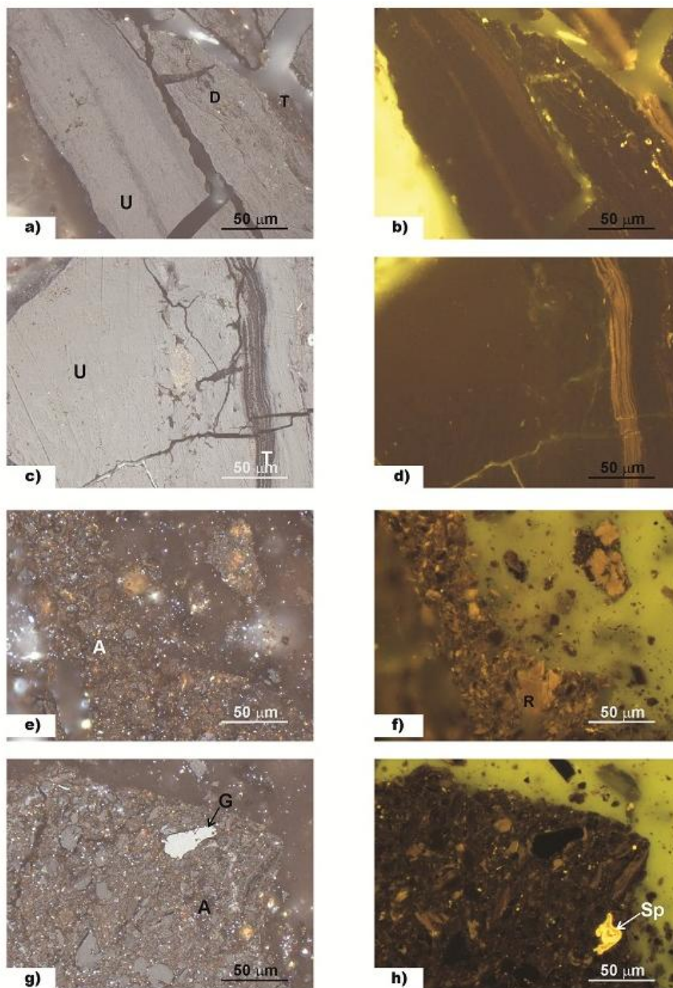
Slika 3. Karakterističan izgled macerala iz ležišta uglja „Kovin“ u normalnoj svetlosti (a, c, e, g) i ultraljubičastoj svetlosti (b, d, f, h).
