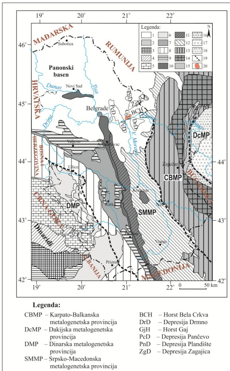
Slika 57. Metalogenetska karta Srbije sa položajem ležišta uglja „Kovin“ (prema Dimitrijević, 2000; dopunjeno prema Schmid et al., 2008; Matenco i Radivojević, 2012).
