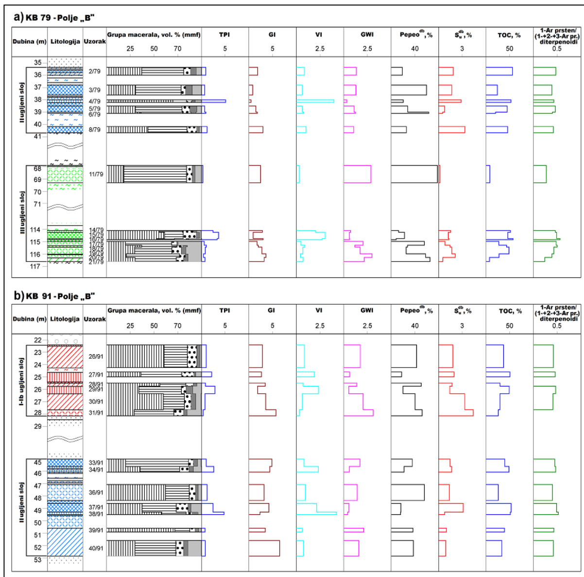
Slika 65. Makropetrografski profili bušotina KB-79 (a) i KB-91 (b) i vertikalna distribucija maceralnih grupa, TPI, GI, VI, GWI, pepela, ukupnog sumpora (S u ), ukupnog organskog ugljenika (TOC) i parametra 1-Ar prsten/(1+ 2- + 3-Ar pr.)diterpenoidi.
