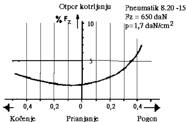
Slika 48. Uticaj iskorišćenog prijanjanja na koeficijent otpora kotrljanja [9]
