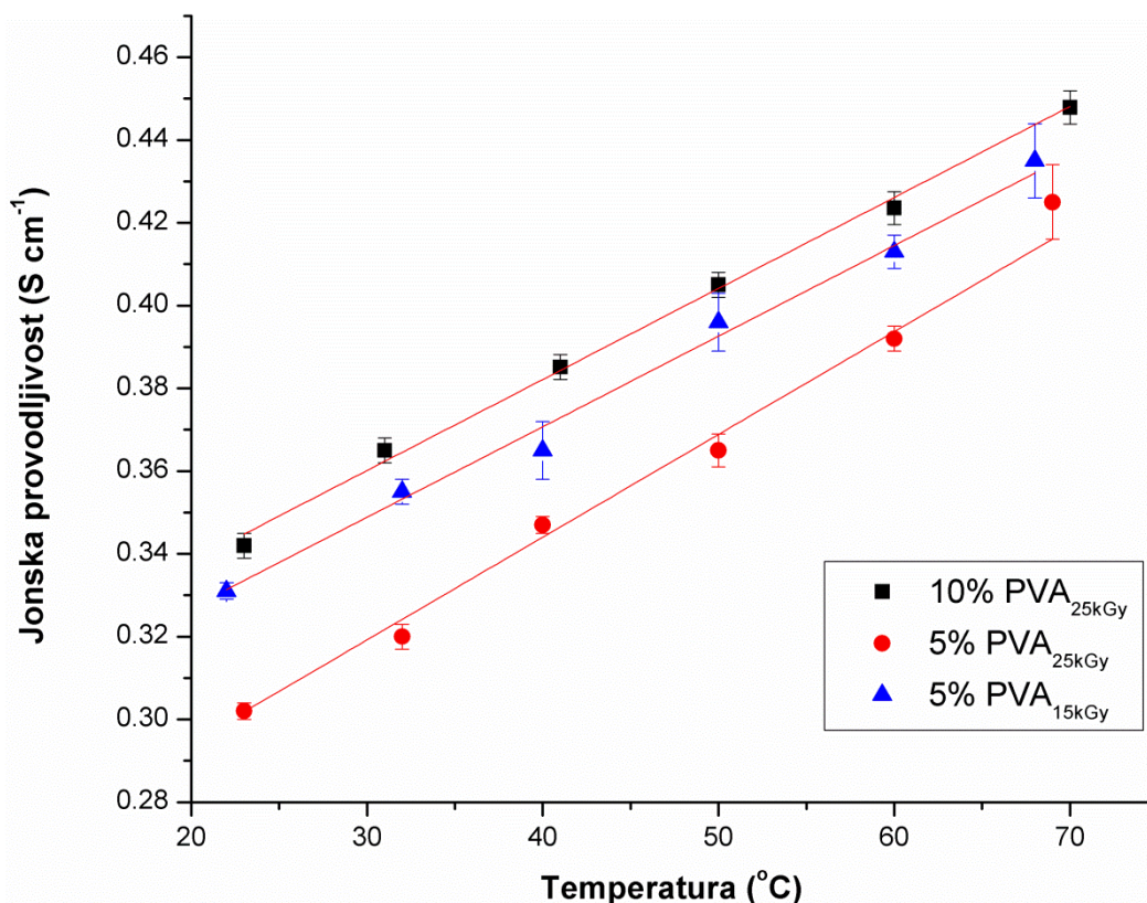
Slika 11. Temperaturska zavisnost jonske provodljivosti (kroz ravan) nesušениh PVA membrana natopljenih 6 M rastvorom KOH.
