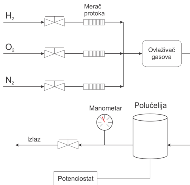
Slika 24. Šematski prikaz sistema za napajanje gasovima i testiranje elektroda u polučeliji.
