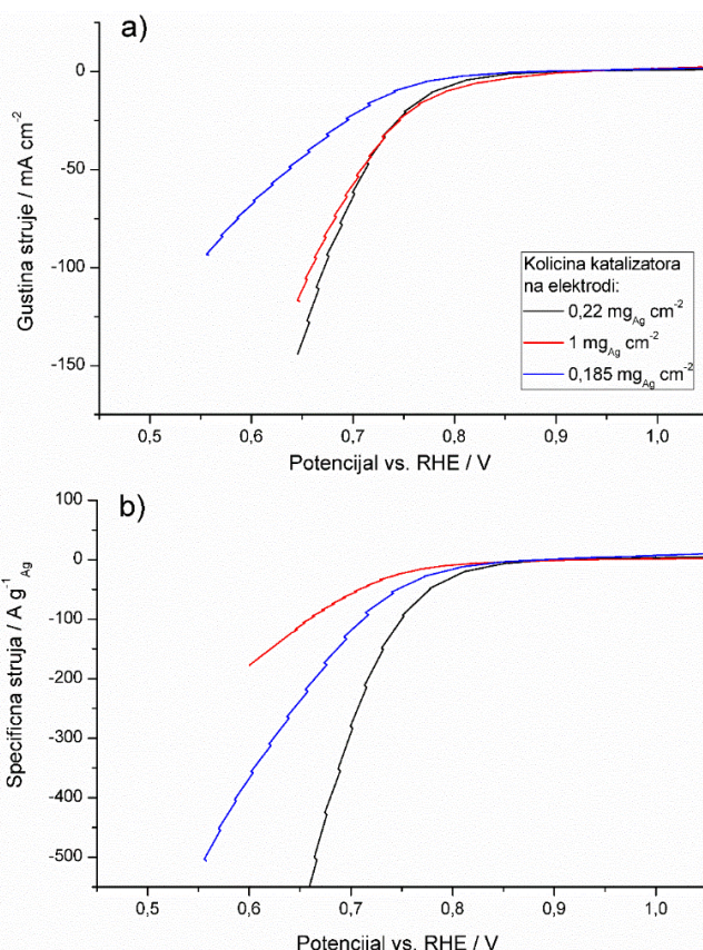
Slika 30. Određivanje optimalne količine srebrnog katalizatora u elektrodi. Gustina struje i specifična struja u funkciji potencijala korigovanog za omski otpor elektrolita. Protok kiseonika (0 % relativne vlažnosti) je 10 mL min -1 pri temperaturi ćelije od 25 °C.
