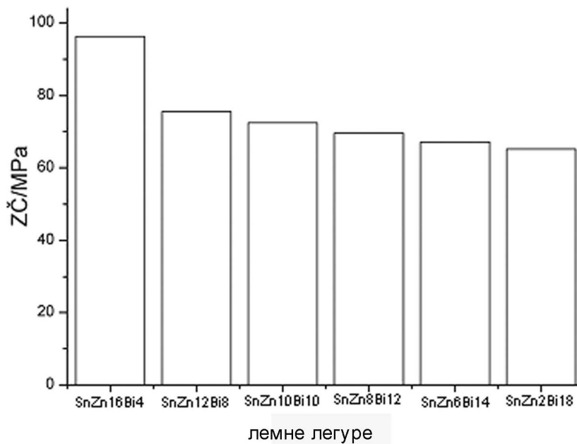
Слика 68 Затезна чврстоћа легура из система Sn-Zn-Bi
