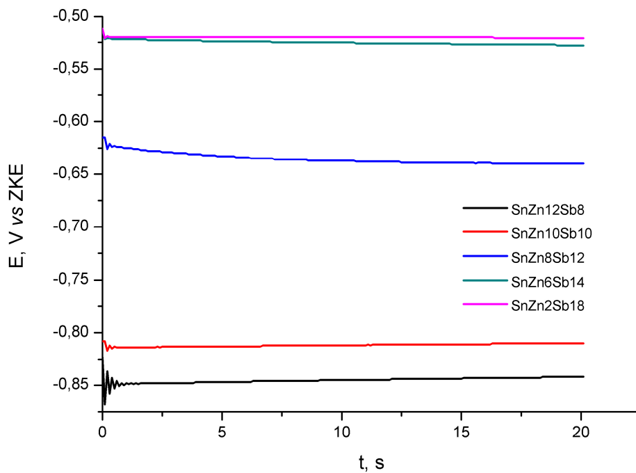
Слика 72 Потенцијали отвореног кола ливених узорака легура система Sn-Zn-Sb у 0,1\text{M}\text{H}_2\text{SO}_4 и на температури 25\pm 0,5^\circ\text{C}
