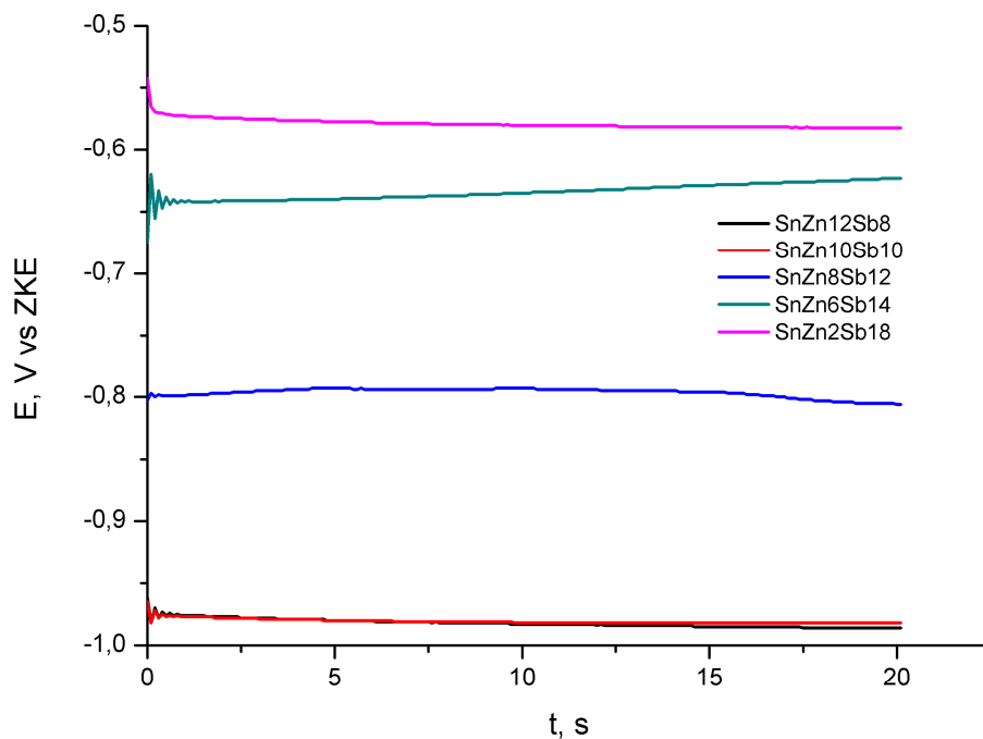
Слика 73 Потенцијали отвореног кола ливених узорака легура система Sn-Zn-Sb у 0,01\text{M}\text{NaOH} и на температури 25\pm 0,5^\circ
