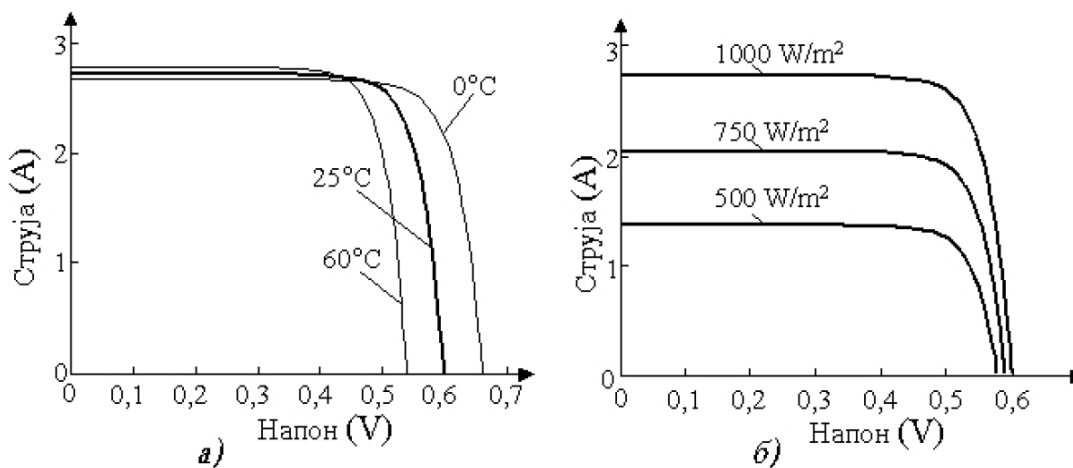
Slika 7.2. Uticaj temperature i iradijacije na U - I karakteristiku fotonaponske ćelije [4]
