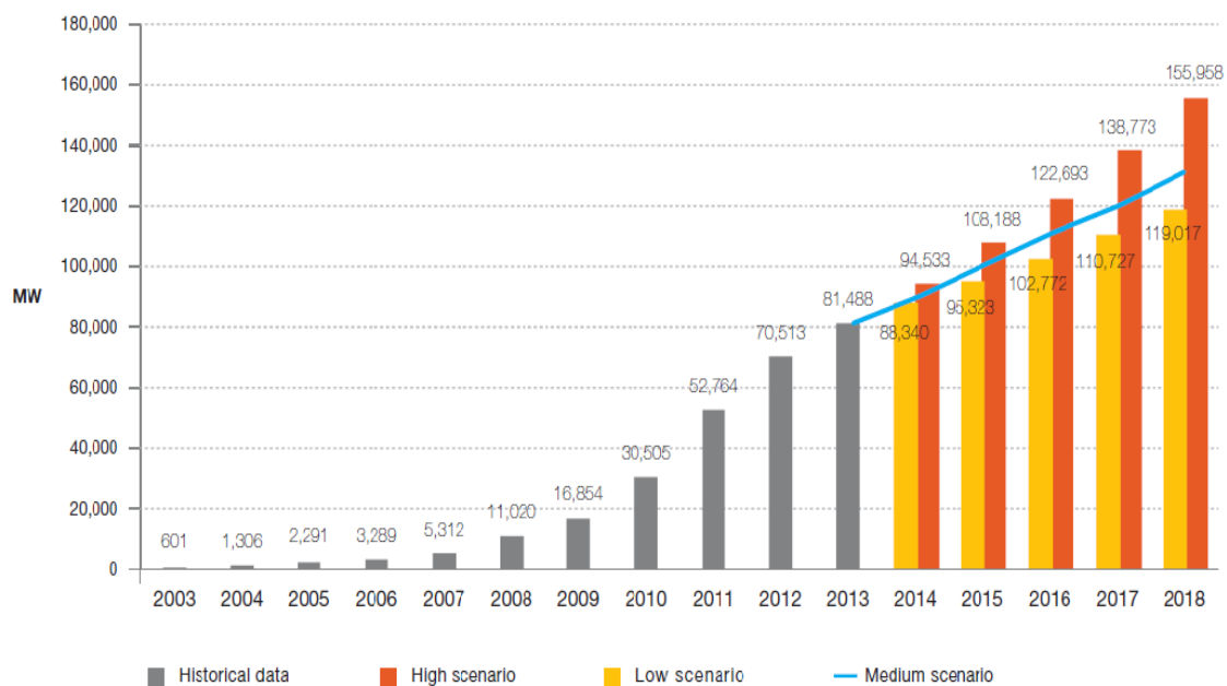
Slika 1.2. Trend porasta instaliranih kapaciteta fotonaponskih sistema u zemljama Evropske Unije [119]
