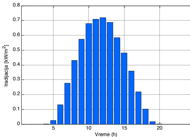
Slika 6.16. Srednje satne vrednosti horizontalne iradijacije za prosečan dan u maju [150]
