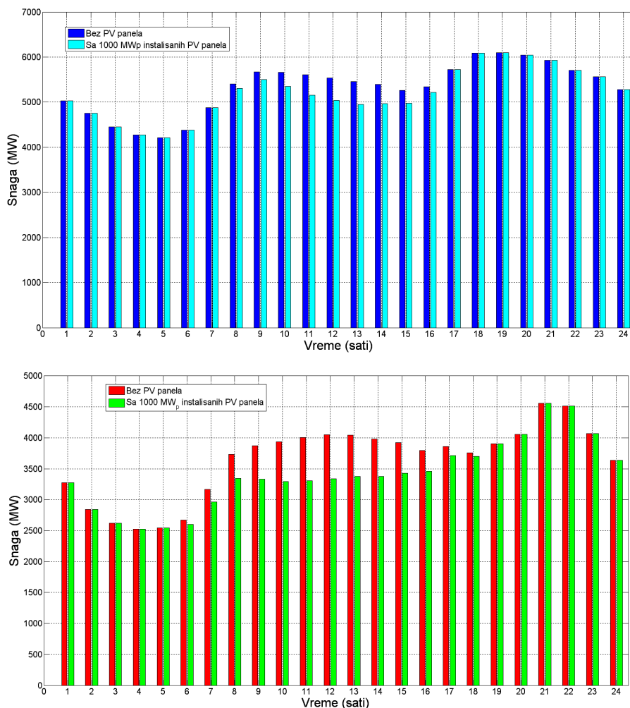
Slika 6.12. Uporedni vremenski dijagrami aktivne snage injecciona u Distributivni sistem Srbije za reprezentativni dan u zimskom i letnjem periodu pre i posle instalacije 1000 MW p disperzovanih krovno i fasadno integrisanih fotonaponskih sistema
