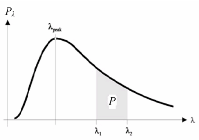
Slika 2.1. Spektar zračenja crnog tela [12]
