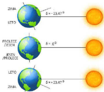
Slika 3.2. Predstava odnosa položaja Zemlje i Sunca [105]
