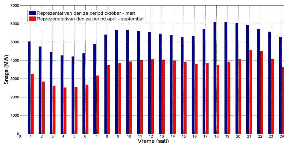
Slika 6.6.. Procenjeni reprezentativni dnevni dijagrami injeckiranja snage u Distributivni sistem Srbije za 2009. godinu
