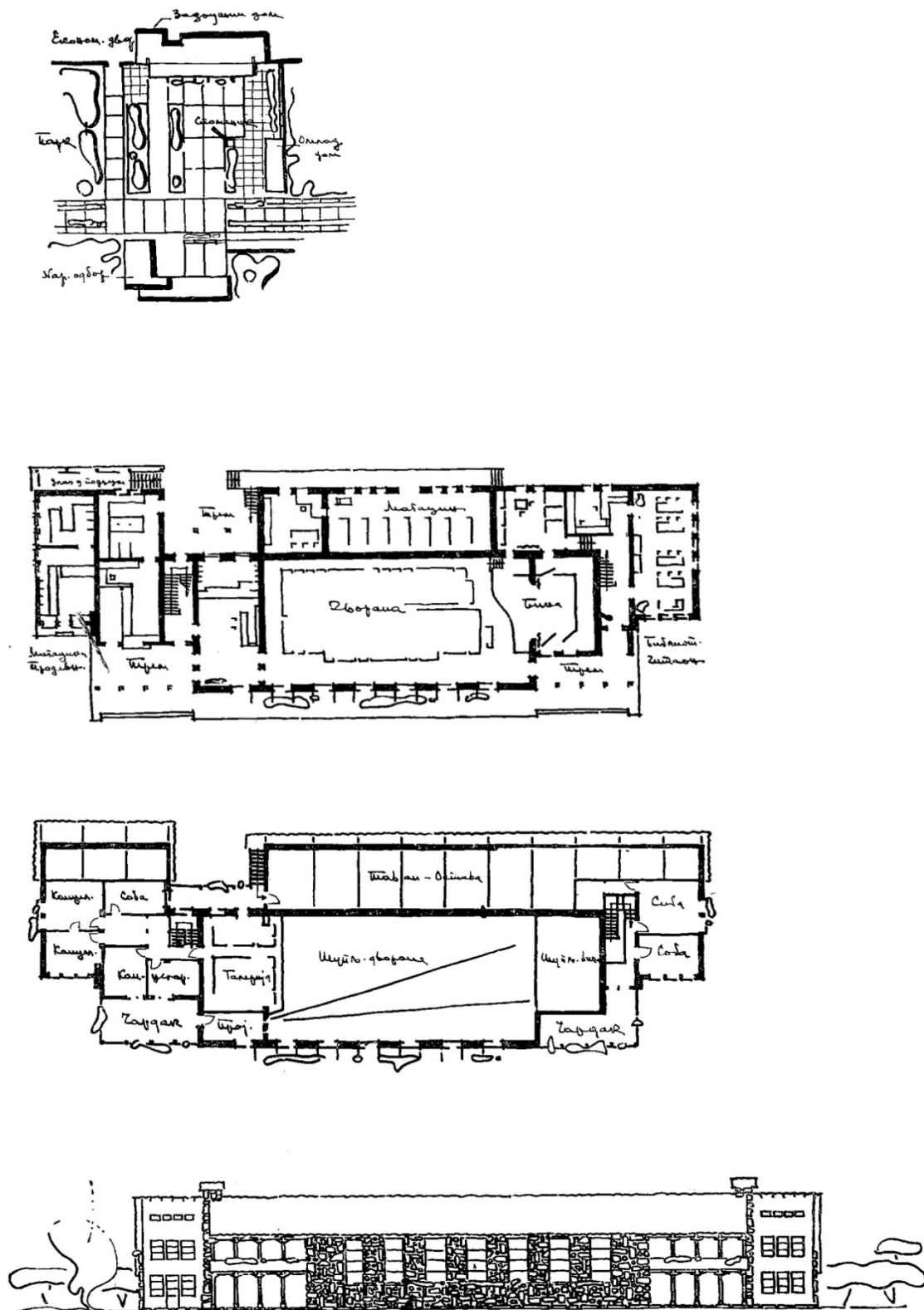
Слика 5.9 - Задружни дом тип 8, арх Станко Мандић, Урбанистичка служба главног архитекта Београда. Milorad Macura, „Zadružni domovi na teritoriji NR Srbije“, Arhitektura, br. 11-12 (1948): 29.
