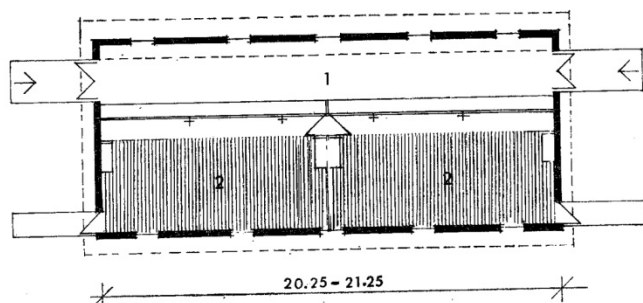
Слика 5. 44 – Стаја за тов 50 јунади од 220 до 420 кг тежине, Према типском пројекту бироа „Наш стан – ИАУС“ Београд 5.41-5.44
