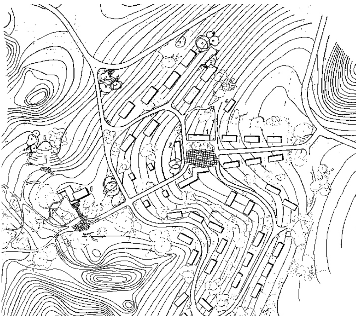
Слика 4.12 – Регулациони план стамбеног насеља Шупља Стијена, Црна Гора Аутор: Михајло Митровић Mihajlo Mitrović „O nekim problemima projektovanja naselja“, Urbanizam –Arhitektura , br. 5-8, (1951): 62..
