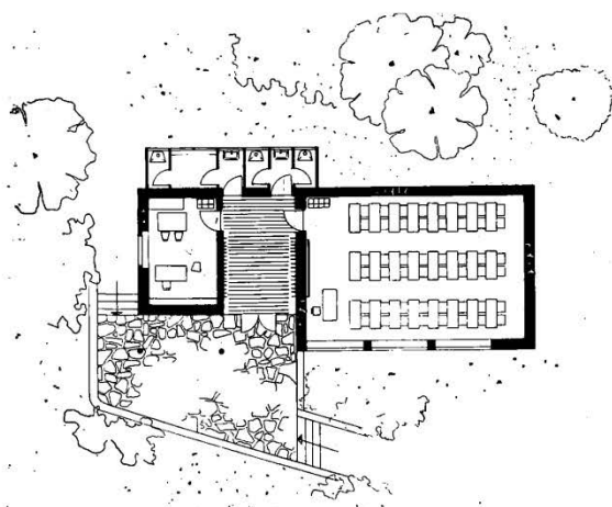
Слика 5. 24 – Једноразредна сеоска школа у Перјасици, Пројектант: Божидар Тушек.
