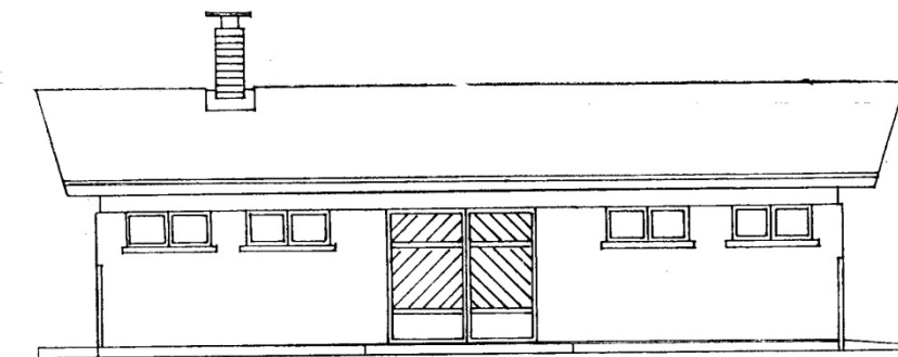
Слика 5. 45 – Типски пројекат овчарника за 50 оваца, Пројектант Ђорђе Симоновић Бранислав Којић и Ђорђе Симоновић, Пољопривредне зграде и комплекси (Београд: Грађевинска књига, 1978), 361.
