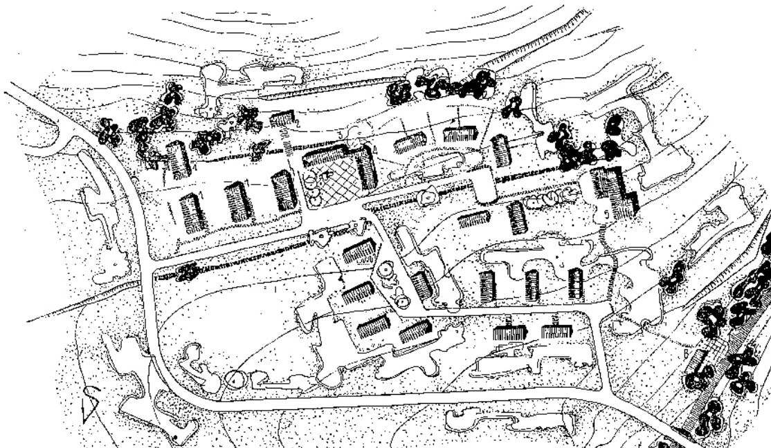
Слика 4.10 – Регулациони план стамбеног насеља Градац, Црна Гора Аутор: Михајло Митровић. Mihajlo Mitrović „O nekim problemima projektovanja naselja“, Urbanizam –Arhitektura , br. 5-8, (1951): 60.
