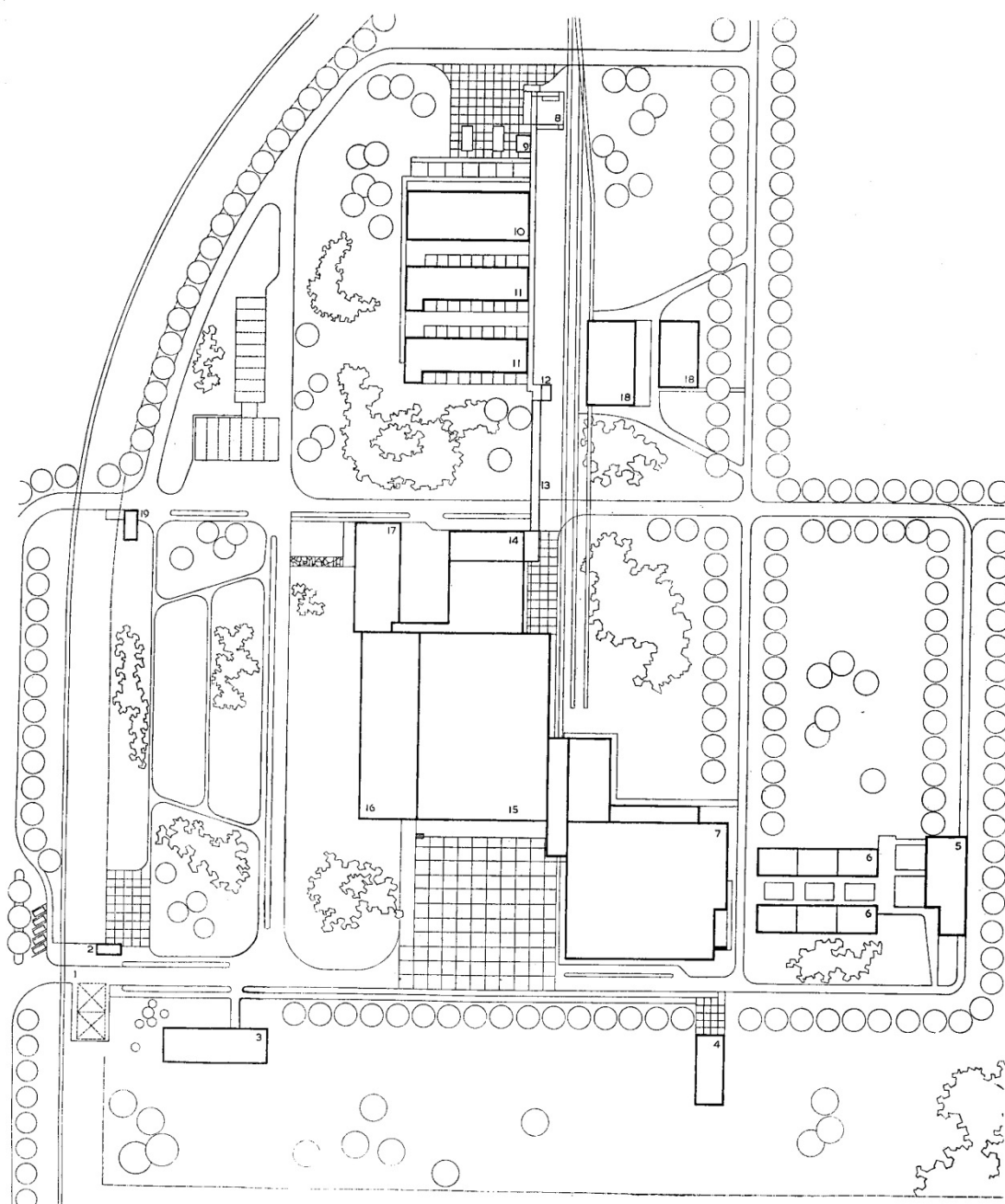
Слика 5. 35a – Комплекс индустријске спратне кланице у Новом Саду, Према пројекту: И. Костић, М. Вујић, С. Гајић
