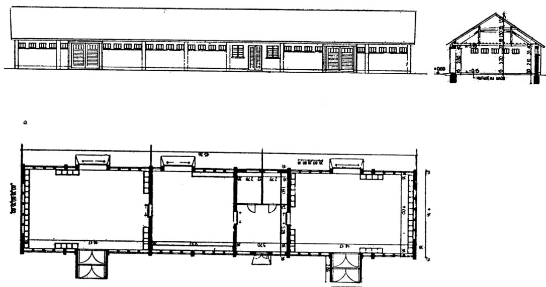
Слика 5. 37 – Типска стаја за подмладак коња до узраста од три године, Пројектант Р. Кадих, према пројектима пољопривредних зграда Министарства грађевина ФНРЈ, 1950.
