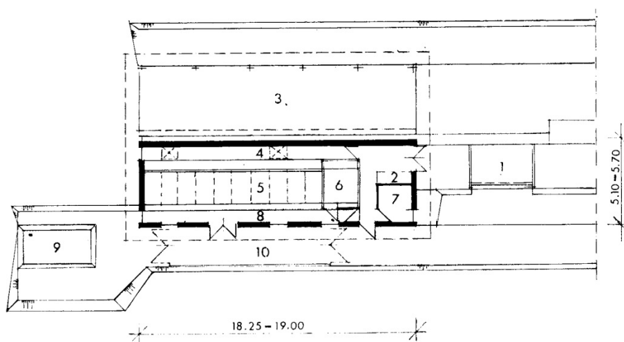
Слика 5. 40 – Стаја за 10 крава музара на планинском терену,
