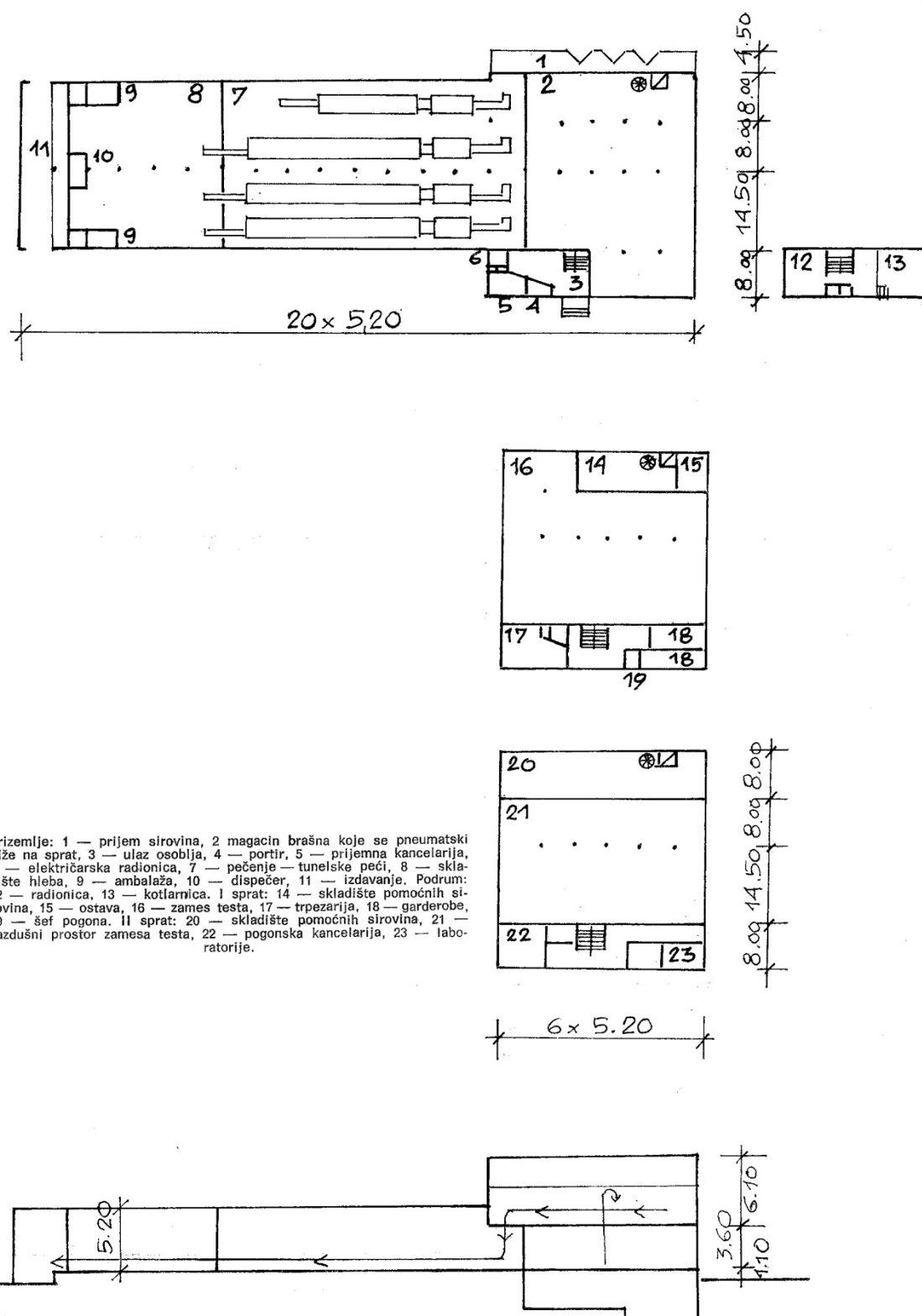
Слика 5. 35 б – Шематски приказ индустријског погона пекаре у Нишу капацитета 84 000 кг хлеба.
