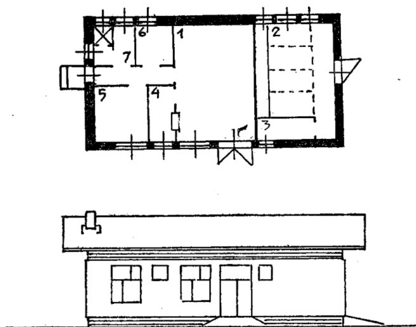
Слика 5. 73 – Тип ветеринарске амбуланте на фарми за 600 крава, Пројектант: Ђорђе Симоновић Бранислав Којић и Ђорђе Симоновић, Пољопривредне зграде и комплекси (Београд: Грађевинска књига, 1978), 386.
