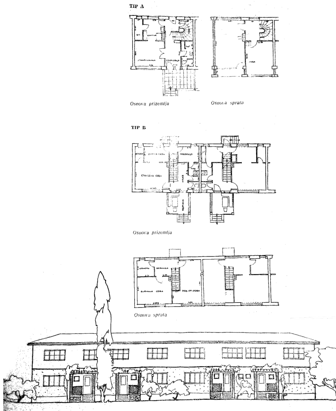
Слика 4.4 – Пројекат типских стамбених јединица „Rudarsko naselje Banovići“, Tehnika , br.1 (1946):267.
