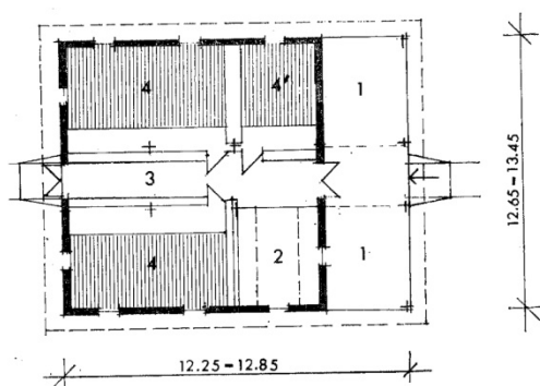
Слика 5. 41 – Стаја за тов 50 телади до 220 кг тежине, Према типском пројекту бироа „Наш стан – ИАУС“ Београд
