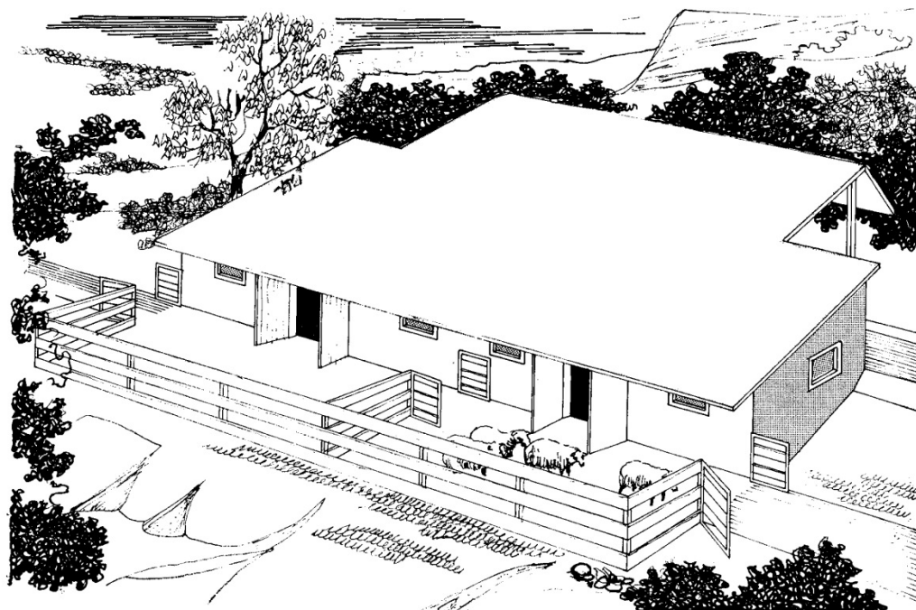
Слика 5. 47 – Типски пројекат овчарника за 100 оваца на равничарском терену (горе), Типски пројекат овчарника за 100 оваца на планинском терену (доле)Према типском пројекту бироа „Наш стан – ИАУС“ Београд Бранислав Којић и Ђорђе Симоновић, Пољопривредне зграде и комплекси (Београд: Грађевинска књига, 1978), 362.
