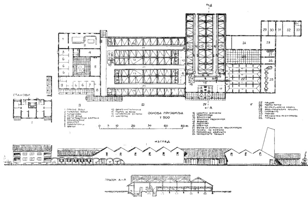
Слика 5. 56 – Винарски подрум у Александровцу, Пројектант: В. Жанко. Предраг Зрнић, „Подаци за пројектовање винарских подрума“, Зборник Архитектонског факултета , књига III, свеска 11 (1956/57): 7.
