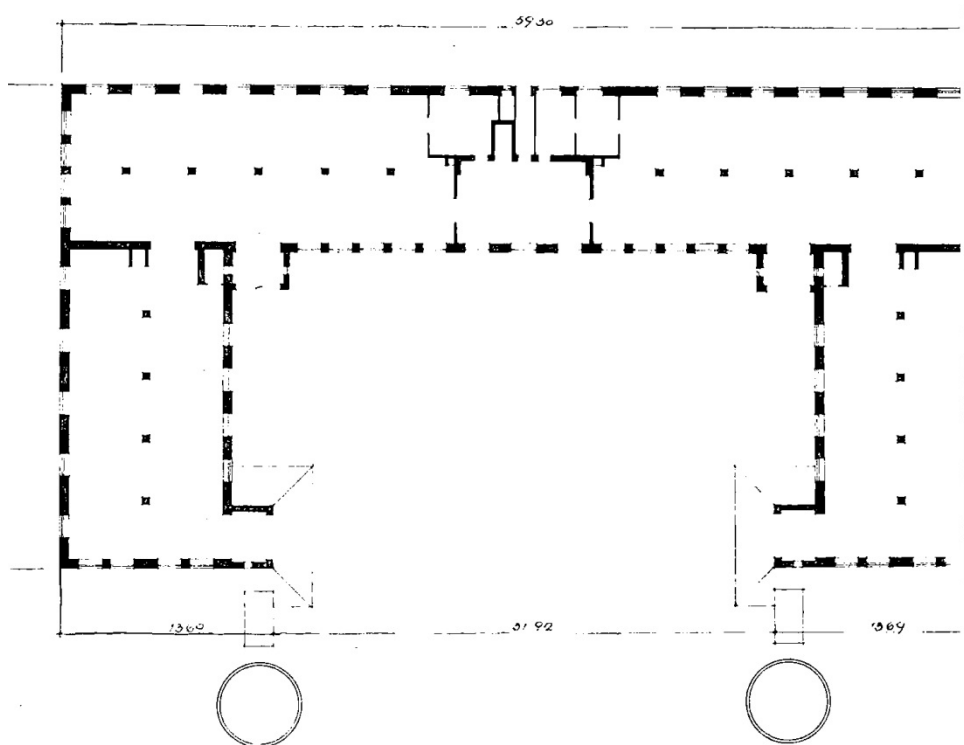
Слика 5. 72 – Нови овчарник у Љубову, Лика, Пројектант: Звонимир Црнокрак. Zvonimir Crnokrak, „Ovčarnici“, Urbanizam-Arhitektura , br. 9-12 (1951): 29.
