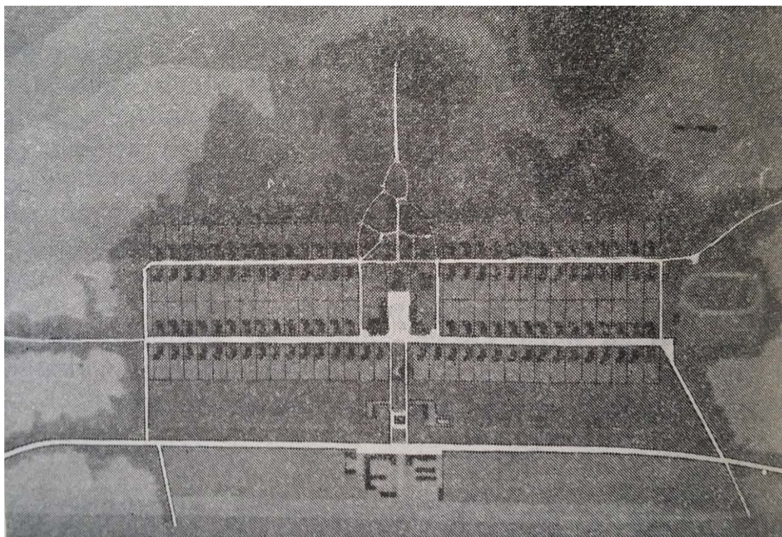
Слика 4.2 – Реконструкција постојећег сеоског насеља Врело Saša Sedlar, „Pitanje planske izgradnje sela u Srbiji“, Tehnika , br.1 (1946): 130.
