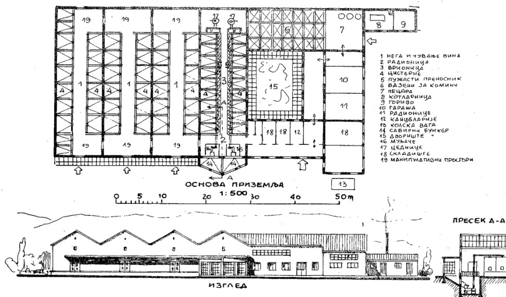
Слика 5. 59 – Винарски подрум у Прокупљу. Предраг Зрнић, „Подаци за пројектовање винарских подрума“, Зборник Архитектонског факултета, књига III, свеска 11 (1956/57): 6.
