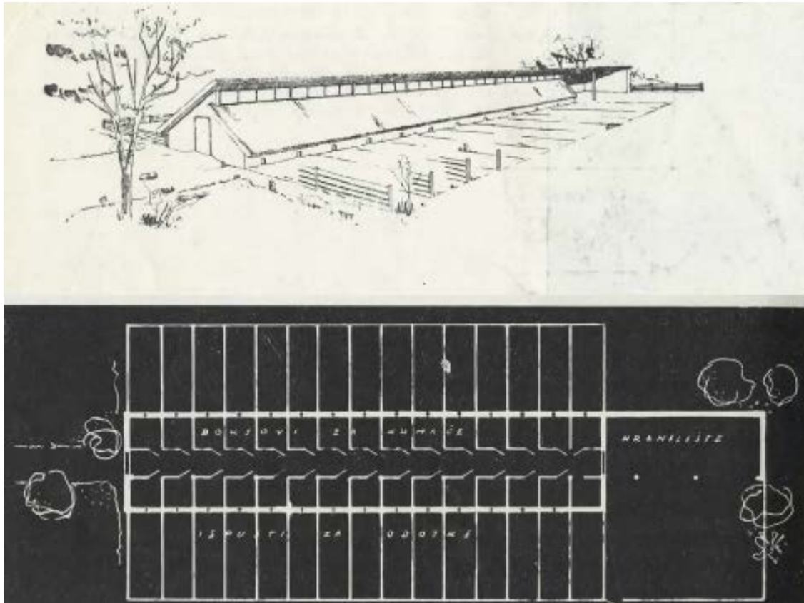
Слика 5. 69 – Тип прасилишта, Пројектант: Жарко Винцек. Žarko Vincek, „Staje za svinje“, Urbanizam-Arhitektura , br. 9-12 (1951): 24.
