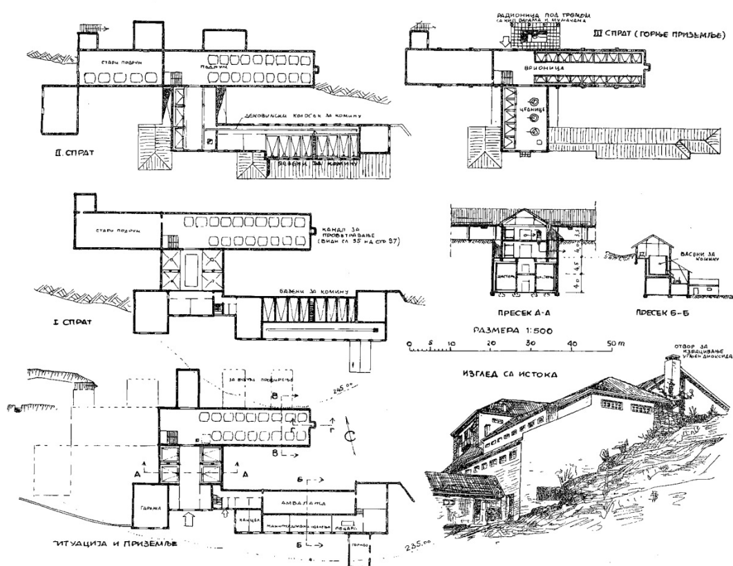
Слика 5. 57 – Винарски подрум у Књажевцу, Пројектант: Аристов Предраг Зрнић, „Подаци за пројектовање винарских подрума“, Зборник Архитектонског факултета , књига III, свеска 11 (1956/57): 5.
