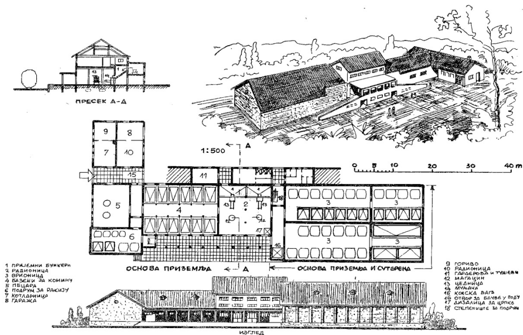
Слика 5. 58 – Винарски подрум у Свилајнцу. Предраг Зрнић, „Подаци за пројектовање винарских подрума“, Зборник Архитектонског факултета, књига III, свеска 11 (1956/57):4.
