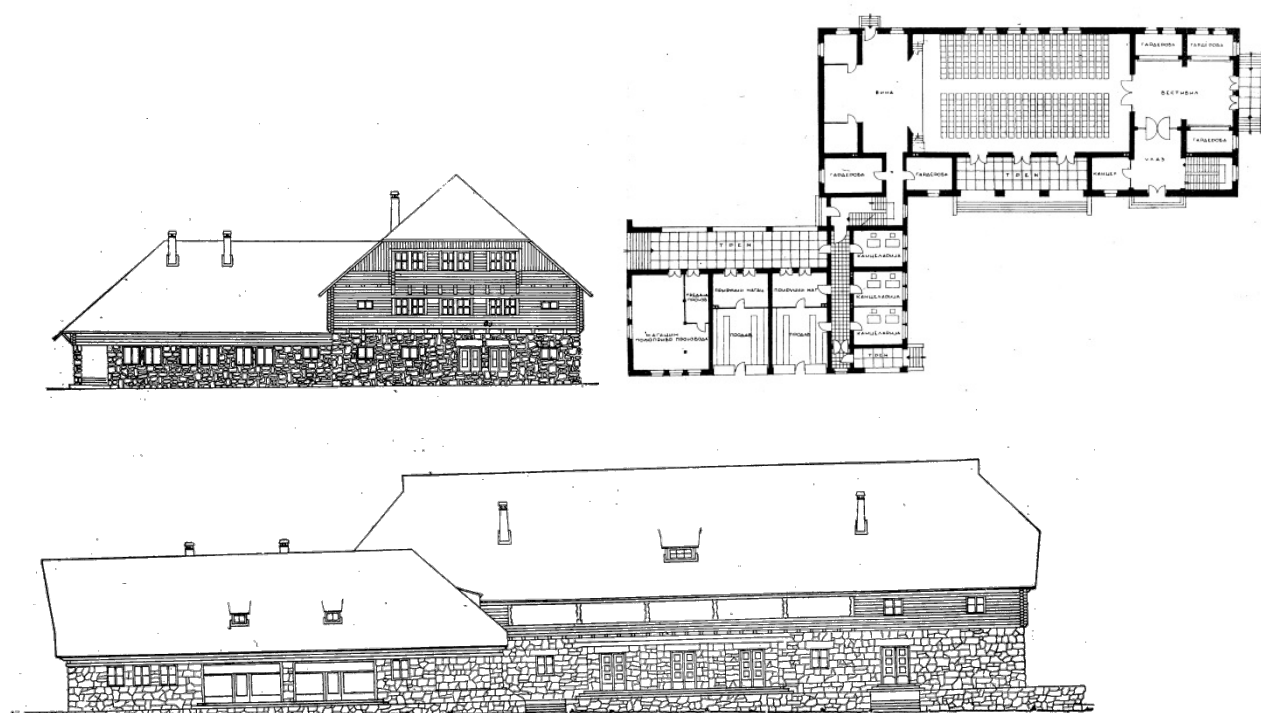
Слика 5.13 - Задружни дом тип 5, архитект Рајко Татић.
