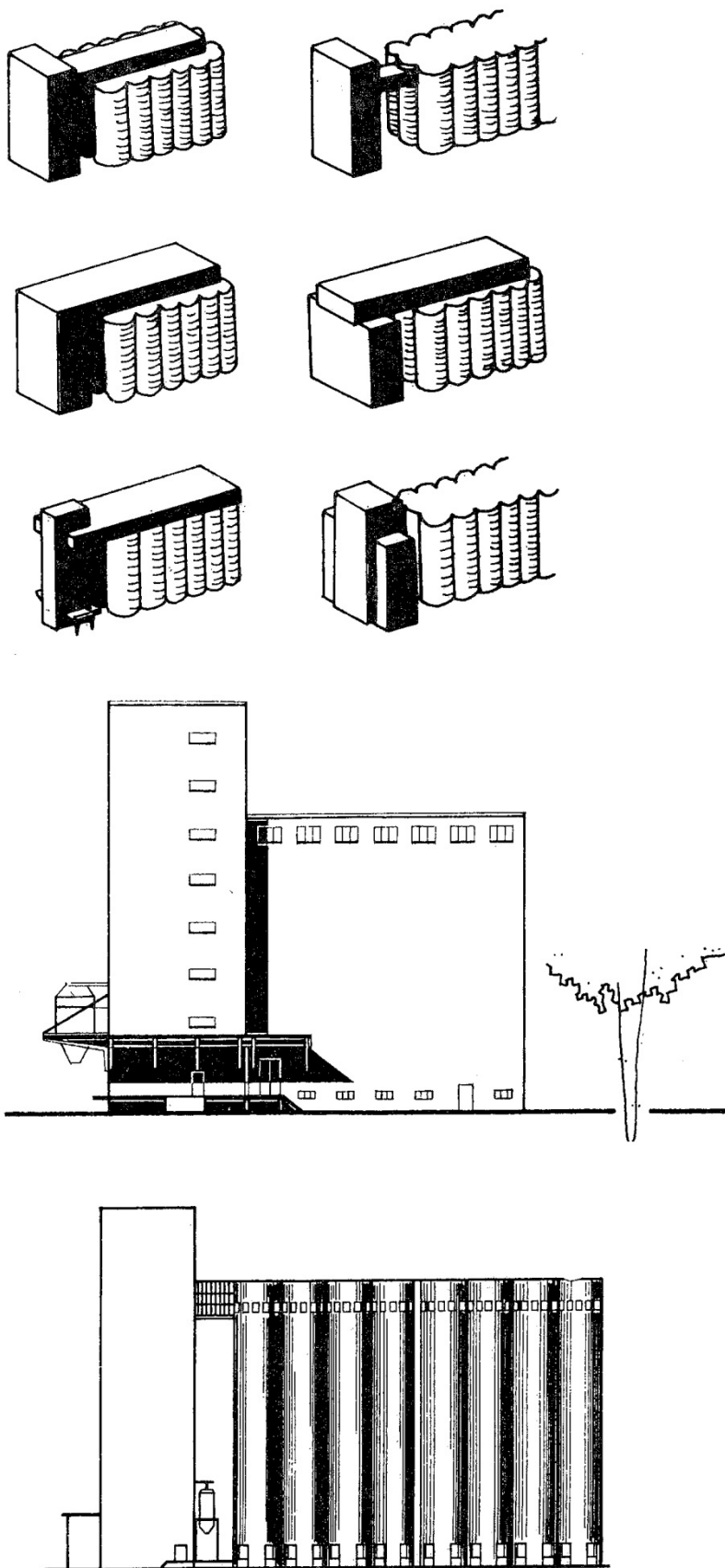
Слика 5.1в – Неколико начина композиције елемената силоса. Бранислав Којић и Ђорђе Симоновић, Пољопривредне зграде и комплекси (Београд: Грађевинска књига, 1978), 80.
