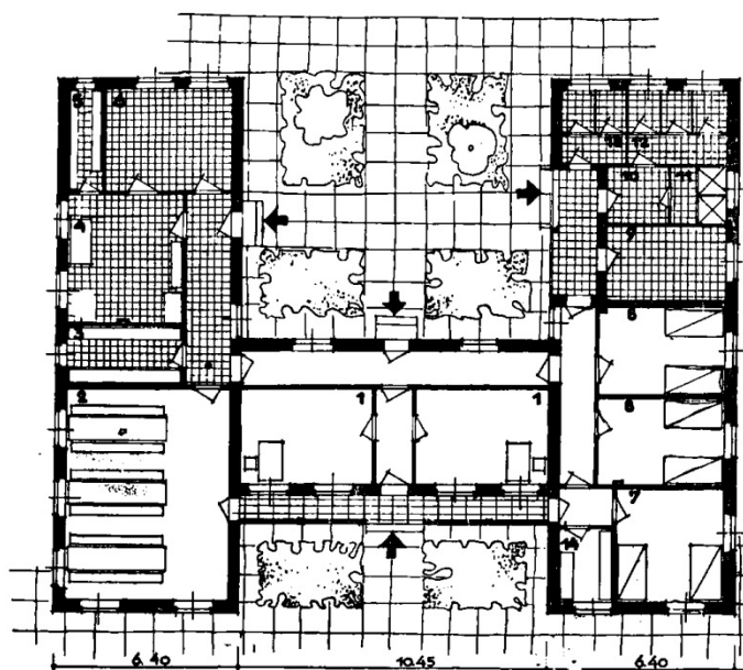
Brigadni dom veće seljačke radne zadruge za ravničarske krajeve: 1. kancelarije ~ 2. trpezarija i sala za sastanke – 3. ostava za torbice sa hranom – 4. sezonska kuhinja – 5. ostava – 6. magacin hrane – 7. i 8. sobe za spavanje – 9. magacin sitnog alata – 10. garderoba – 11. tuševi – 12. WC za muške – 13. WC za ženske – 14. ostava veterinarskog materijala
