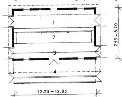
Слика 5. 42 – Стаја за тов 25 јунади од 220 до 420 кг тежине, Према типском пројекту бироа „Наш стан – ИАУС“ Београд,
