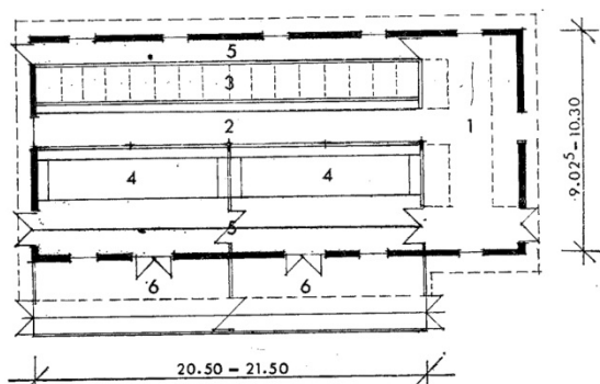
Слика 5. 43 – Стаја за тов 50 телади до 420 кг тежине, Према типском пројекту бироа „Наш стан – ИАУС“ Београд
