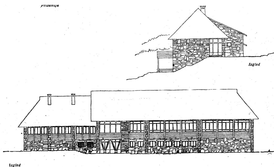
Слика 5. 22 – Тип сеоске основне школе са два разреда за брдовите пределе,
