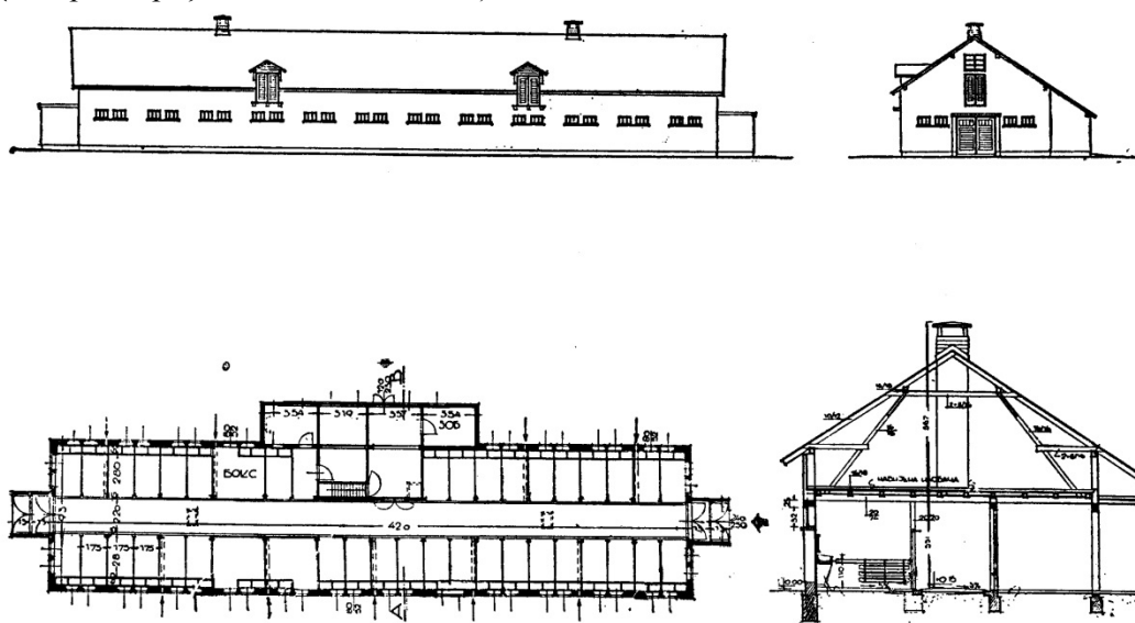
Слика 5. 38 – Типска коњушница за тридесет и осам радних грла са три бокса, са посебном спремницом хране и складиштем за зрнасту храну, Пројектант Р. Кадих, према пројектима пољопривредних зграда Министарства грађевина ФНРЈ, 1950.
