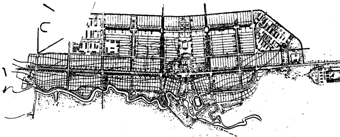
Слика 4.7 - Генерални план сеоског насеља Јурте у колхозу „Гигант“, Новосибирск Аутор: арх. К.И. Трапезников и др. Kazimir Ostrogović, „Arhitektura SSSR 1917. – 1947. Povodom 30. godišnjice Oktobarske revolucije“, Arhitektura, br 4-6 (1947/48): 13.
