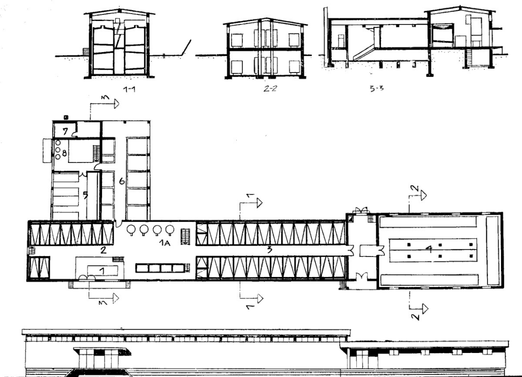
Слика 5. 33 – Полуукопани подрум за вино у селу Рајац капацитета 150 вагона, Према пројекту „Инвест завода“ Београд. Бранислав Којић и Ђорђе Симоновић, Пољопривредне зграде и комплекси (Београд: Грађевинска књига, 1978), 163.
