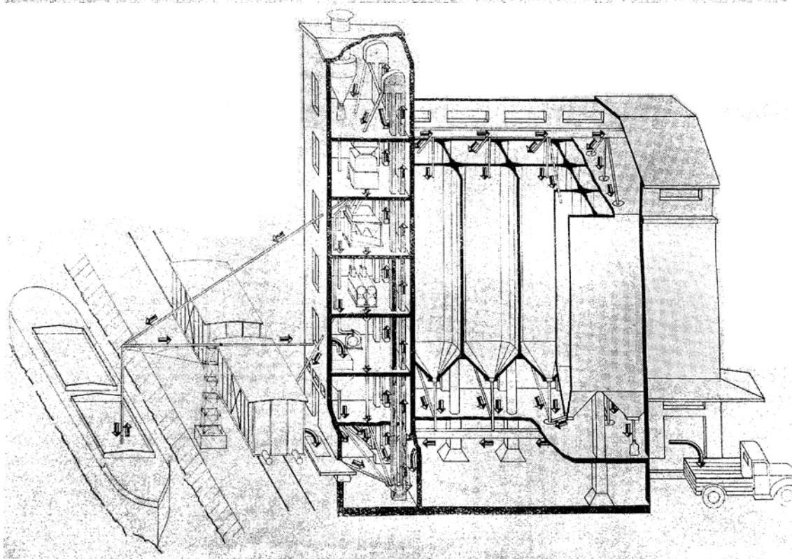
Слика 5.1a - Пресек комбинованог силоса у Сиску.
