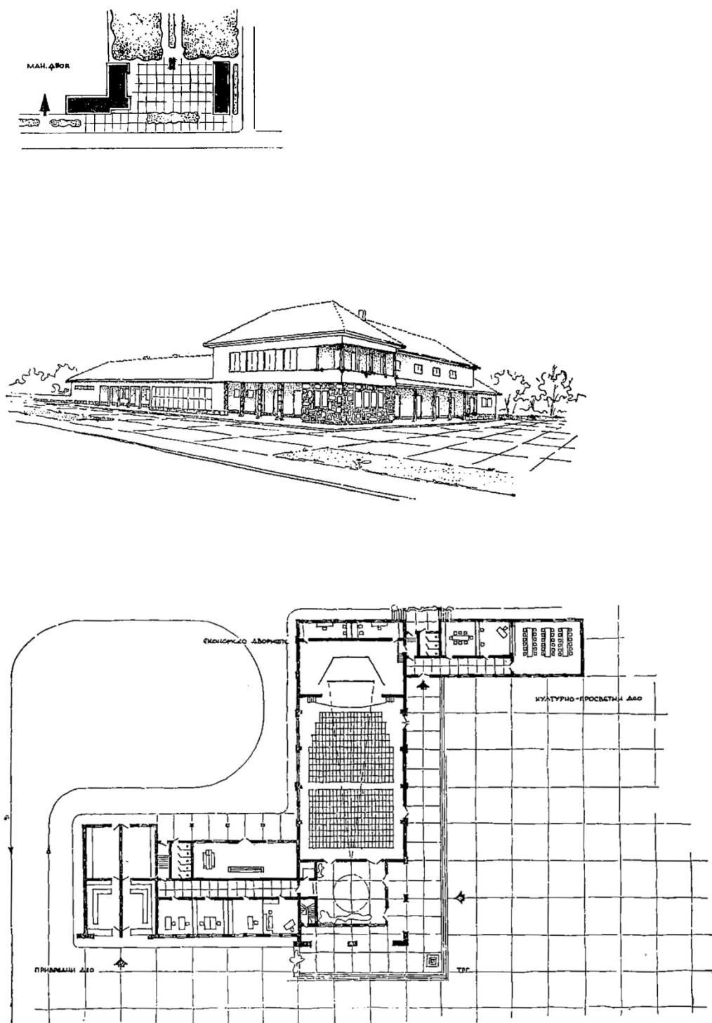
Слика 5.5 - Задружни дом тип 7, арх Никола Гавриловић. Milorad Macura, „Zadružni domovi na teritoriji NR Srbije“, Arhitektura , br. 11-12 (1948): 31.
