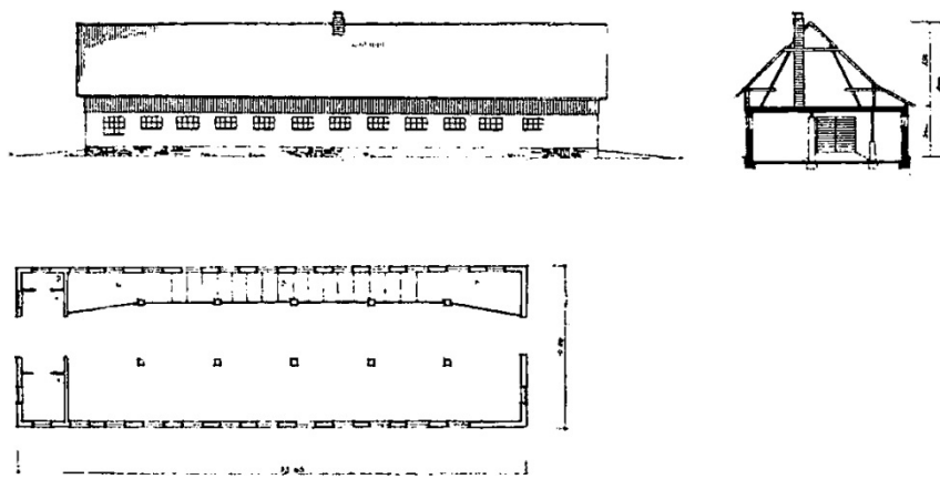
Слика 5. 70 – Тип мање стаје за овце, Пројектант: Звонимир Црнокрак. Zvonimir Crnokrak „Ovčarnici“, Urbanizam-Arhitektura , br. 9-12 (1951): 29.
