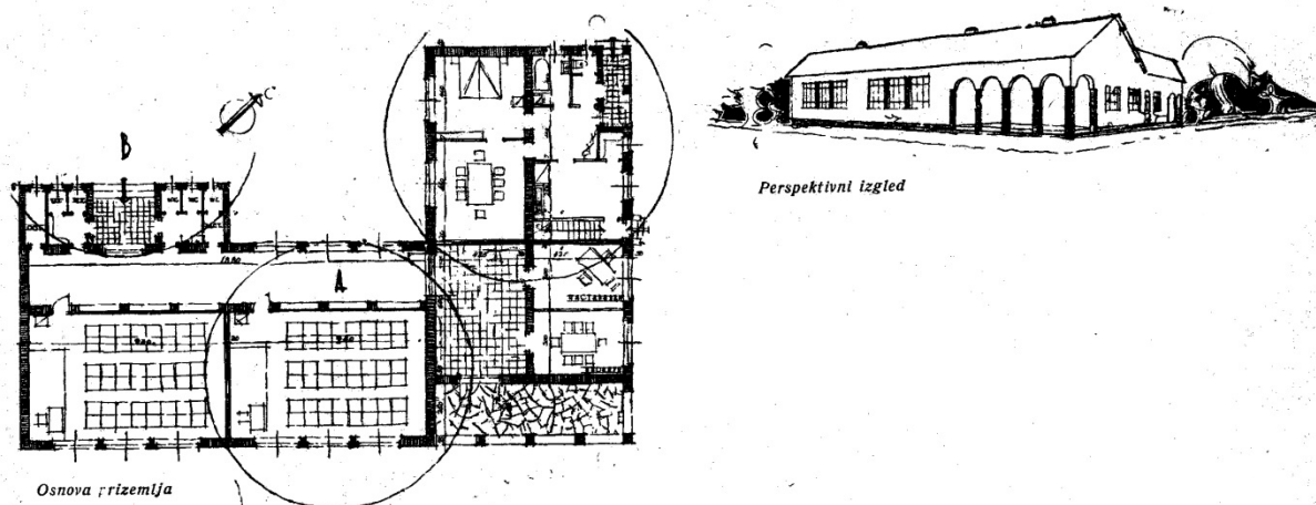
Слика 5. 21 – Тип сеоске основне школе са два разреда за равничарске пределе,
