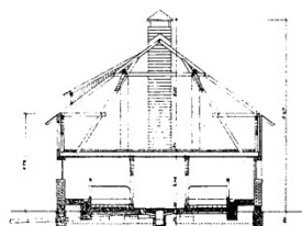
Слика 5. 61 – Тип стаје за телад са кравама хранилишћима, Пројектант: Звонимир Црнокрак. Zvonimir Crnokrak „Staje za goveda“, Urbanizam-Arhitektura , br. 9-12 (1951): 19.
