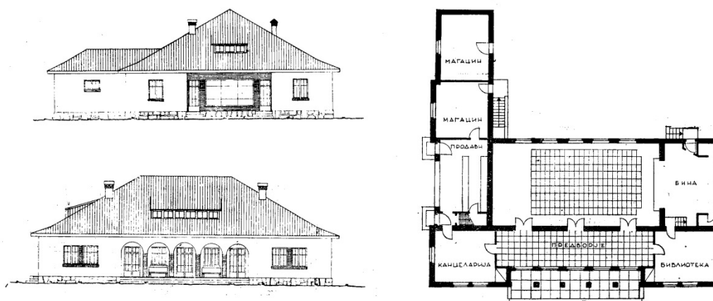
Слика 5.11 - Задружни дом тип 1, архитект Димитрије Маринковић.
