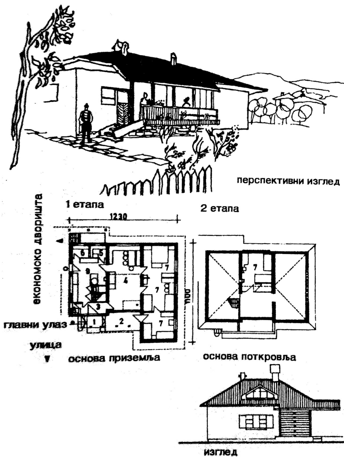
Слика 4.15 – Предлог за типски план сеоске куће у равници, 1954. Пројектант: арх. Бранислав Миленковић Ђорђе Симоновић и Милорад Рибар, Уређење сеоских насеља и територија (Београд: ИБИ, 1993), 141.
