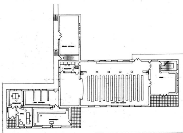
Tloort prizemlja • План нижнего этажа • Plan du rez-de-chaussée
