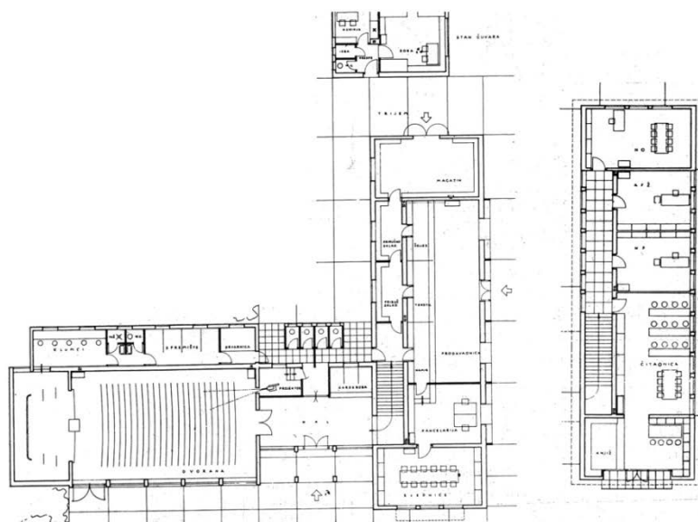
Слика 5.8 - Задружни дом тип 9, арх Божидар Тушек. „Tipovi zadružnih domova u NRH“, Arhitektura , br. 7 (1948):15.
