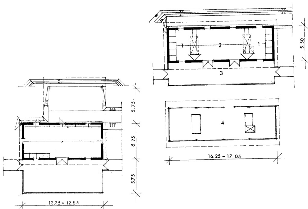
Слика 5. 46 – Типски пројекат овчарника за 50 оваца на планинском терену, Према типском пројекту бироа „Наш стан – ИАУС“ Београд Бранислав Којић и Ђорђе Симоновић, Пољопривредне зграде и комплекси (Београд: Грађевинска књига, 1978), 361.
