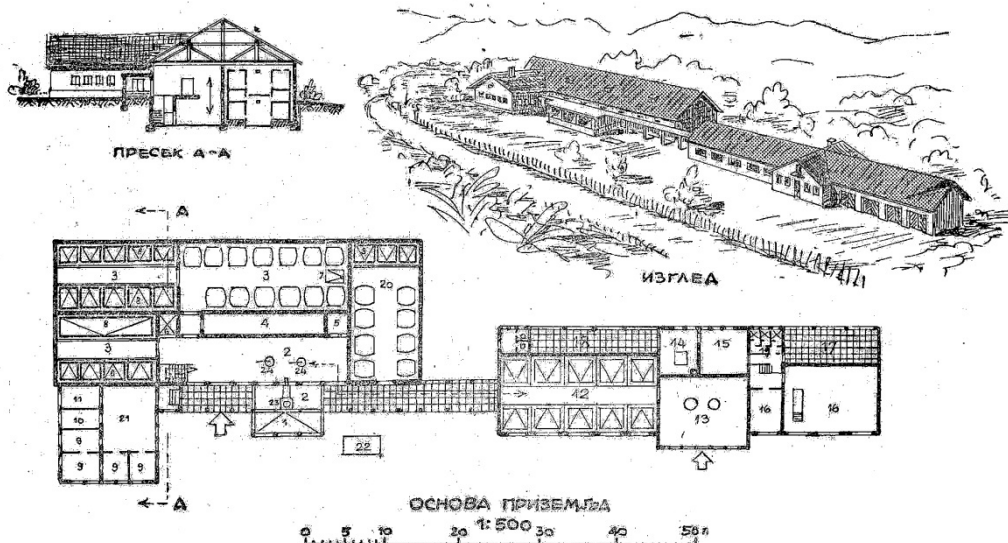
Слика 5. 55 – Винарски подрум у Рековцу, Пројектант: Предраг Зрнић. Предраг Зрнић, „Подаци за пројектовање винарских подрума“, Зборник Архитектонског факултета, књига III, свеска 11 (1956/57): 3.
