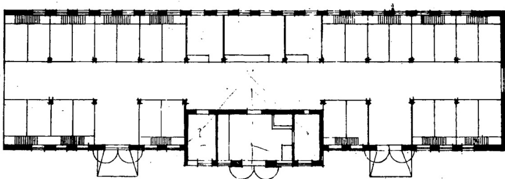
Слика 5. 68 – Идејни пројекат стаје за коње, Пројектант: Звонимир Црнокрак. Zvonimir Pavešić, „Staje za konje“, Urbanizam-Arhitektura , br. 9-12 (1951): 16.
