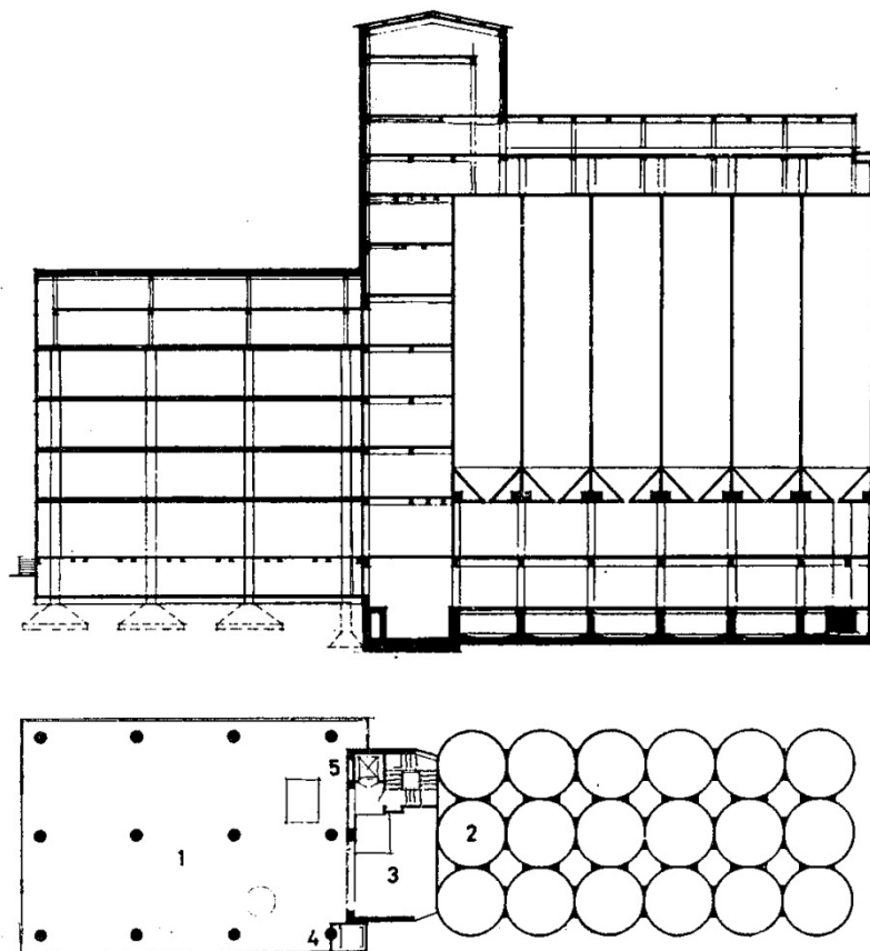
Слика 5.1 г – Силос у Сенти. Бранислав Којић и Ђорђе Симоновић, Пољопривредне зграде и комплекси (Београд: Грађевинска књига, 1978), 76.
