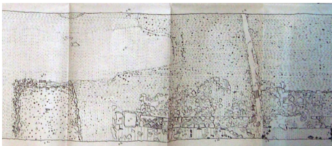
127. GRAĐEVINA ISTOČNO OD FORUMA, SEKTOR B, BLOK III, SONDA 2 UPRAVA ZA KULTURNU BAŠTINU, CETINJE, DUKLJA 1998, CRTEŽ 50 CRTEŽ: T. MIJOVIĆ (1998)
