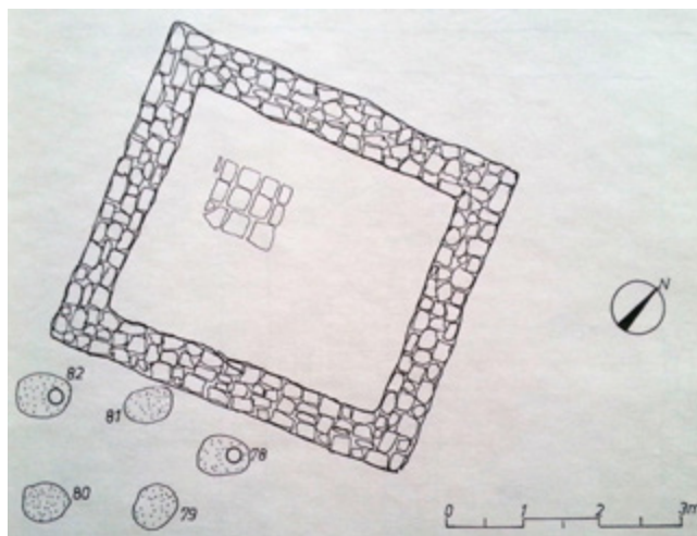
6. JUGOISTOČNA NEKROPOLA, GROBNA KONSTRUKCIJA I A. ЦЕРМАНОВИЋ-КУЗМАНОВИЋ, О. ВЕЛИМИРОВИЋ-ЖИЖИЋ, Д. СРЕЈОВИЋ, АНТИЧКА ДУКЉА. НЕКРОПОЛЕ, ЦЕТИЊЕ 1975, 31, SL. 17.
