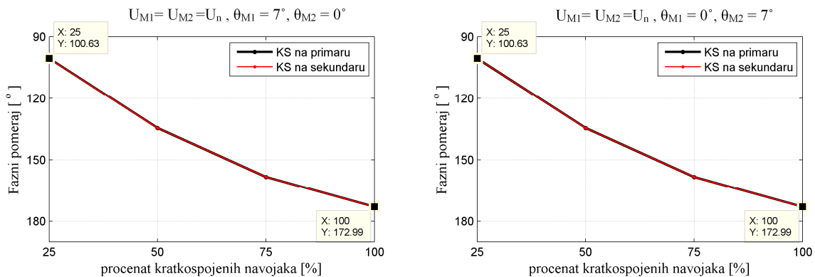
Sl. 3.19 Promena faznog pomeraža u zavisnosti od broja KS-enih navojaka kada je smer aktivne snage: (a) od mreže 1 do mreže 2 i (b) od mreže 2 do mreže 1
