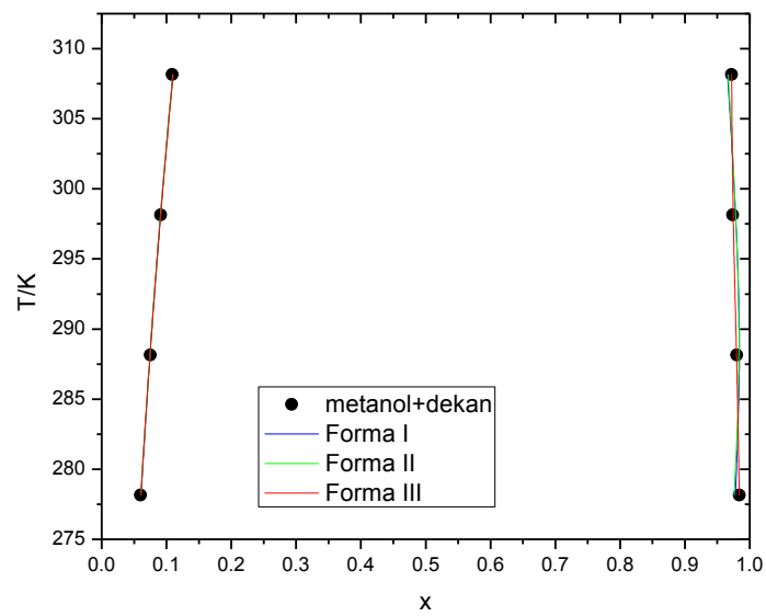
Slika 5.15 metanol+dekan
