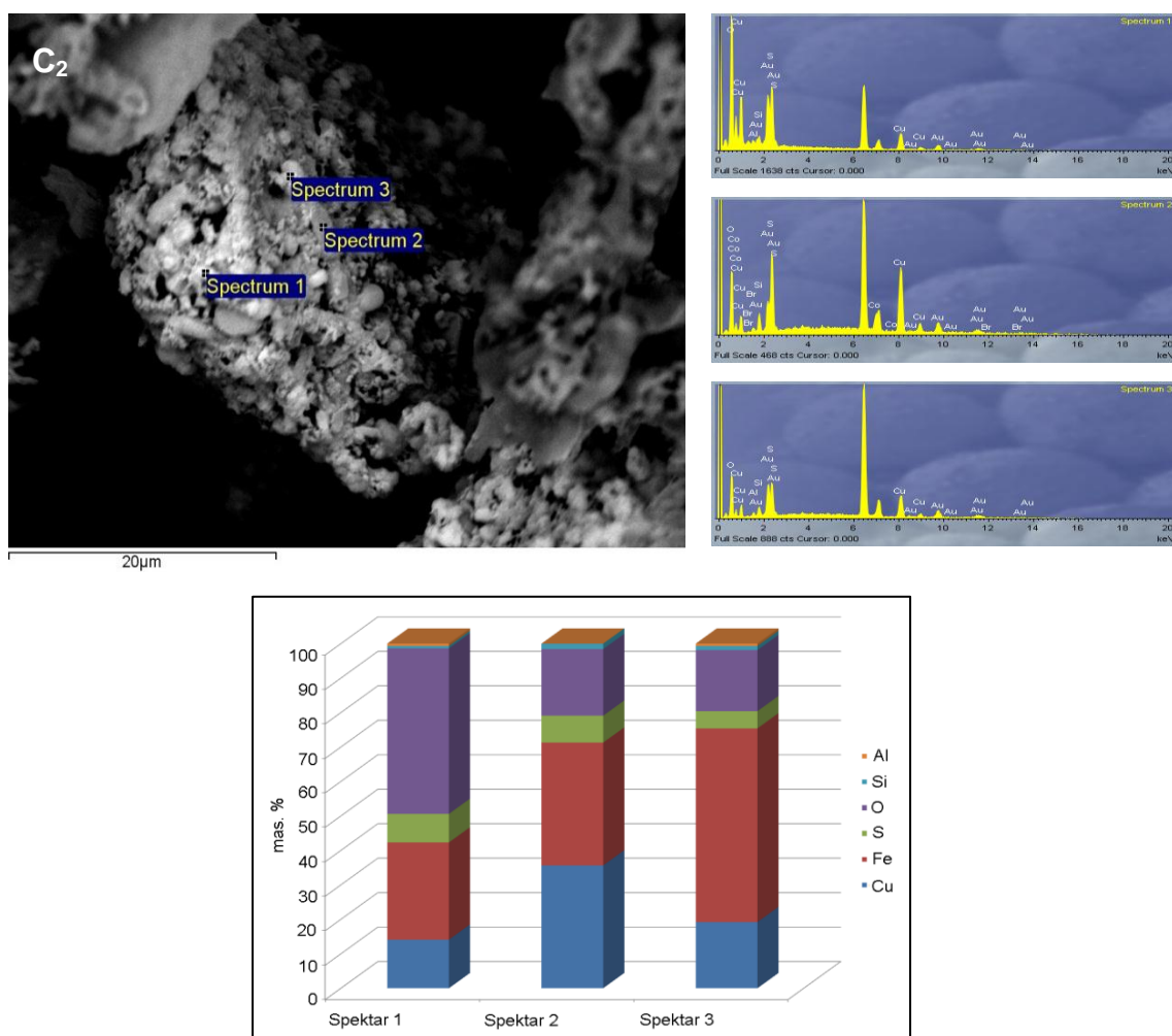
Slika 51. Rezultati SEM/EDS analize uzorka koncentrata C 2 , žarenog 1 h na 675 °C u atmosferi vazduha (SEM mikrofotografija sa EDS spektrom i rezultati kvantitativne analize)
