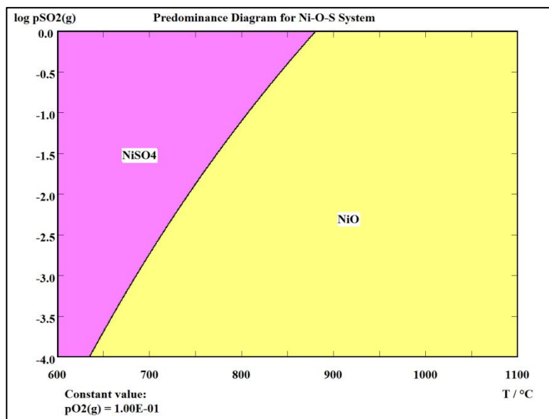
Slika 68. Dijagram stabilnosti faza u Ni-S-O sistemu kao zavisnost \log pSO_2(g) = f(T) , pri konstantnom pritisku kiseonika od 0,1 bar
