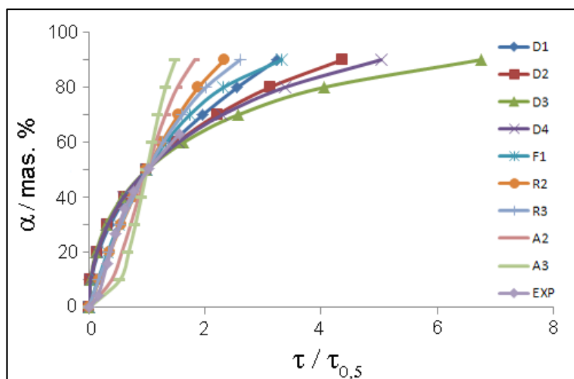
Slika 105. Izbor kinetičkog modela za linearizaciju eksperimentalnih izoterma prema metodi H.J. Sharpa
