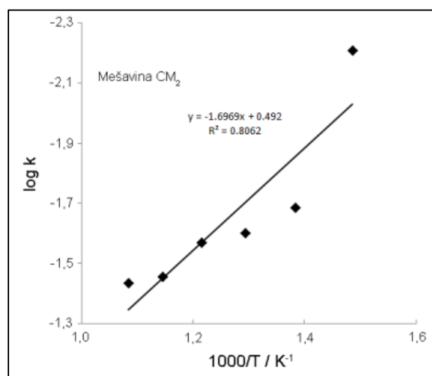
Slika 115. Arrheniusov dijagram za proces oksidacije mešavine CM_2
