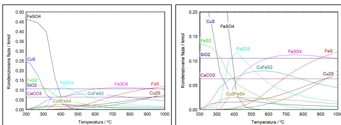
Slika 74. Dijagram ravnotežnog sastava u sistemu koncentrat A + gas (71 % N_2 , 19 % O_2 , 10 % SO_2 ) u zavisnosti od temperature pri molskom odnosu gas : šarža = 10 : 1, pri pritisku gasa od 1 bar
