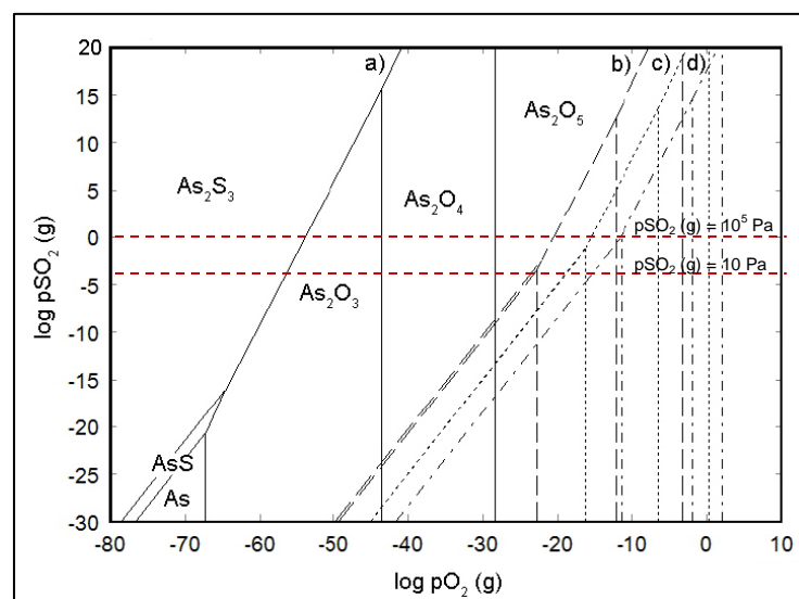
Slika 69. Dijagram stabilnosti faza u As-S-O sistemu na 25 °C (a), 450 °C (b), 650 °C (c) i 900 °C (d) kao zavisnost \log pSO_2 = f(\log pO_2)
