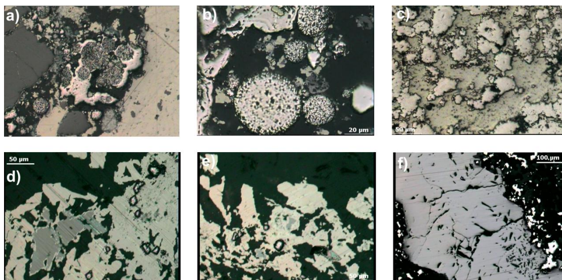
Slika 42. Optička mikroskopija uzorka koncentrata B_0
