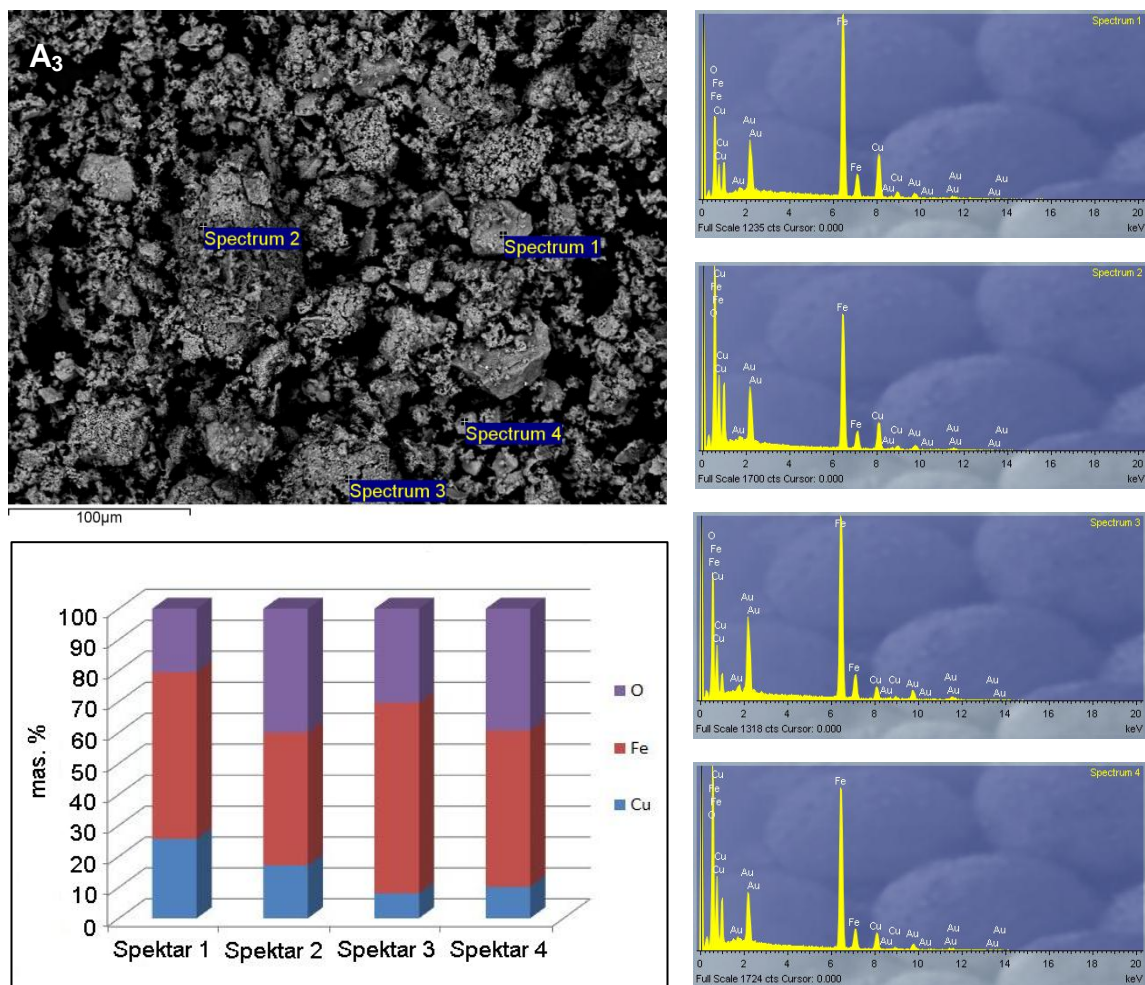
Slika 39. SEM/EDS analiza uzorka koncentrata A 3 žarenog 1 h na 900 °C u atmosferi vazduha (SEM mikrofotografija sa EDS spektrom i rezultati kvantitativne analize)
