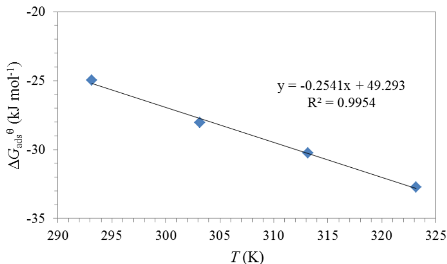
Slika 49. Zavisnost \Delta G_{ads}^{\theta} određene iz Tjomkinove adsorpcione izoterme za adsorpciju TOFA/DETA imidazolina na površini niskougličnog čelika u temperaturnom opsegu od 293 K do 323 K.
