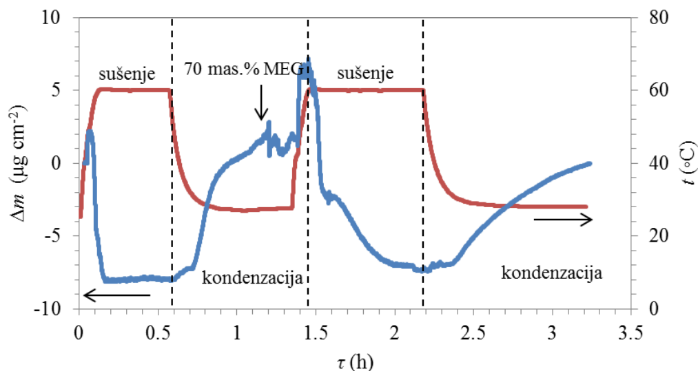
Slika 58. Vremenska zavisnost \Delta m i temperature, merena kvarcnom mikro vagom u gasovitoj fazi rastvora 3 mas. % NaCl zasićenog sa \text{CO}_2 u prisustvu 70 mas. % MEG.
