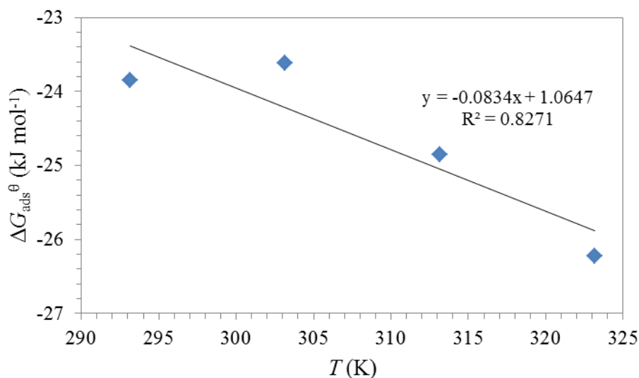
Slika 48. Zavisnost \Delta G_{ads}^{\theta} određene iz Lengmirove adsorpcione izoterme za adsorpciju TOFA/DETA imidazolina na površini niskougleničnog čelika u temperaturnom opsegu od 293 K do 323 K.
