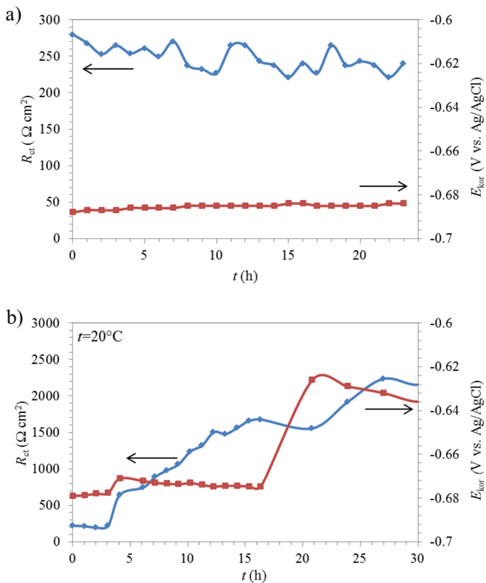
Slika 33. Vrednost polarizacione otpornosti, R_{ct} , i potencijala otvorenog kola, E_{kor} , čelika od vremena delovanja 3 mas. % NaCl, na temperaturi od 20°C: a) bez inhibitora i b) u prisustvu 90 ppm v inhibitora, TOFA/DETA imidazolina.
