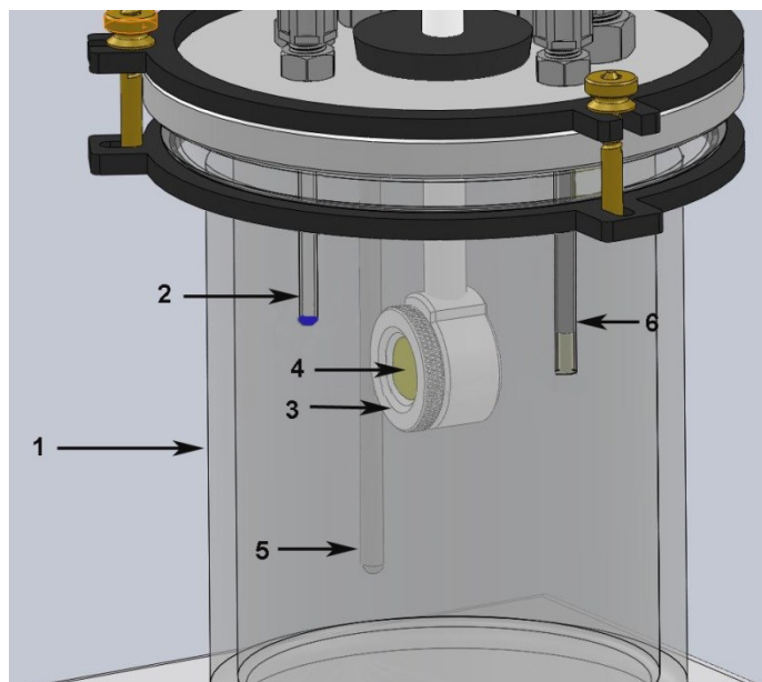
Slika 20. Shema aparature za ispitivanje adsorpcije inhibitora korozije na površini metala (1 –staklena ćelija, 2 –pH metar, 3 –nosač kristala kvarcne mikro vage, 4 –kristal kvarca, 5 – temperaturna sonda, 6 – frita za CO 2 ) (autor: Institute for Corrosion and Multiphase Technology, Ohio).
