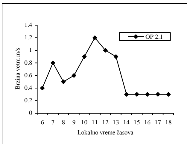
Grafikon 105: Dnevni hod brzine vetra
