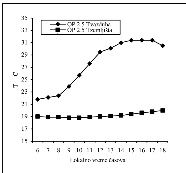
Grafikon 83: Dnevni hod temperature vazd. i zemljišta
