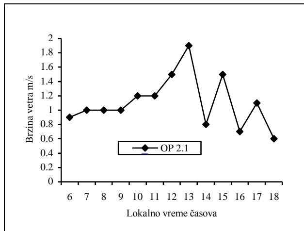
Grafikon 70: Dnevni hod brzine vetra
