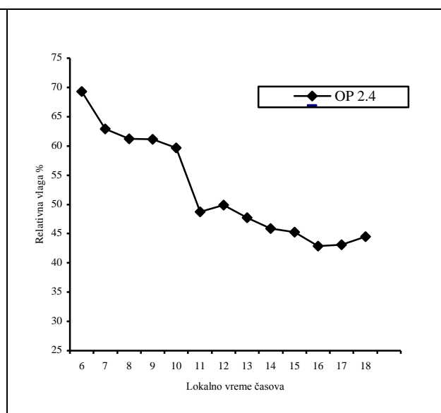
Grafikon 79: Dnevni hod relativne vlažnosti vazduha
