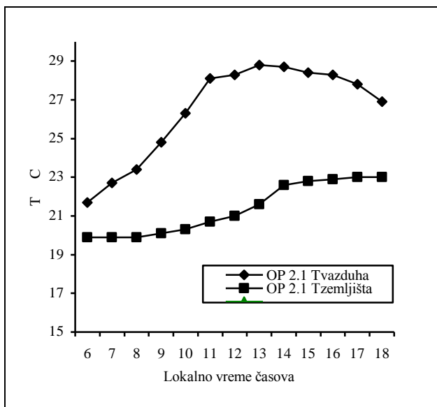
Grafikon 103: Dnevni hod temperature vazd. i zemljišta
