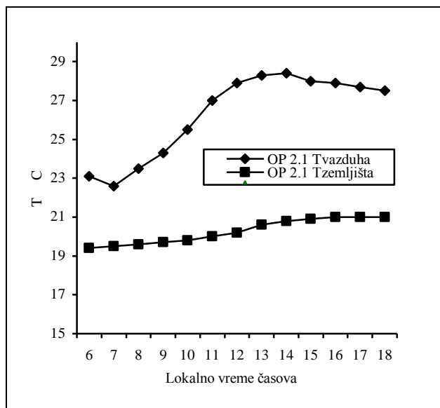
Grafikon 68: Dnevni hod temperature vazd. i zemljišta
