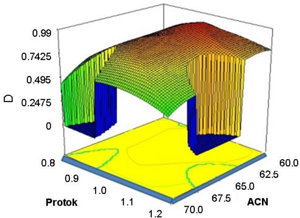
Slika 41. Dijagram 3D globalne funkcije poželjnih odgovora D = f (protok, % ACN); temperatura kolone T = 31,44 \text{ } ^\circ\text{C}
