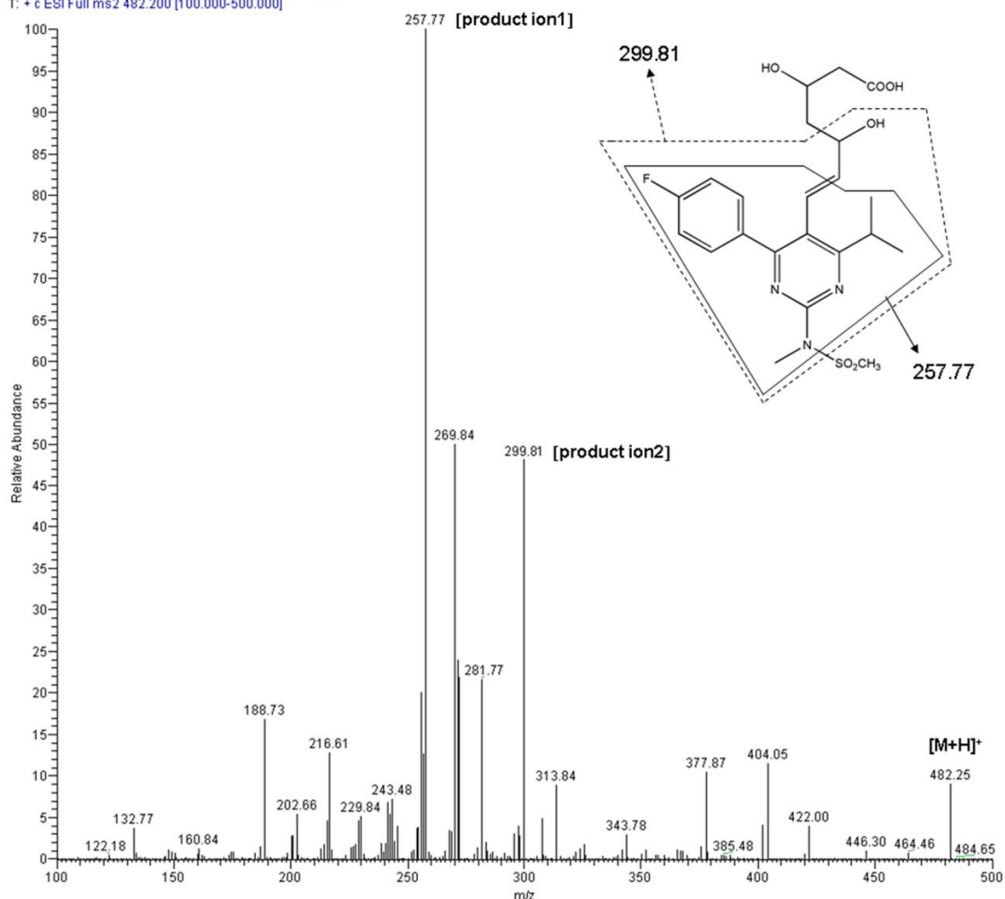
Slika 49. ESI+ maseni spektar produkt jona rosvastatina
