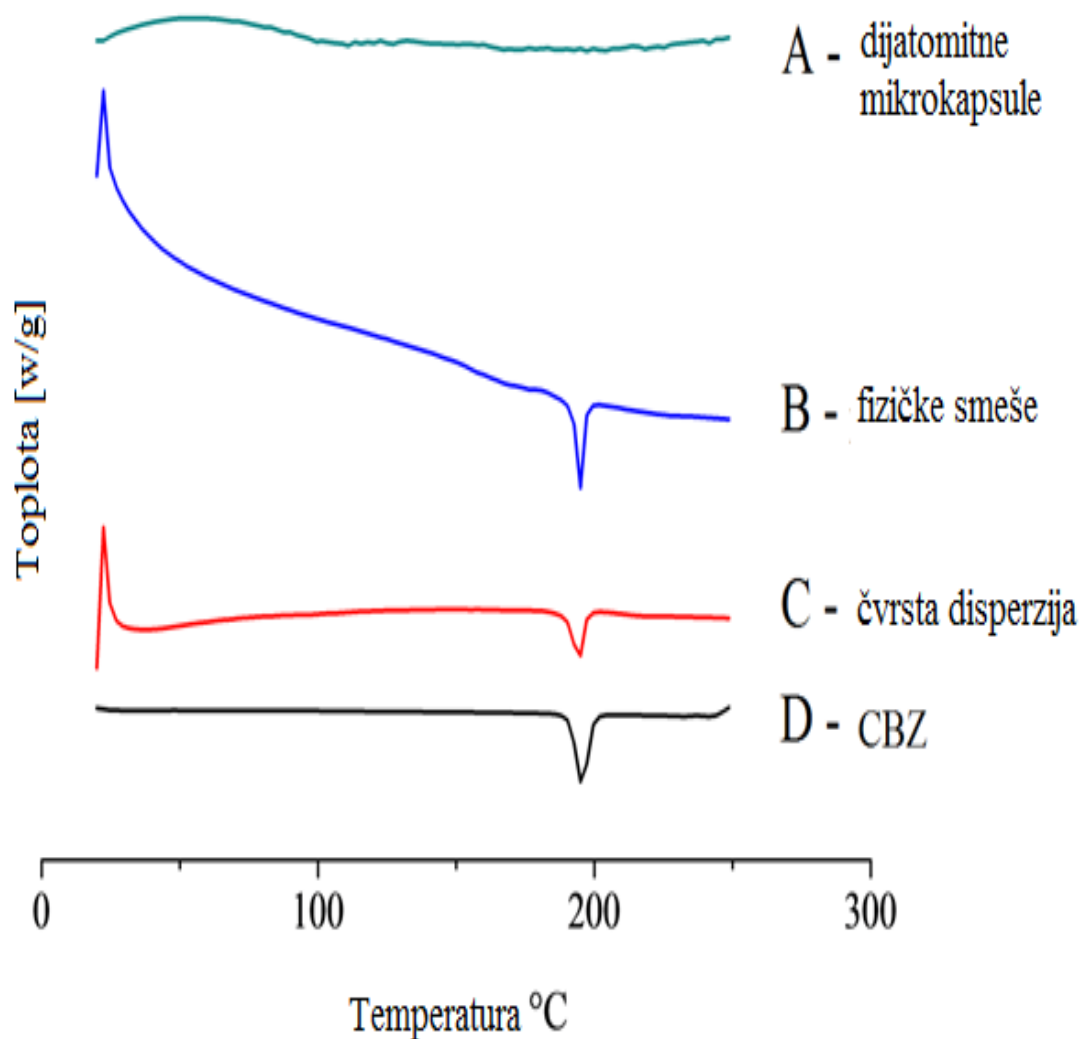
Slika 10.7 - DSC krive različitih formulacija: A – diatomitne mikrokapsule; B – fizička smeša (sadržaj CBZ 20 % (m/m)); C – čvrsta disperzija (sadržaj CBZ 20 % (m/m)); D – CBZ 20 % intenziteta signala
