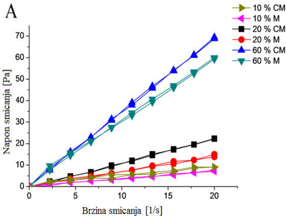
Slika 9.2A - Zavisnost napona smicanja ( \tau ) od brzine smicanja ( \dot{\gamma} ) za voda(V)/polisorbit 80 (S)/PEG-40 hidrogenizovano ricinusovo ulje (C)/trigliceridi srednjeduzine lanca (O) sisteme, SC/O odnos 8:2, K_m 1:1, sa 10, 20 i 60 % V (m/m). M – uzorak bez CBZ; CM - uzorak sa CBZ.
