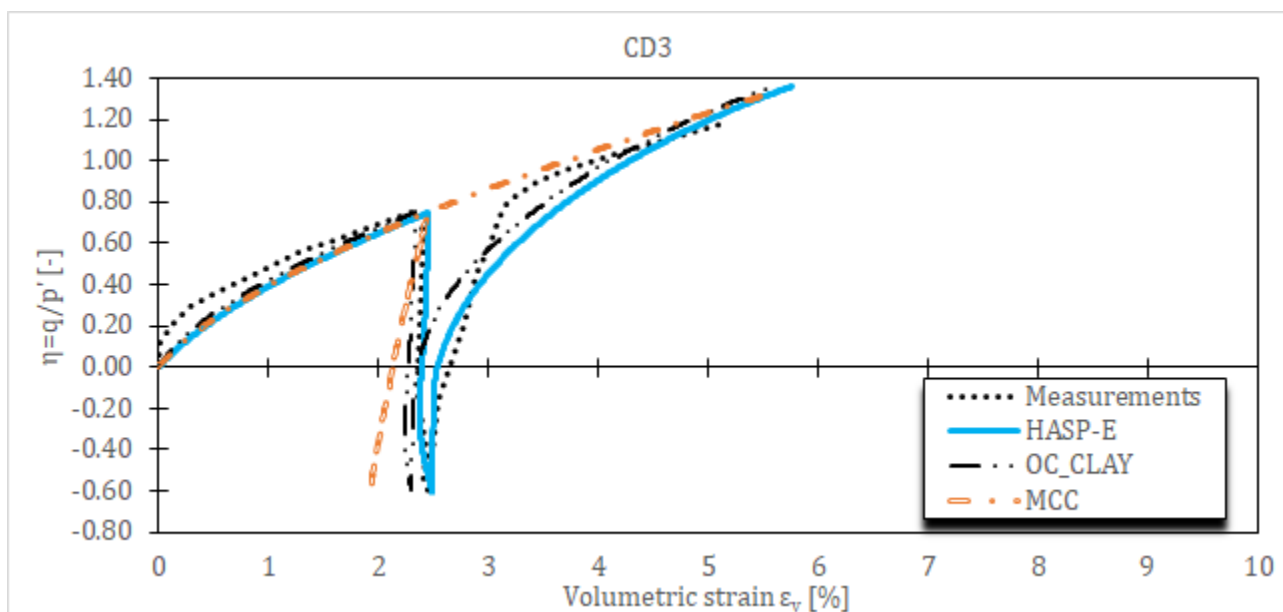
Слика 5-2 Запреминске деформације за CD цикличне триаксијалне опите на Fujinomi глини за различите конститутивне modele и иницијални сет материјалних параметара
