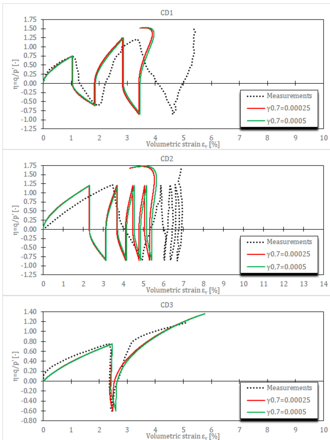
Слика 5-10 Запреминске деформације за CD цикличне триаксијалне опите на Фуџијоториџ глини за HASP-E модел и различите вредности параметра \gamma_{0,7}
