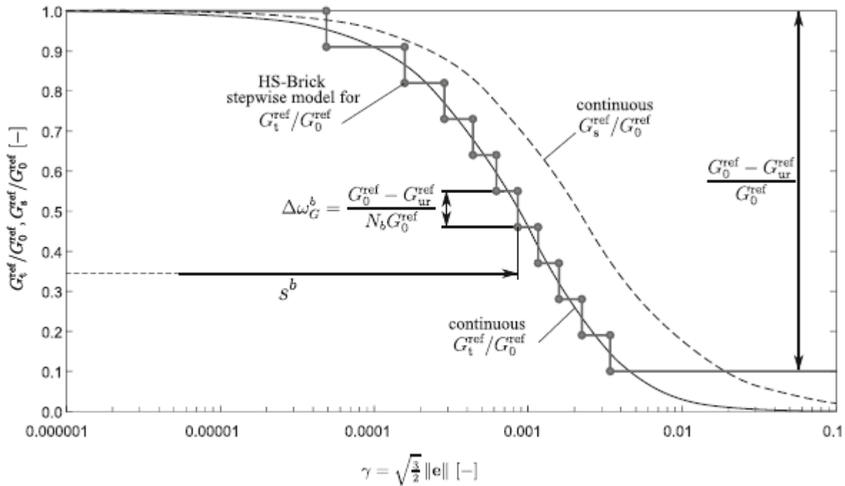
Слика 3-13 Степенаста S-крива у HS-Brick моделу за N_b = 10 цигли – преузето из (Cudny & Truty, 2020)
