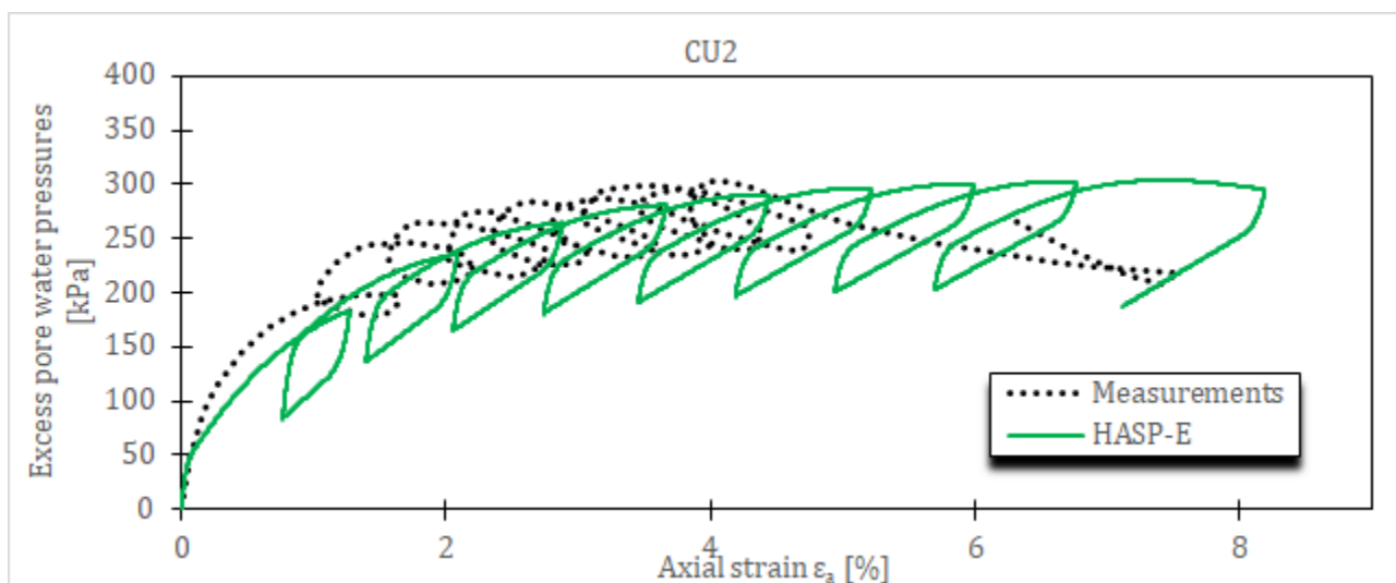
Слика 5-24 Додатни порни притисци за CU цикличне триаксијалне опите на Newfield глине за HASP-E модел и усвојени сет материјалних параметара
