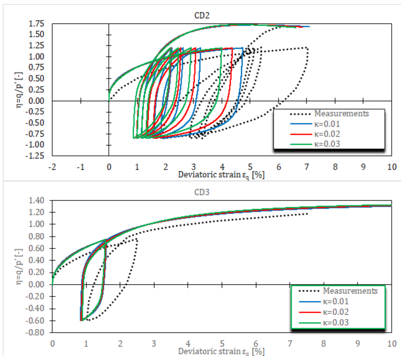
Слика 5-5 Напонско-деформацијске криве за CD цикличне триаксијалне опите на Фуџијотори глини за HASP-E модел и различите вредности параметра \kappa
