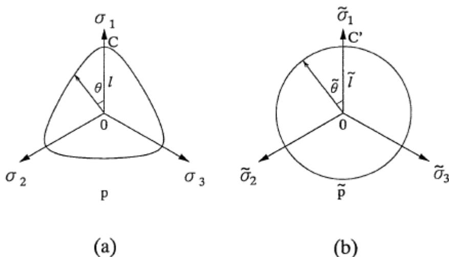
Слика 3-7 SMP критеријум у девијаторској равни: (a) простор главних напона; (b) простор трансформисаних напона – преузето из (Matsuoka, et al., 1999)
