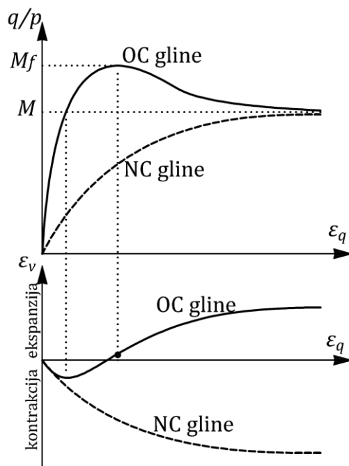
Слика 2-8 Карактеристично понашање преконсолидоване глине у дренираним условима – преузето из (Vukićević & Jocković, 2019)
