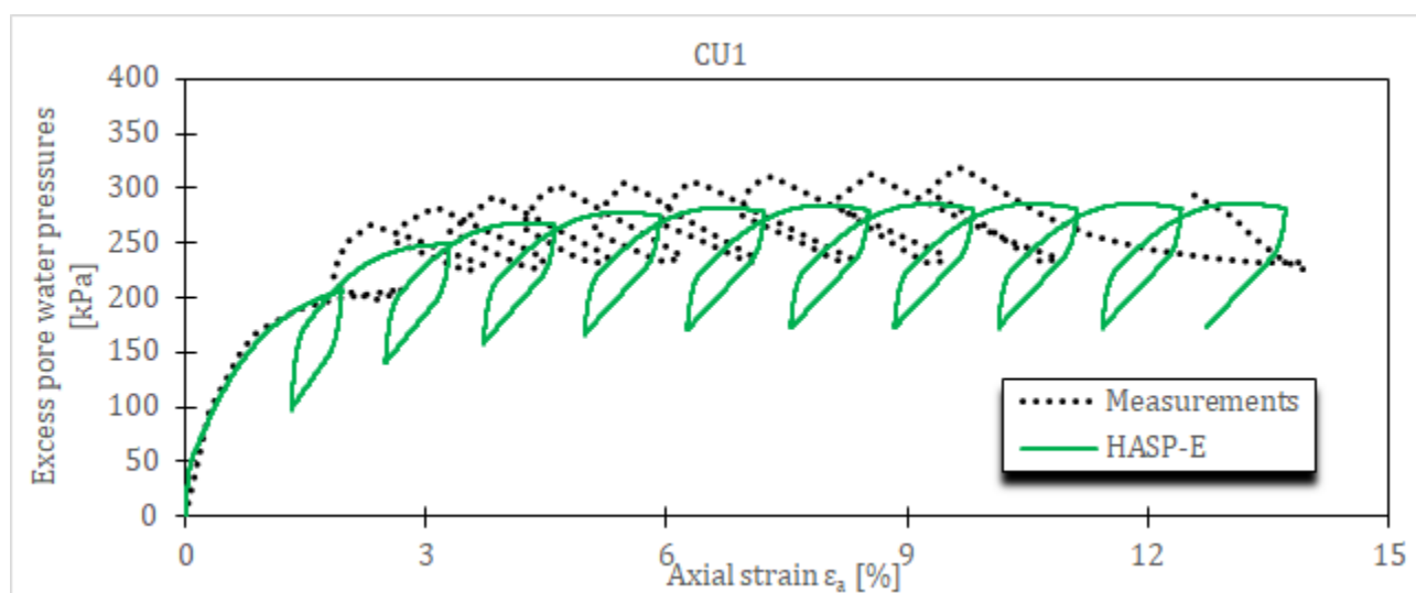
Слика 5-23 Напонско-деформацијске криве за CU цикличне триаксијалне опите на Newfield глини за HASP-E модел и усвојени сет материјалних параметара
