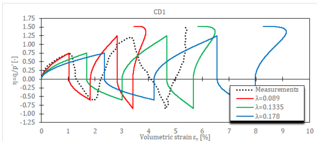
Слика 5-3 Напонско-деформацијске криве за CD цикличне триаксијалне опите на Фујипотори глини за HASP-E модел и различите вредности параметра \lambda
