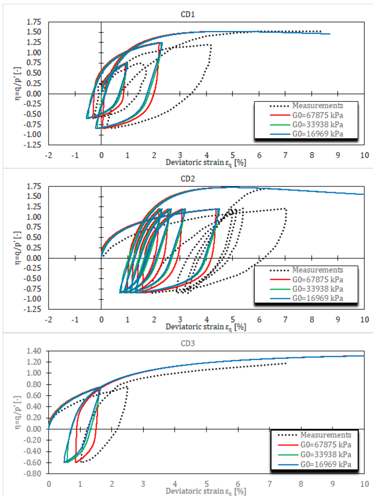
Слика 5-7 Напонско-деформацијске криве за CD цикличне триаксијалне опите на Фуџијодори глини за HASP-E модел и различите вредности параметра G_0^{ref}
