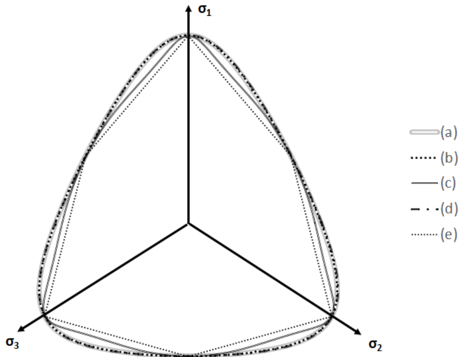
Слика 3-9 Облик критеријума лома у девијаторској равни за \phi_C = \phi_E = \phi_{cv} = 30^\circ за: (a) усвојена зависност M(\theta) и Z = -0.229 , (b) LMN критеријум - израз (3-65), (c) (Zdravković, et al., 2020) са Z = -0.1 , (d) (Sheng, et al., 2000) израз (3-67), (e) Mohr-Coulomb-ов хексагон
