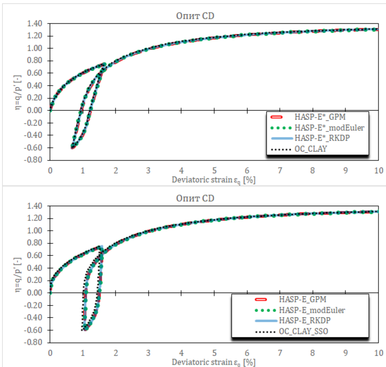
Слика 4-11 Напонско-деформацијске криве за CD циклични триаксијални опит на Fujinotori глине
