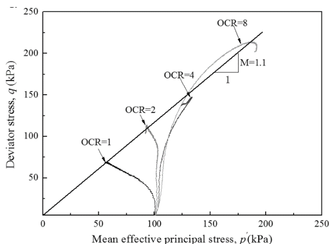
Слика 2-9 Путање ефективних напона у недренираном триаксијалном опиту – преузето из (Gu, et al., 2016)
