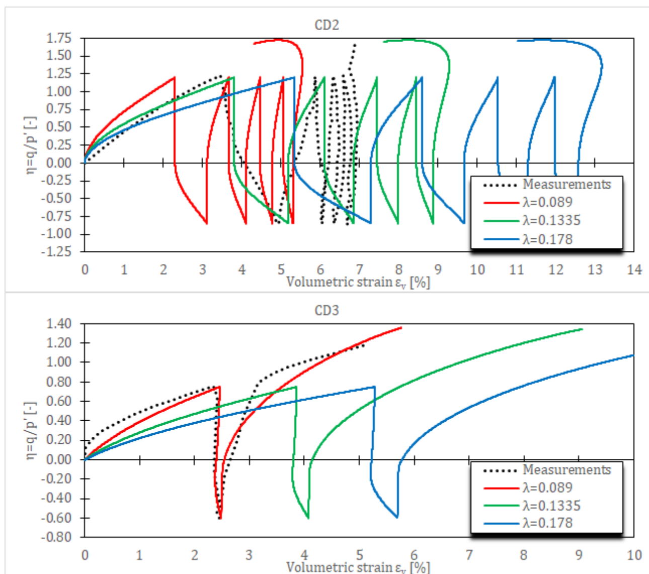
Слика 5-4 Запреминске деформације за CD цикличне триаксијалне опите на Фујинотори глини за HASP-E модел и различите вредности параметра \lambda
