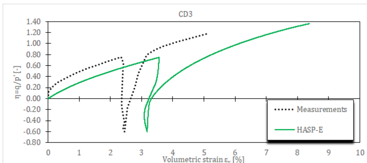
Слика 5-12 Запреминске деформације за CD цикличне триаксијалне опите на Fujinotori глини за HASP-E модел и усвојени сет материјалних параметара
