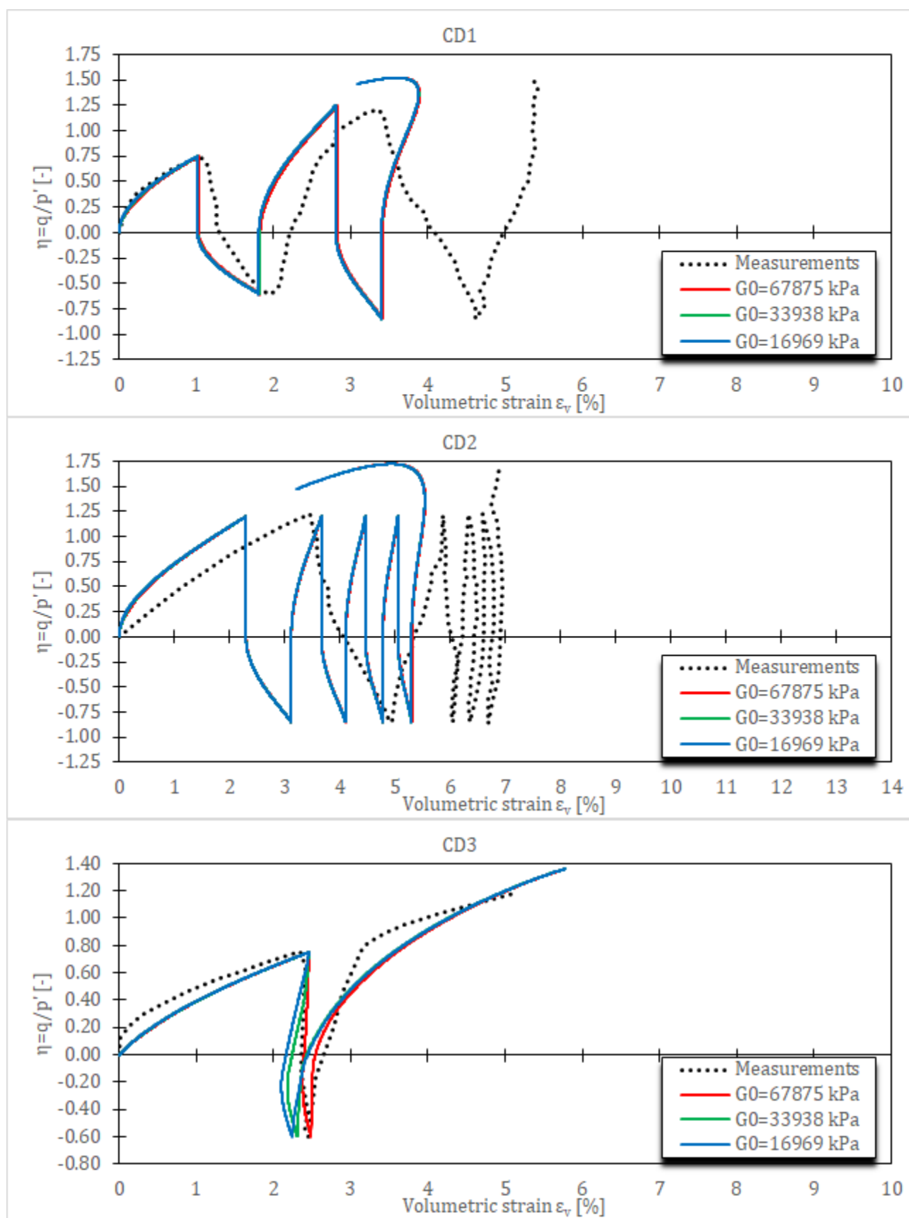
Слика 5-8 Запреминске деформације за CD цикличне триаксијалне опите на Фуџимори глини за HASP-E модел и различите вредности параметра G_0^{ref}
