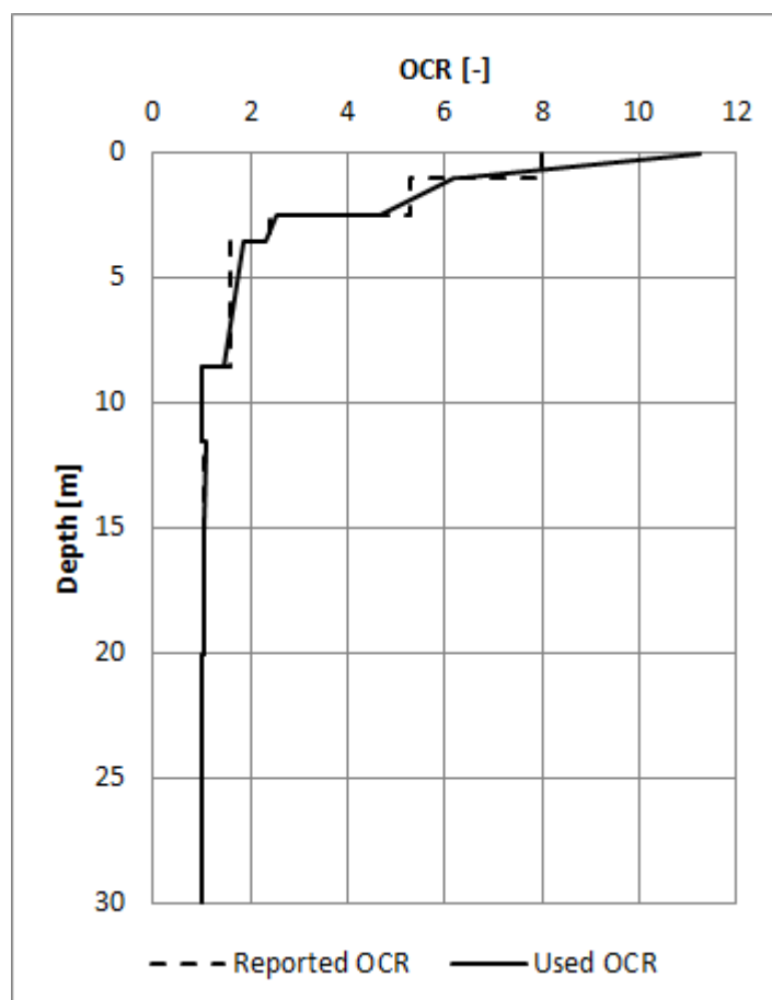
Слика 5-37 Промена степена преkonsolidације са порастом дубине у зависности од вредности параметра POP за Teven Road Trial Embankment
