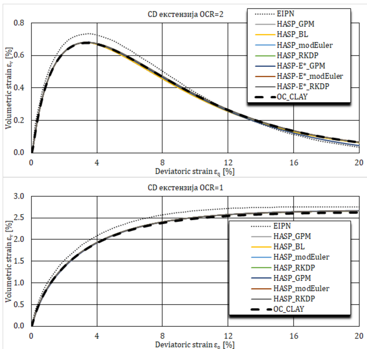
Слика 4-10 Запреминске деформације за CD триаксијалне опите на Fujiyomori глини
