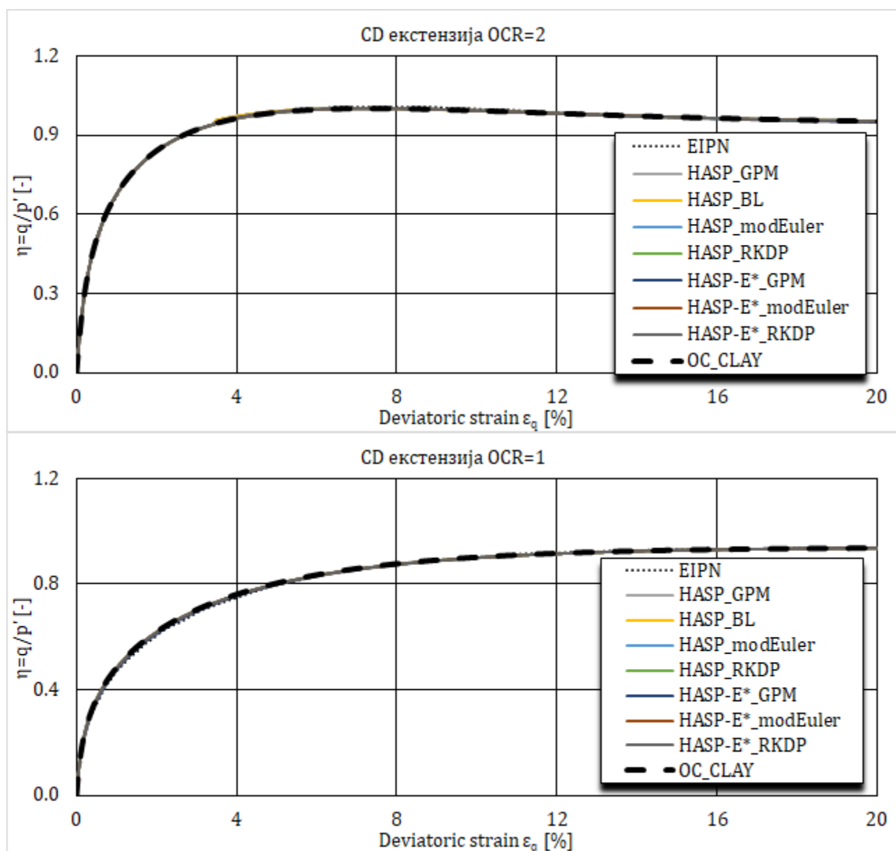
Слика 4-9 Напонско-деформацијске криве за CD триаксијалне опите на Fujinotomori глини
