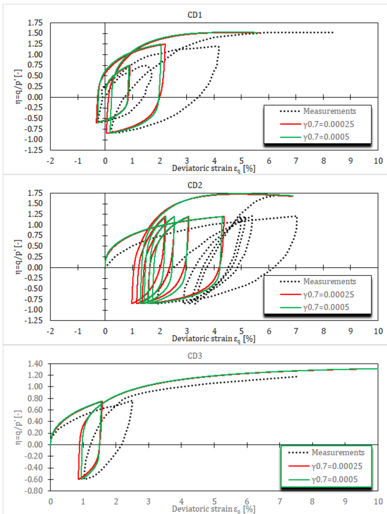
Слика 5-9 Напонско-деформацијске криве за CD цикличне триаксијалне опите на Fujiploti глини за HASP-E модел и различите вредности параметра \gamma_{0,7}
