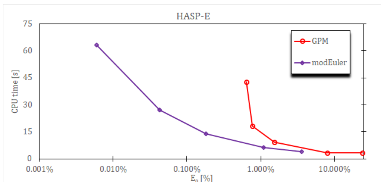
Слика 4-18 Тачност и ефикасност алгоритама за нумеричку интеграцију HASP и HASP-E модела за POP = 100 kPa и различит број инкремената
