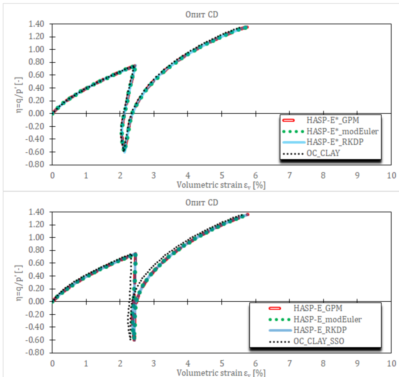
Слика 4-12 Запреминске деформације за CD циклични триаксијални опит на Fujiyomori глини
