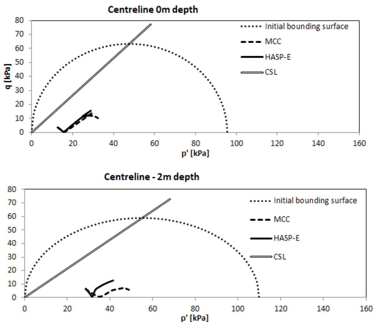
Слика 5-41 Путање ефективних напона за HASP-E и MCC модел испод средине насипа за тачке на површини терена и на дубини од 2 m
