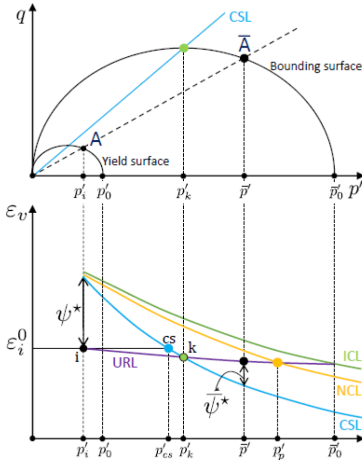
Слика 3-17 Шематски приказ напонско-деформацијског стања у ОС_CLAY моделу – преузето из (Bentley, 2019)
