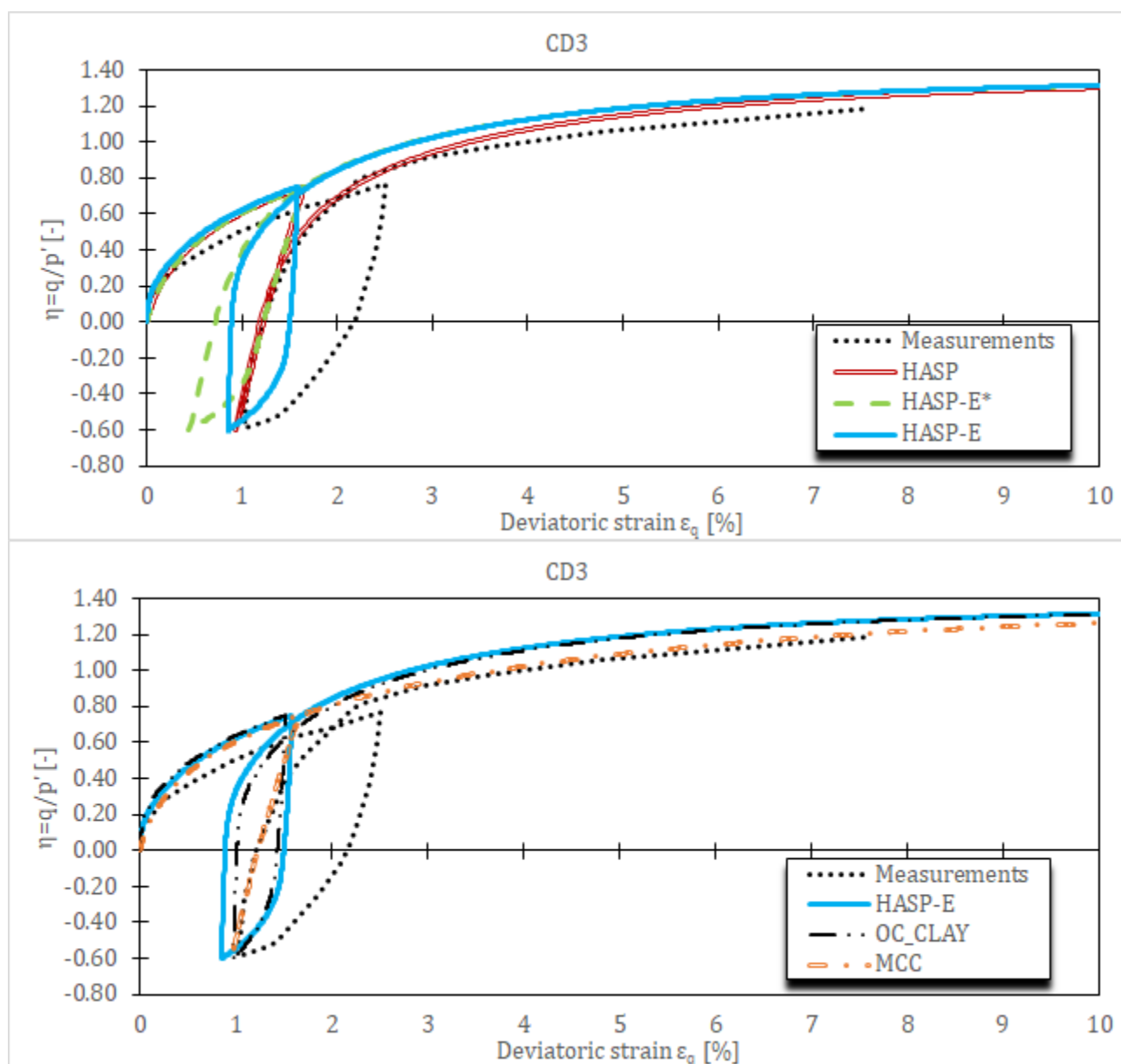
Слика 5-1 Напонско-деформацијске криве за CD цикличне триаксијалне опите на Fijipotori глини за различите конститутивне modele и иницијални сет материјалних параметара
