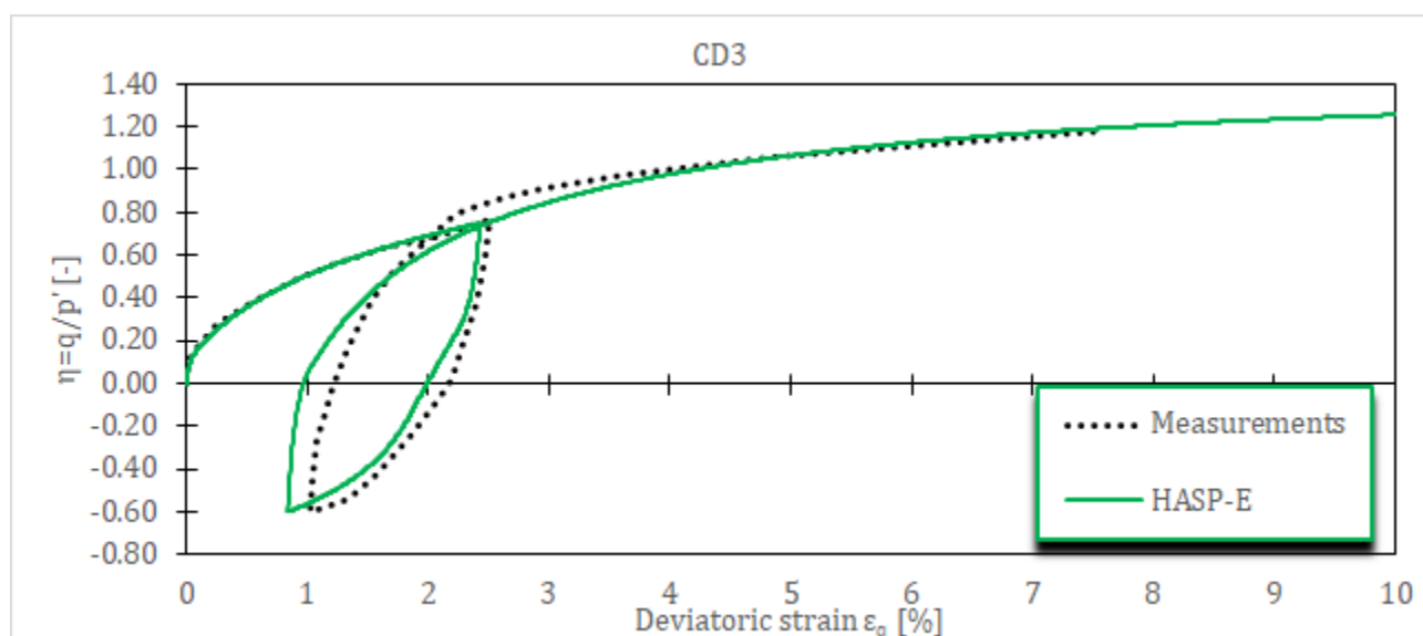
Слика 5-11 Напонско-деформацијске криве за CD цикличне триаксијалне опите на Фујипоторі глини за HASP-E модел и усвојени сет материјалних параметара
