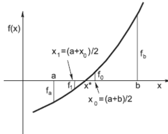
Слика 4-1 Метода бисекције за тражење нуле функције – преузето из (Kojić & Bathe, 2003)
