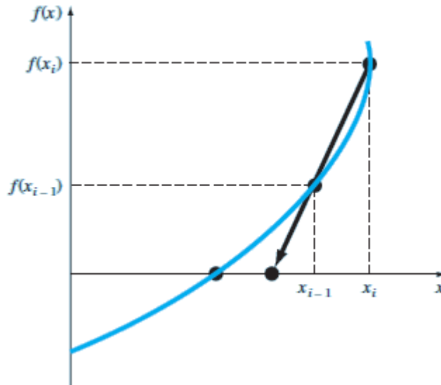
Слика 4-4 Секантна метода за тражење нуле функције – преузето из (Chapra & Canale, 2021)
