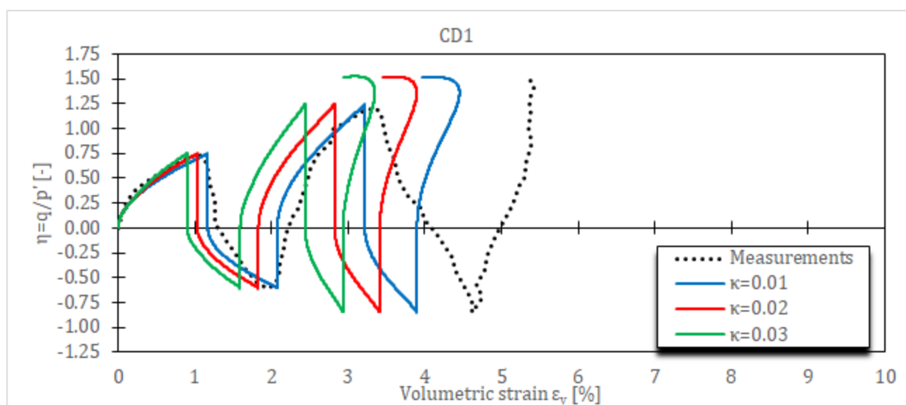
Слика 5-5 Напонско-деформацијске криве за CD цикличне триаксијалне опите на Фуџијотори глини за HASP-E модел и различите вредности параметра \kappa
