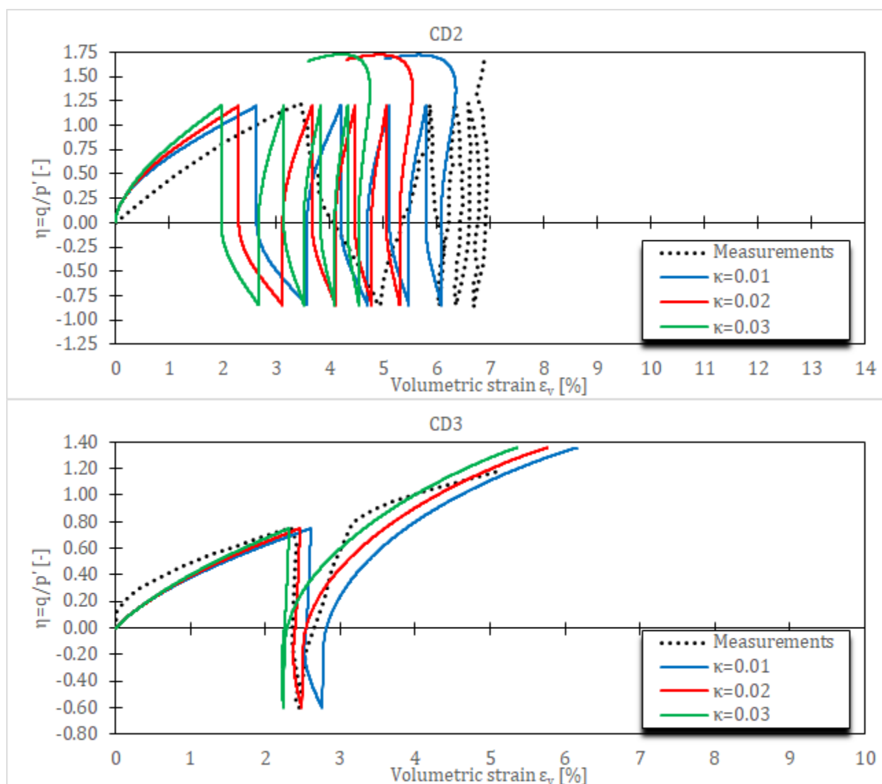
Слика 5-6 Запреминске деформације за CD цикличне триаксијалне опите на Fujinotori глини за HASP-E модел и различите вредности параметра \kappa
