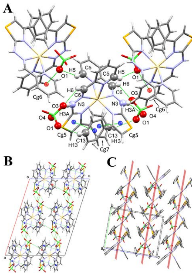
Slika 31. (A) Interakcije odgovorne za formiranje kristalnog pakovanja kompleksa 1–Se . (B) 2D sloj koji je paralelan ac ravni. (C) Međusobno paralelni 2D slojevi koji formiraju 3D kristalno pakovanje. Zbog preglednosti atomi vodonika su uklonjeni iz prikaza.
