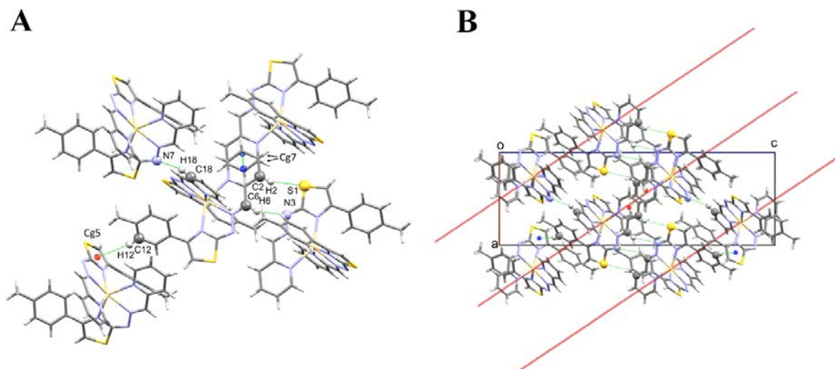
Slika 39. (A) Interakcije odgovorne za formiranje kristalnog pakovanja kompleksa 8-S . (B) 2D sloj koji je paralelan ac kristalografskoj ravni.
