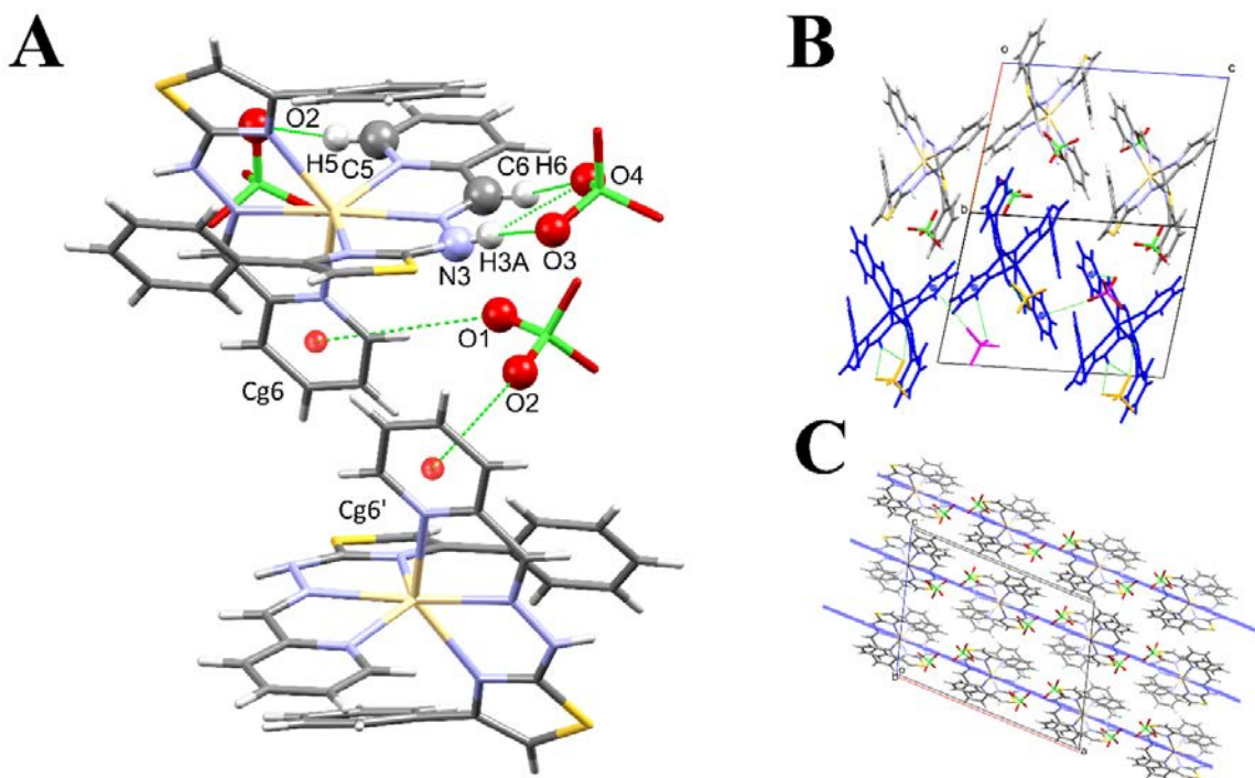
Slika 26. (A) Interakcije odgovorne za formiranje kristalnog pakovanja u kompleksu 1-S . (B) 2D sloj paralelan ravni (0 0 1). (C) Međusobno paralelni 2D slojevi koji formiraju 3D kristalno pakovanje.
