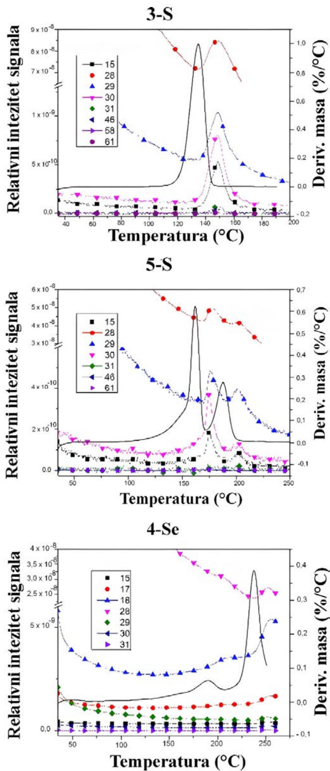
Slika 50. Pikovi koji potiču od 1,4-dioksana i nitrometana ( m/z vrednosti su date na grafiku) nastalih dekompozicijom 3-S i 5-S (crna boja) i pikovi karakteristični za 1,4-dioksan i vodu nastalih dekompozicijom 4-Se (crna boja).
