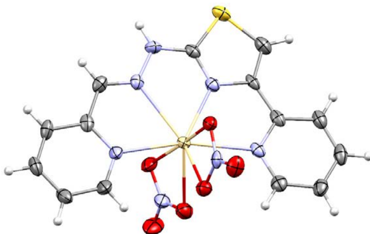
Slika 13. ORTEP prikaz molekulske strukture kompleksa [Cd(L1)(NO_3)_2] . Termalni elipsoidi su prikazani sa 50 % verovatnoće. Sivom bojom predstavljeni su atomi ugljenika, belom bojom atomi vodonika, ljubičastom bojom atomi azota, žutom bojom atom sumpora, crvenom bojom atomi kiseonika i oker bojom atom kadmijuma.
