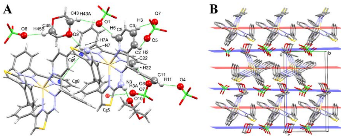
Slika 28. (A) Interakcije odgovorne za formiranje kristalnog pakovanja kompleksa 3-S . (B) 2D slojevi koji su paralelni ab ravni. Zbog preglednosti atomi vodonika su uklonjeni iz prikaza.
