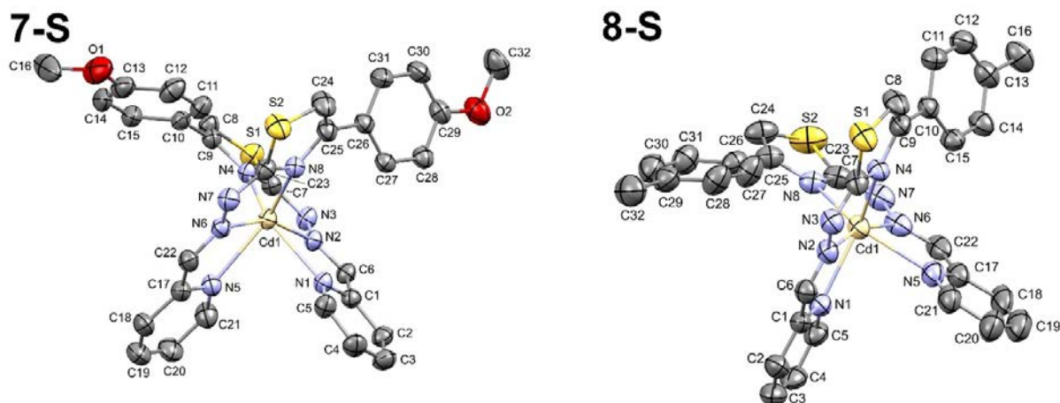
Slika 25. ORTEP prikazi molekulskih struktura kompleksa 7-S i 8-S sa oznakama atoma. Termalni elipsoidi su prikazani sa 30 % verovatnoće. Zbog preglednosti atomi vodonika nisu prikazani u svim strukturama.
