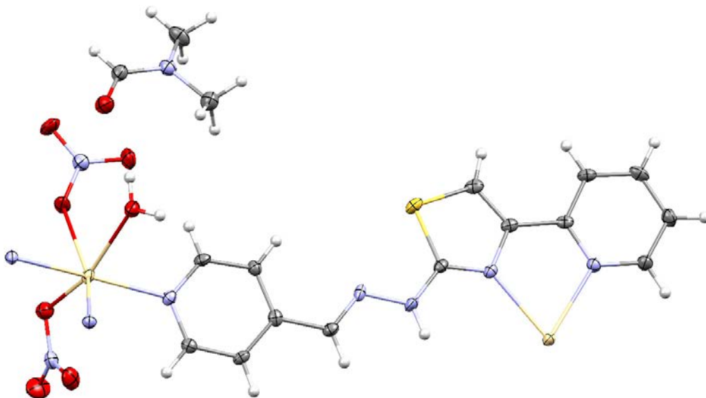
Slika 15. ORTEP prikaz dela molekulske strukture kompleksa 5 . Termalni elipsoidi su prikazani sa 50 % verovatnoće. Sivom bojom predstavljeni su atomi ugljenika, belom bojom atomi vodonika, ljubičastom bojom atomi azota, žutom bojom atom sumpora, crvenom bojom atomi kiseonika i oker bojom atom kadmijuma.
