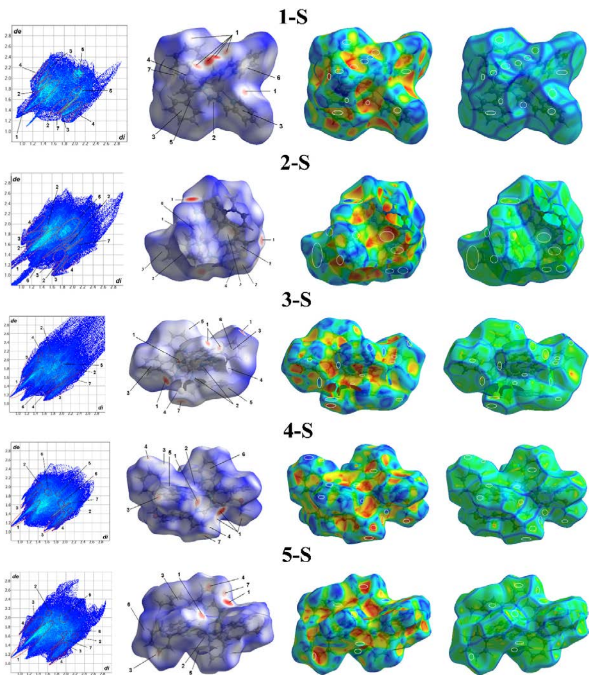
Slika 40. 2D grafikoni otisaka prsta međumolekulskih interakcija i Hiršfeldove površine mapirane sa d_{norm} , indeksom oblika i zakrivljenosti za komplekse (1–5)–S.
