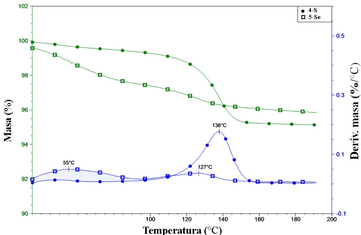
Slika 47. TG i DTG krive za kompleks 4-S i 5-Se snimljene u struji argona. Zelenom bojom označene su TG krive, a plavom bojom DTG krive.
