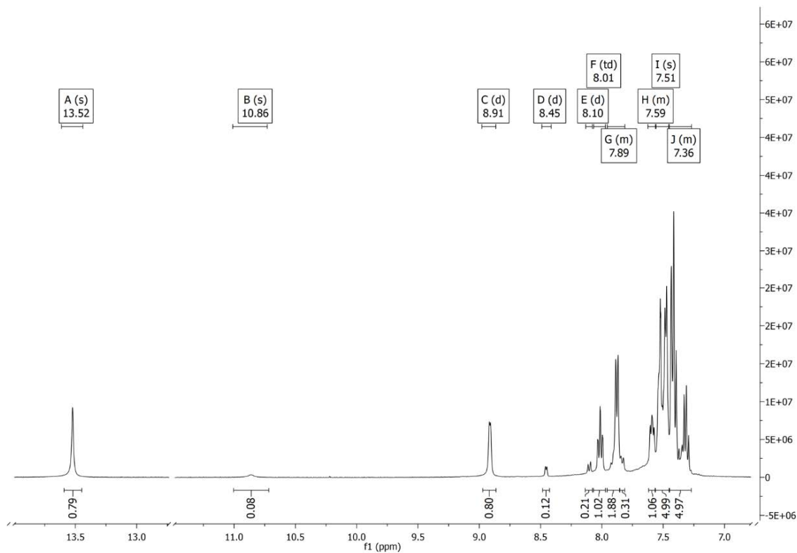
Slika P27. ^1\text{H} NMR spektar HLS 4 snimljen u \text{DMSO-}d_6 .
