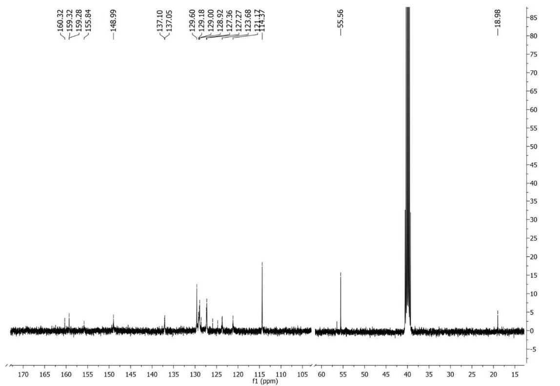
Slika P55. ^{13}\text{C} NMR spektar 4-S snimljen u \text{DMSO-}d_6 .
