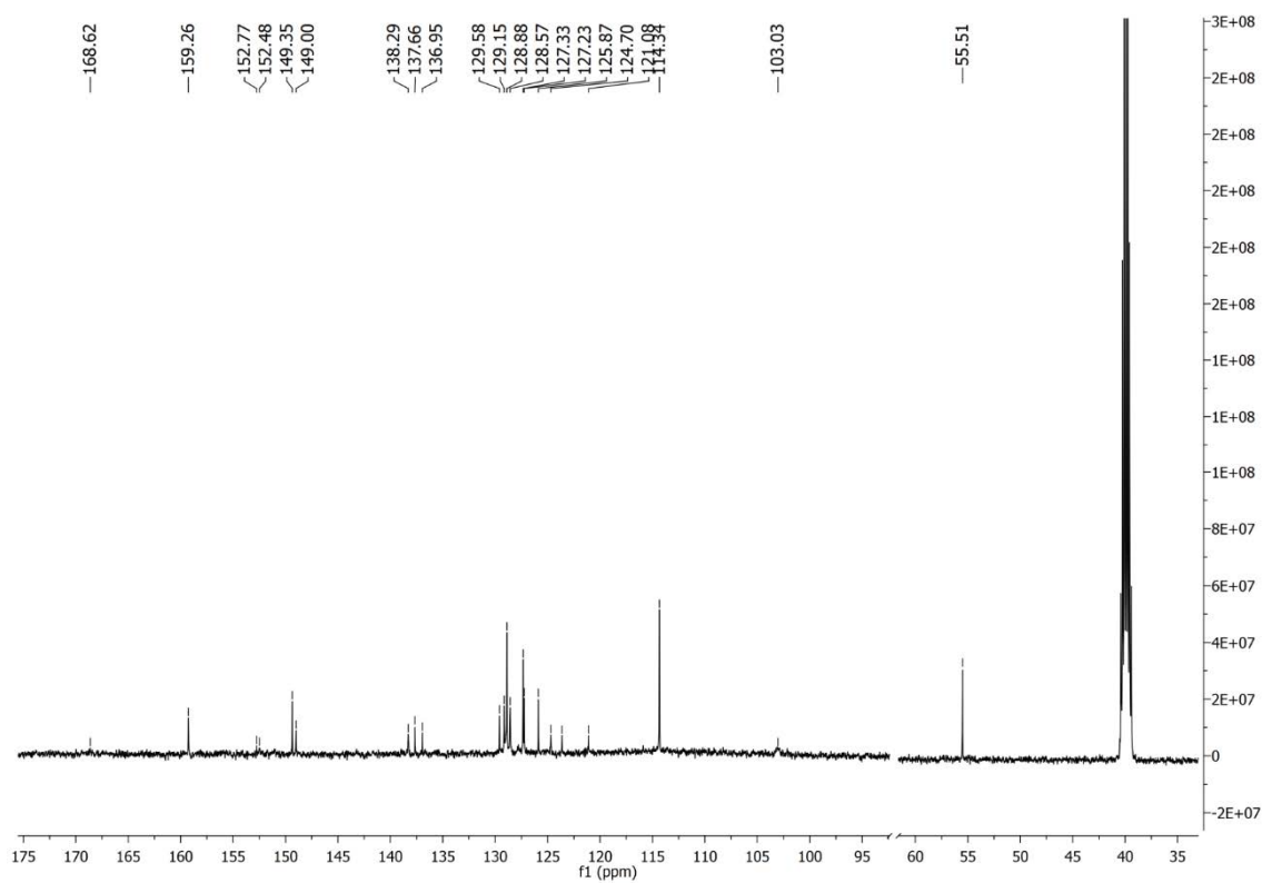
Slika P31. ^{13}\text{C} NMR spektar HLS 5 snimljen u \text{DMSO-}d_6 .
