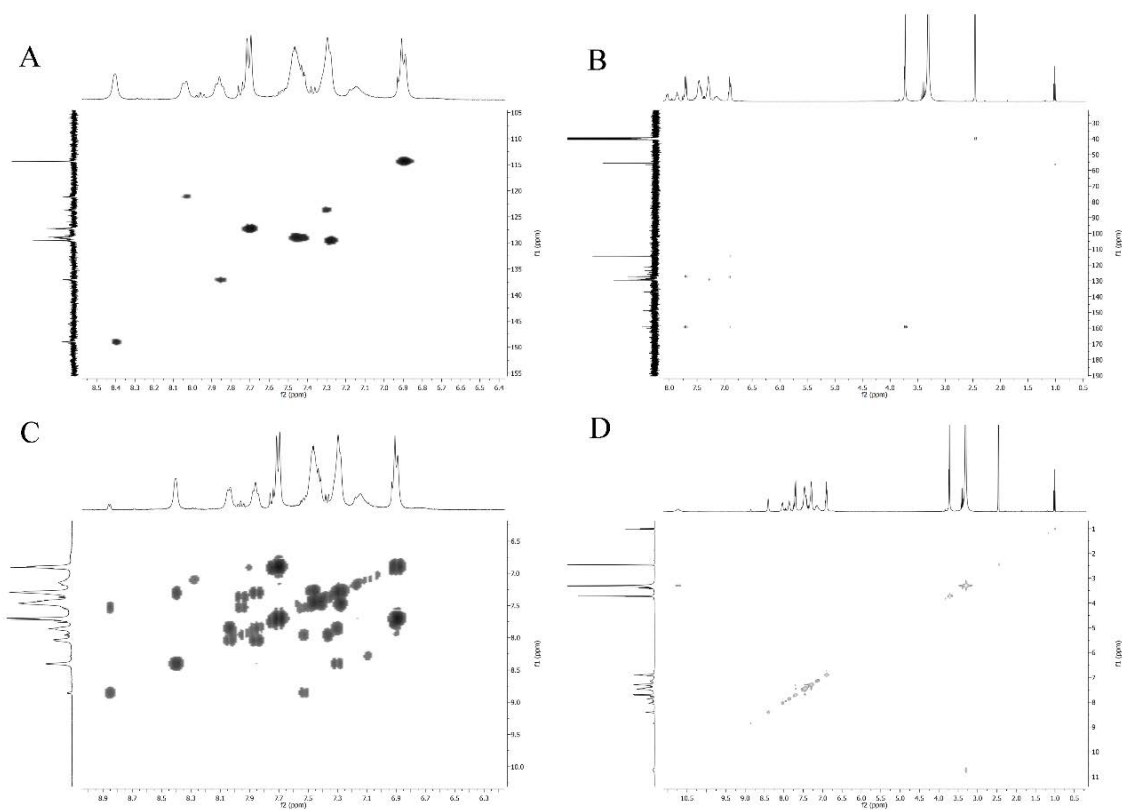
Slika P56. HSQC (A), HMBC (B), COSY (C) i NOESY (D) 2D NMR spektri kompleksa 4-S.
