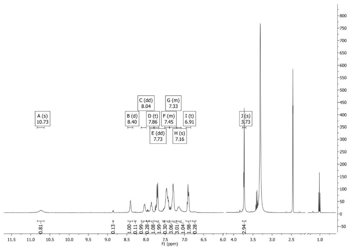
Slika P54. ^1\text{H} NMR spektar 4-S snimljen u \text{DMSO}-d_6 .
