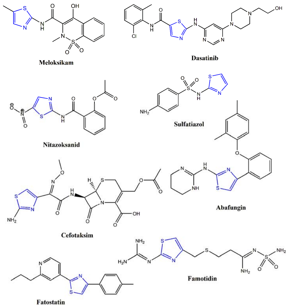
Slika 6. Strukturne formule biološki značajnih jedinjenja na bazi tiazola.
