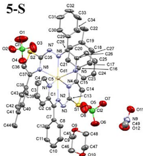
Slika 21. ORTEP prikazi molekulskih struktura kompleksa 3-S , 4-S i 5-S sa oznakama atoma. Termalni elipsoidi su prikazani sa 30 % verovatnoće. Zbog preglednosti u svim strukturama nisu prikazani atomi vodonika.
