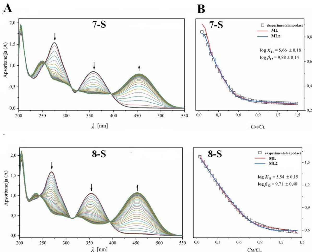
Slika 56. (A) UV-Vis spektri koji pokazuju spektralne promene tokom titracije \text{HLS}^2 ( C_L = 4,24 \cdot 10^{-5} \text{ M} , gore) i \text{HLS}^3 ( C_L = 3,39 \cdot 10^{-5} \text{ M} , dole) rastvorom \text{Cd}(\text{CH}_3\text{COO})_2 ( C_M = 4,50 \cdot 10^{-4} \text{ M} za \text{HLS}^2 ; C_M = 3,61 \cdot 10^{-4} \text{ M} za \text{HLS}^3 ) u metanolu. Podebljana crna linija označava početni spektar (ligand), dok podebljana zelena linija označava krajnji spektar. Strelice označavaju smer promene sa dodatkom \text{Cd}(\text{II}) jona. (B) Grafik zavisnosti promene apsorbancije ( \lambda = 365 \text{ nm} ) u odnosu na molarni odnos metal : ligand ( \text{HLS}^2 gore; \text{HLS}^3 dole).
