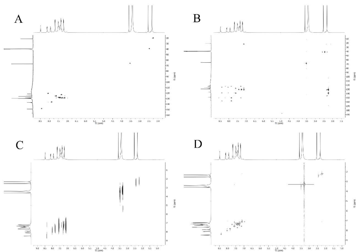
Slika P74. HSQC (A), HMBC (B), COSY (C) i NOESY (D) 2D NMR spektri kompleksa 5-Se .
