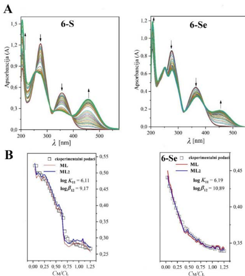
Slika 55. (A) UV-Vis spektri koji pokazuju spektralne promene tokom titracije \text{HLS}^2 ( C_L = 3,22 \cdot 10^{-5} M, levo) i \text{HLSe}^2 ( C_L = 1,00 \cdot 10^{-5} M, desno) rastvorom \text{Cd}(\text{NO}_3)_2 ( C_M = 2,78 \cdot 10^{-4} M za \text{HLS}^2 ; C_M = 8,63 \cdot 10^{-5} M za \text{HLSe}^2 ) u metanolu. Podebljana crna linija označava početni spektar (ligand), dok podebljana zelena linija označava krajnji spektar. Strelice označavaju smer promene tokom dodavanja \text{Cd}(\text{II}) jona. (B) Grafici zavisnosti promene apsorbancije ( \lambda = 365 nm) u odnosu na molarni odnos metal : ligand ( \text{HLS}^2 levo; \text{HLSe}^2 desno).
