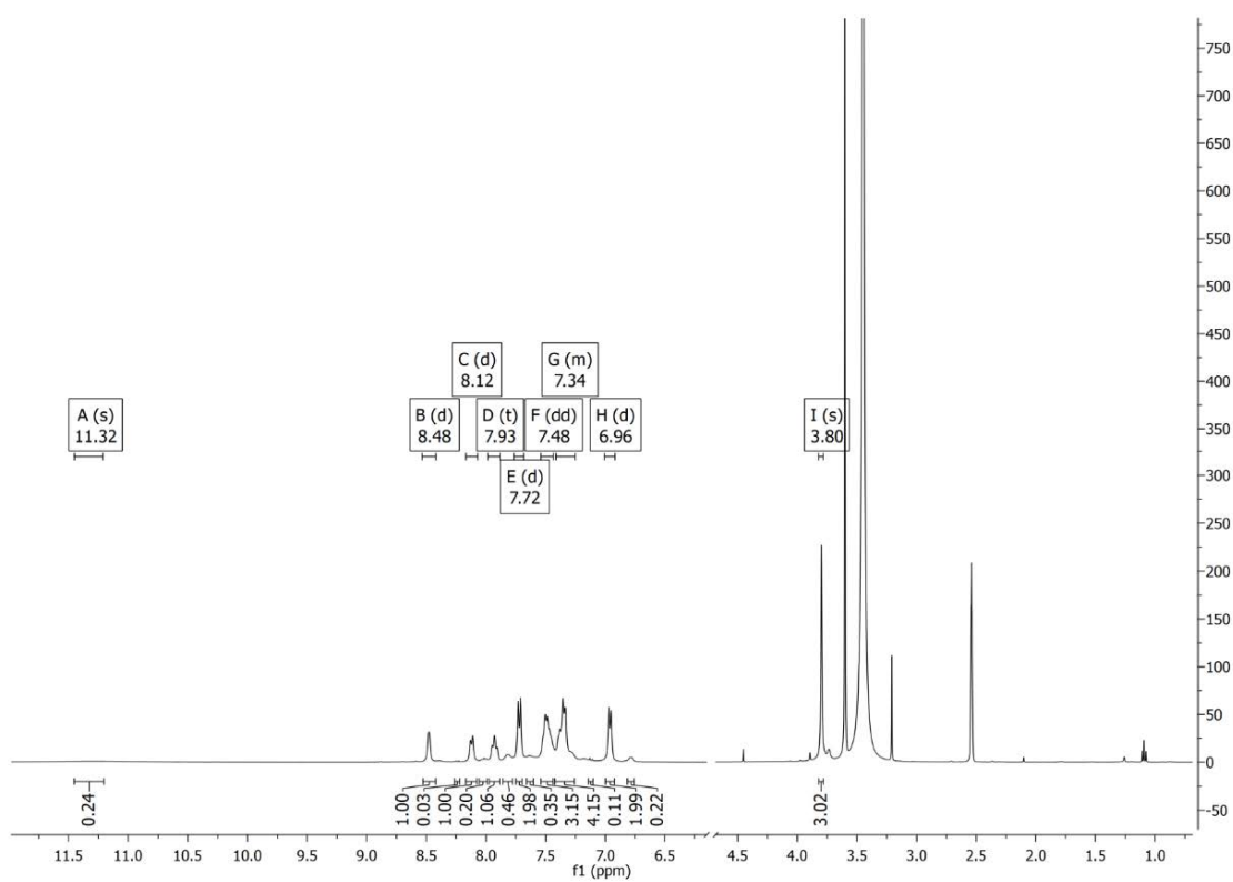
Slika P69. ^1\text{H} NMR spektar 4-Se snimljen u \text{DMSO-}d_6 .
