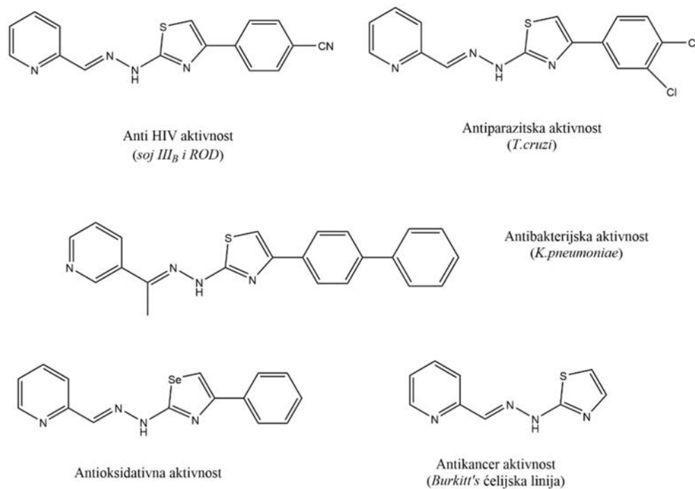
Slika 12. Strukturne formule aktivnih piridinskih hidrazonil-halkogenazola.
