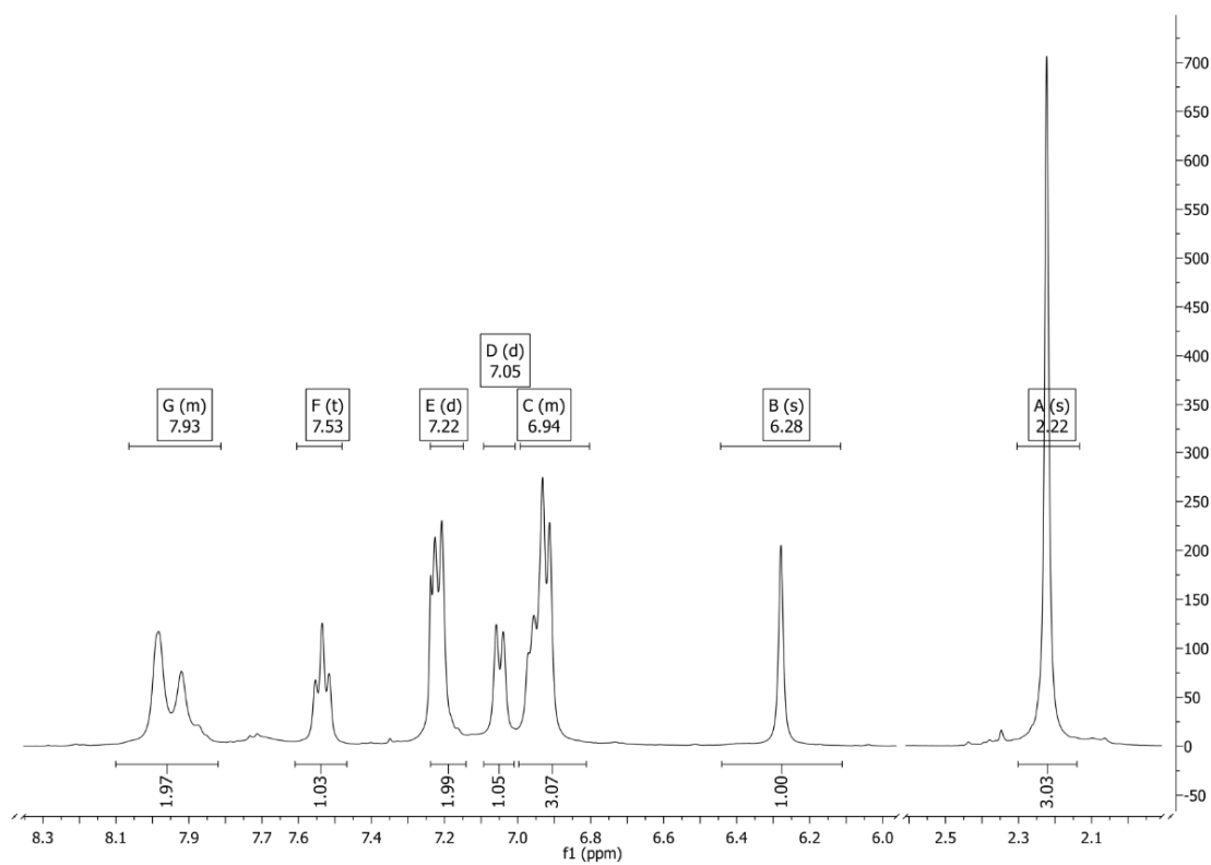
Slika P84. ^1\text{H} NMR spektar 8-S snimljen u \text{CDCl}_3 .
