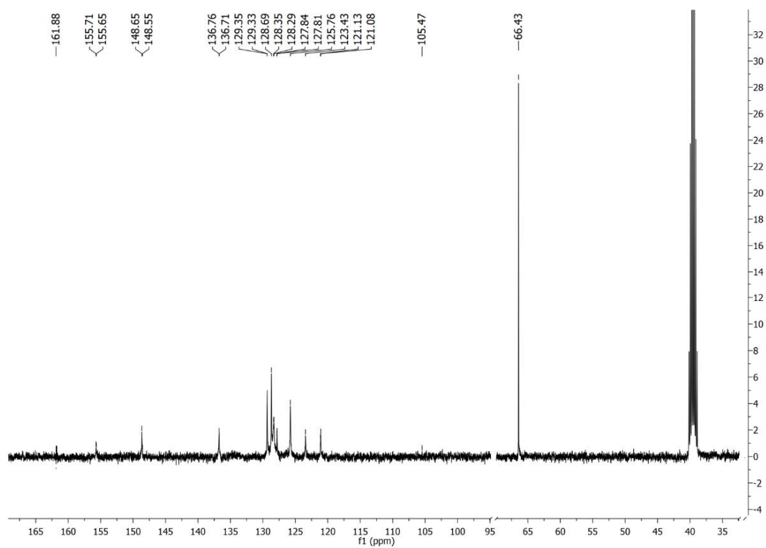
Slika P67. ^{13}\text{C} NMR spektar 3-Se snimljen u \text{DMSO-}d_6 .
