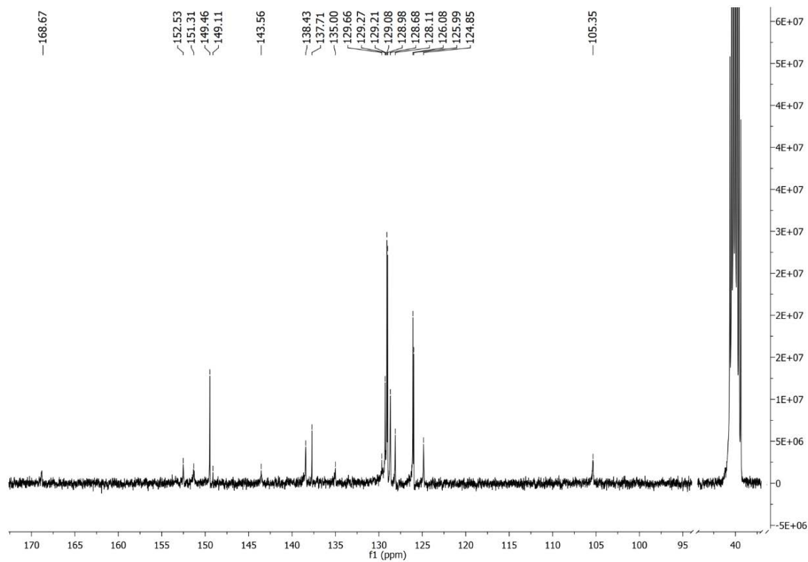
Slika P28. ^{13}\text{C} NMR spektar HLS 4 snimljen u \text{DMSO-}d_6 .
