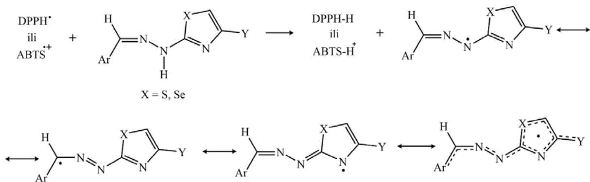
Shema 1. Mehanizam uklanjanja DPPH radikala i ABTS katjon radikala od strane halkogen-azola.
