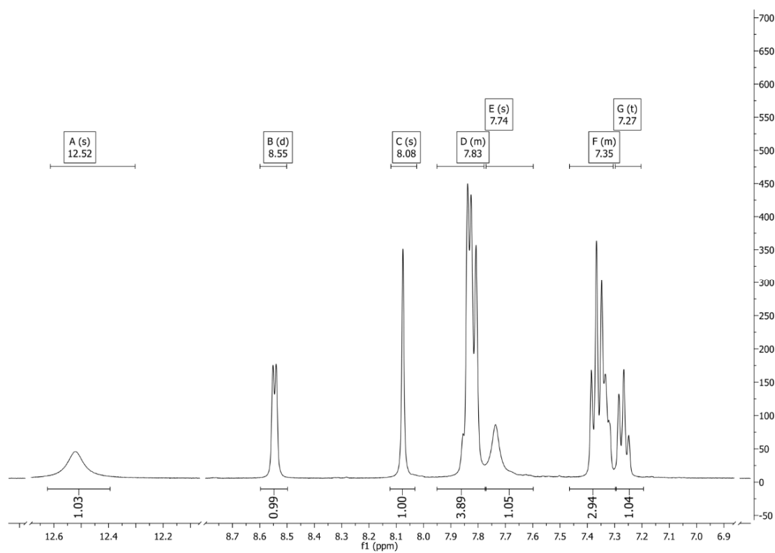
Slika P60. ^1\text{H} NMR spektar 1-Se snimljen u \text{DMSO}-d_6 .
