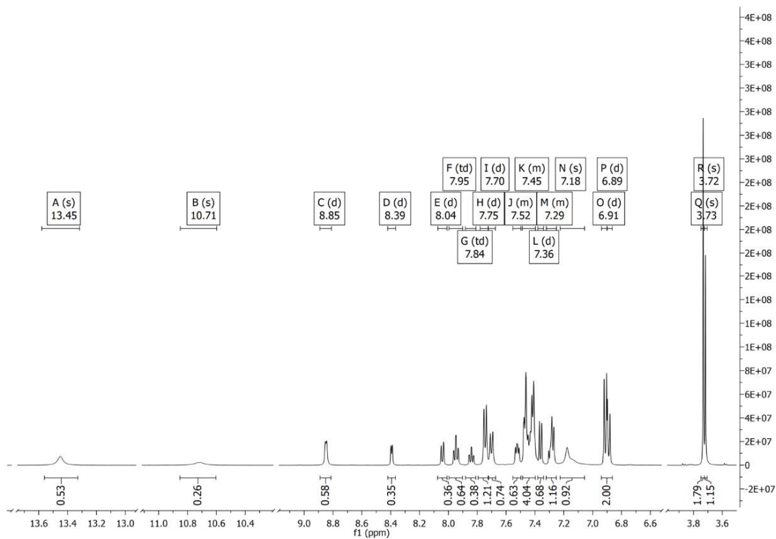
Slika P30. 1 H NMR spektar HLS 5 snimljen u DMSO- d 6 .
