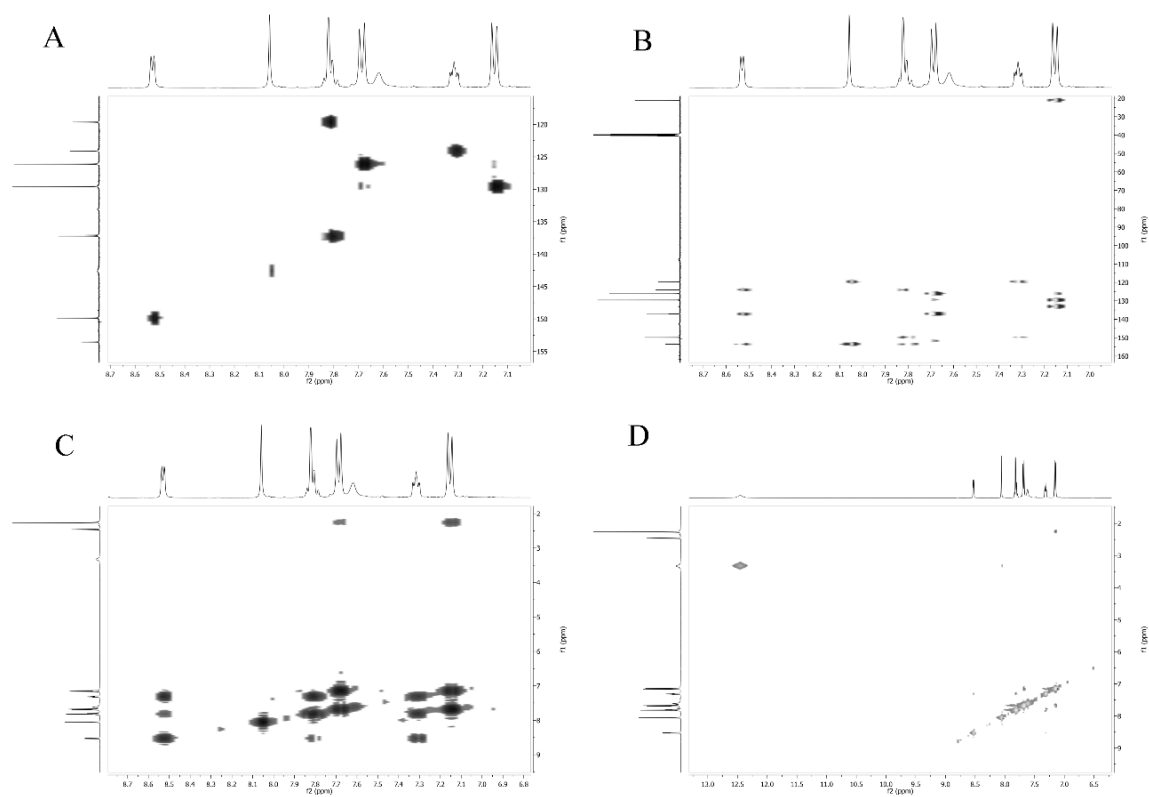
Slika P65. HSQC (A), HMBC (B), COSY (C) i NOESY (D) 2D NMR spektri kompleksa 2-Se .
