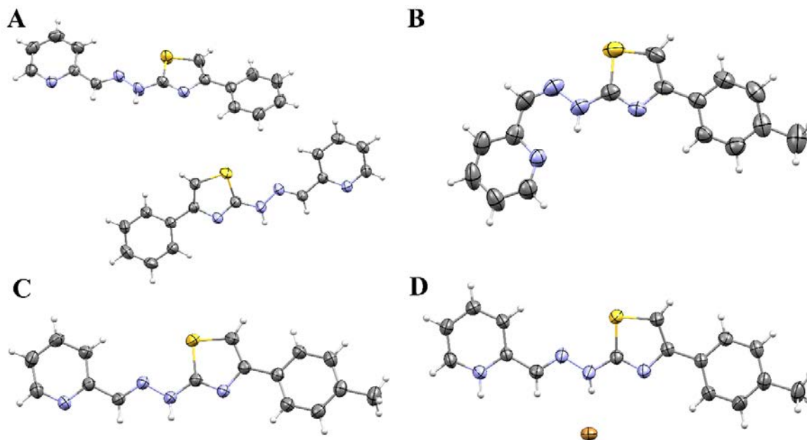
Slika 10. ORTEP prikazi molekulskih struktura 9f (A), 4 (B), HL (C) i HLS 3 ·HBr (D). Termalni elipsoidi su prikazani sa 50 % verovatnoće. Sivom bojom predstavljeni su atomi ugljenika, belom bojom atomi vodonika, ljubičastom bojom atomi azota, žutom bojom atomi sumpora i braon bojom atom broma.
