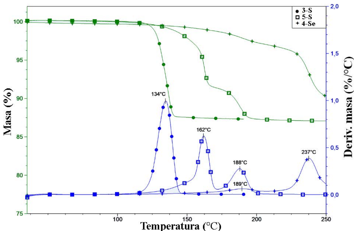
Slika 49. TG i DTG krive za komplekse 3-S , 5-S i 4-Se snimljene u struji argona. Zelenom bojom označene su TG krive, a plavom bojom DTG krive.
