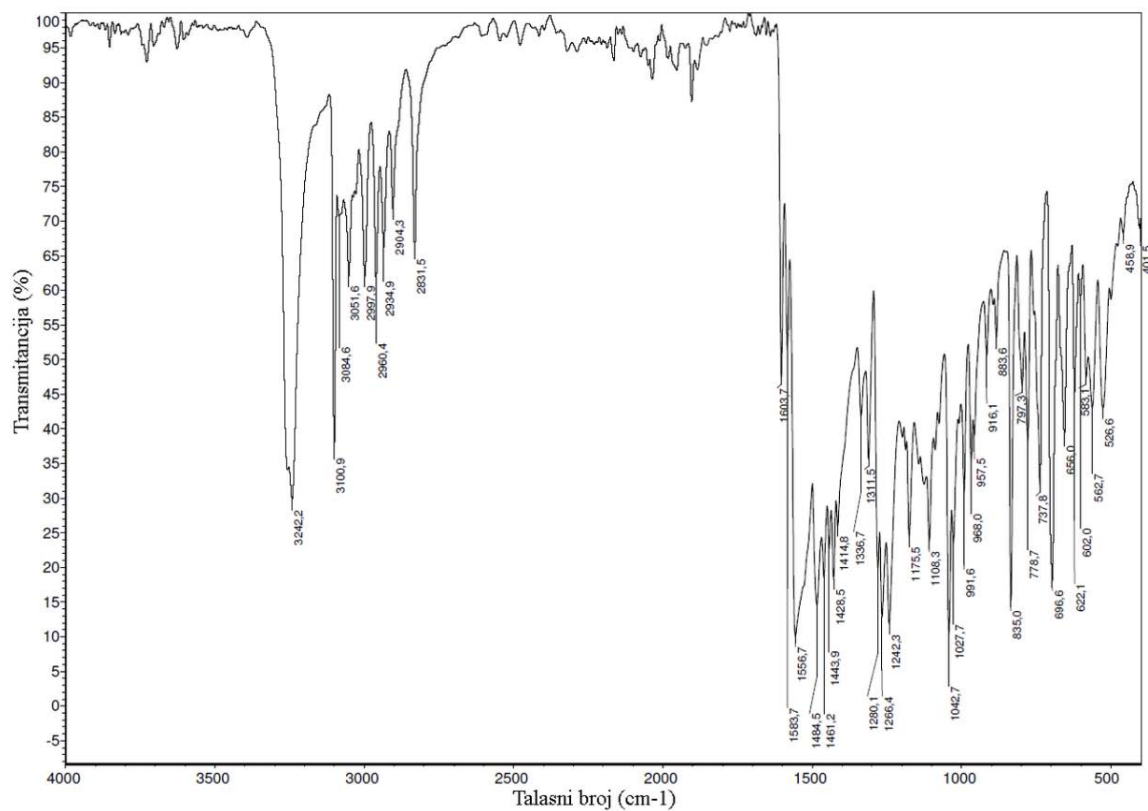
Slika P11. IC spektar liganda HLSe 5 .
