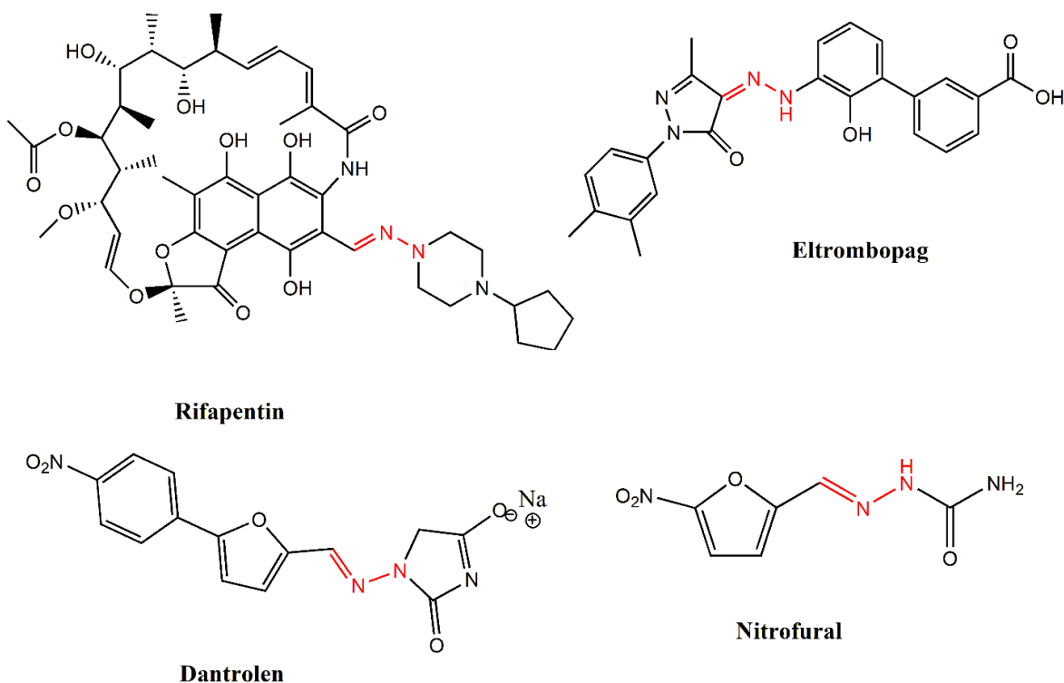
Slika 8. Strukturne formule biološki značajnih jedinjenja na bazi hidrazona.
