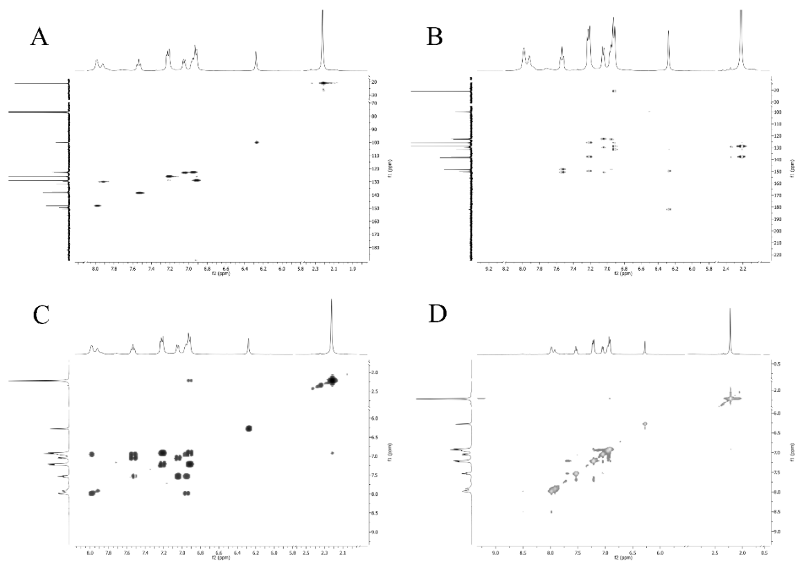
Slika P86. HSQC (A), HMBC (B), COSY (C) i NOESY (D) 2D NMR spektri kompleksa 8-S .
