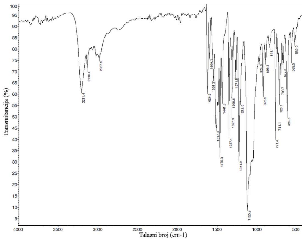
Slika P13. IC spektar kompleksa 1-S.
