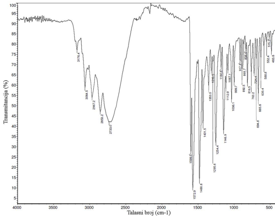
Slika P9. IC spektar liganda HLSe 3 .
