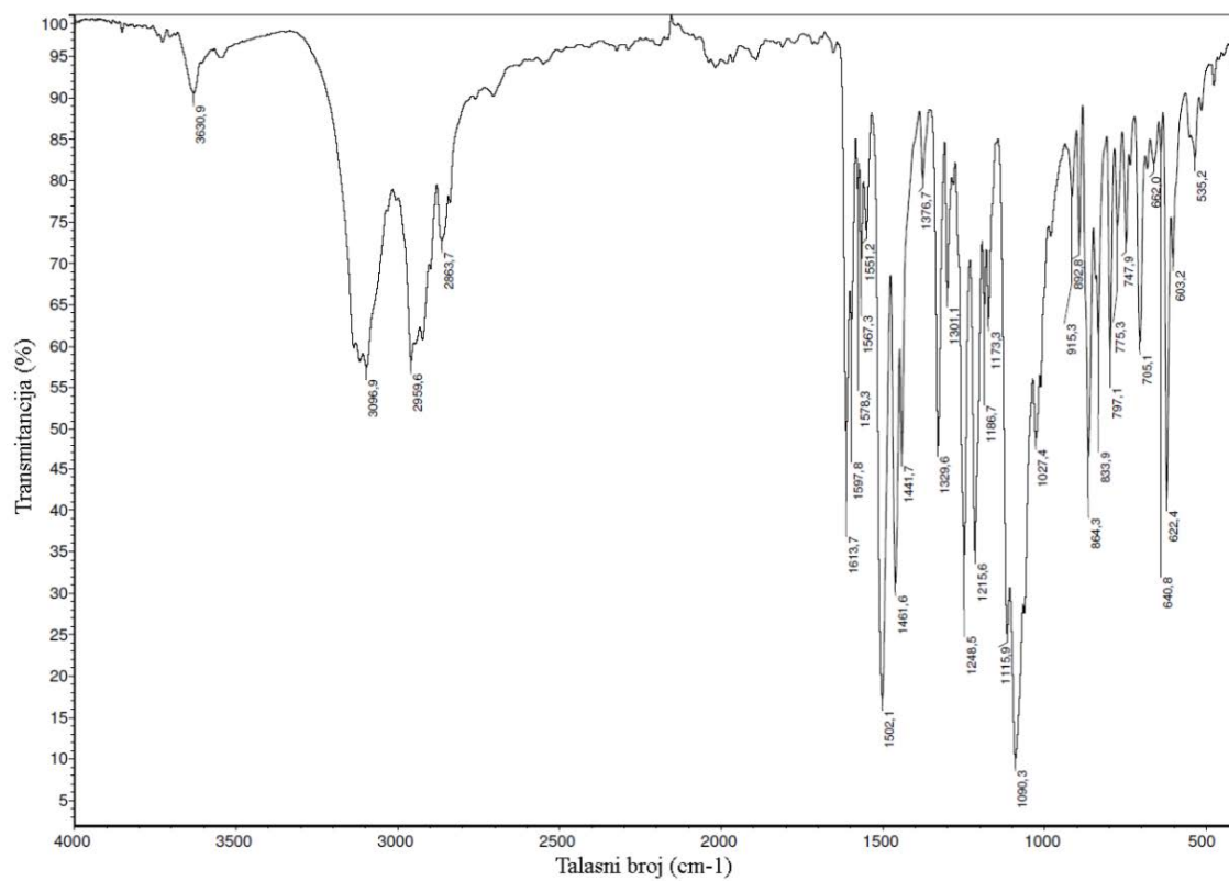
Slika P21. IC spektar kompleksa 4-Se.
