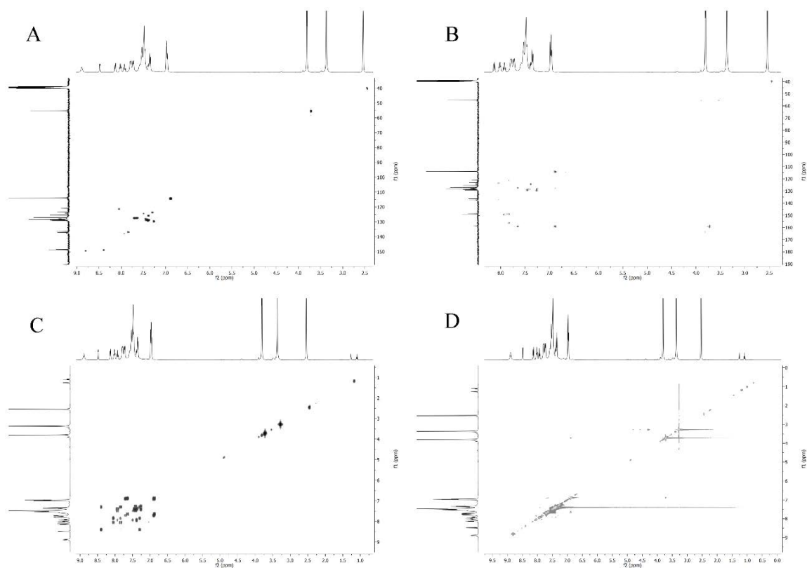
Slika P41. HSQC (A), HMBC (B), COSY (C) i NOESY (D) 2D NMR spektri liganda HLSe 5 .
