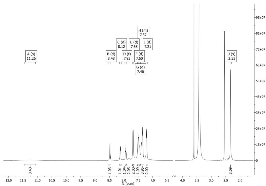
Slika P72. ^1\text{H} NMR spektar 5-Se snimljen u \text{DMSO-}d_6 .
