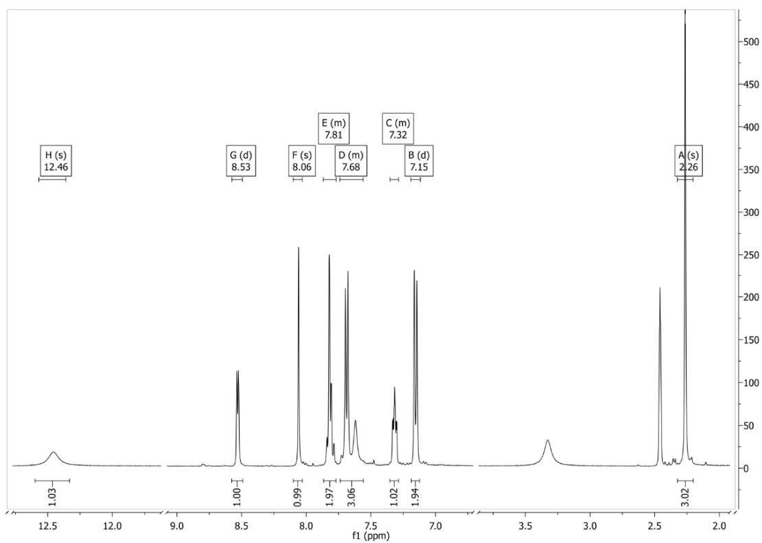
Slika P63. 1 H NMR spektar 2-Se snimljen u DMSO- d 6 .
