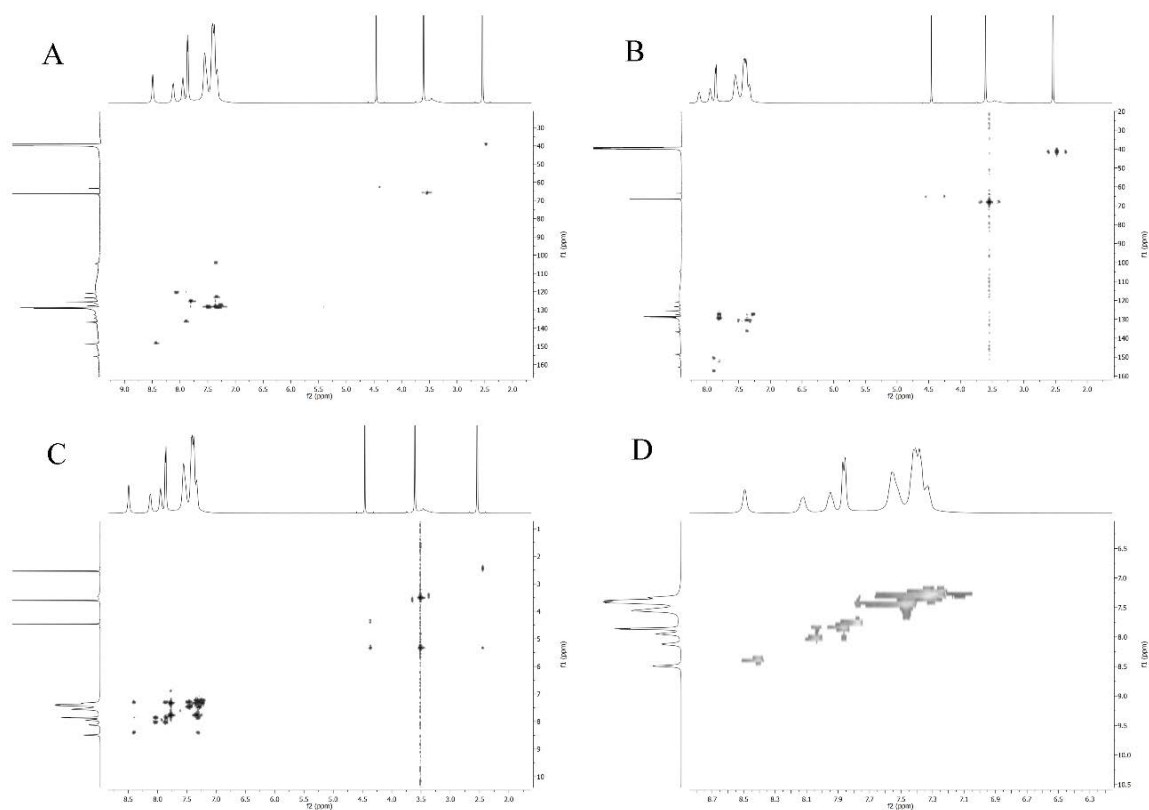
Slika P53. HSQC (A), HMBC (B), COSY (C) i NOESY (D) 2D NMR spektri kompleksa 3-S .
