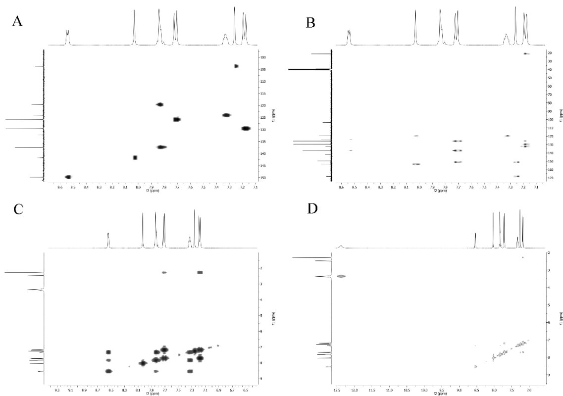
Slika P50. HSQC (A), HMQC (B), COSY (C) i NOESY (D) 2D NMR spektri kompleksa 2-S .
