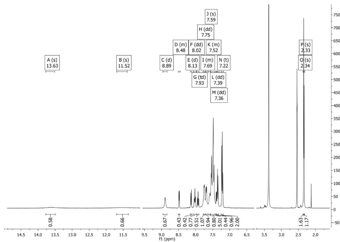
Slika P42. 1 H NMR spektar HLSe 6 snimljen u DMSO- d 6 .
