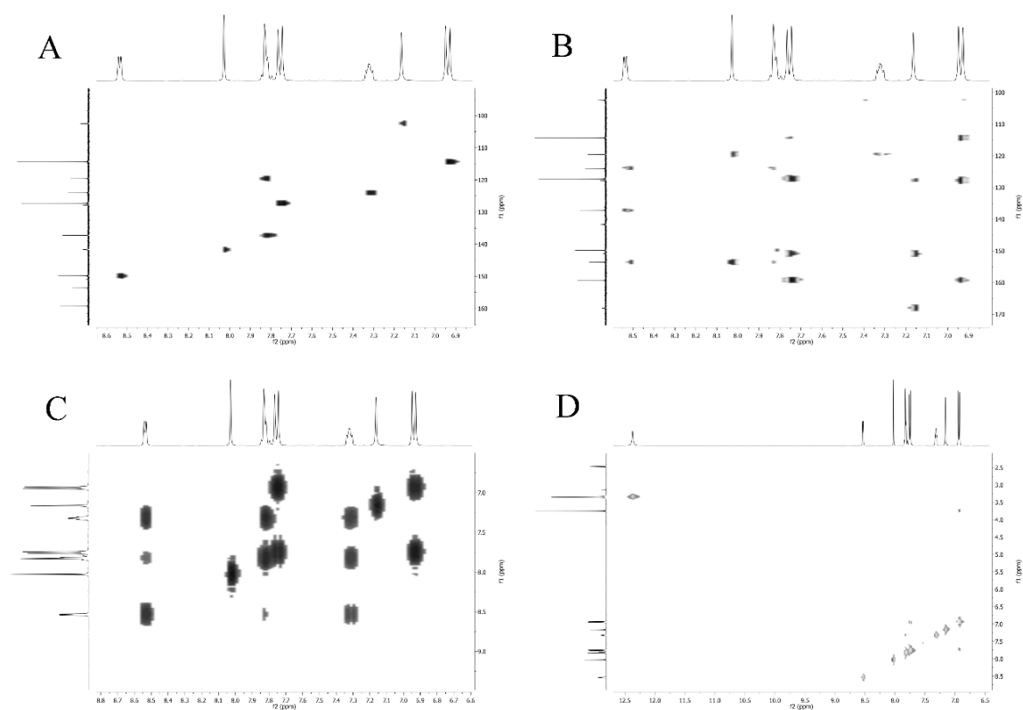
Slika P77. HSQC (A), HMBC (B), COSY (C) i NOESY (D) 2D NMR spektri kompleksa 6-S .
