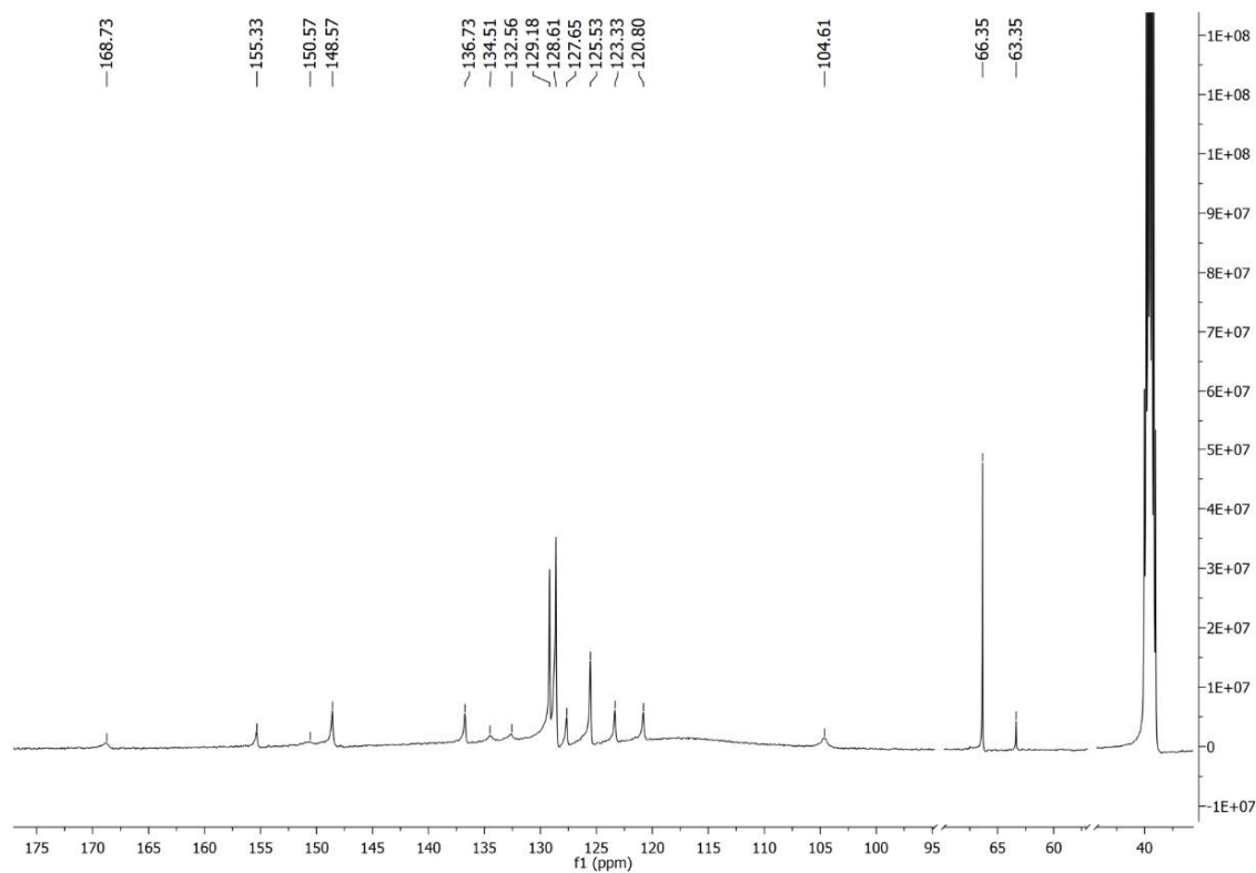
Slika P52. ^{13}\text{C} NMR spektar 3-S snimljen u \text{DMSO-}d_6 .
