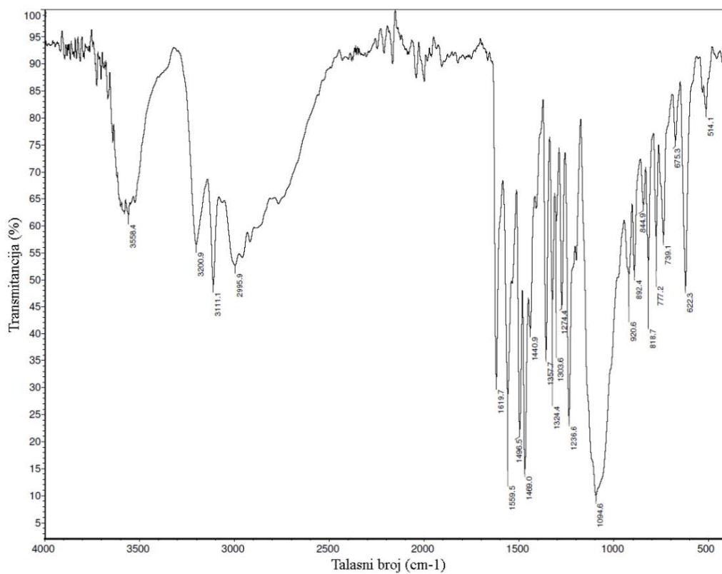
Slika P14. IC spektar kompleksa 2-S.
