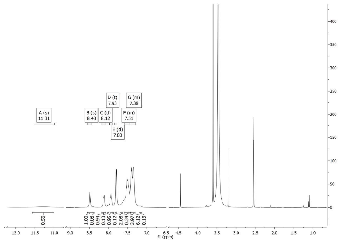
Slika P66. ^1\text{H} NMR spektar 3-Se snimljen u \text{DMSO}-d_6 .
