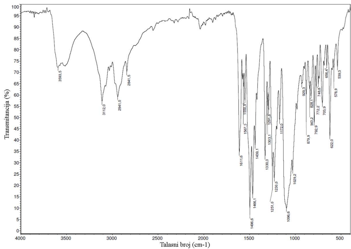
Slika P16. IC spektar kompleksa 4-S.
