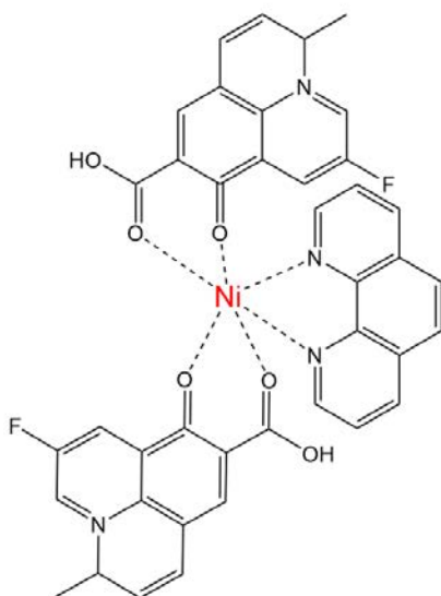
Kompleks Ni(II) sa flumekinom
