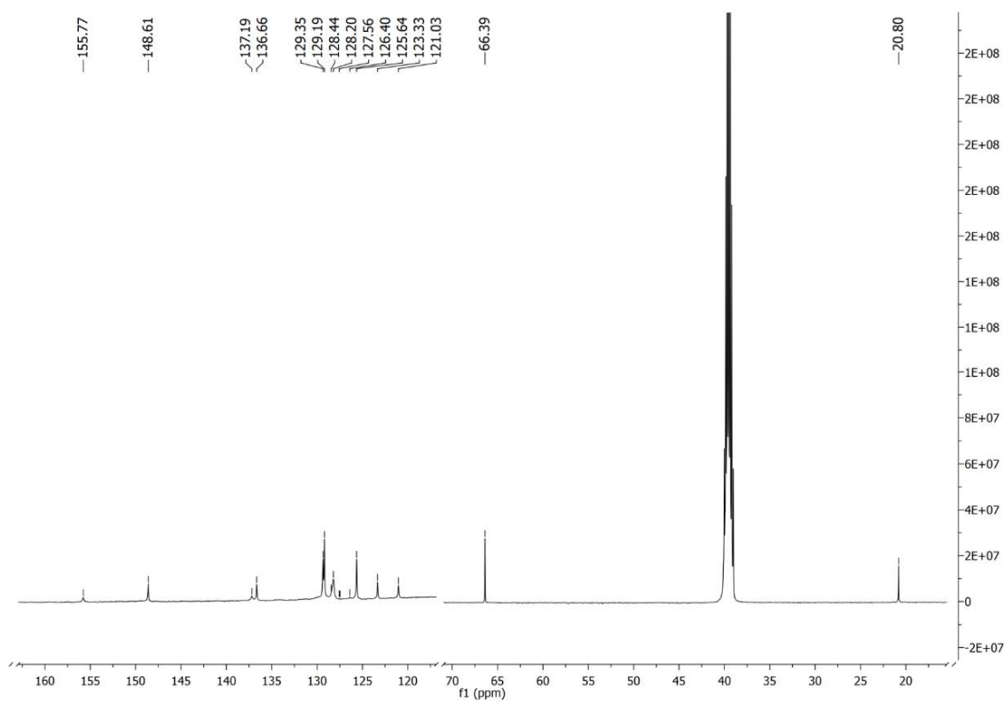
Slika P73. ^{13}\text{C} NMR spektar 5-Se snimljen u \text{DMSO-}d_6 .
