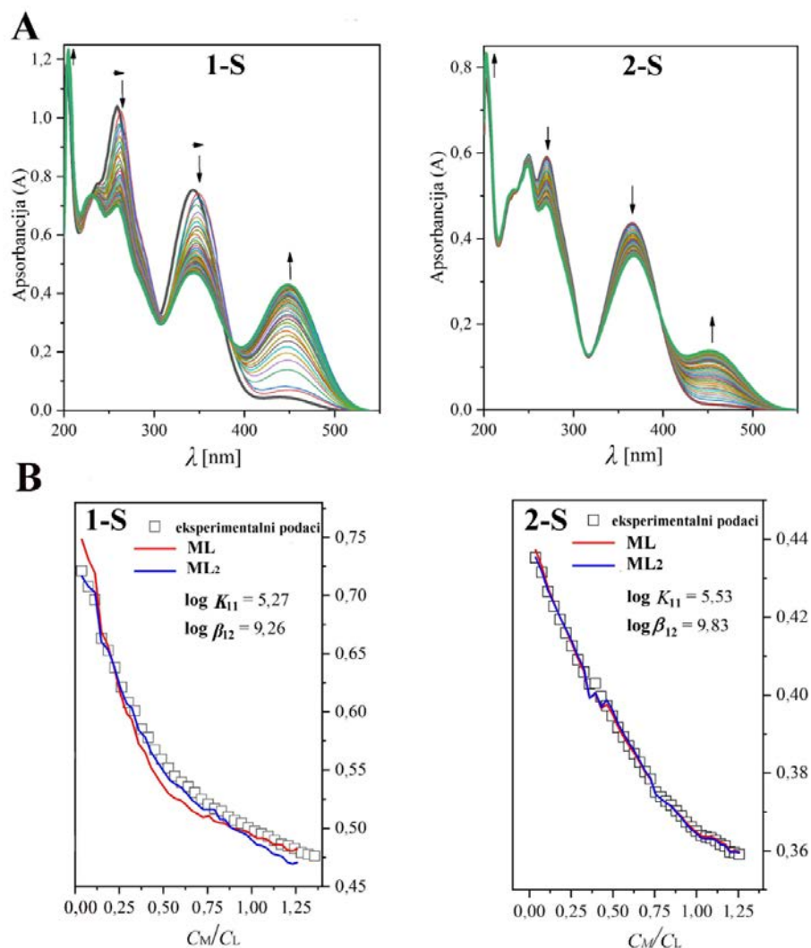
Slika 53. (A) UV-Vis spektri koji pokazuju spektralne promene tokom titracije liganada HLS 1 ( C_L = 4,17 \cdot 10^{-5} M, levo) i HLS 3 ( C_L = 1,58 \cdot 10^{-5} M, desno) rastvorom Cd(ClO 4 ) 2 ( C_M = 3,6 \cdot 10^{-4} M za titraciju HLS 1 ; C_M = 1,36 \cdot 10^{-4} M za titraciju HLS 3 ) u metanolu. Crna linija označava početni spektar (ligand), dok podebljana zelena linija označava krajnji spektar. Strelice označavaju smer promena uočenih pri dodatku Cd(II) jona. (B) Grafici zavisnosti promene apsorpcije ( \lambda = 365 nm) u odnosu na molarni odnos metal : ligand (HLS 1 levo; HLS 3 desno).
