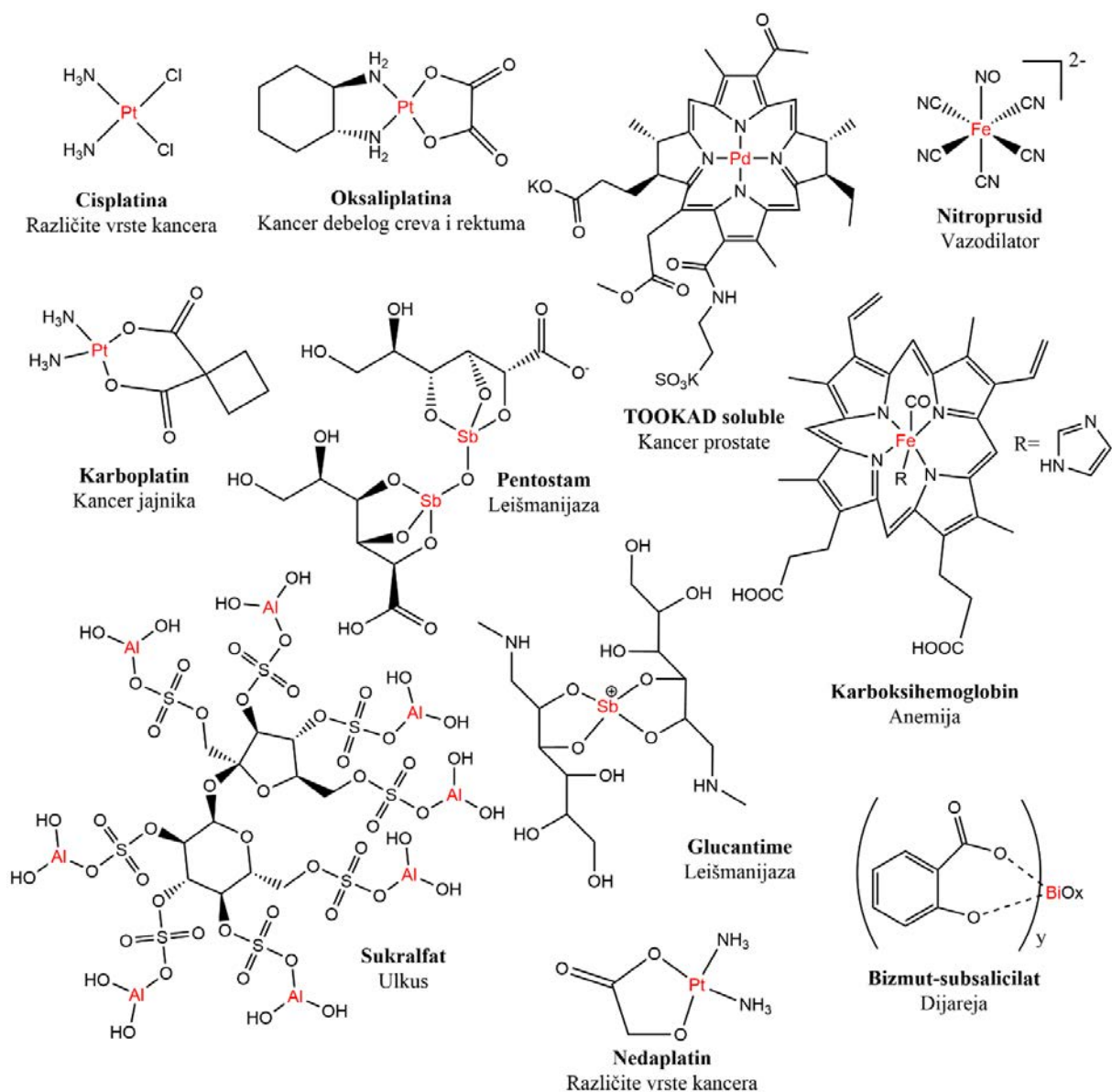
Slika 3. Strukturne formule klinički odobrenih lekova na bazi kompleksnih jedinjenja.
