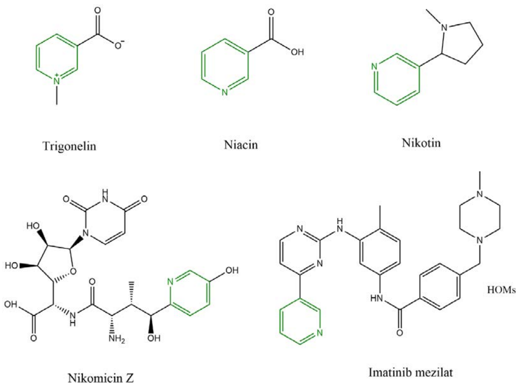
Slika 5. Strukturne formule biološki značajnih jedinjenja na bazi piridina.
