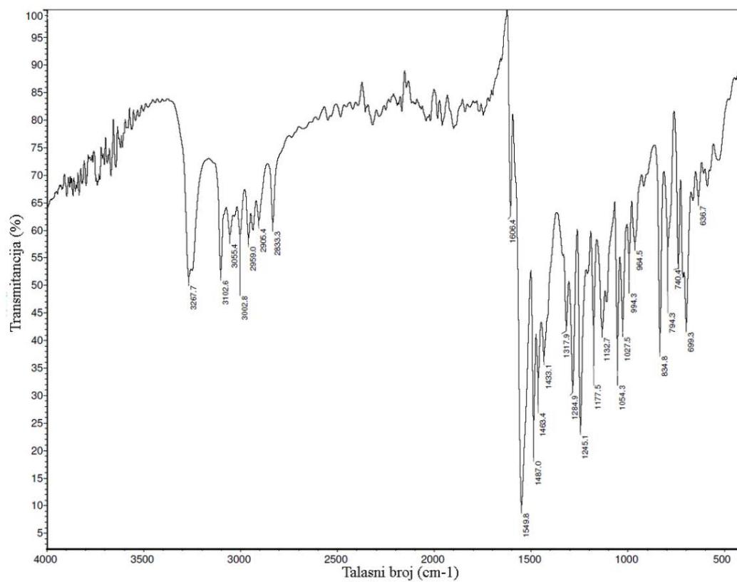
Slika P5. IC spektar liganda HLS 5 .
