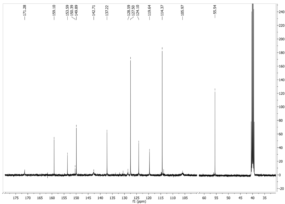
Slika P79. ^{13}\text{C} NMR spektar 6-Se snimljen u \text{DMSO-}d_6 .
