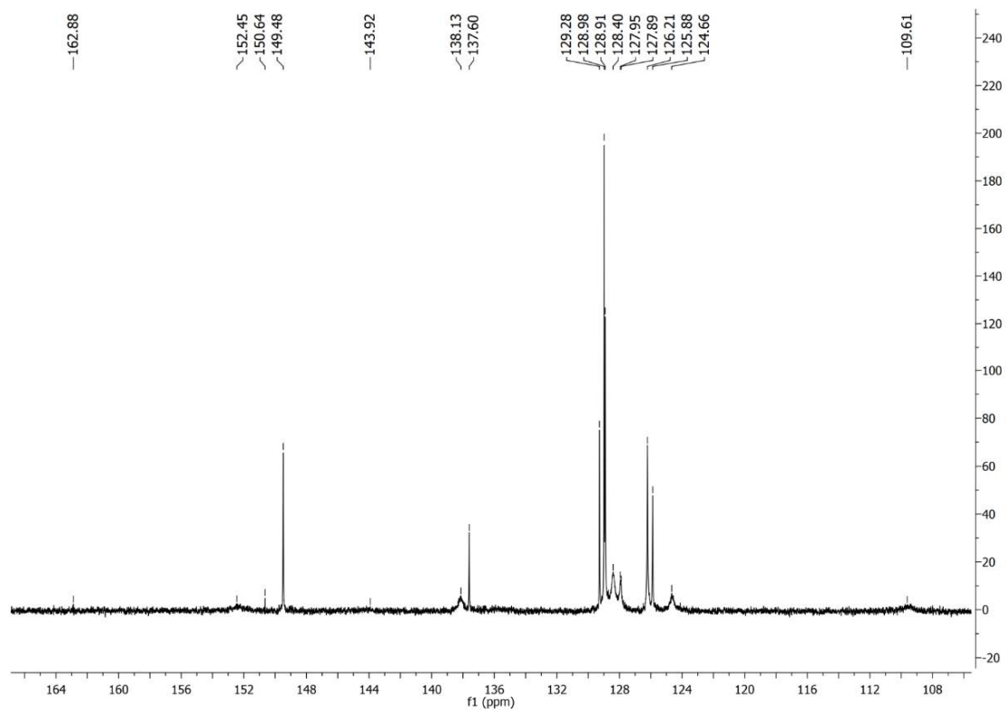
Slika P37. ^{13}\text{C} NMR spektar HLSe 4 snimljen u \text{DMSO-}d_6 .
