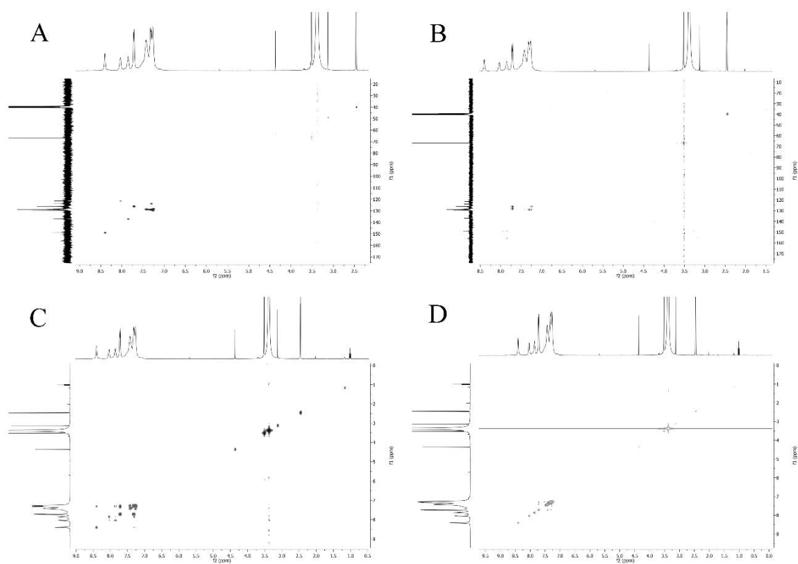
Slika P68. HSQC (A), HMBC (B), COSY (C) i NOESY (D) 2D NMR spektri kompleksa 3-Se .
