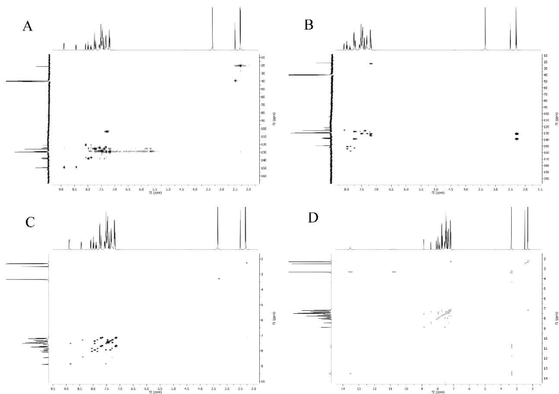
Slika P35. HSQC (A), HMBC (B), COSY (C) i NOESY (D) 2D NMR spektri liganda HLS 6 .
