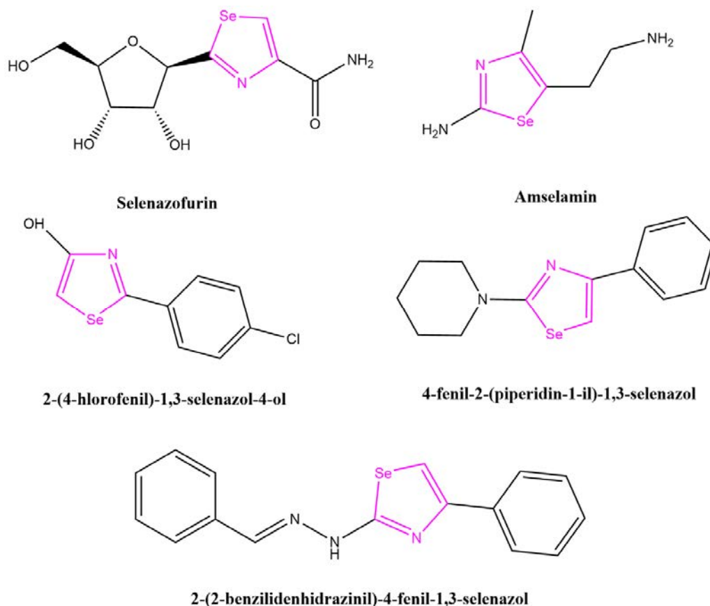
Slika 7. Strukturne formule biološki značajnih jedinjenja na bazi 1,3-selenazola.
