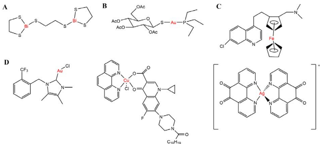
Slika 1. Strukturne formule aktivnih supstanci na bazi kompleksa metala koji su odobreni od strane FDA (A i B), organometalnog jedinjenja na bazi gvožđa koji je ušao u II fazu kliničkih ispitivanja (C) i kompleksnih jedinjenja koja imaju potencijal za dalja ispitivanja (D).
