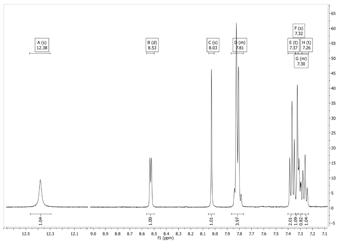
Slika P45. 1 H NMR spektar 1-S snimljen u DMSO- d 6 .
