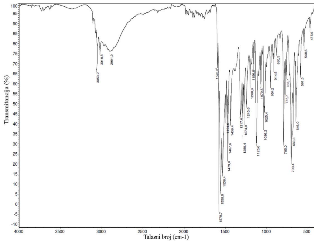
Slika P10. IC spektar liganda HLSe 4 .
