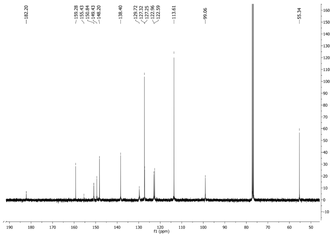
Slika P82. 13 C NMR spektar 7-S snimljen u CDCl 3 .
