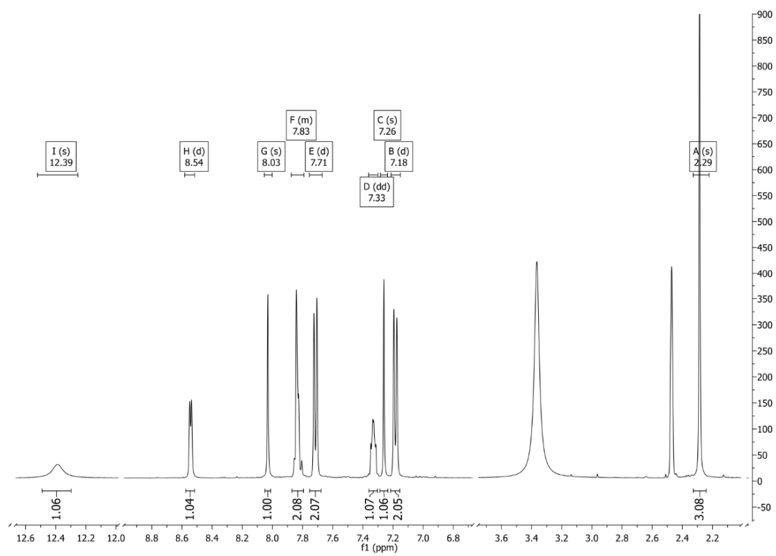
Slika P48. ^1\text{H} NMR spektar 2-S snimljen u \text{DMSO}-d_6 .
