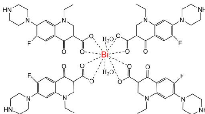
Kompleks Bi(III) sa norfloksacinom
