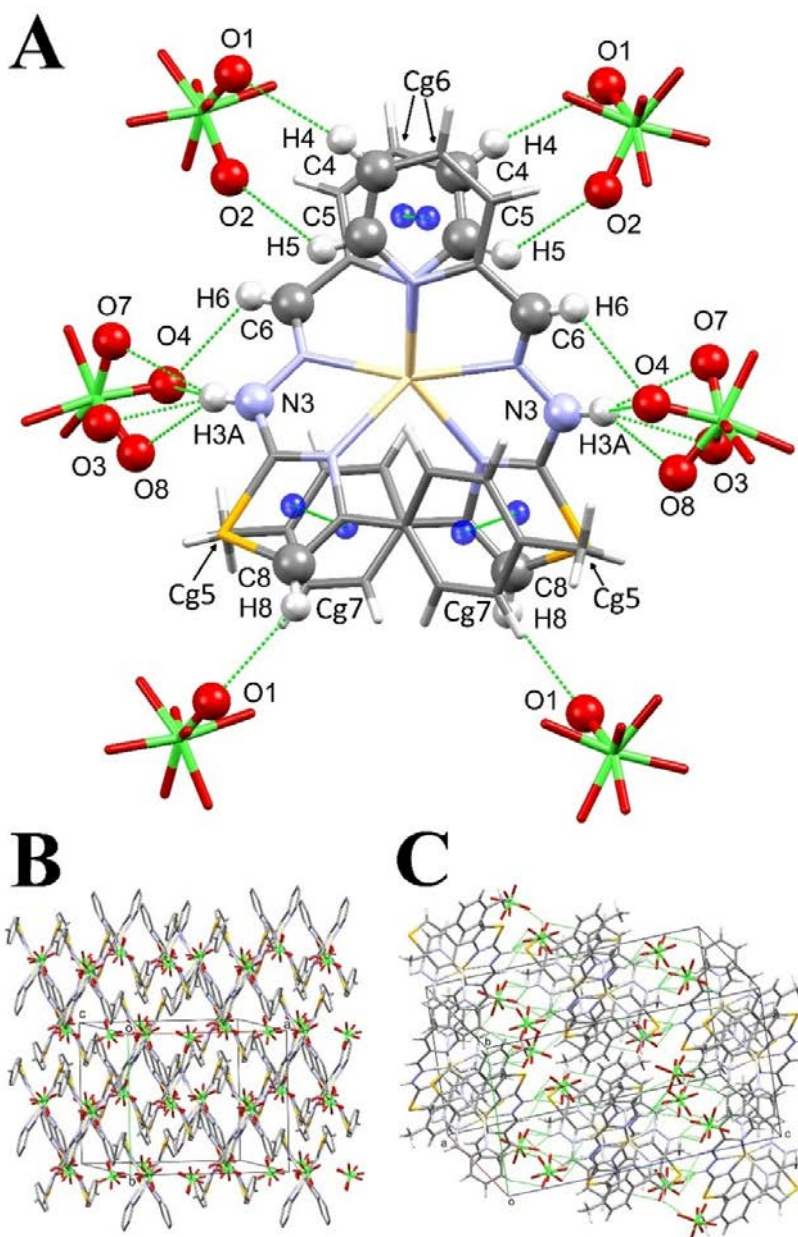
Slika 32. (A) Interakcije odgovorne za formiranje kristalnog pakovanja kompleksa 2–Se . (B) 2D sloj koji je paralelan ab ravni. (C) Međusobno paralelni 2D slojevi koji formiraju 3D kristalno pakovanje.
