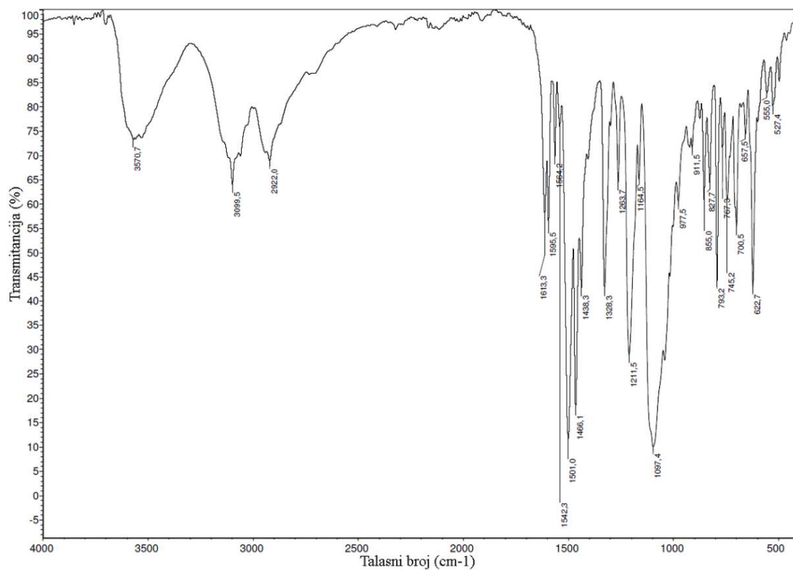
Slika P22. IC spektar kompleksa 5-Se.
