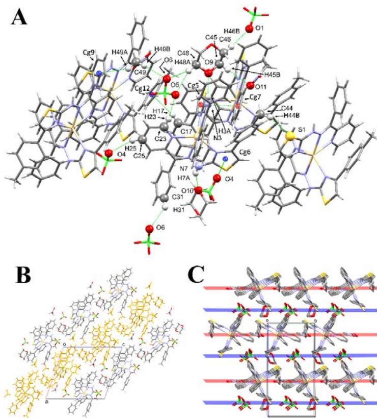
Slika 30. (A) Interakcije odgovorne za formiranje kristalnog pakovanja kompleksa 5–S . (B) 2D sloj koji je paralelan ac ravni. (C) Međusobno paralelni 2D slojevi koji formiraju 3D kristalno pakovanje. Zbog preglednosti atomi vodonika su uklonjeni iz prikaza.
