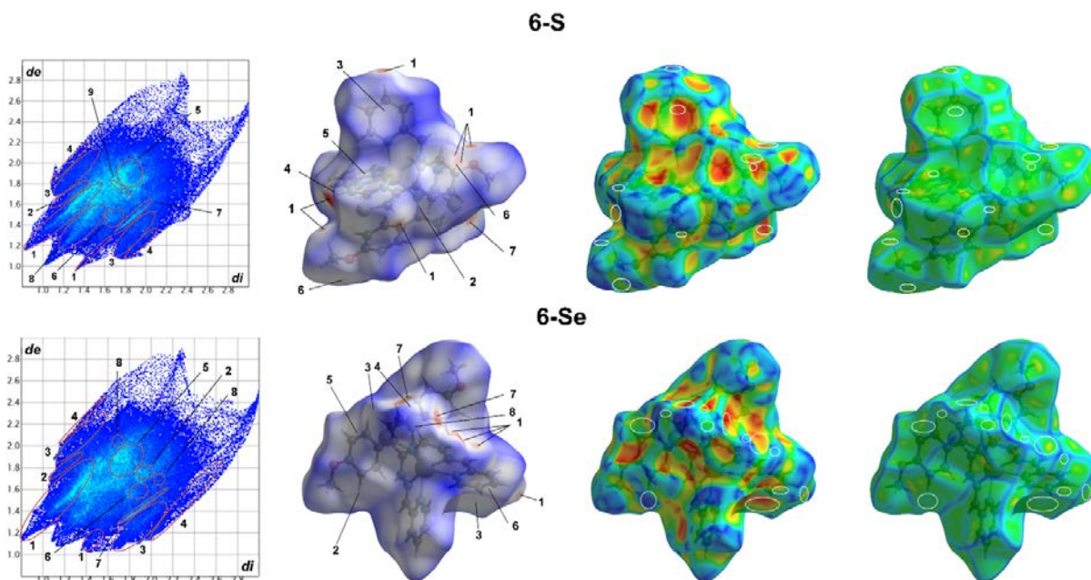
Slika 42. 2D grafikoni otisaka prsta međumolekulskih kontakata i Hiršfeldove površine mapirane sa d_{\text{norm}} , indeksom oblika i zakrivljenosti za komplekse 6–S i 6–Se.
