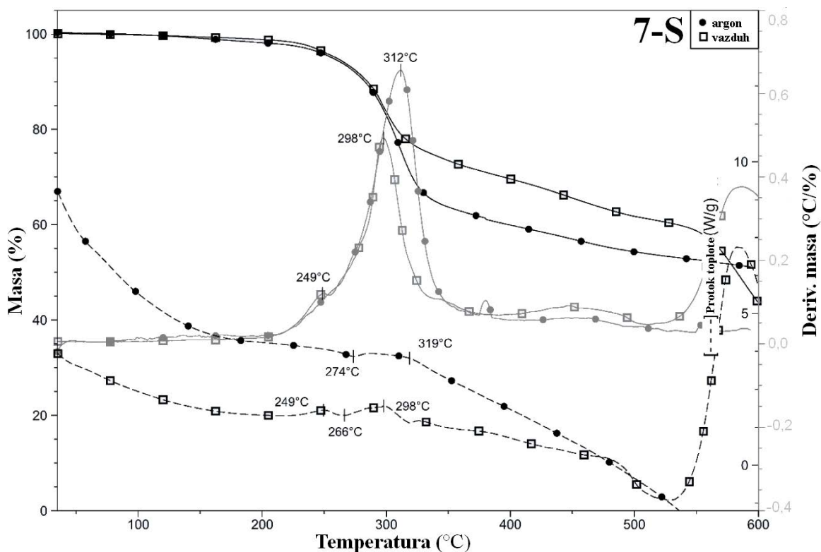
Slika 51. TG, DTG i DSC krive za kompleks 7-S snimljene u struji argona i vazduha. Pune linije crne boje predstavljaju TG krive, pune linije sive boje predstavljaju DTG krive, a ispekidane crne linije predstavljaju DSC krive.
