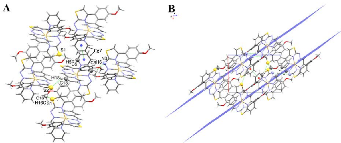
Slika 38. (A) Interakcije odgovorne za formiranje kristalnog pakovanja kompleksa 7-S . (B) 2D sloj koji je paralelan ac ravni.
