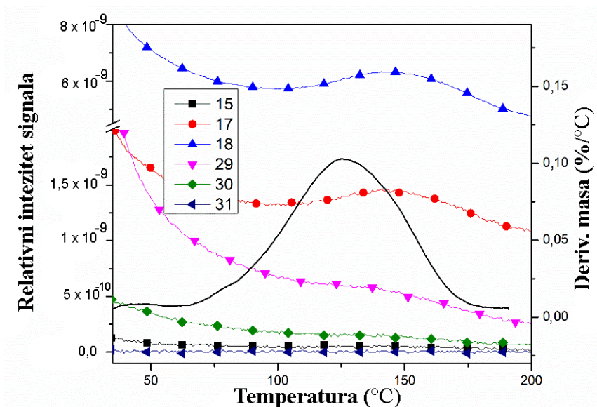
Slika 46. Pikovi koji potiču od vode i 1,4-dioksana ( m/z vrednosti su date na grafiku) nastalih dekompozicijom 3–Se (crna boja).
