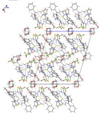
Slika 34. (A) Interakcije odgovorne za formiranje kristalnog pakovanja kompleksa 4- Se . (B) 2D sloj koji je paralelan (20–1) ravni. (C) Međusobno paralelni 2D slojevi koji formiraju 3D kristalno pakovanje.
