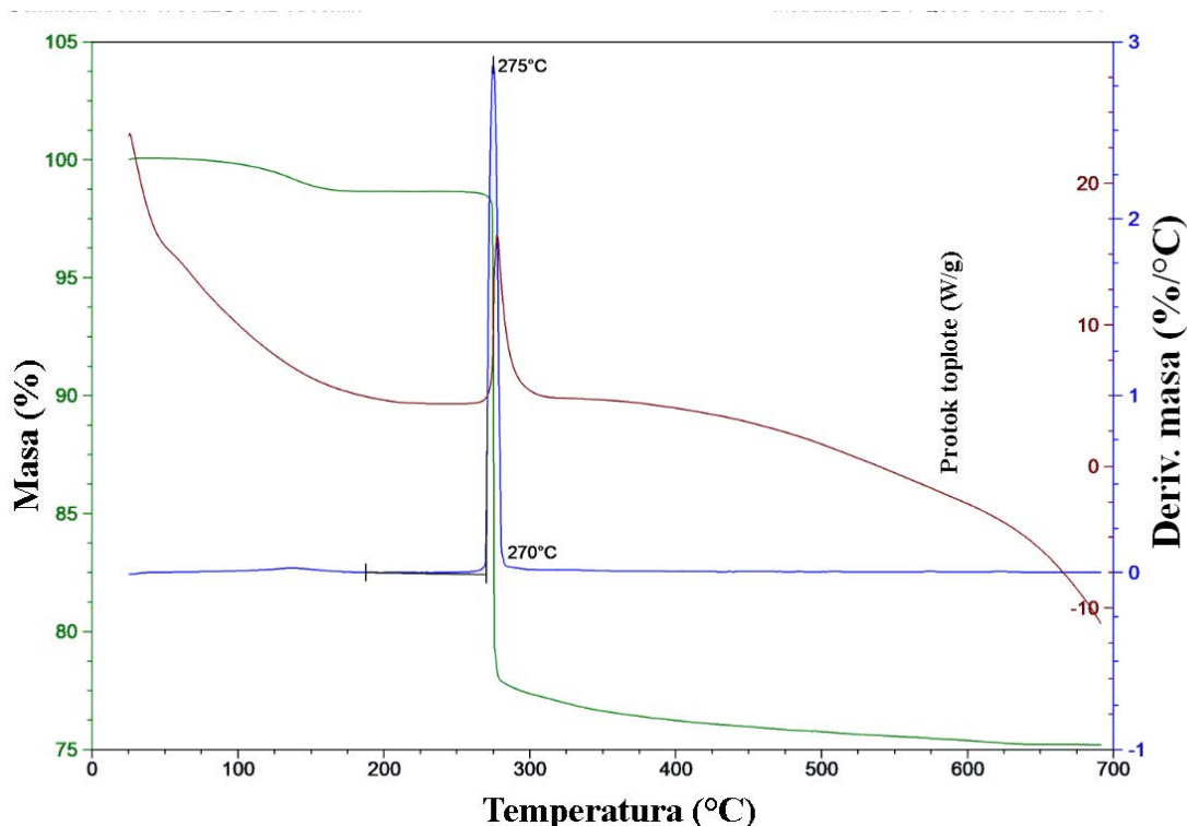
Slika 45. TG, DTG i DSC krive za kompleks 3–Se snimljene u struji azota. Zelenom bojom je označena TG kriva, plavom bojom DTG kriva, a braon bojom DSC kriva.
