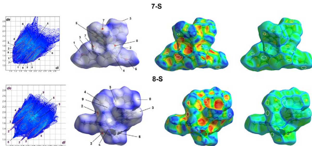
Slika 43. 2D grafikoni otisaka prsta međumolekulskih kontakata i Hiršfeldove površine mapirane sa d_{norm} , indeksom oblika i zakrivljenosti za komplekse 7-S i 8-S .
