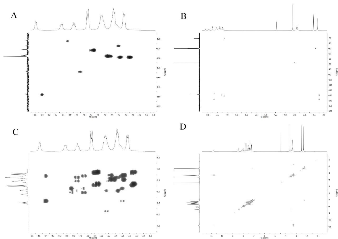
Slika P59. HSQC (A), HMBC (B), COSY (C) i NOESY (D) 2D NMR spektri kompleksa 5-S .
