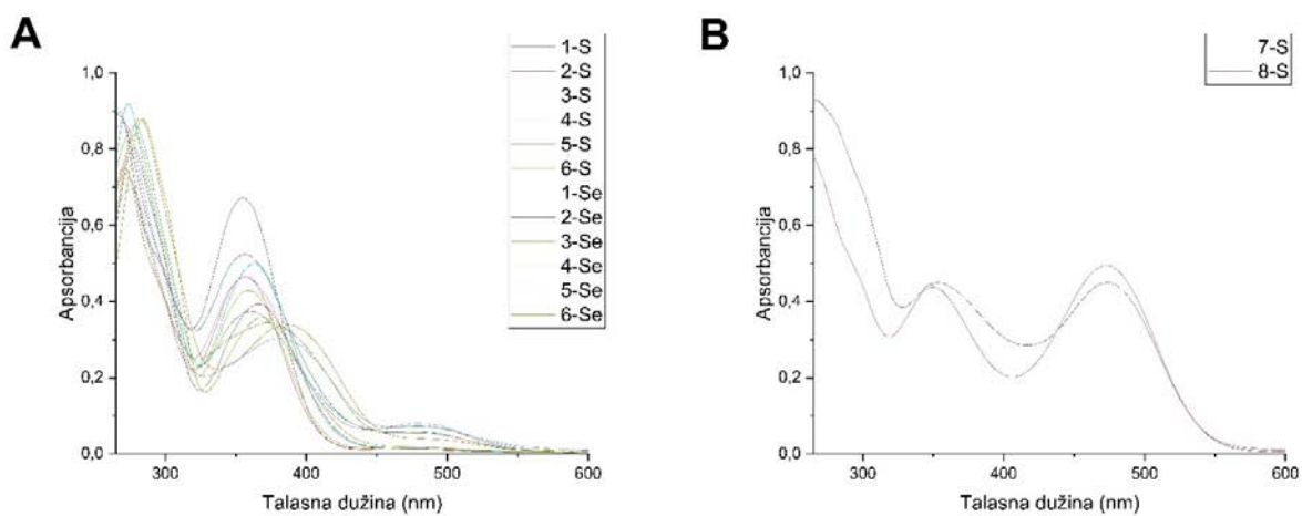
Slika P88. UV-Vis spektri katjonskih kompleksa (A) i neutralnih kompleksa (B).
