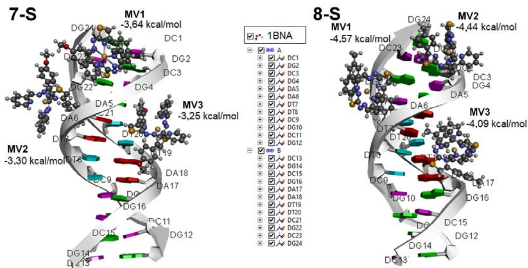
Slika 57. Mesta vezivanja i jačina interakcija vezivanja kompleksa 7–S i 8–S za oligonukleotid (PDB kod: 1BNA) dobijenih doking studijom.
