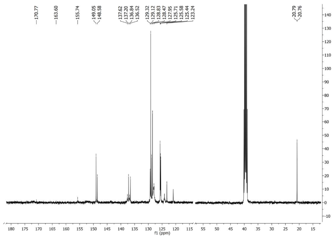
Slika P43. ^{13}\text{C} NMR spektar HLSe 6 snimljen u DMSO- d 6 .
