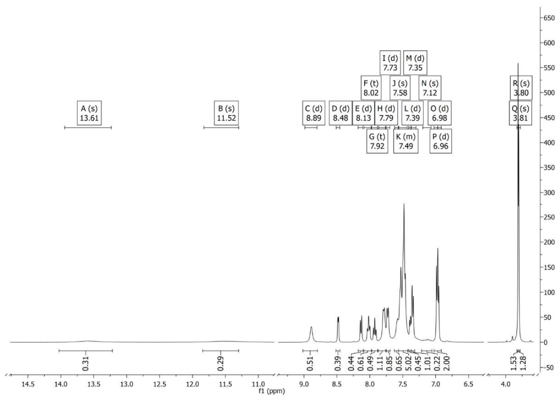
Slika P39. ^1\text{H} NMR spektar HLSe 5 snimljen u \text{DMSO-}d_6 .
