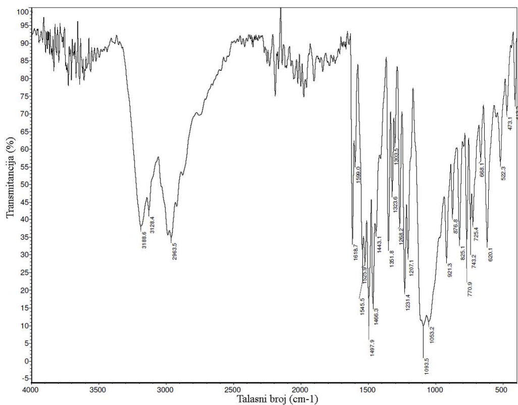
Slika P19. IC spektar kompleksa 2-Se .
