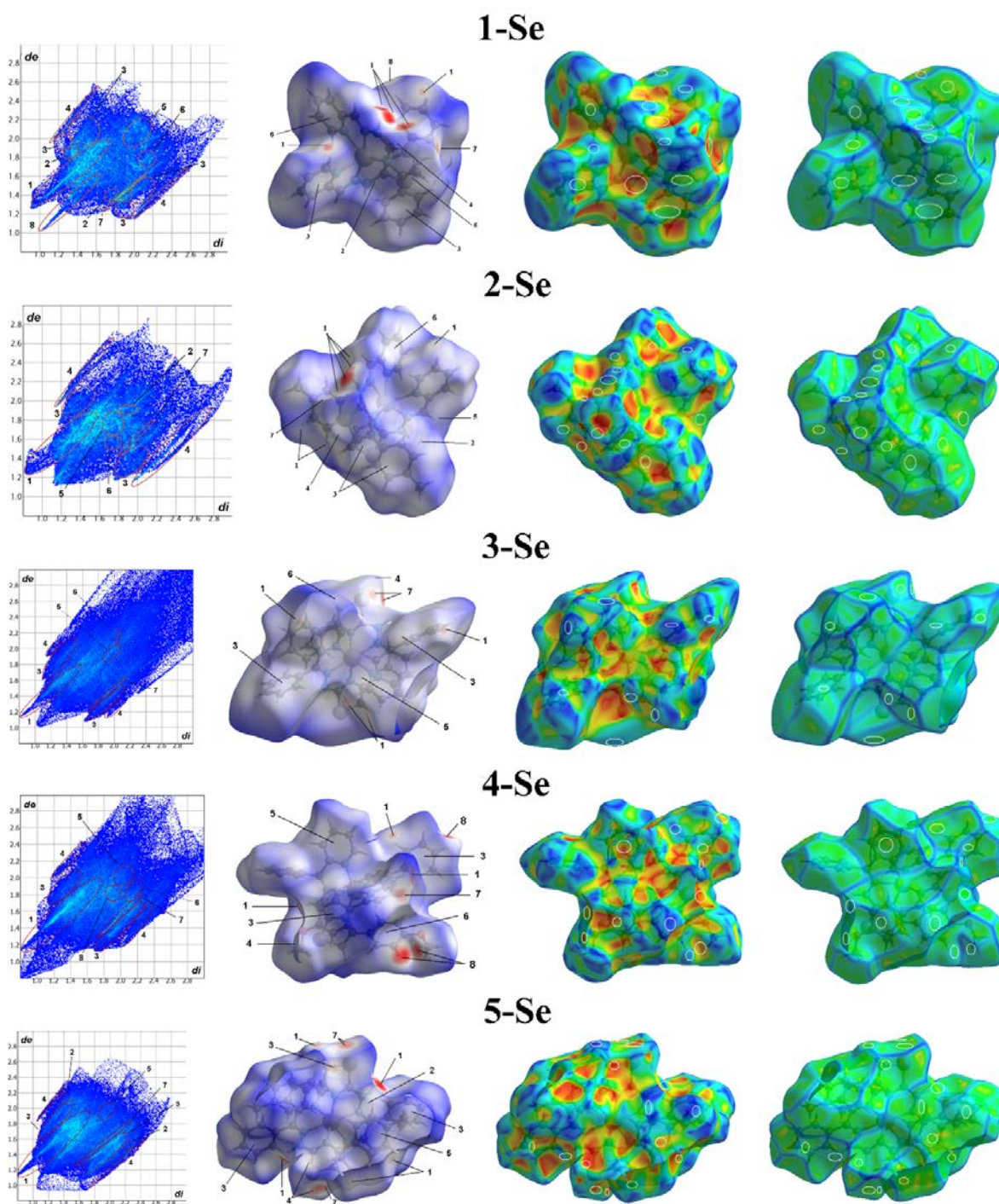
Slika 41. 2D grafikoni otisaka prsta međumolekulskih kontakata i Hiršfeldove površine mapirane sa d_{norm} , indeksom oblika i zakrivljenosti za komplekse (1–5)–Se.
