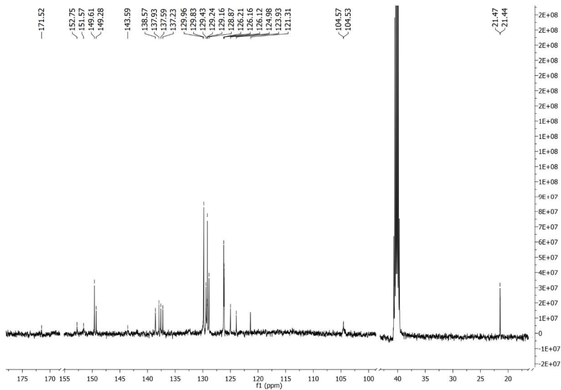
Slika P34. ^{13}\text{C} NMR spektar HLS 6 snimljen u \text{DMSO-}d_6 .
