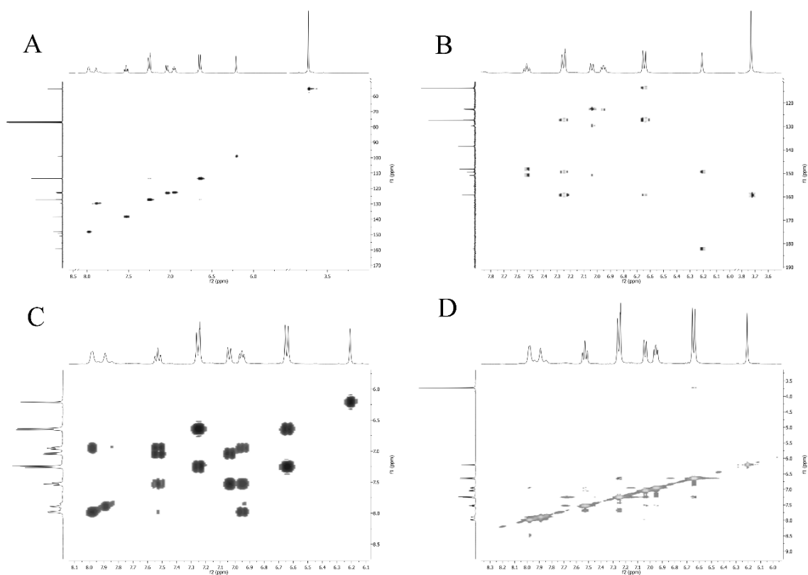
Slika P83. HSQC (A), HMBC (B), COSY (C) i NOESY (D) 2D NMR spektri kompleksa 7-S.
