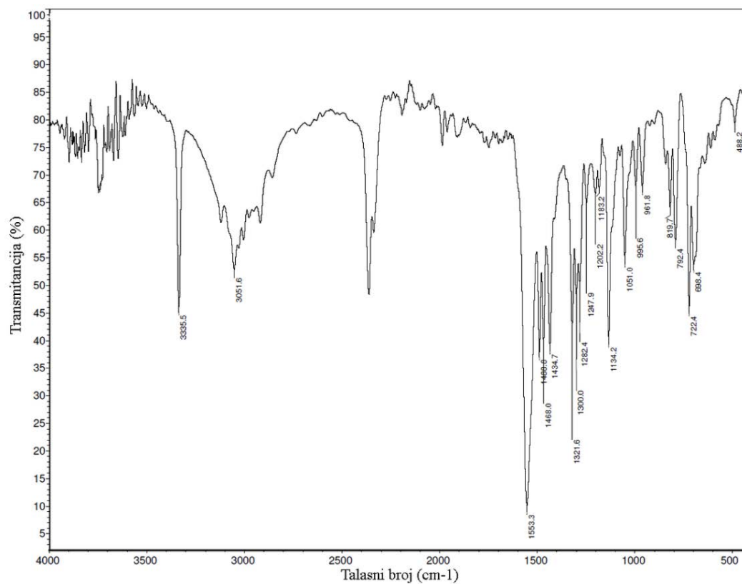
Slika P6. IC spektar liganda HLS 6 .
