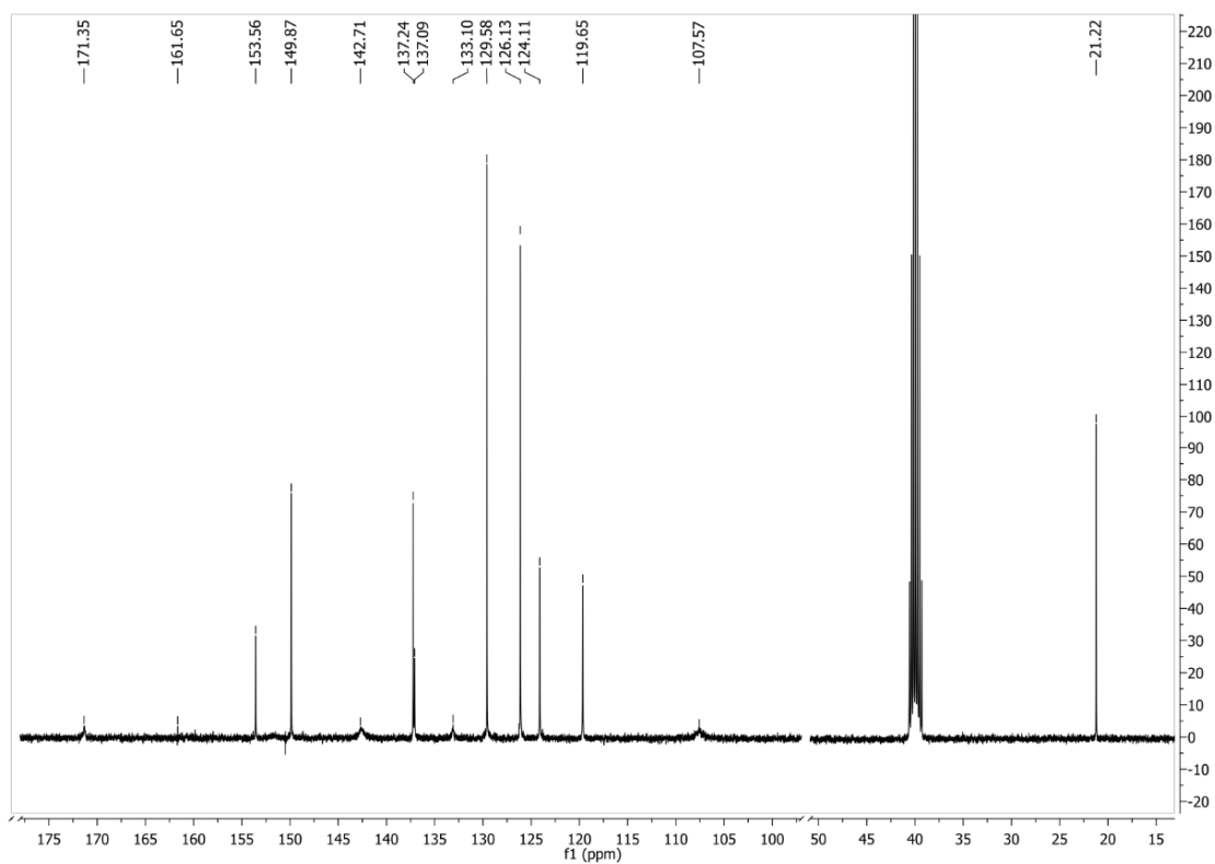
Slika P64. 13 C NMR spektar 2-Se snimljen u DMSO- d 6 .
