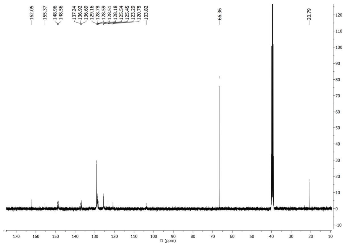
Slika P58. 13 C NMR spektar 5-S snimljen u DMSO- d 6 .
