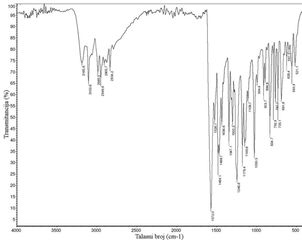
Slika P8. IC spektar liganda HLSe 2 .
