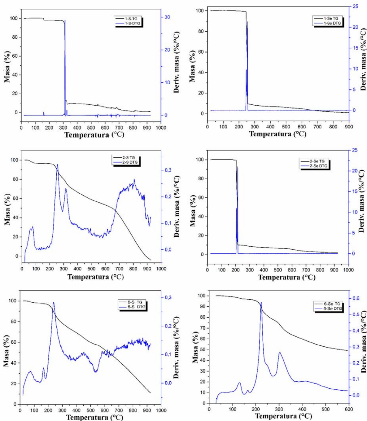
Slika 44. TG i DTG krive za komplekse (1–2)–S/Se i 6–S/Se snimljene u struji argona. Plavom bojom je označena DTG kriva dok je crnom bojom označena TG kriva.
