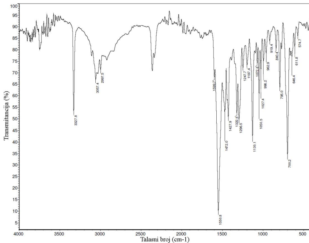
Slika P4. IC spektar liganda HLS 4 .
