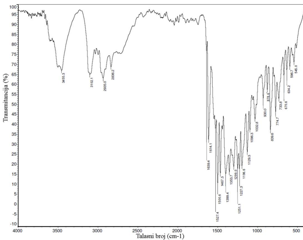
Slika P24. IC spektar kompleksa 6-Se.
