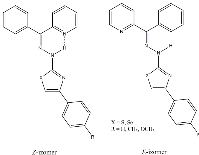
Slika 19. Strukturne formule dva moguća izomerna oblika liganada na bazi 2-benzoilpiridina.
