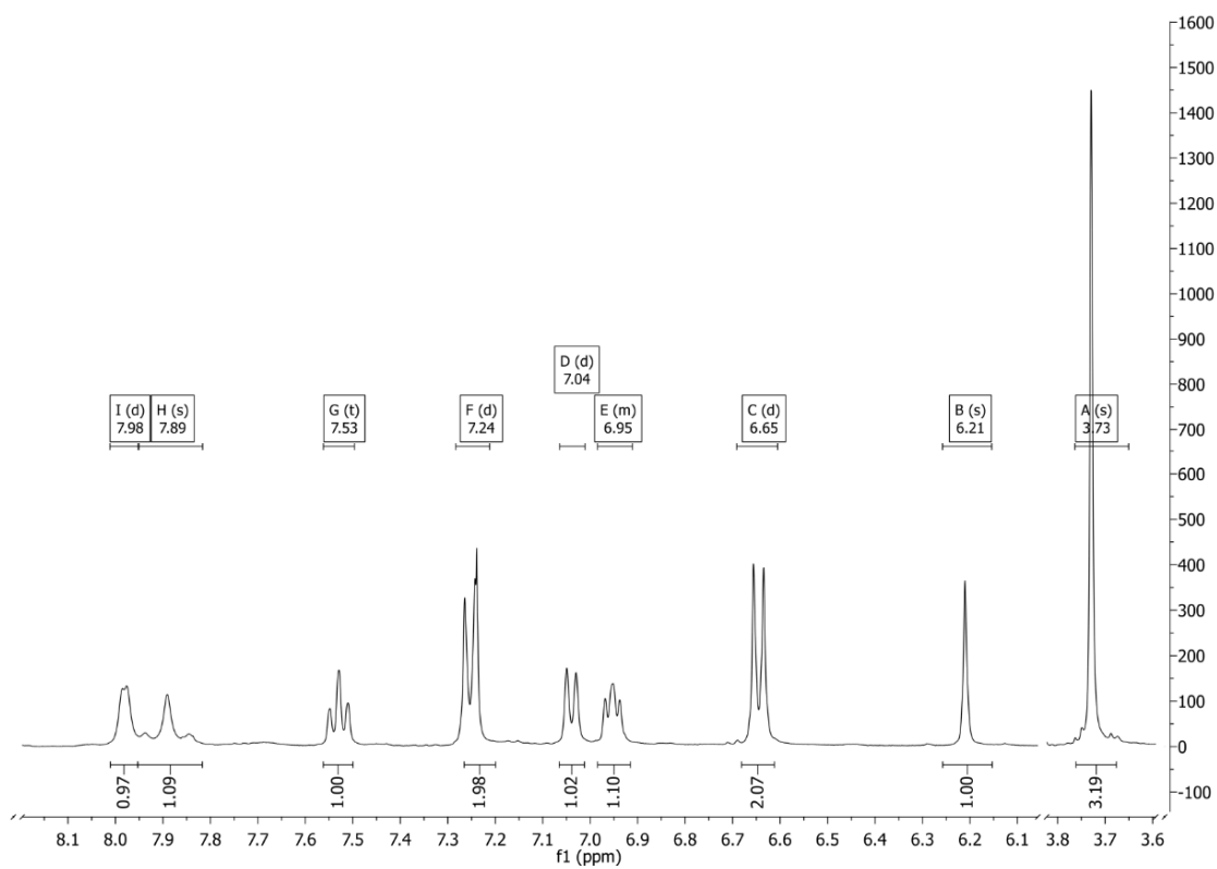
Slika P81. 1 H NMR spektar 7-S snimljen u CDCl 3 .
