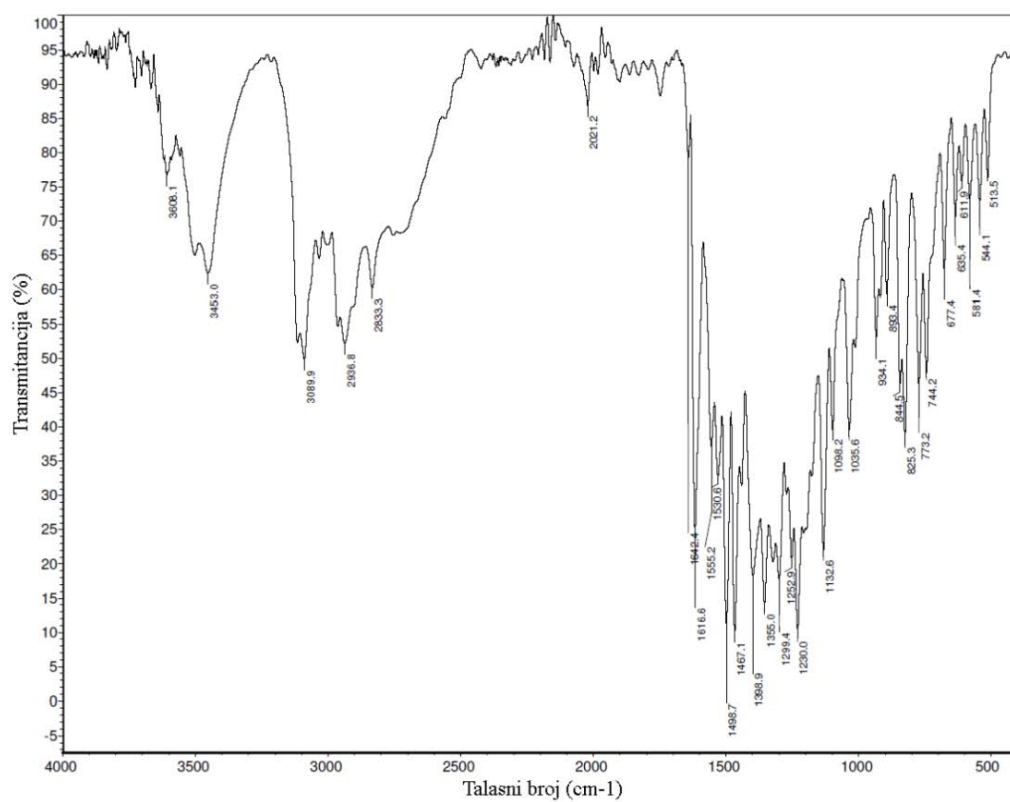
Slika P23. IC spektar kompleksa 6-S.
