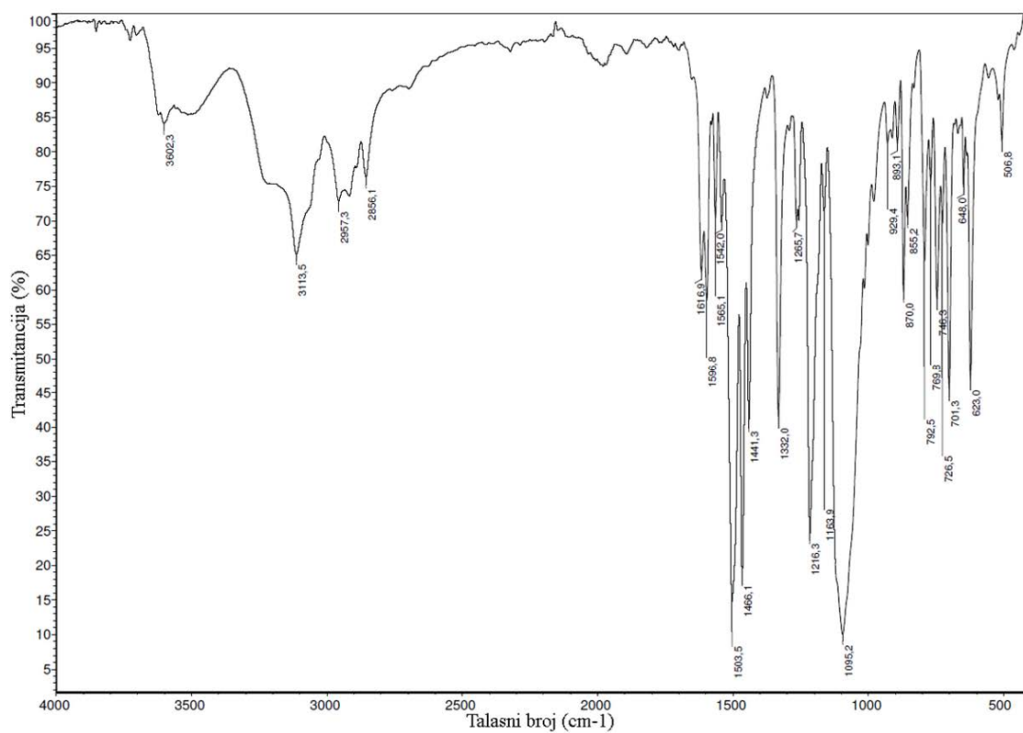
Slika P20. IC spektar kompleksa 3-Se .
