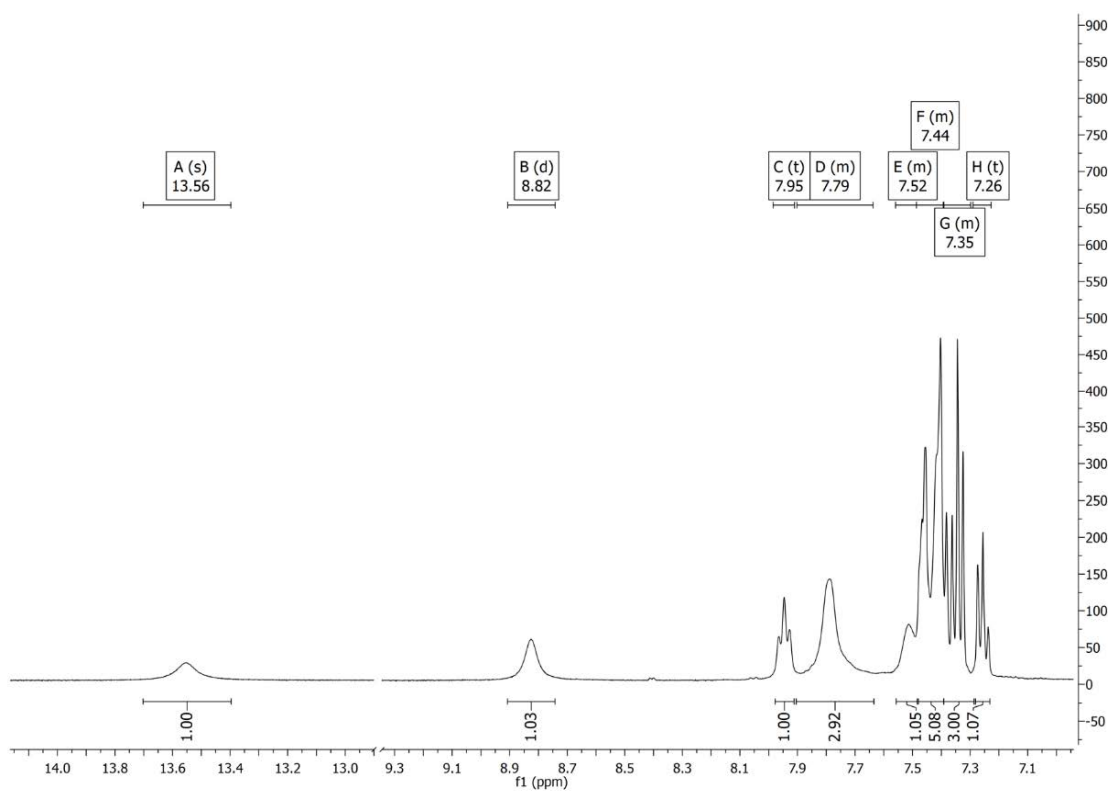
Slika P36. ^1\text{H} NMR spektar HLSe 4 snimljen u \text{DMSO}-d_6 .
