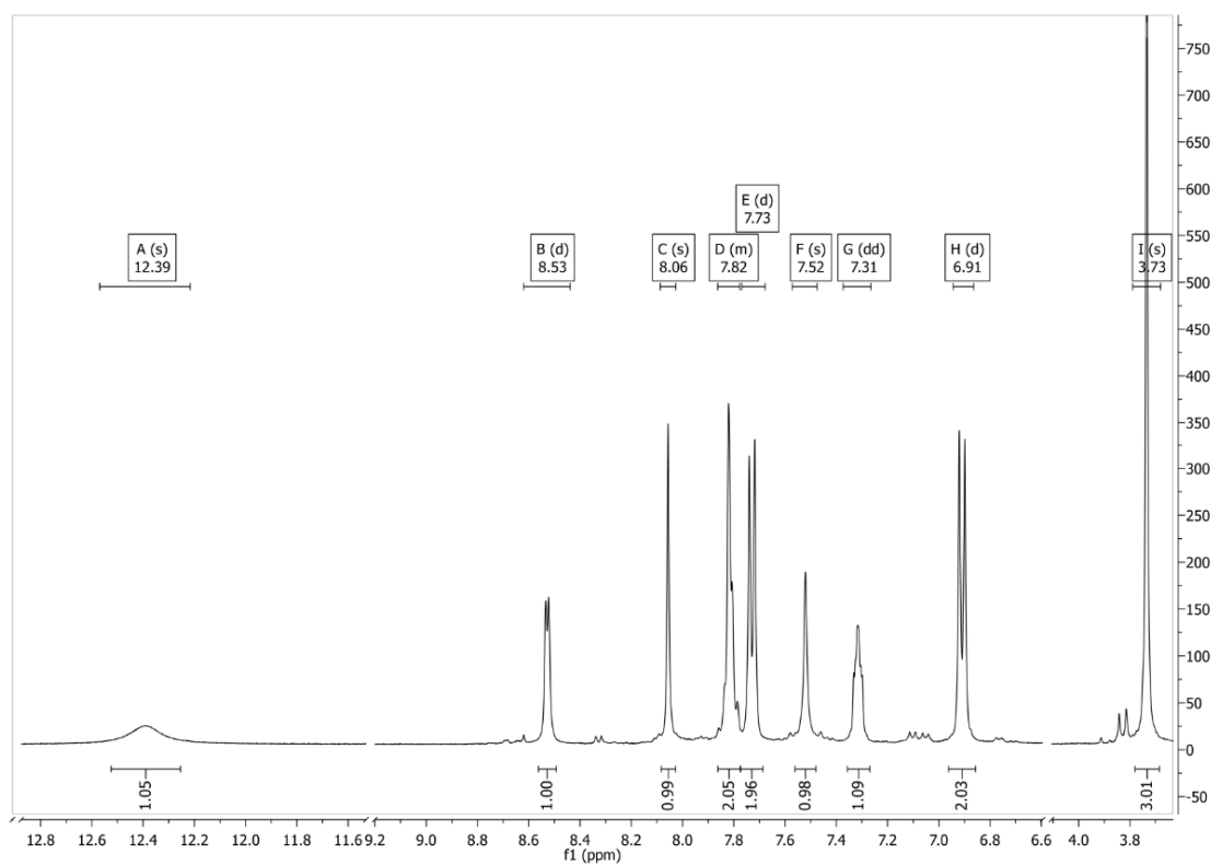
Slika P78. ^1\text{H} NMR spektar 6-Se snimljen u \text{DMSO}-d_6 .
