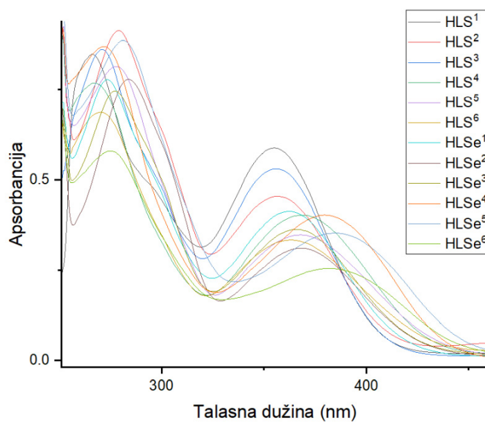
Slika P87. UV-Vis spektri liganada.
