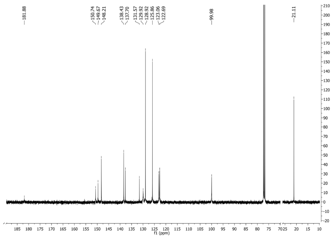
Slika P85. ^{13}\text{C} NMR spektar 8-S snimljen u \text{CDCl}_3 .
