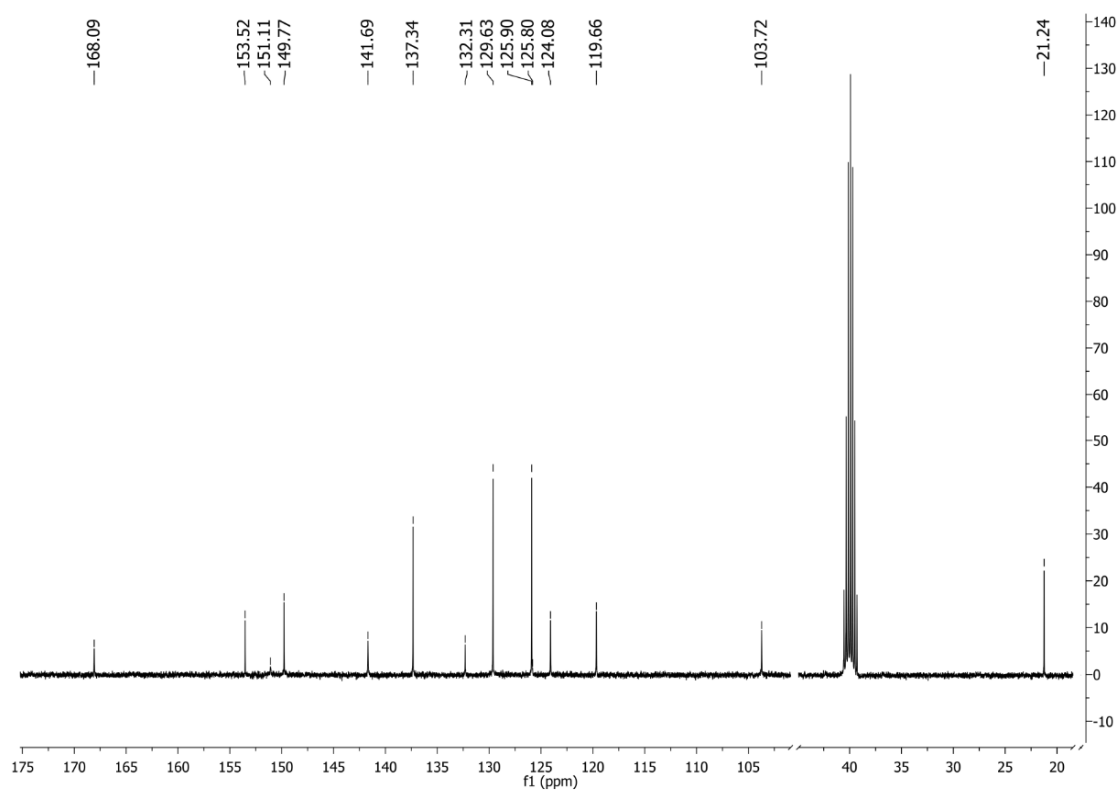
Slika P49. ^{13}\text{C} NMR spektar 2-S snimljen u \text{DMSO-}d_6 .
