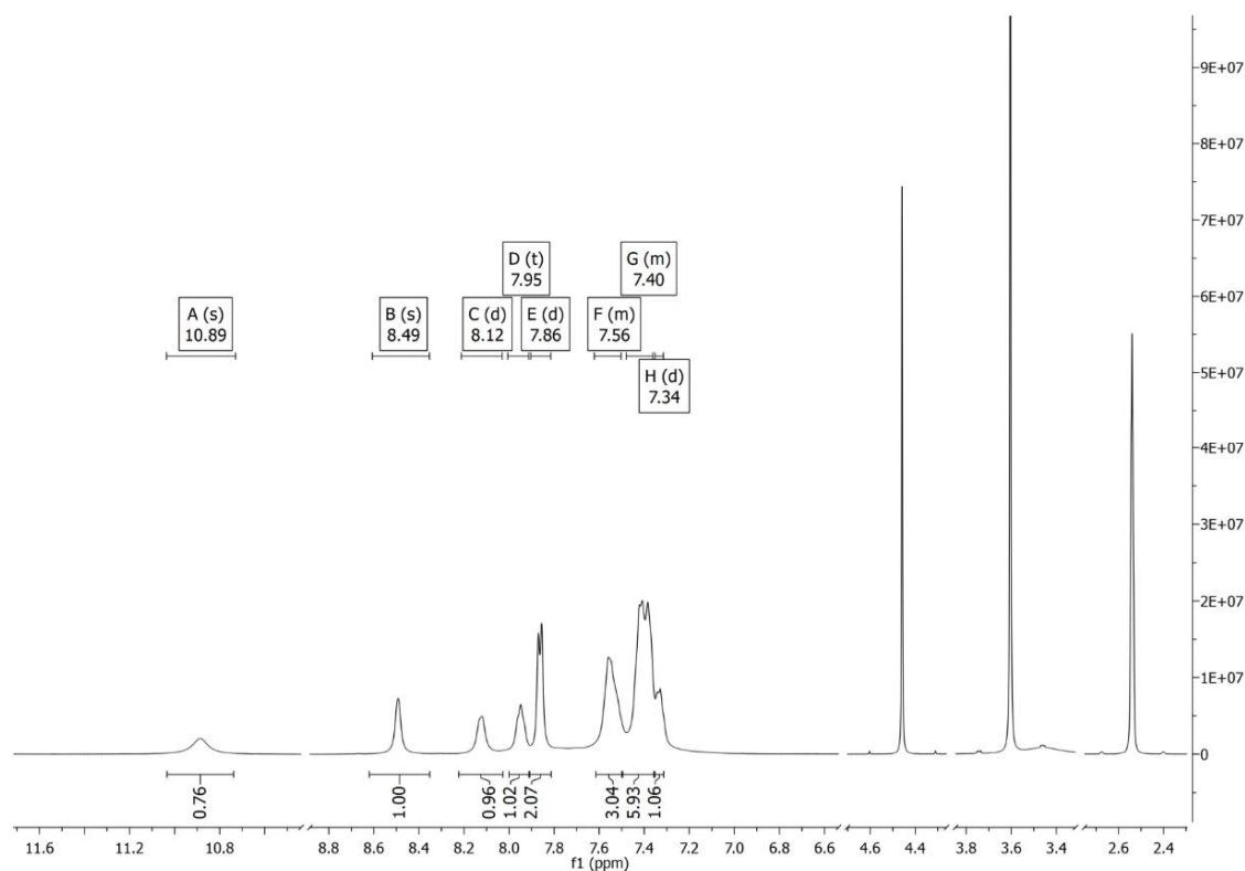
Slika P51. ^1\text{H} NMR spektar 3-S snimljen u \text{DMSO-}d_6 .
