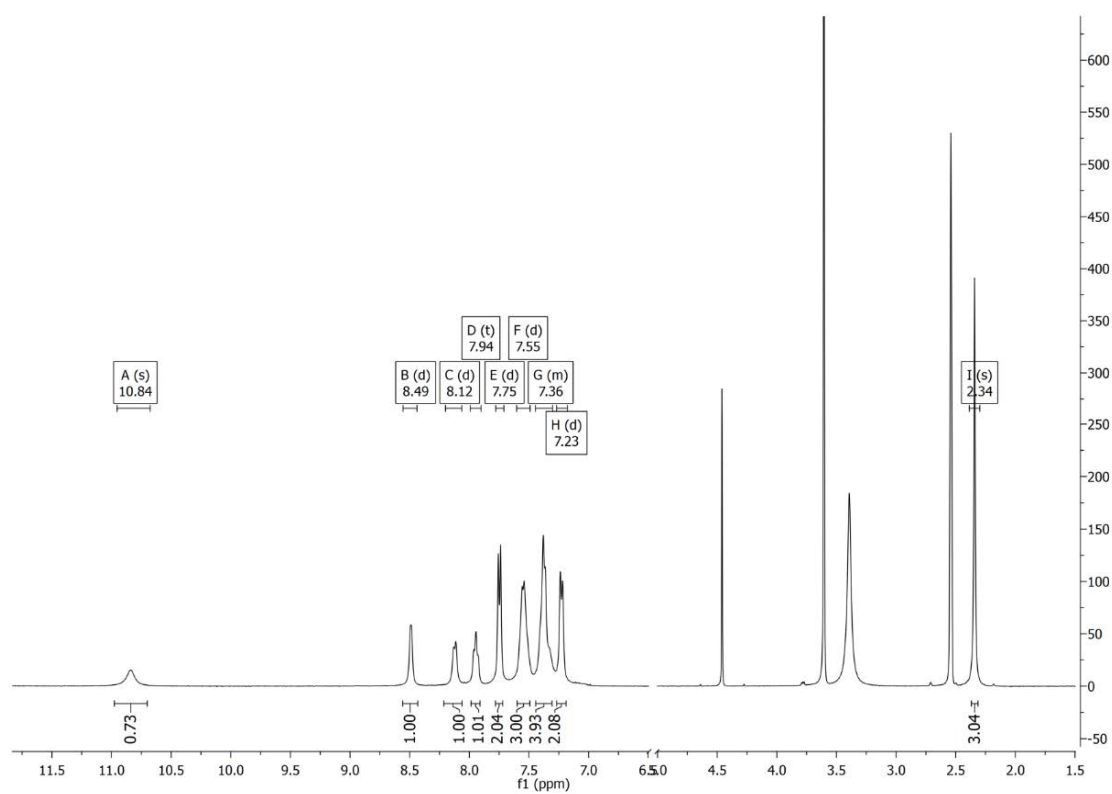
Slika P57. 1 H NMR spektar 5-S snimljen u DMSO- d 6 .
