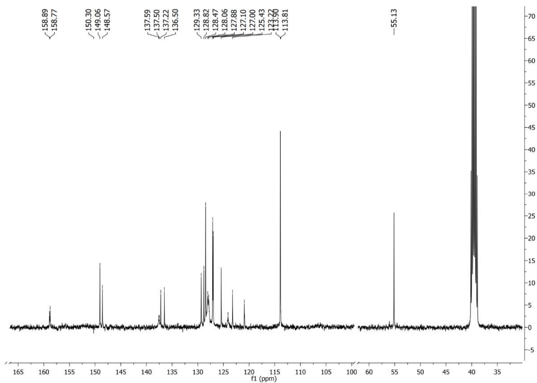
Slika P40. ^{13}\text{C} NMR spektar HLSe 5 snimljen u \text{DMSO-}d_6 .
