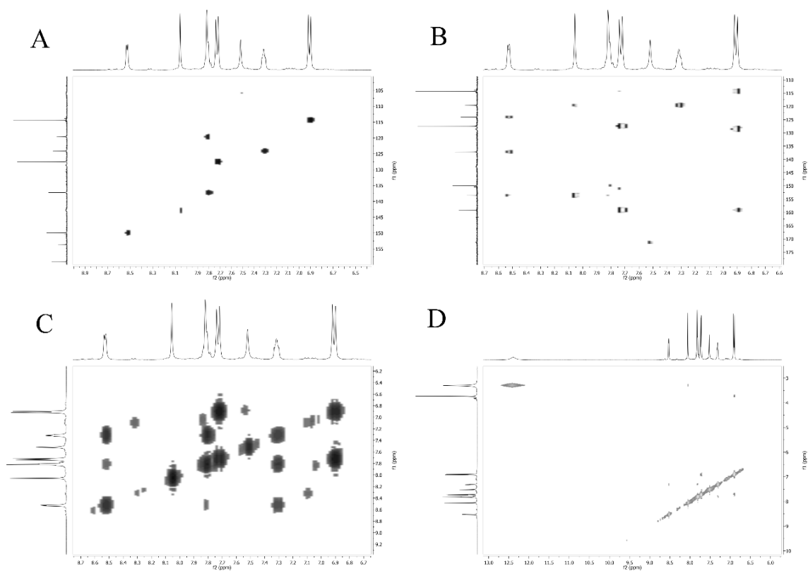
Slika P80. HSQC (A), HMBC (B), COSY (C) i NOESY (D) 2D NMR spektri kompleksa 6-Se .
