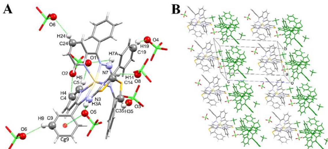
Slika 33. (A) Interakcije odgovorne za formiranje kristalnog pakovanja kompleksa 3–Se . (B) 2D sloj koji je paralelan ab ravni.
