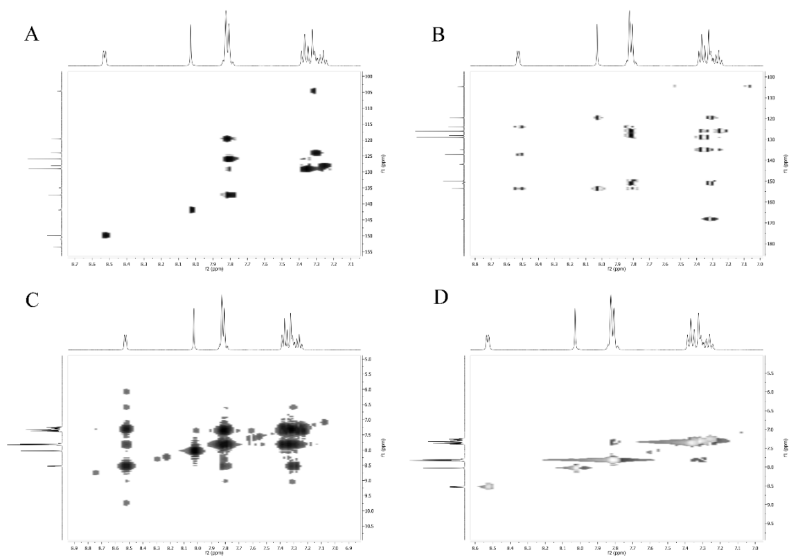
Slika P47. HSQC (A), HMBC (B), COSY (C) i NOESY (D) 2D NMR spektri kompleksa 1-S.
