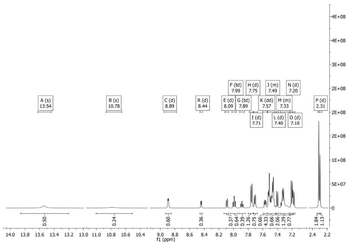
Slika P33. ^1\text{H} NMR spektar HLS 6 snimljen u \text{DMSO-}d_6 .
