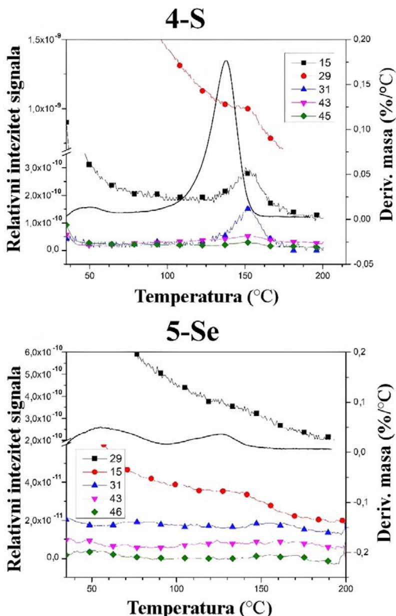
Slika 48. Pikovi koji potiču od etanola ( m/z vrednosti su date na grafiku) nastalih dekompozicijom 4-S i 5-Se (crna boja).
