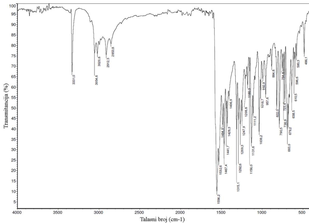
Slika P12. IC spektar liganda HLSe 6 .
