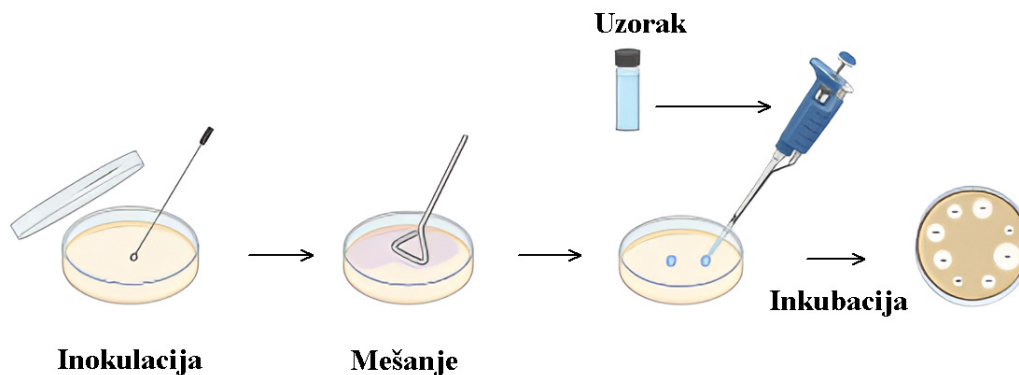
Slika 16. Shematski prikaz agar disk-difuzione metode kreiran na sajtu BioRender.com.
