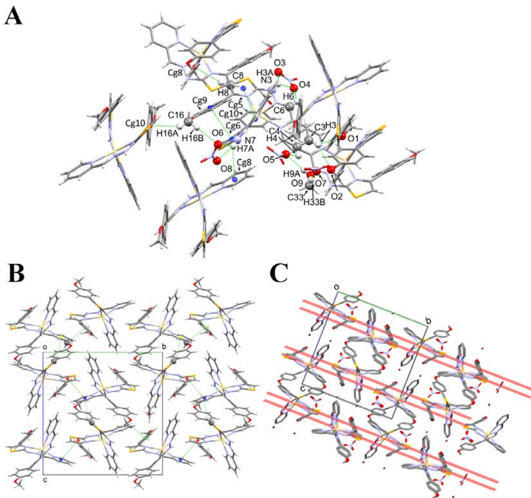
Slika 37. (A) Interakcije odgovorne za formiranje kristalnog pakovanja kompleksa 6–Se . (B) 2D sloj koji je paralelan ac ravni. (C) Međusobno paralelni 2D slojevi koji formiraju 3D kristalno pakovanje. Zbog preglednosti atomi vodonika su uklonjeni iz prikaza.
