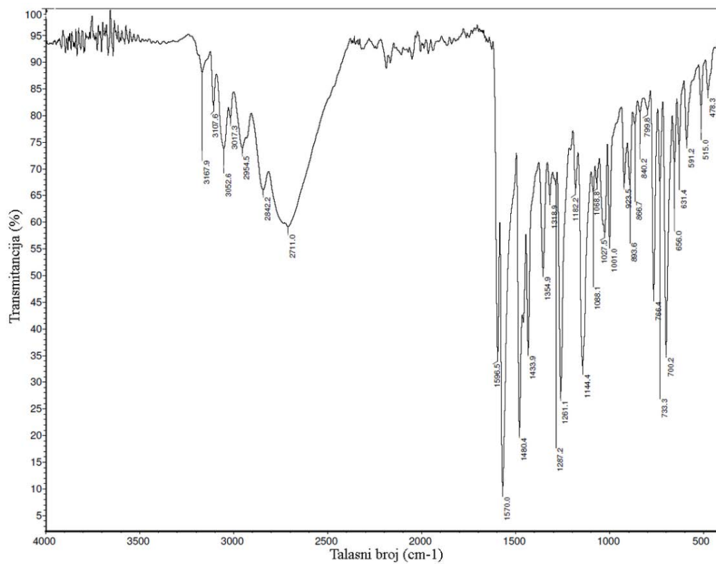
Slika P7. IC spektar liganda HLSe 1 .
