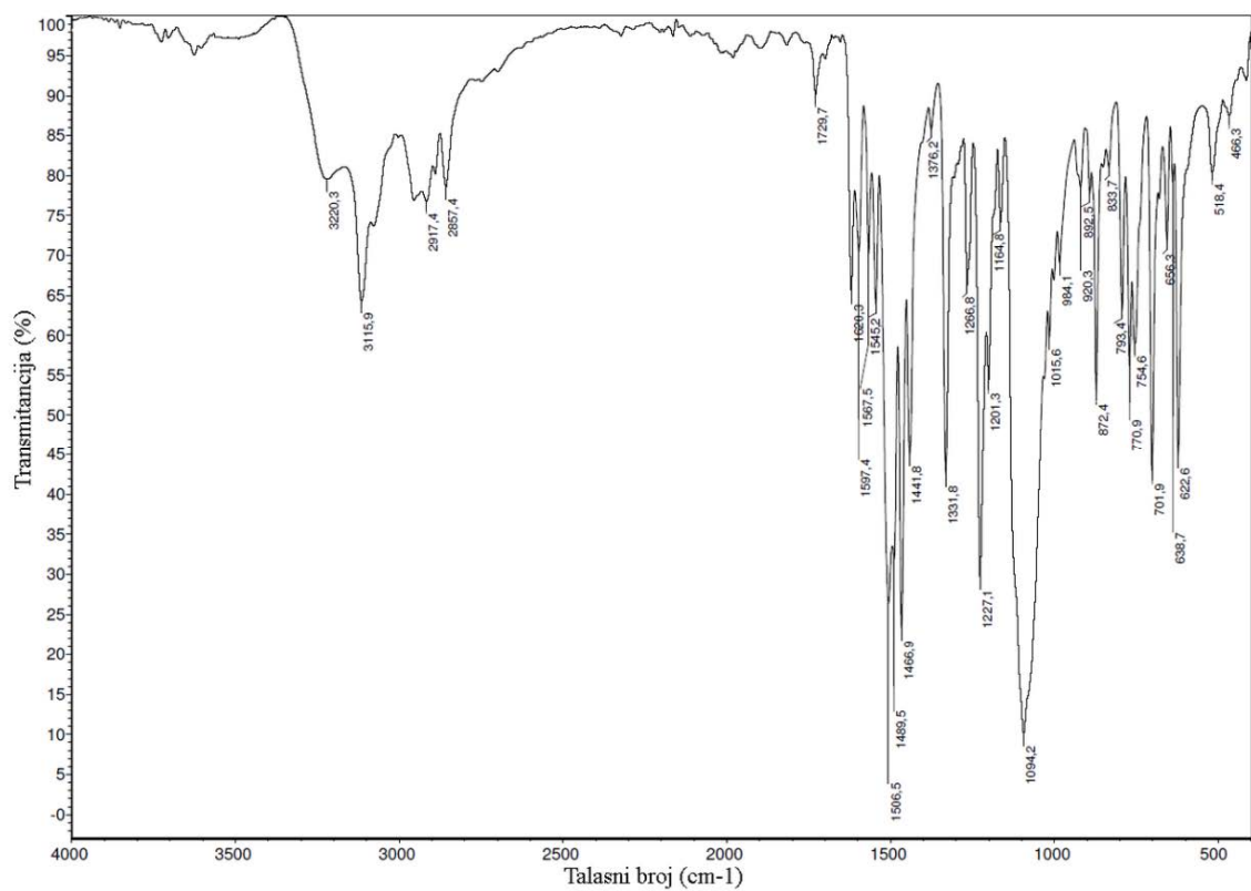
Slika P15. IC spektar kompleksa 3-S.
