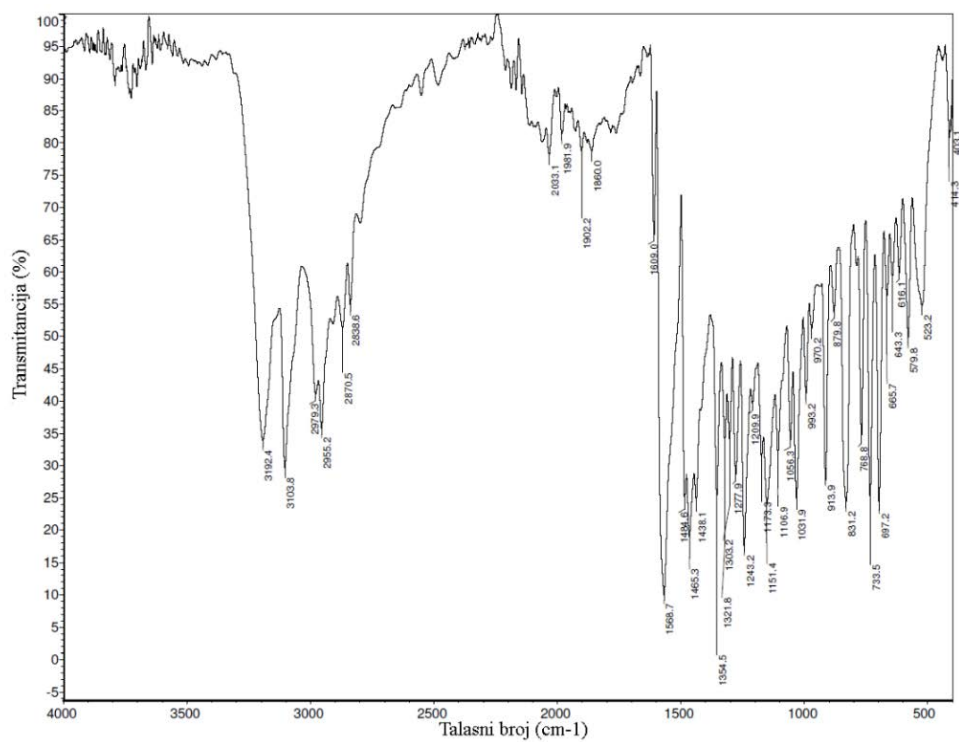
Slika P2. IC spektar liganda HLS 2 .
