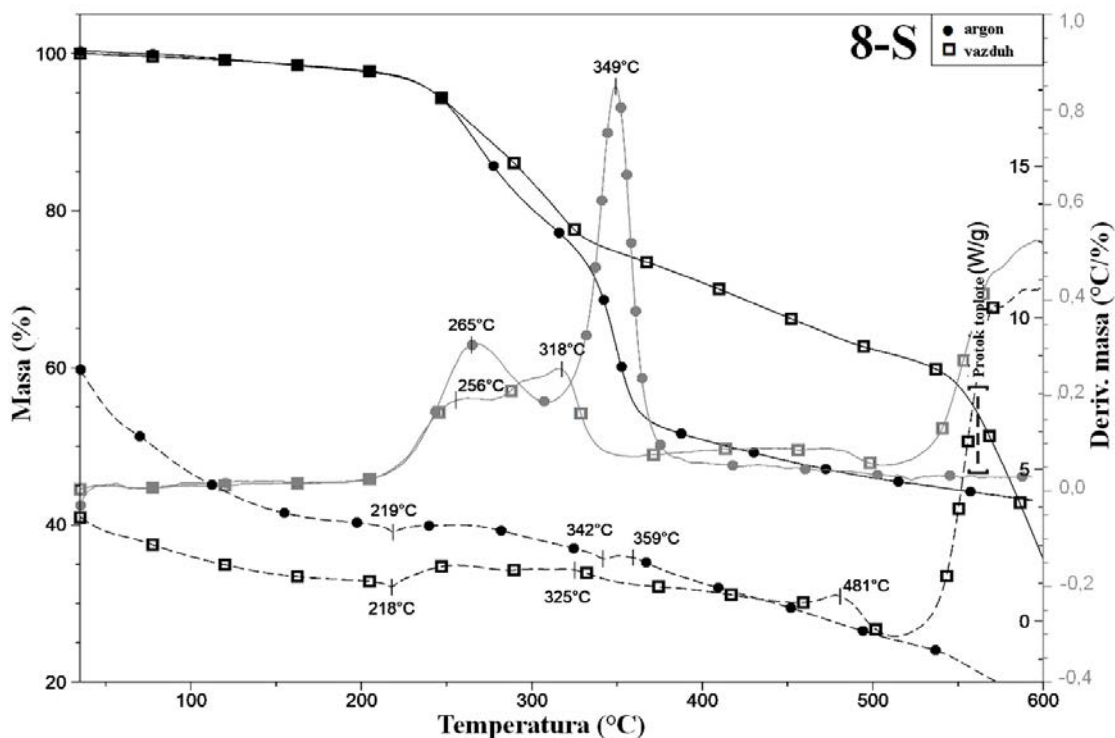
Slika 52. TG, DTG i DSC krive za kompleks 8-S snimljene u struji argona i vazduha. Pune linije crne boje predstavljaju TG krive, pune linije sive boje predstavljaju DTG krive, a isprekidane crne linije predstavljaju DSC krive.
