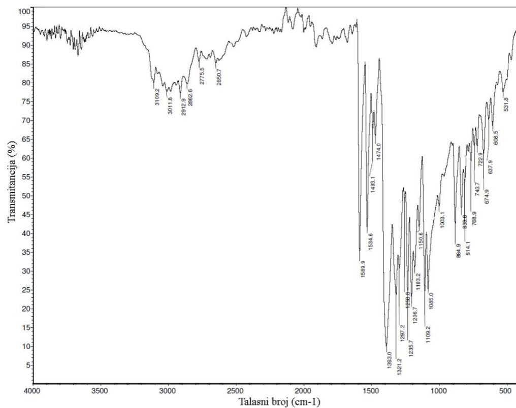
Slika P26. IC spektar kompleksa 8-S.
