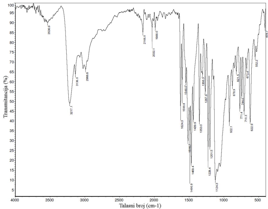
Slika P18. IC spektar kompleksa 1-Se .
