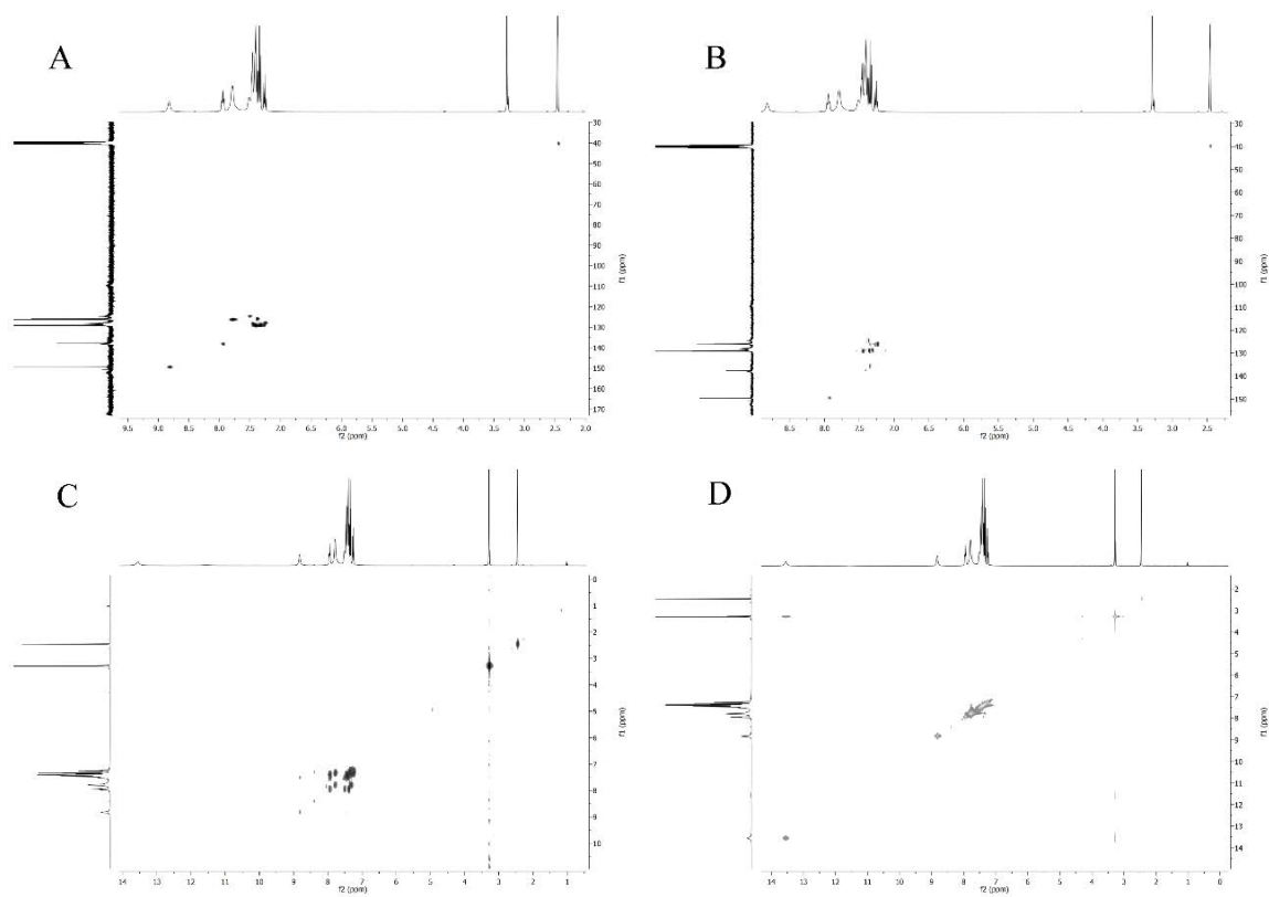
Slika P38. HSQC (A), HMBC (B), COSY (C) i NOESY (D) 2D NMR spektri liganda HLSe 4 .
