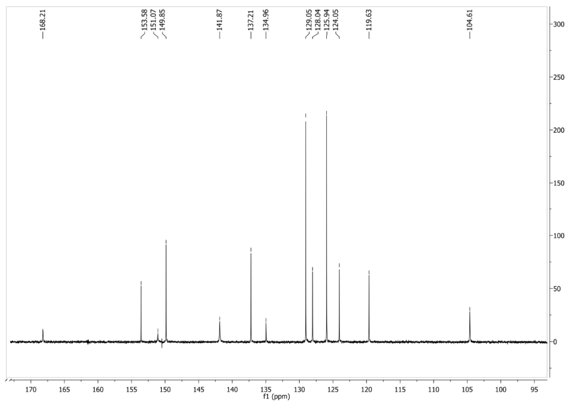
Slika P46. 13 C NMR spektar 1-S snimljen u DMSO- d 6 .
