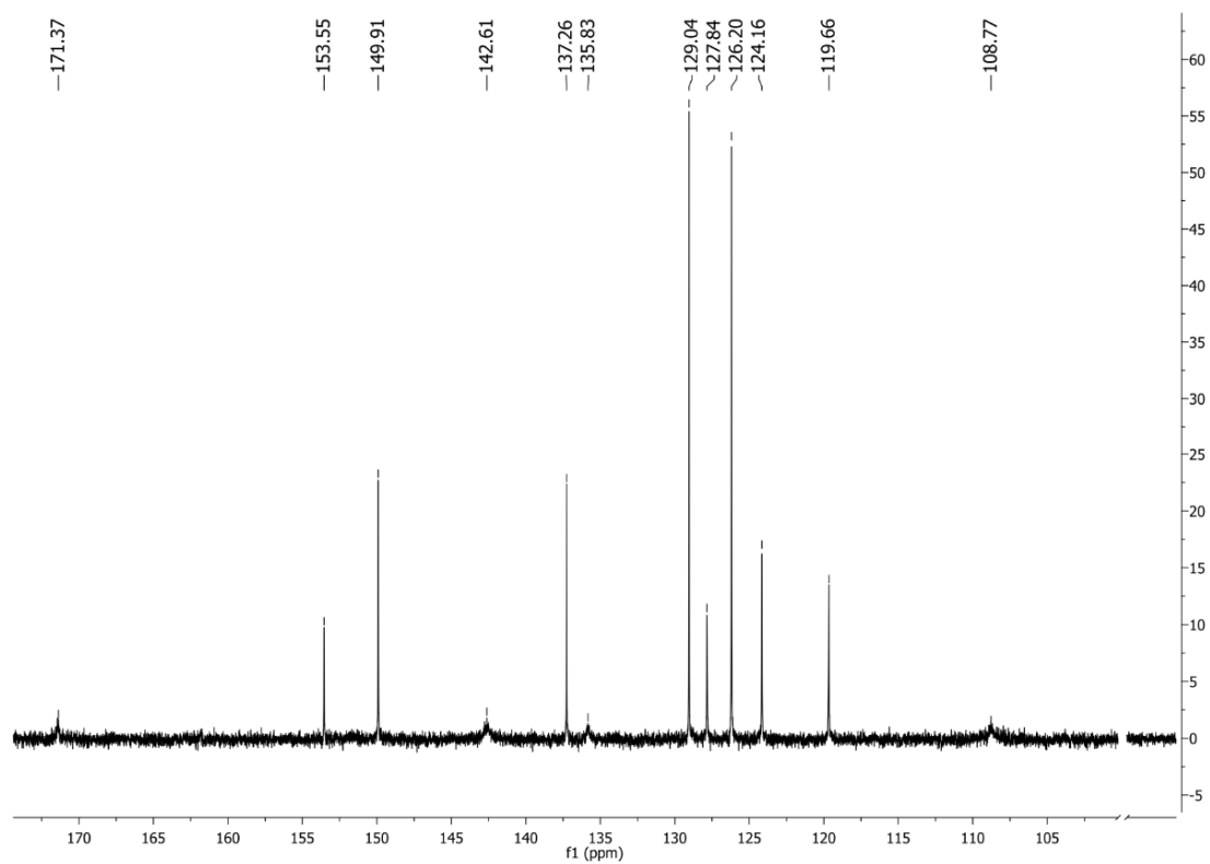
Slika P61. ^{13}\text{C} NMR spektar 1-Se snimljen u \text{DMSO-}d_6 .
