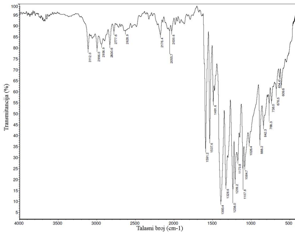
Slika P25. IC spektar kompleksa 7-S.
