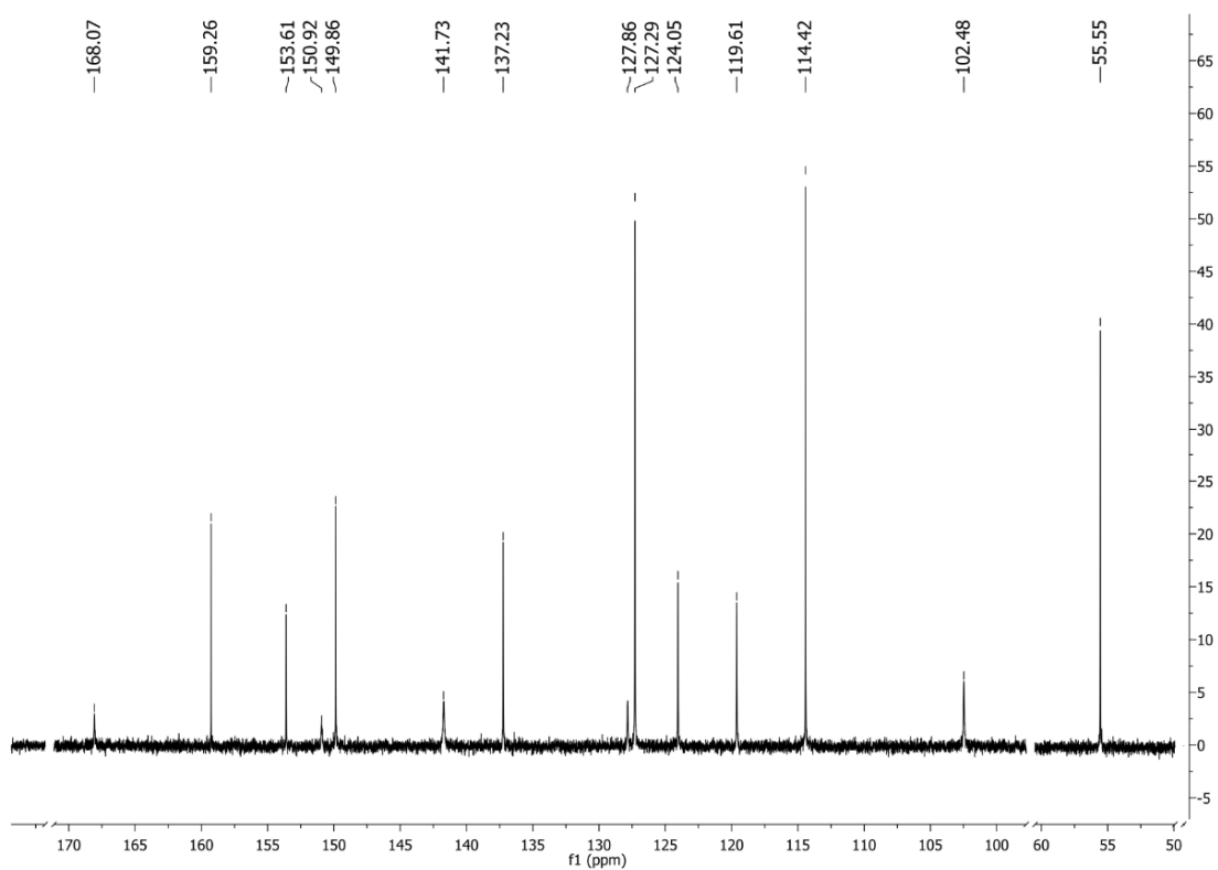
Slika P76. 13 C NMR spektar 6-S snimljen u DMSO- d 6 .
