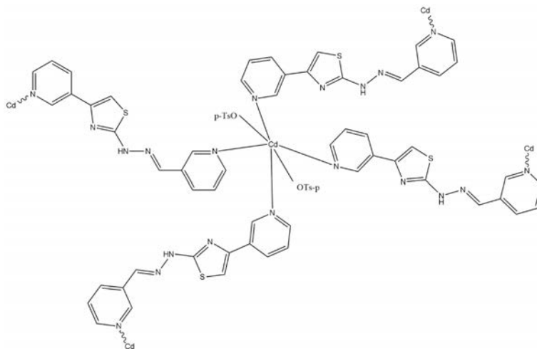
Slika 14. Pretpostavljena molekulska struktura kompleksa 4 .
