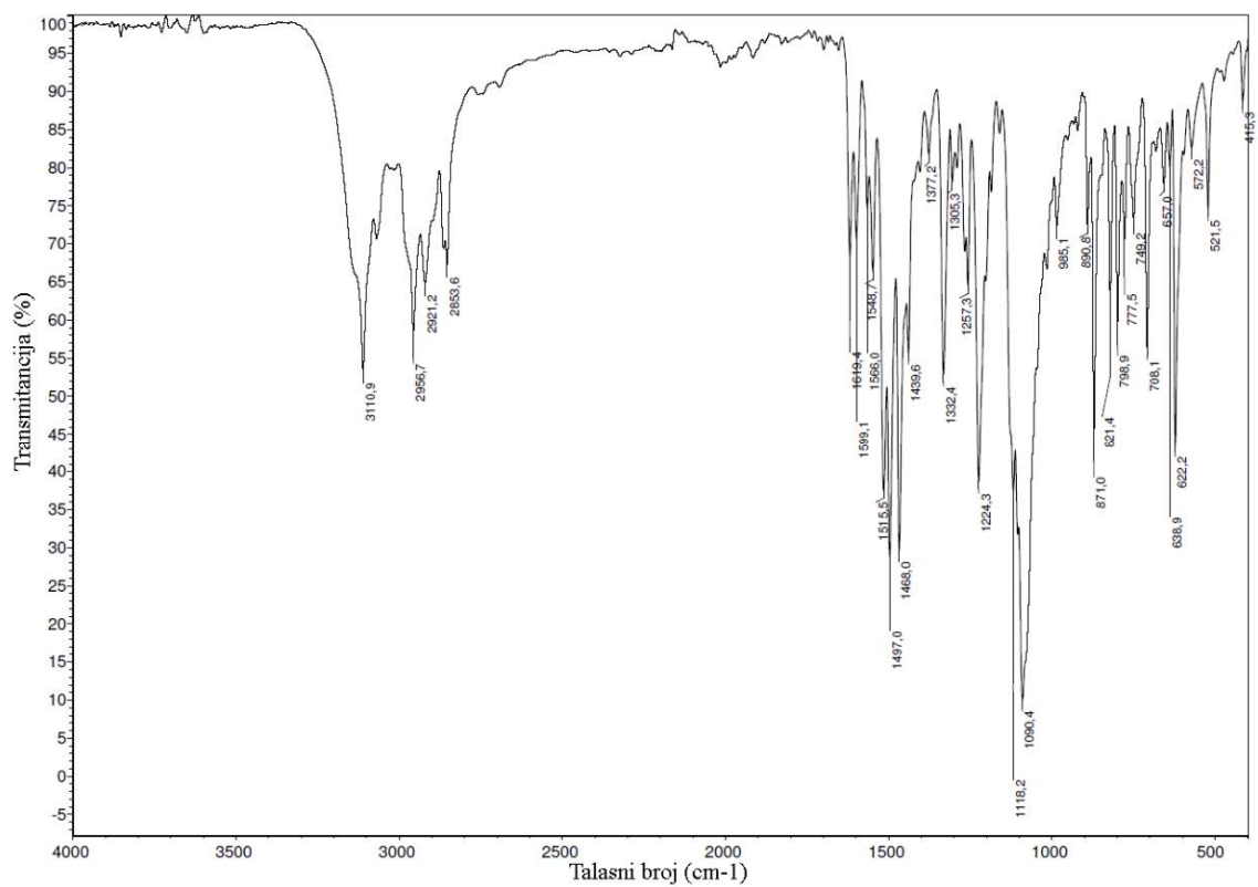
Slika P17. IC spektar kompleksa 5-S .
