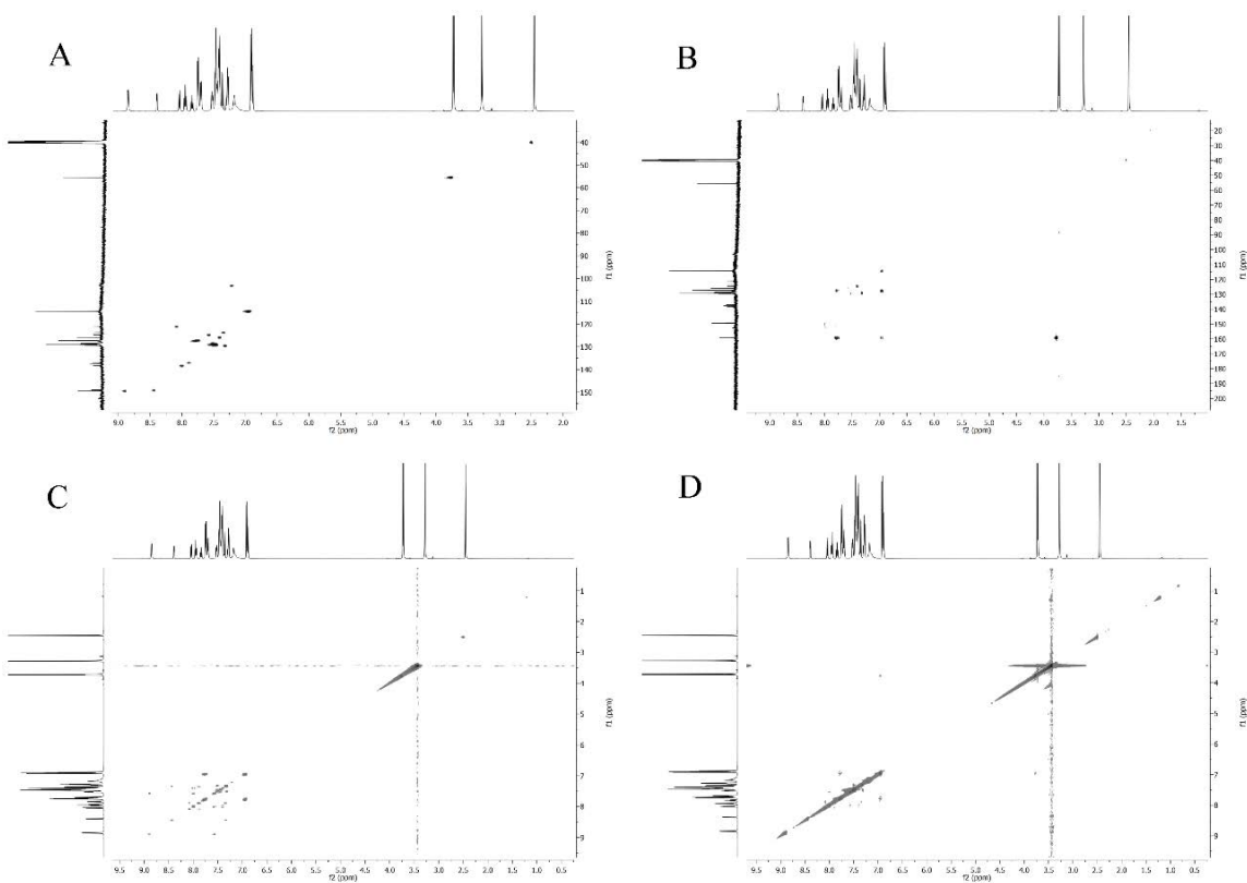
Slika P32. HSQC (A), HMBC (B), COSY (C) i NOESY (D) 2D NMR spektri liganda HLS 5 .
