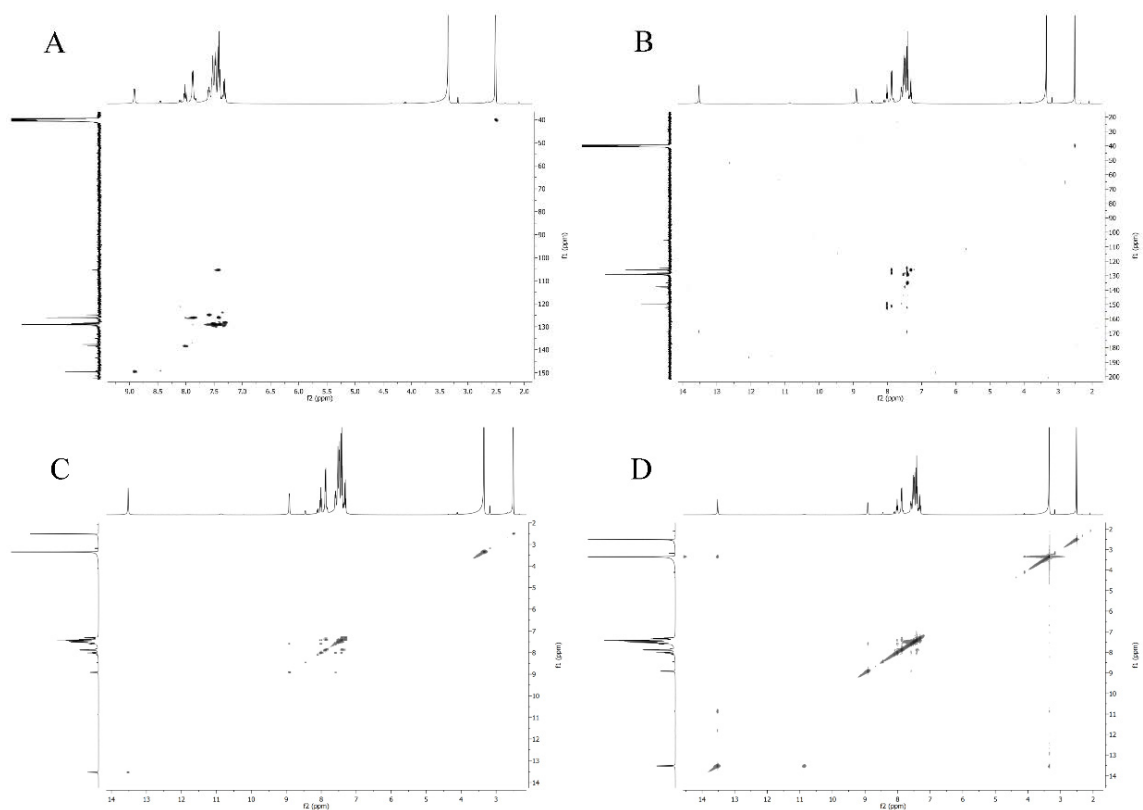
Slika P29. HSQC (A), HMBC (B), COSY (C) i NOESY (D) 2D NMR spektri liganda HLS 4 .
