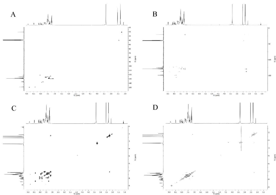
Slika P44. HSQC (A), HMBC (B), COSY (C) i NOESY (D) 2D NMR spektri liganda HLSe 6 .
