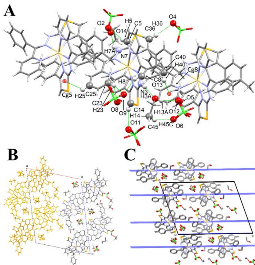
Slika 35. (A) Interakcije odgovorne za formiranje kristalnog pakovanja kompleksa 5–Se . (B) 2D sloj koji je paralelan (10–1) ravni. (C) Međusobno paralelni 2D slojevi koji formiraju 3D kristalno pakovanje. Zbog preglednosti atomi vodonika su uklonjeni iz prikaza.
