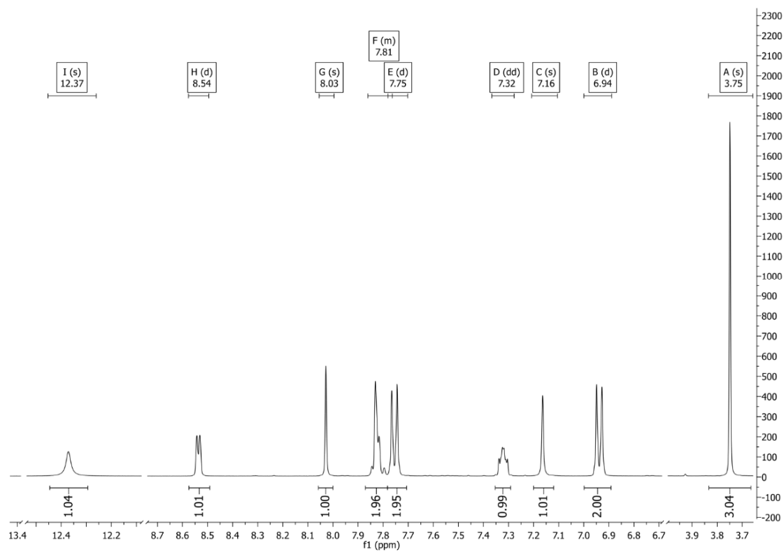
Slika P75. 1 H NMR spektar 6-S snimljen u DMSO- d 6 .
