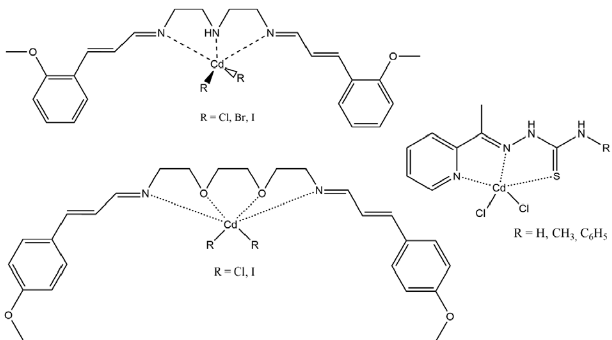
Slika 18. Strukturne formule odabranih kompleksa Cd(II) koji pokazuju antioksidativni potencijal.
