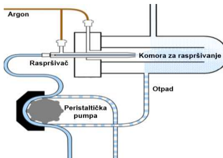
Slika 35. Prikaz sistema za uvođenje uzorka u plazmu
