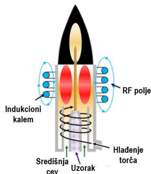
Slika 36. Prikaz torča (plamenika)
