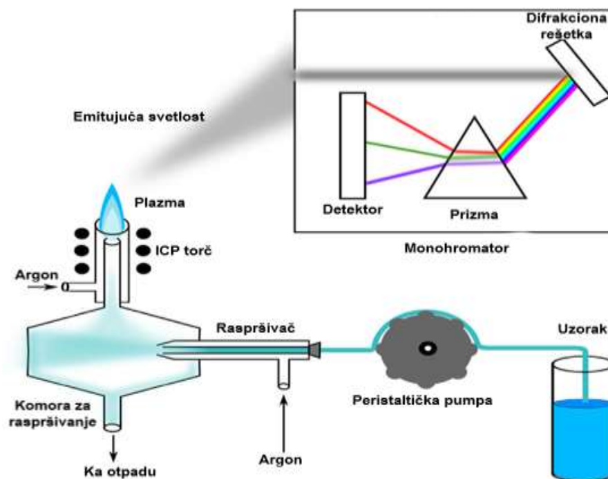
Slika 41. Šema ICP-OES uređaja
