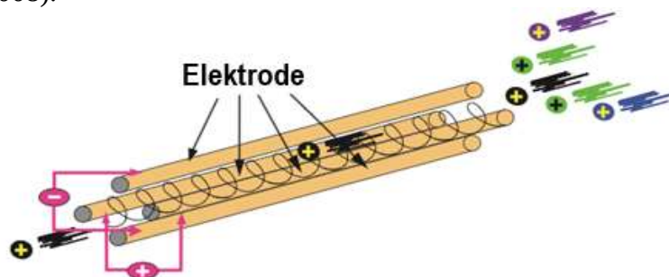
Slika 38: Prikaz kvadrupola
