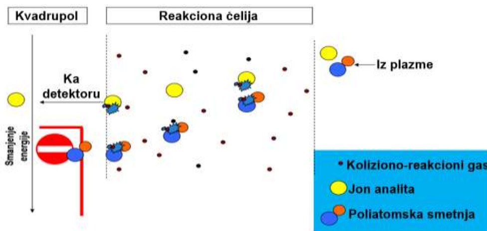
Slika 40. Princip koliziono-reakcione ćelije
