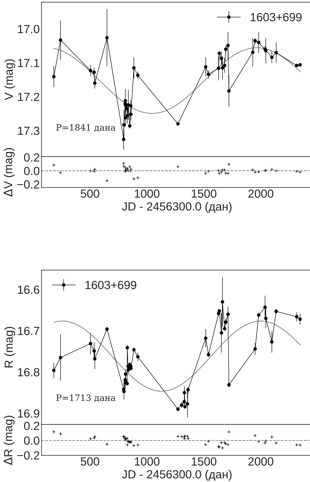
Слика 3.24: Криве сјаја објекта 1603+699 са функцијом усклађивања чији су параметри одређени методом DCDFT: у V домену (горе) и R домену (доле). У доњем левом углу је вредност периода P .
