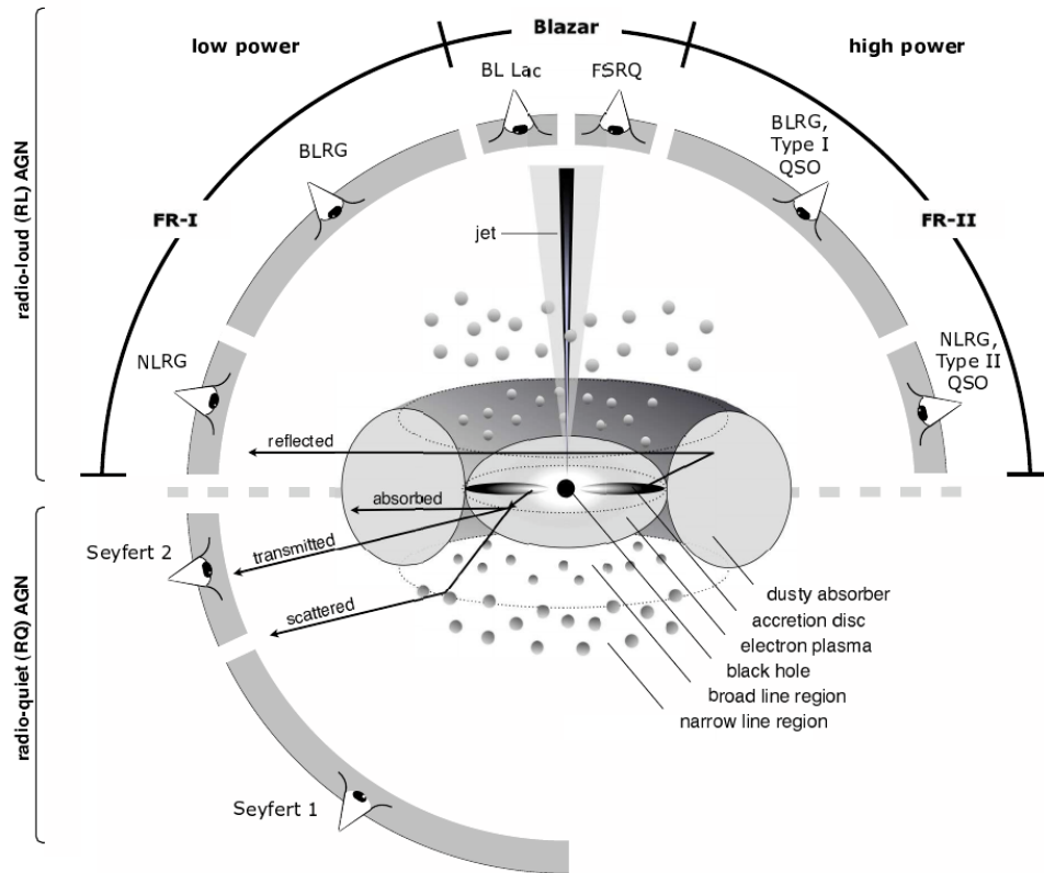
Слика 1.2: Шематски приказ унификационог модела преузет из Beckmann & Shrader (2012a).
