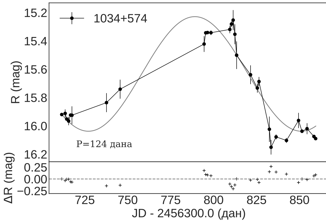
Слика 3.16: Криве сјаја објекта 1034+574 са функцијом усклађивања чији су параметри одређени методом DCDFT: у V домену (горе) и R домену (доле), само ТЈО посматрања. У доњем левом углу је вредност периода у данима.
