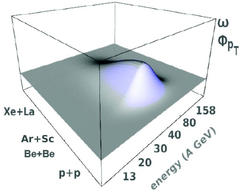
Slika 11: Očekivana slika (3D) povećanja fluktuacija sa maksimumom koji odgovara poziciji kritične tačke faznog prelaza hadronski gas - QGP. Ose su redom: veličine sistema koji se sudaraju na eksperimentu, vrednosti impulsa projektila i varijable čije se ponašanje analizira.
