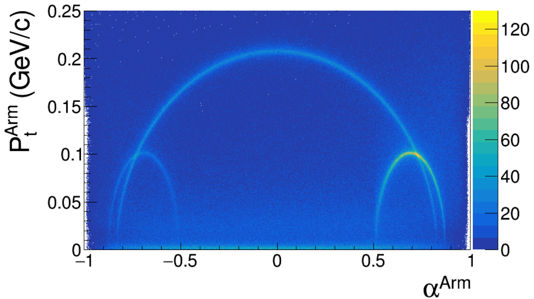
Slika 65: Armenteros-Podolanski kontrolni histogram nakon primene selekcionog kriterijuma za minimalno dozvoljeno rastojanje između primarnog i sekundarnog verteksa ( \Delta z ).
