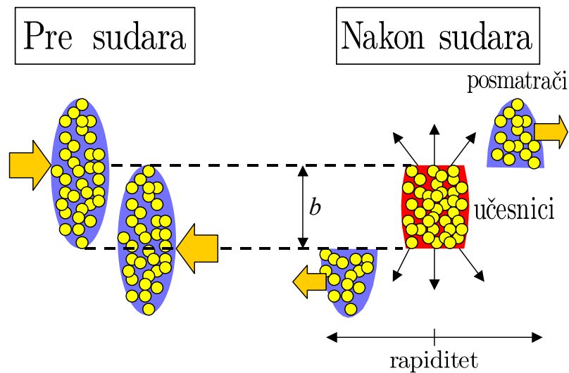
Slika 6: Shematski prikaz sudara relativističkih jona. Nukleoni su podeljeni na učesnike i posmatrače pomoću impakt parametra sudara b .
