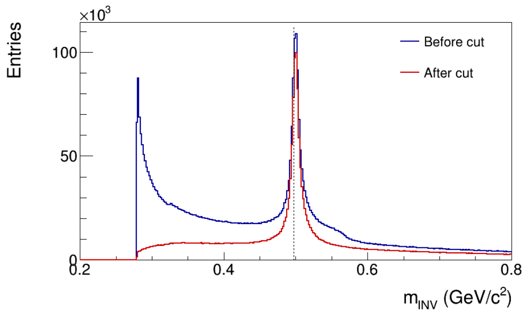
Slika 60: Histogram invarijantne mase pre (plava boja) i nakon (crvena boja) primene selekcionog kriterijuma za identifikaciju piona u intervalu \pm 3\sigma od nominalne Bete-Blohove krive.
