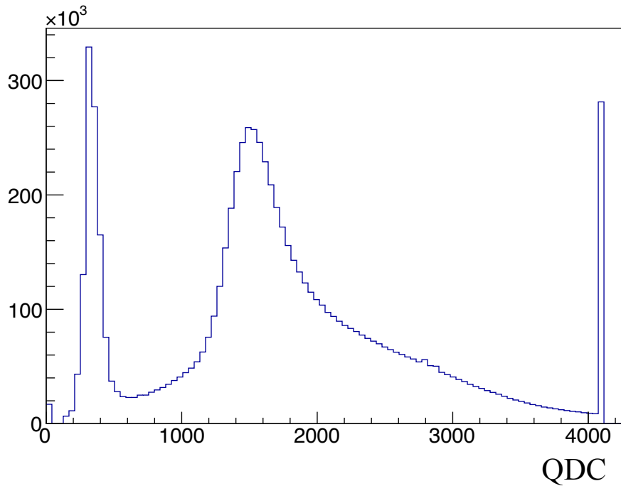
Slika 27: QDC raspodela.
