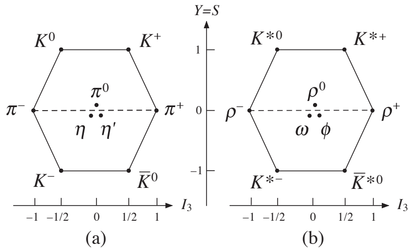
Slika 3: Pseudoskalarni (a) i vektorski (b) mezonski okteti.
