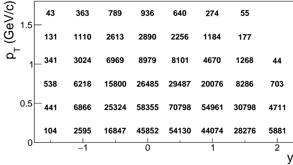
Slika 52: Nekorogovan broj K_S^0 mezona u rapiditet-transverzalni impuls binovima.
