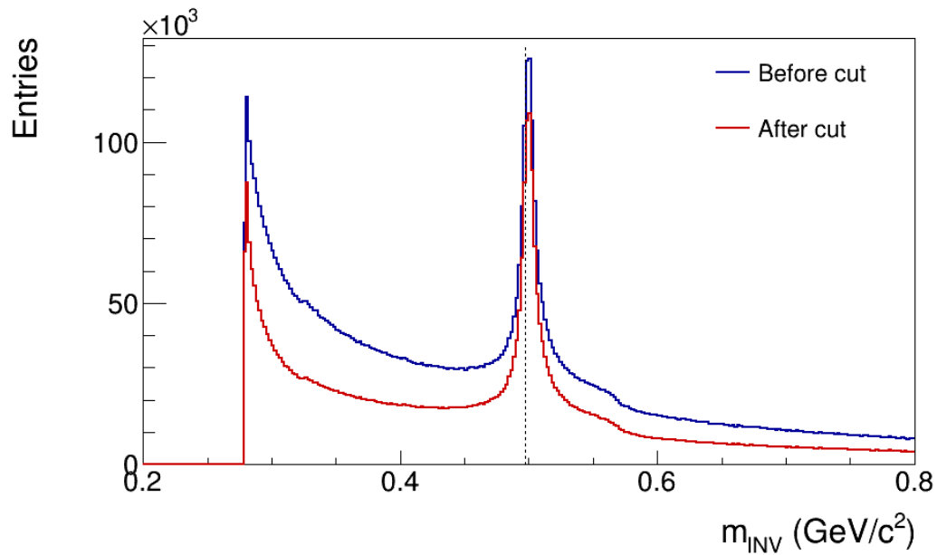
Slika 59: Histogram invarijantne mase pre (plava boja) i nakon (crvena boja) primene selekcionog kriterijuma za odstranjivanje svih sekundarnih čestica (piona) iz primarnog verteksa.
