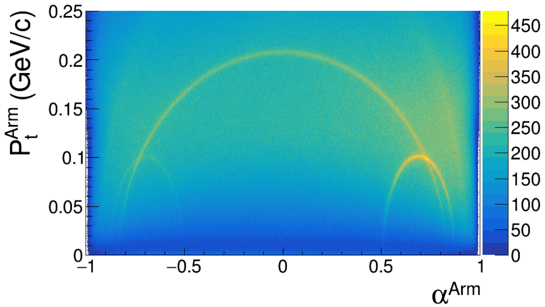
Slika 64: Armenteros-Podolanski kontrolni histogram nakon primene DCA selekcionog kriterijuma.
