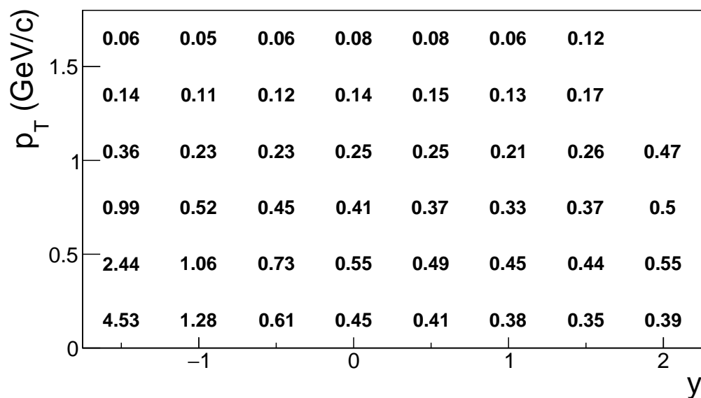
Slika 55: Statističke nesigurnosti korigovanog broja K_S^0 mezona u rapiditet-transverzalni impuls binovima, prikazano u skali \times 10^{-3} .
