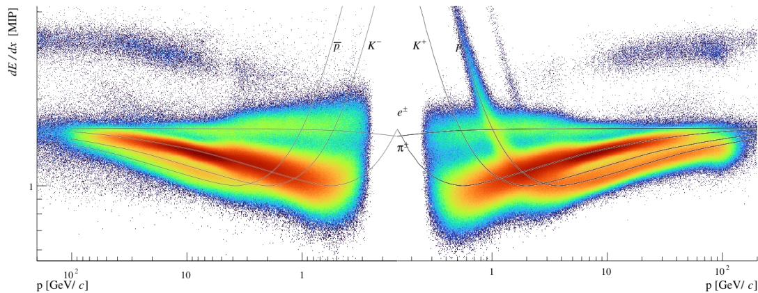
Slika 18: Na slici je prikazana deponovana energija u funkciji impulsa upadnih čestica snimljena na NA61/SHINE eksperimentu u p+p sudarima energije 158 GeV. Crnim linijama su predstavljene parametrizovane Bete-Bloch funkcije za odgovarajuće čestice (oblik funkcije elektrona odstupa od oblika ostalih čestica, videti tekst).
