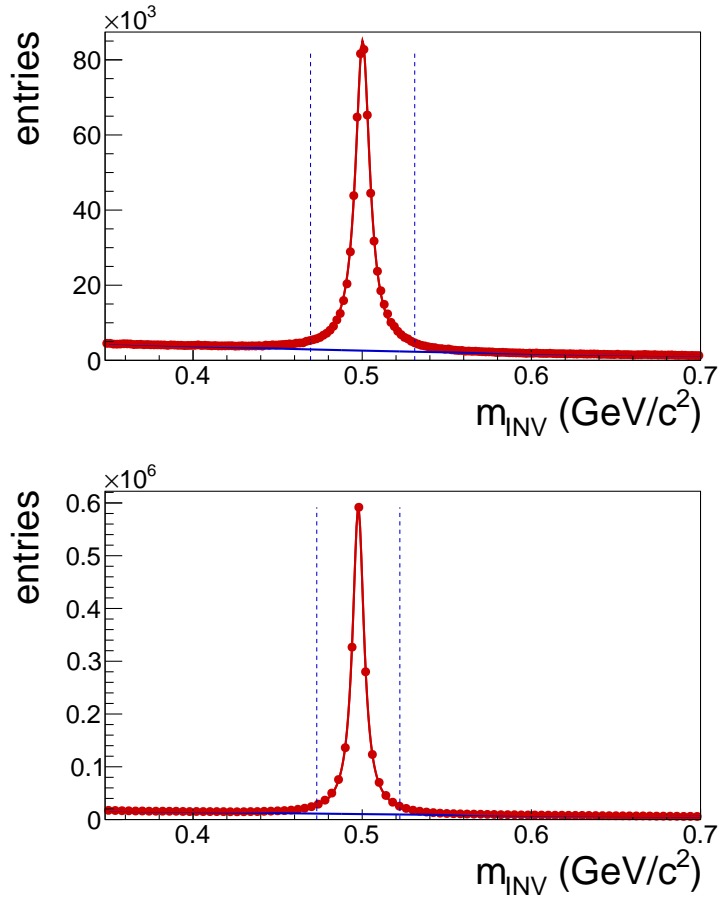
Slika 41: Raspodela invarijantne mase K_S^0 kandidata za merene podatke (gore) i simulirane podatke (dole). Crvena linija predstavlja globalnu funkciju (suma polinomijalne i Lorencove raspodele), dok plava linija odgovara fitu pozadinskog signala polinomijalnom funkcijom. Plave vertikalne linije ukazuju na interval unutar koga je vršena integracija i računat broj K_S^0 kandidata. Rezolucije dobijene iz fita su: \sigma = (0.01026 \pm 0.00002) \text{ GeV/c}^2 za eksperimentalne podatke i \sigma = (0.00819 \pm 0.00001) \text{ GeV/c}^2 za simulirane podatke.
