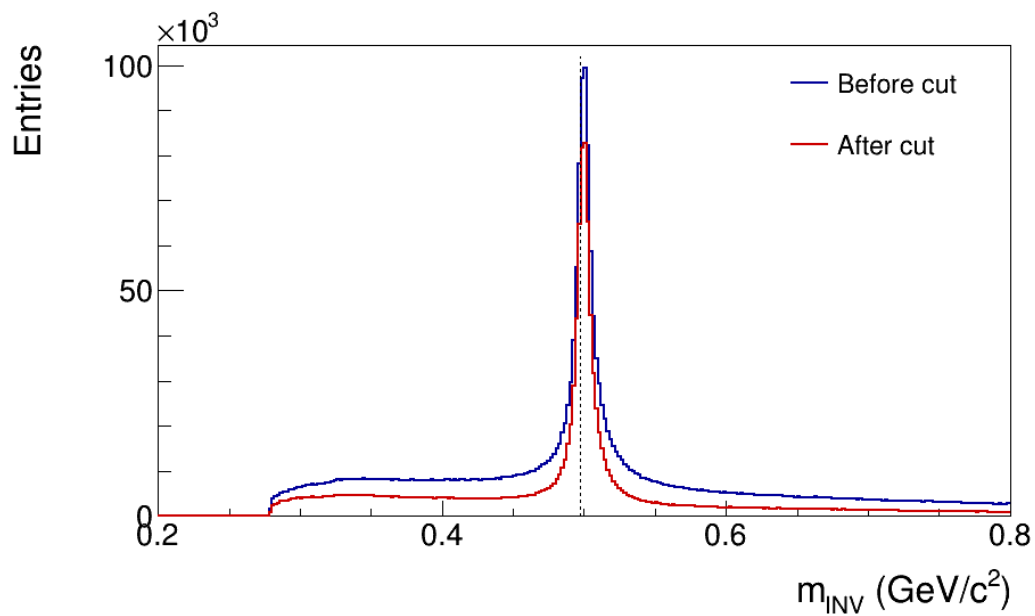
Slika 61: Histogram invarijantne mase pre (plava boja) i nakon (crvena boja) primene selekcionog kriterijuma koji se odnosi na azimutalni ugao \phi .
