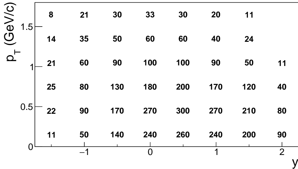
Slika 53: Statističke nesigurnosti nekorogovanog broja K_S^0 mezona u rapiditet-transverzalni impuls binovima.
