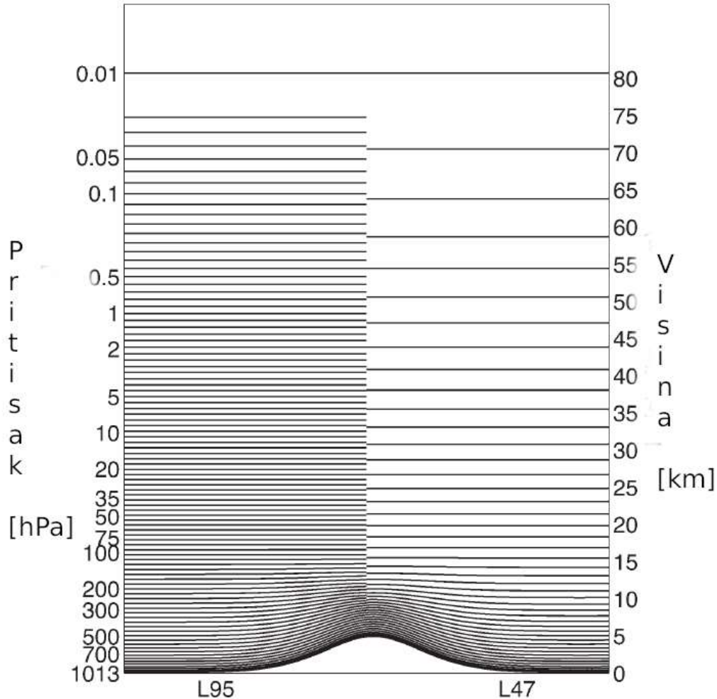
Slika p1.2 Vertikalna rezolucija ECHAM6 modela.
