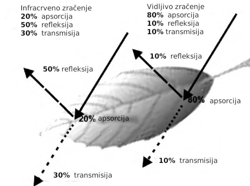
Slika p3.1 Uticaj lista na apsorpciju, refleksiju i transmittivnost zračenja (Brown i Gillespie 1995).
