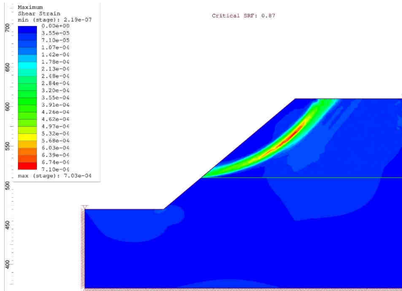
Слика 103. Резултати анализе стабилности на растојању границе од 100 m ( \alpha_z=40^\circ - без ТЗ)
