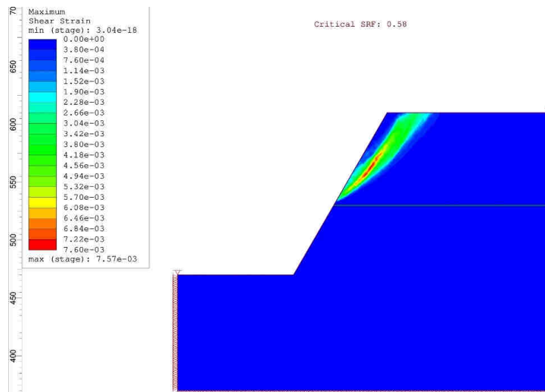
Слика 96. Резултати анализе стабилности на растојању границе од 80 m ( \alpha_z=60^\circ - без ТЗ)
