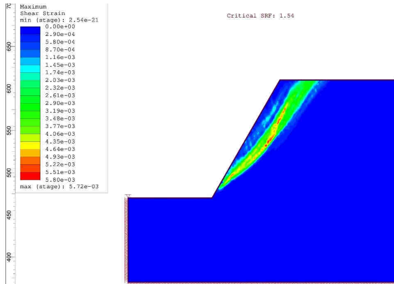
Слика 52. Резултати анализе стабилности на растојању границе од 0 m ( \alpha_z=60^\circ - без ТЗ)
