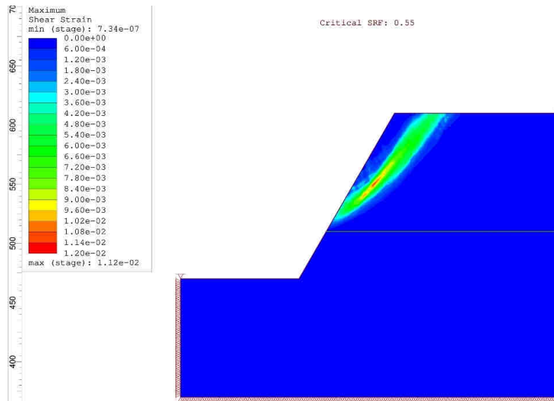
Слика 107. Резултати анализе стабилности на растојању границе од 100 m ( \alpha_z=60^\circ - без ТЗ)
