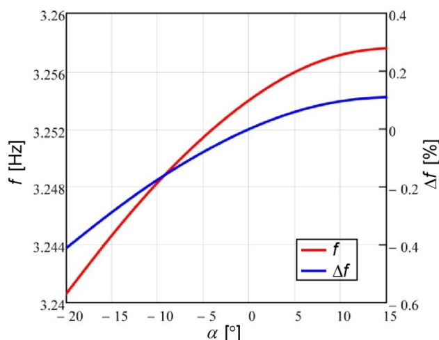
Слика 4.9 Девета сопствена фреквенција
