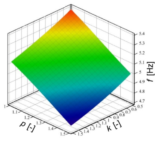
Слика 5.31 Дванаеста сопствена фреквенција
