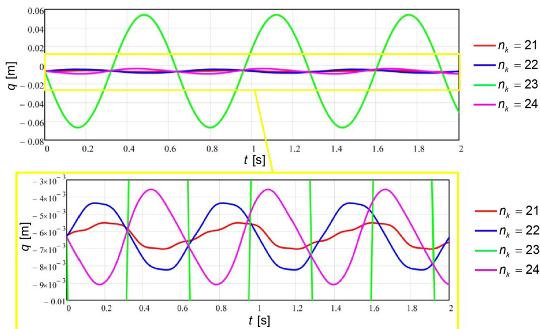
Слика 6.24 Одзив по генералисаној координати q_2 за m_{k,\max} = 6
