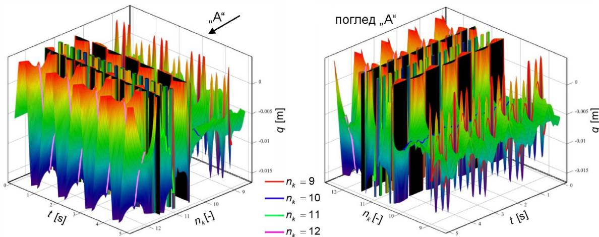
Слика 6.10 Бочно померање центра ротора за дијапазон од 8,5 до 12,5 кашика
