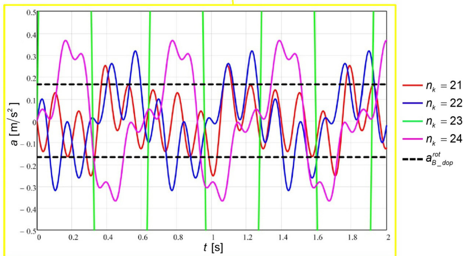
Слика 6.37 Дијаграм бочног убрзања центра ротора за n_k = 21, 22, \dots, 24
