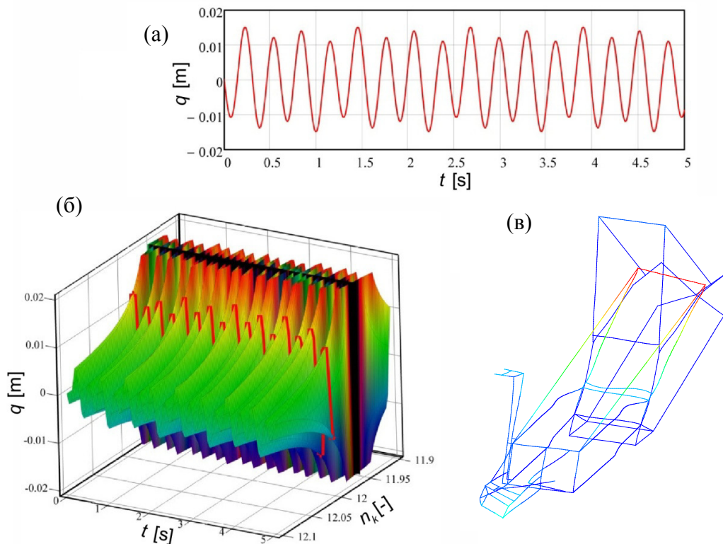
Слика 6.12 Одзив по генералисаној координати q_{38} : а) дијаграм померања за 12 кашика на ротору; б) одзив за дијапазон кашика од 11,9 до 12,1; в) девети мод осциловања
