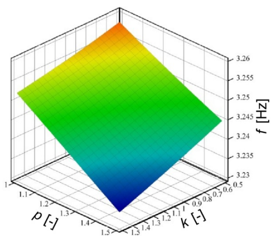
Слика 5.28 Девета сопствена фреквенција
