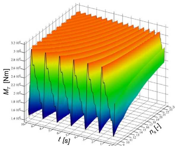
Слика 6.1 Момент копања
