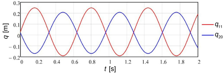
Слика 6.26 Одзив по генералисаним координатама q_{11} и q_{20} за 23 кашике на ротору Резонанца R24 има утицаја и на вертикална и бочна померања центра
