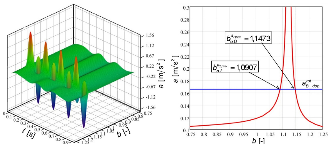
а) дијаграм генералисаног убрзања a_2 б) дијаграм максималних убрзања Слика 5.11 Бочно убрзање центра ротора
