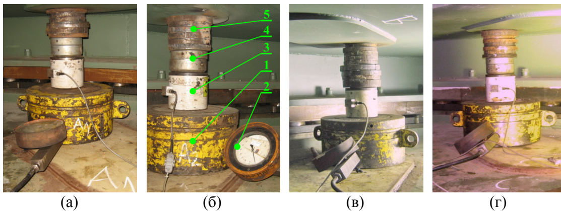
Слика 2.12 Мерна места (1 – хидро цилиндар, 2 – манометар, 3 – динамометар, 4 – калота, 5 – компензационе плоче): (а) мерно место A_1 ; (б) мерно место A_2 ; (в) мерно место B ; (г) мерно место C [59]
