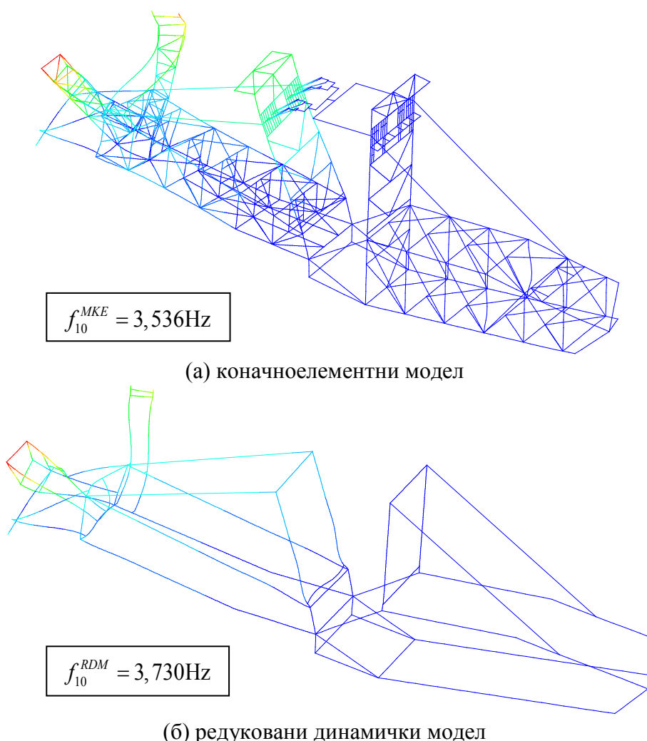
Слика 3.20 Десети облик осциловања
