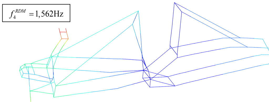
(б) редуковани динамички модел Слика 3.14 Четврти облик осциловања
