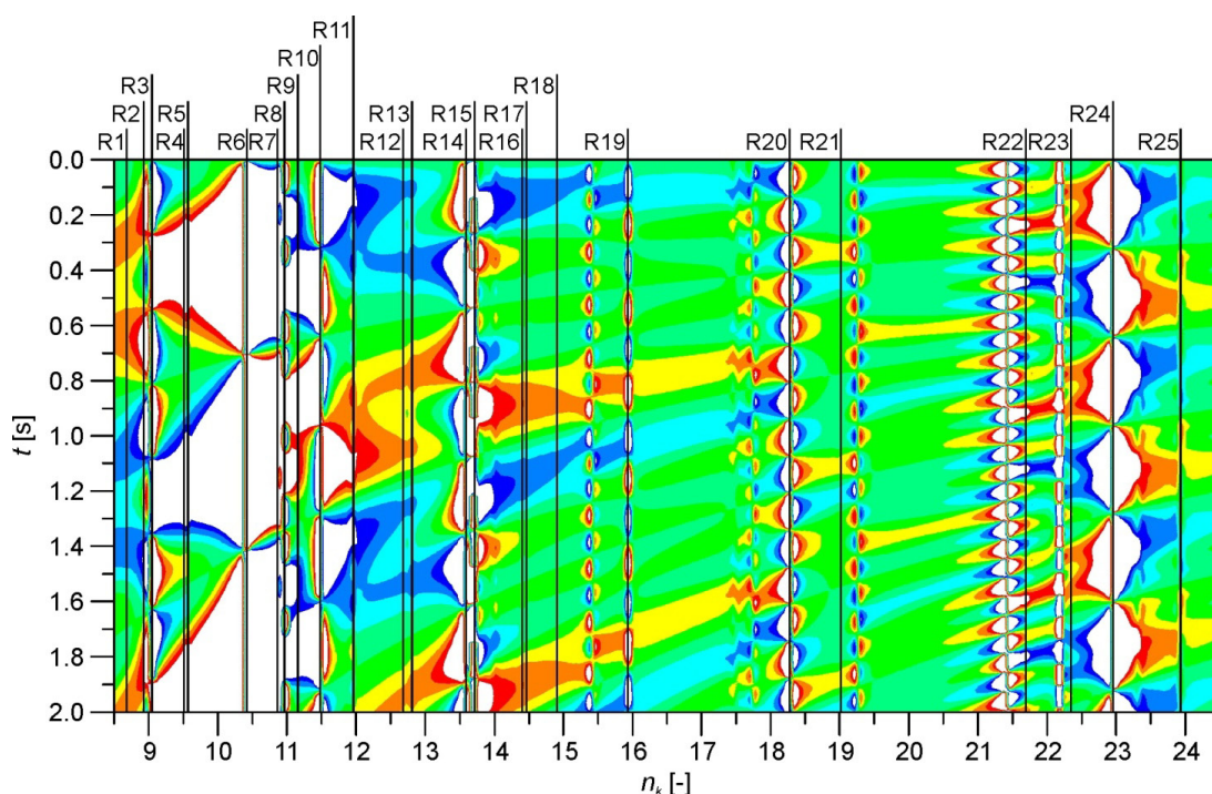
Слика 6.38 Вертикална убрзања центра ротора за дијапазон од 8,5 до 24,5 кашика
