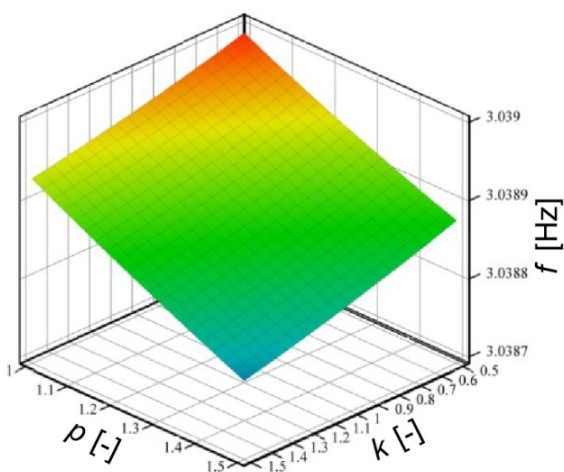
Слика 5.27 Осма сопствена фреквенција
