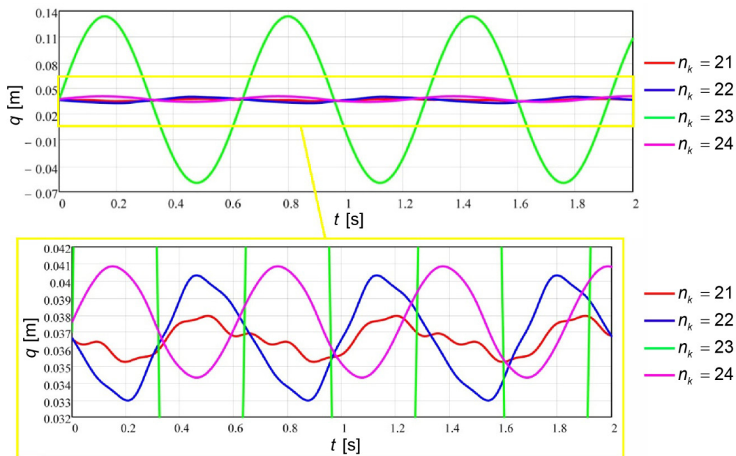
Слика 6.23 Одзив по генералисаној координати q_1 за m_{k,\max} = 6
