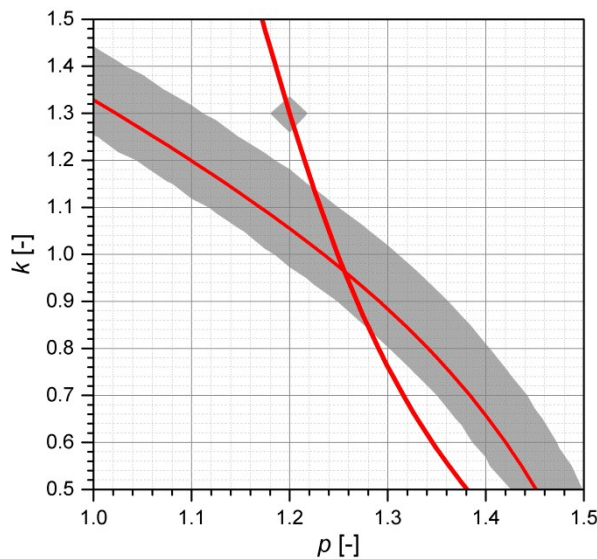
б) зоне убрзања тежишта противтега (беле области: a_{55,max} \leq 0,4 \text{ m/s}^2 )
