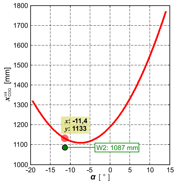
Слика 2.17 Упоредни приказ апсциса тежишта горње градње добијених на основу коригованог 3D модела и другог вагања (маса противтега m_{CW2} = 231,997 \text{ t} ) [59]
