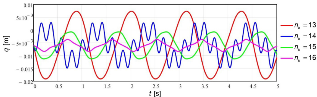
Слика 6.14 Одзив по генералисаној координати q_2 за m_{k,\max} = 4
