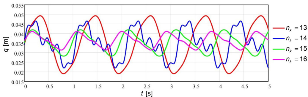
Слика 6.13 Одзив по генералисаној координати q_1 за m_{k,\max} = 4
