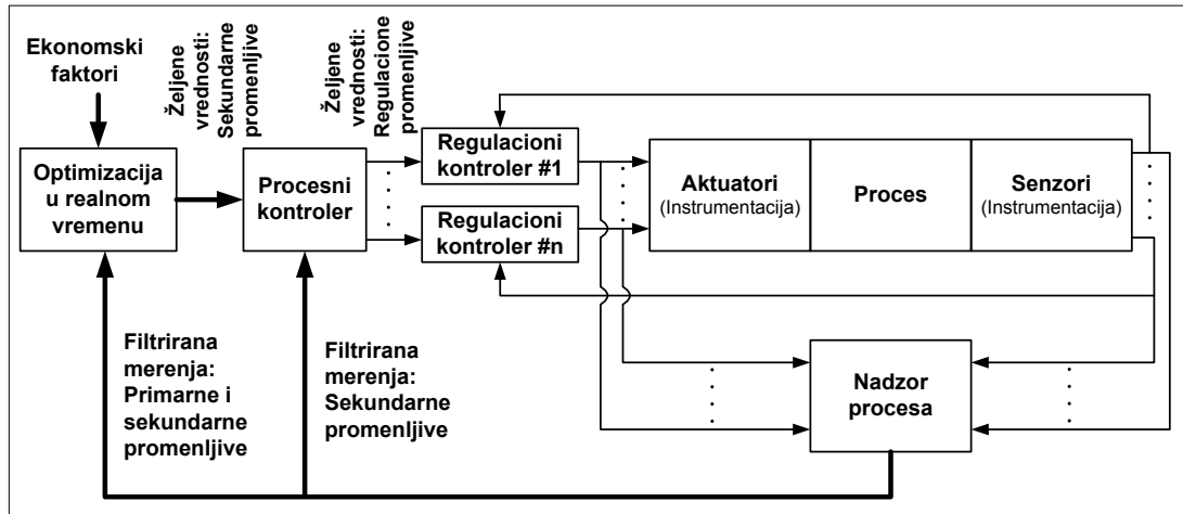
Slika 45. Kontrolna hijerarhija u upravljanju procesima pripreme mineralnih sirovina [Del Villar et al. (2010)].
