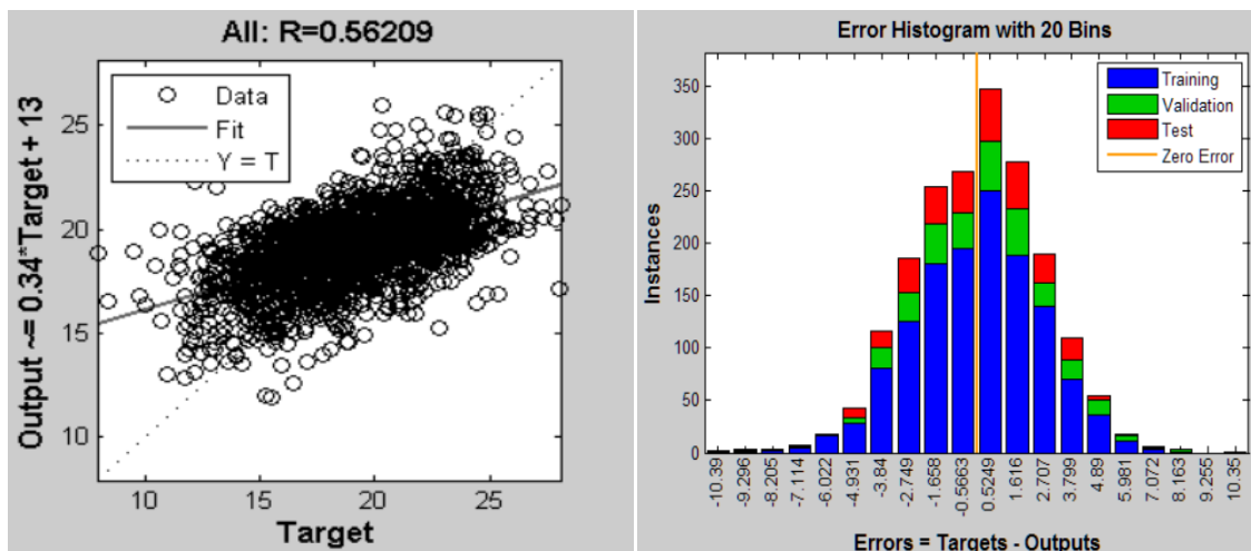
Slika 103. Grafički prikaz rezultata VNM1 modela sa histogramom greške treniranja, validacije i testiranja.
