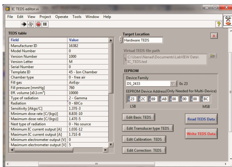
Slika 5.23. Grafički korisnički interfejs TEDS editor programa za upis parametara jonizacione komore M1000
