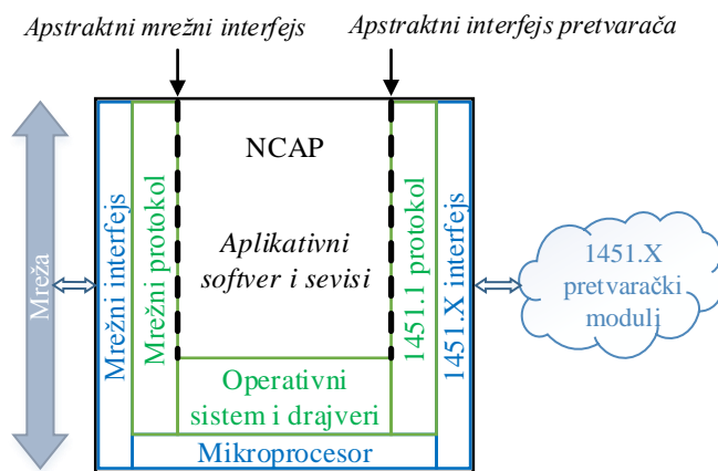
Slika 4.1. Model mrežnog procesora prema IEEE 1451.1 standardu
