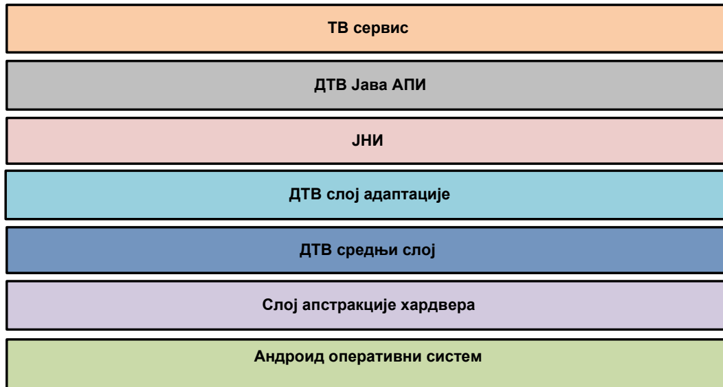
Слика 3.13 Позиција компоненте „ТВ сервис“ у оквиру софтверског стека на Андроид уређајима са интегрисаном дигиталном телевизијом
