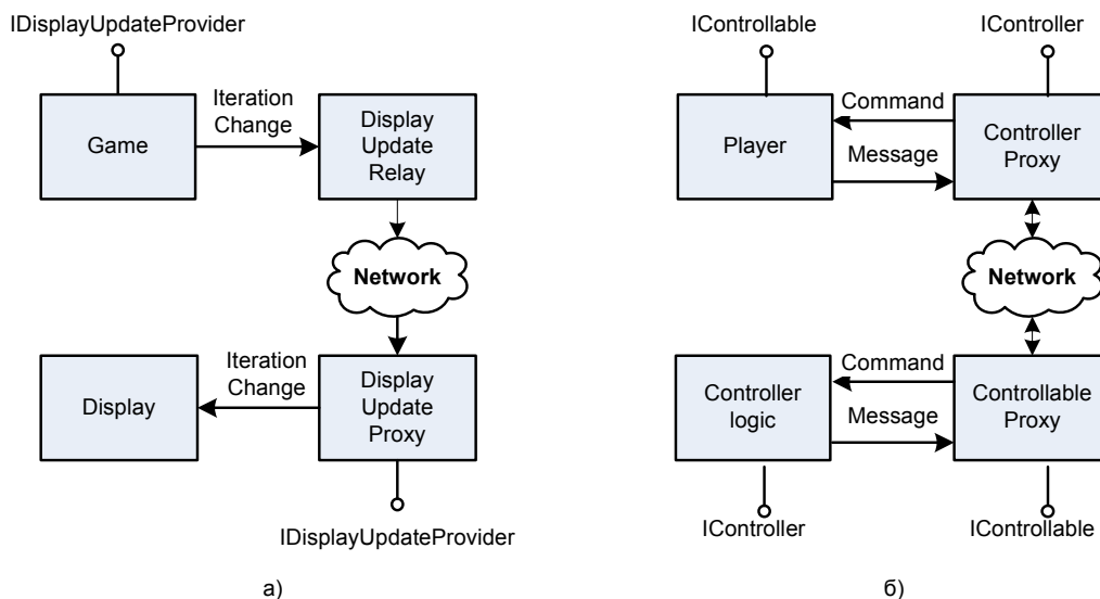
Слика 3.21a) Размена информација између објекта Game и компоненте „Приказ“ б) Размена информација између објекта Player и логике контролера
