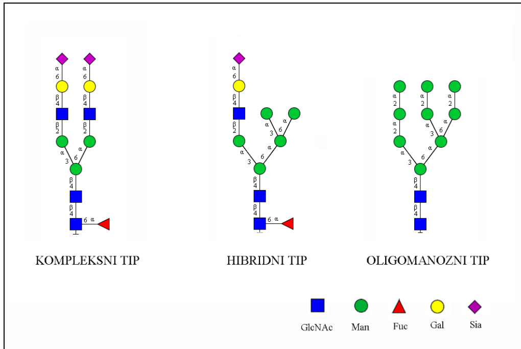
Slika 2. Tipovi N-glikana. GlcNAc: N-acetilglukozamin; Man: manoza; Fuc: fukoza; Gal: galaktoza; Sia: sijalinska kiselina. (Izvor: modifikovano prema: Stanley i sar., 2009 )
